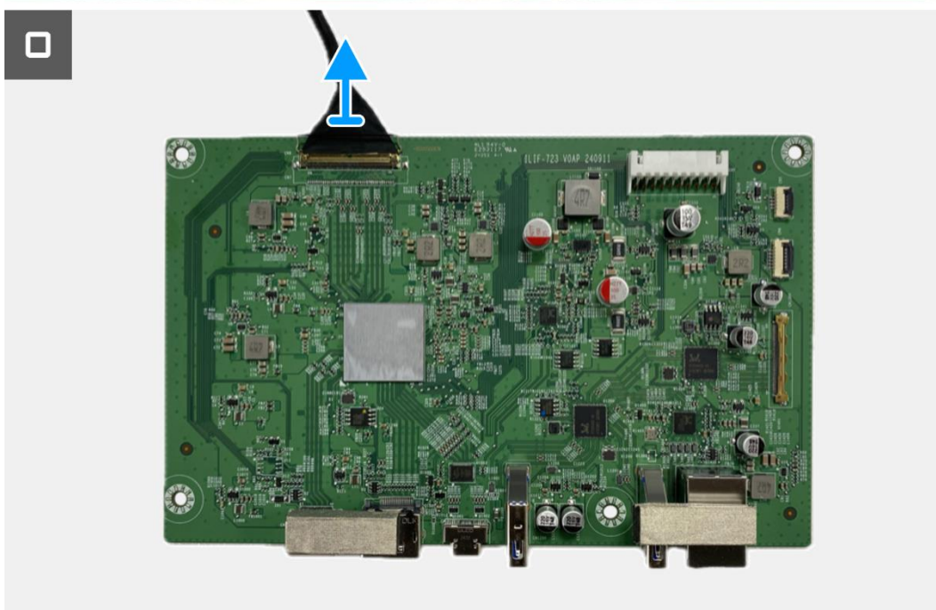
Imagen 98. Extracción de la placa de la interfaz
