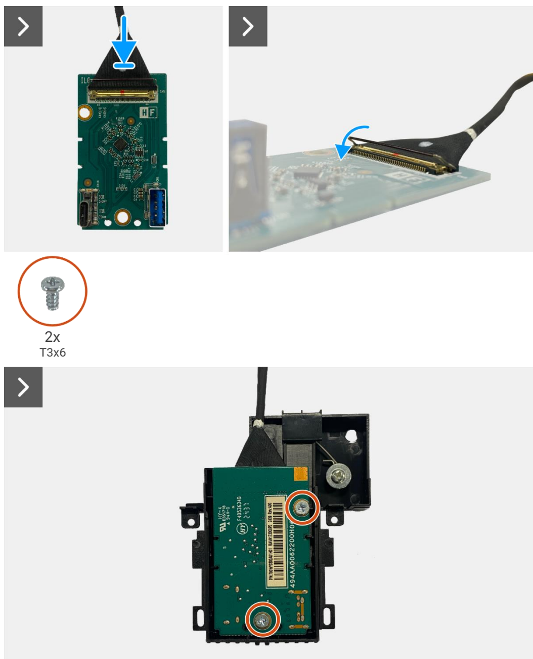
Rysunek 73. Instalowanie płytki QAP
