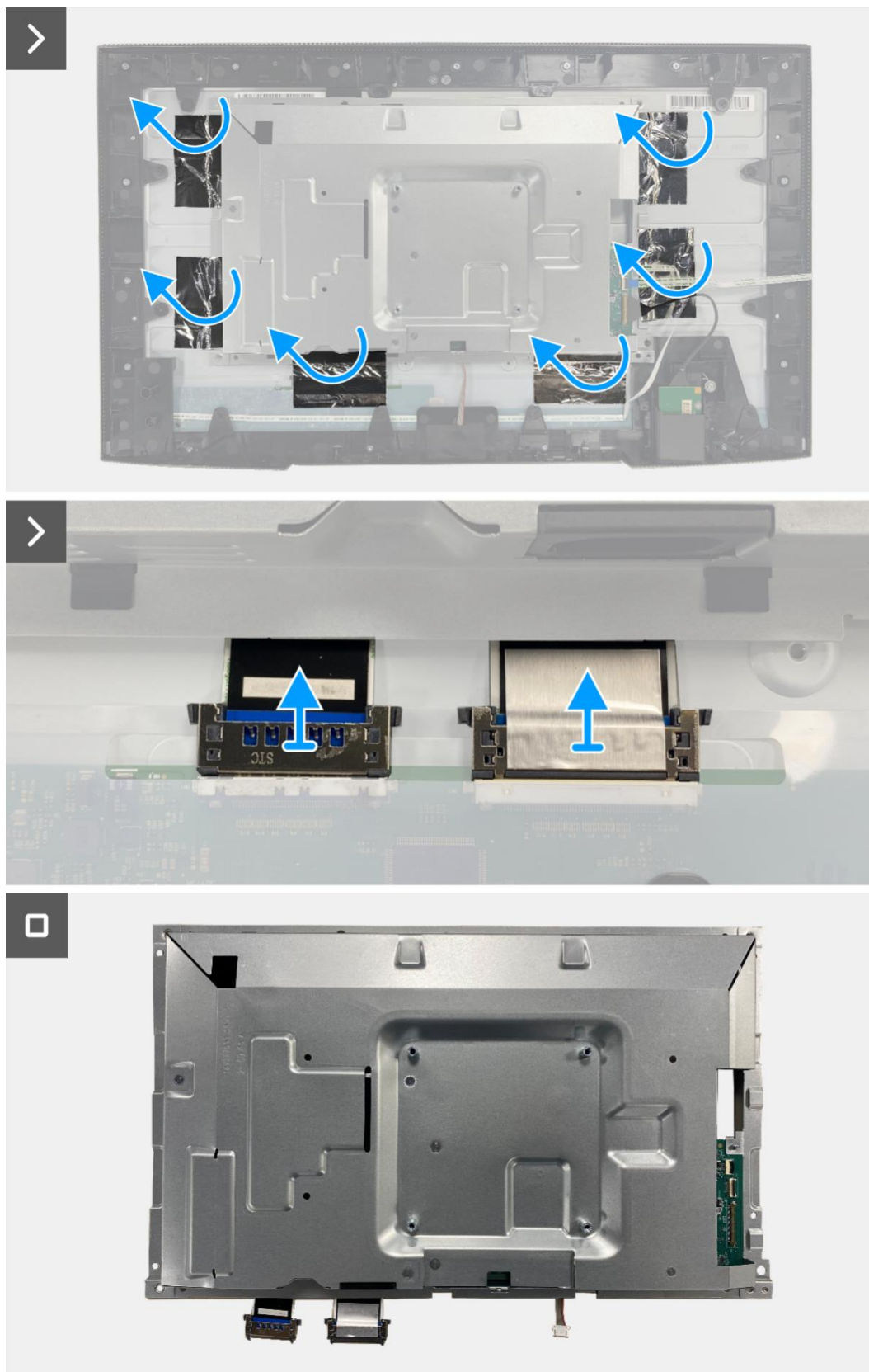
Rysunek 16. Demontaż zespołu obudowy
