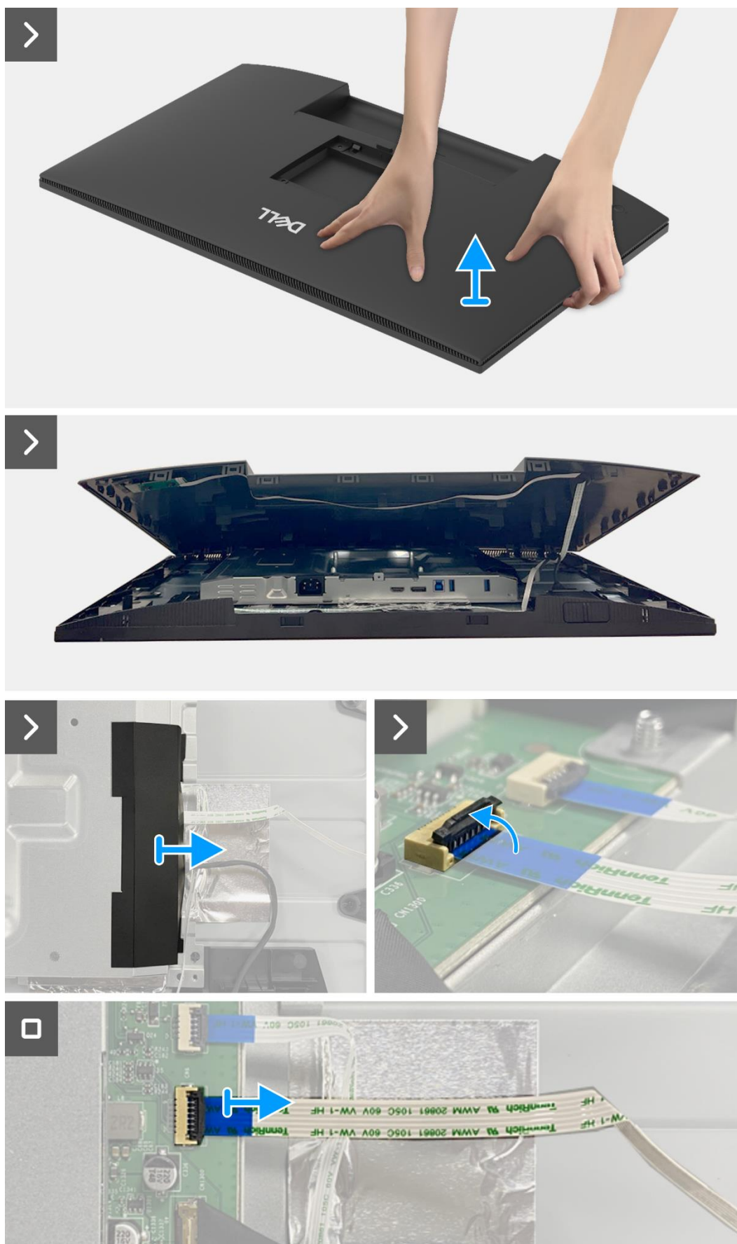
Rysunek 36. Zdejmowanie tylnej pokrywy
