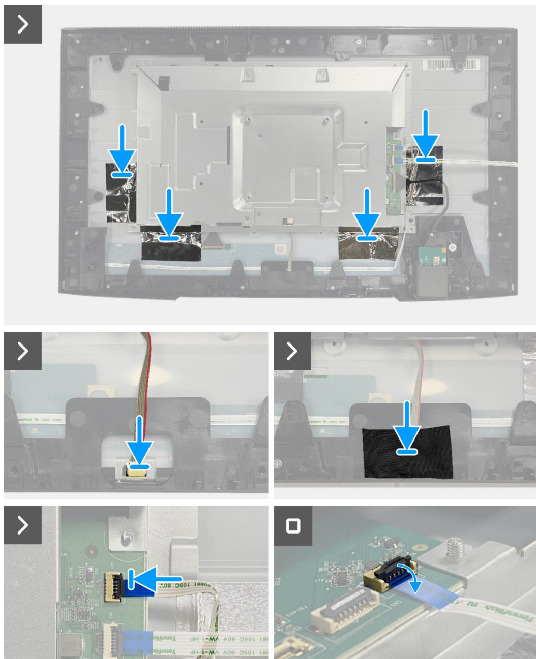
Rysunek 78. Instalowanie zespołu obudowy
