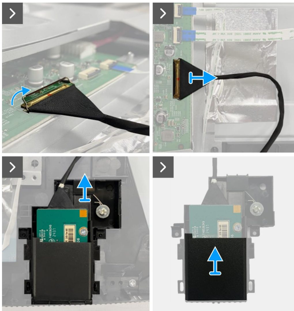
Rysunek 11. Wyjmowanie płytki QAP
