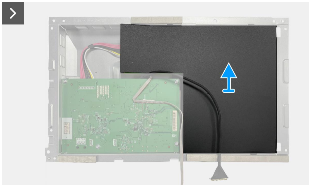
Rysunek 79. Wyjmowanie karty interfejsu
