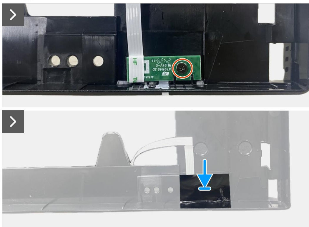
Rysunek 59. Instalowanie płytki LED
