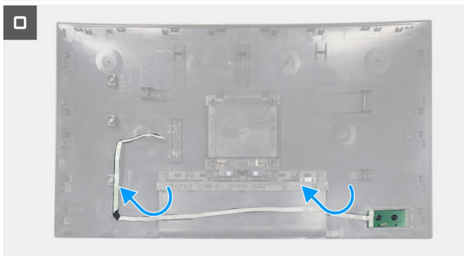
Rysunek 39. Wyjmowanie płytki klawiatury
