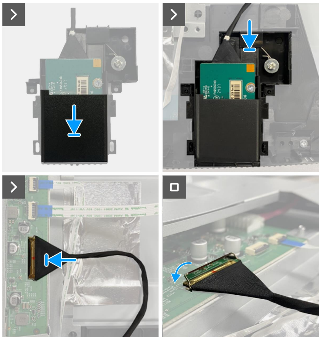
Rysunek 74. Instalowanie płytki QAP
