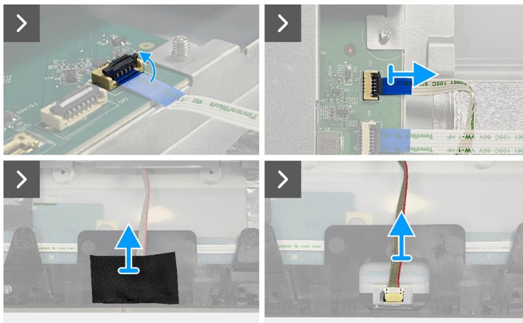
Rysunek 45. Demontaż zespołu obudowy
