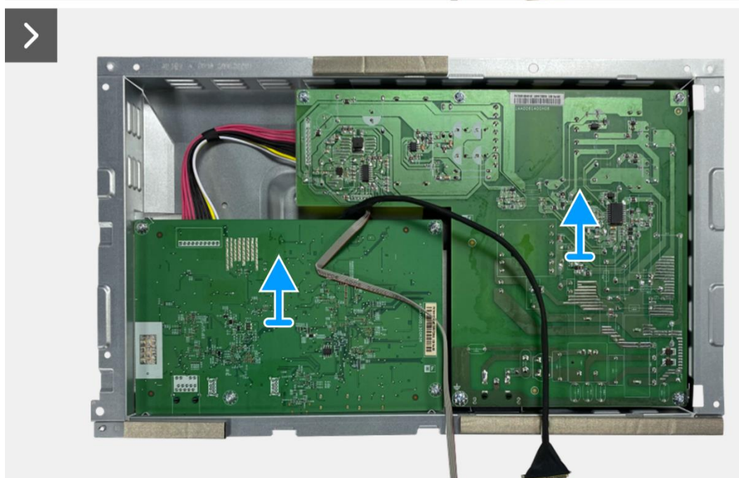
Rysunek 80. Wyjmowanie karty interfejsu
