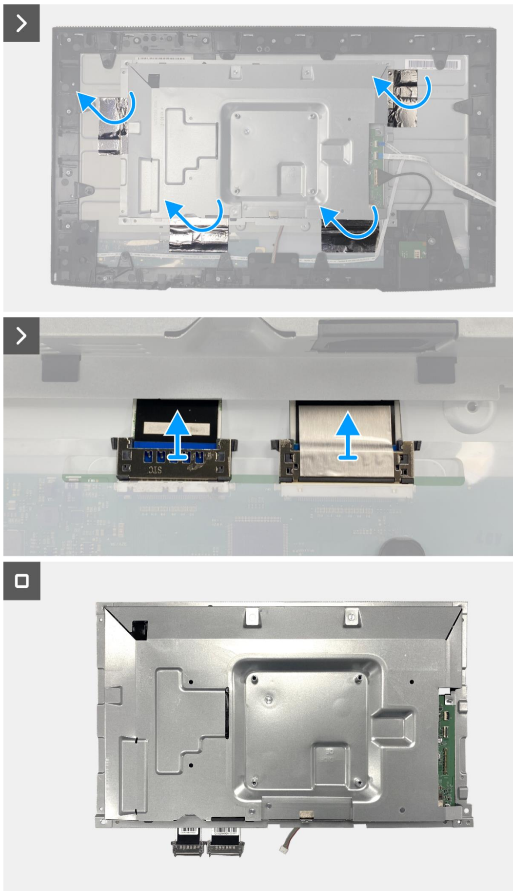
Rysunek 46. Demontaż zespołu obudowy
