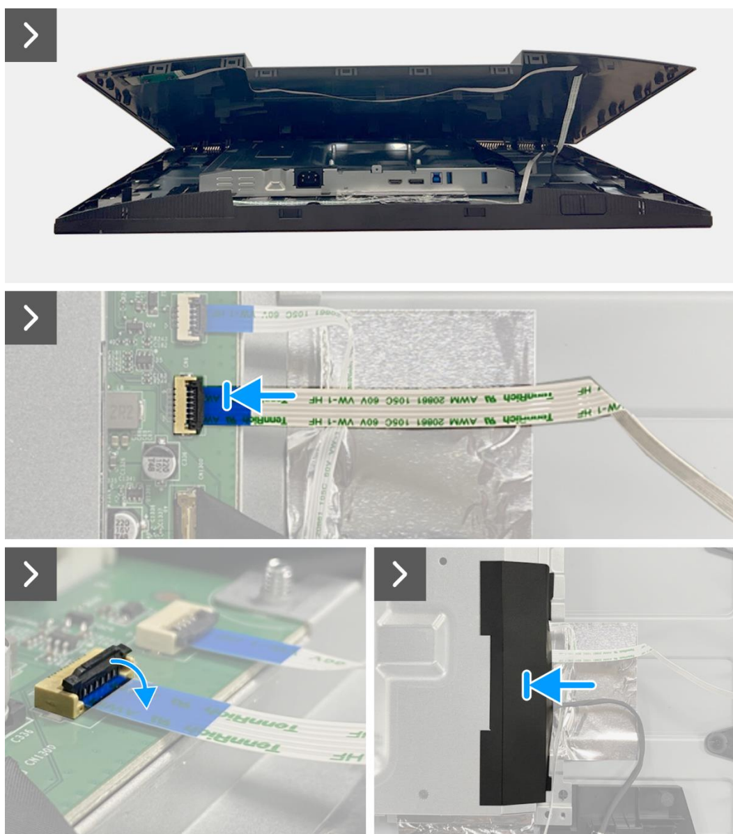
Rysunek 37. Instalowanie tylnej pokrywy
