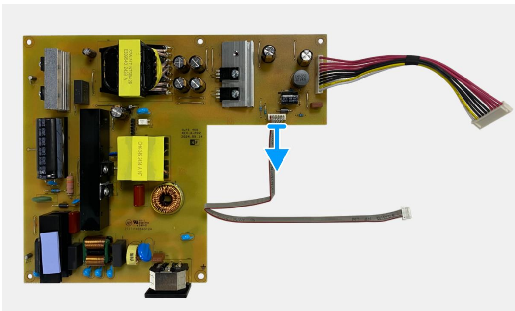
Rysunek 55. Wyjmowanie płyty zasilania
