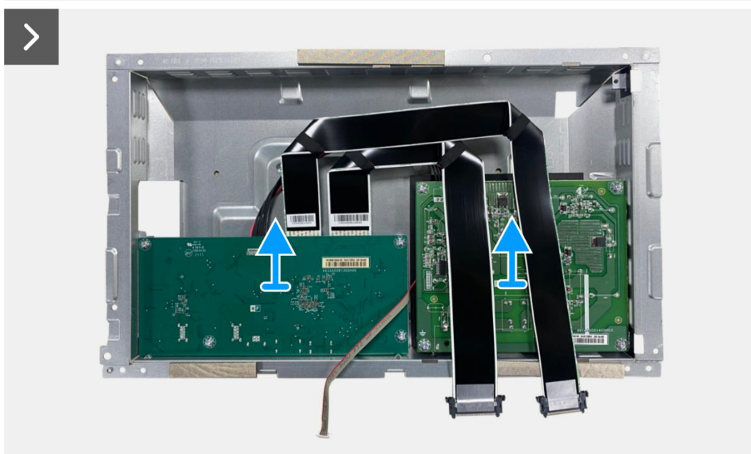
Rysunek 20. Wyjmowanie karty interfejsu
