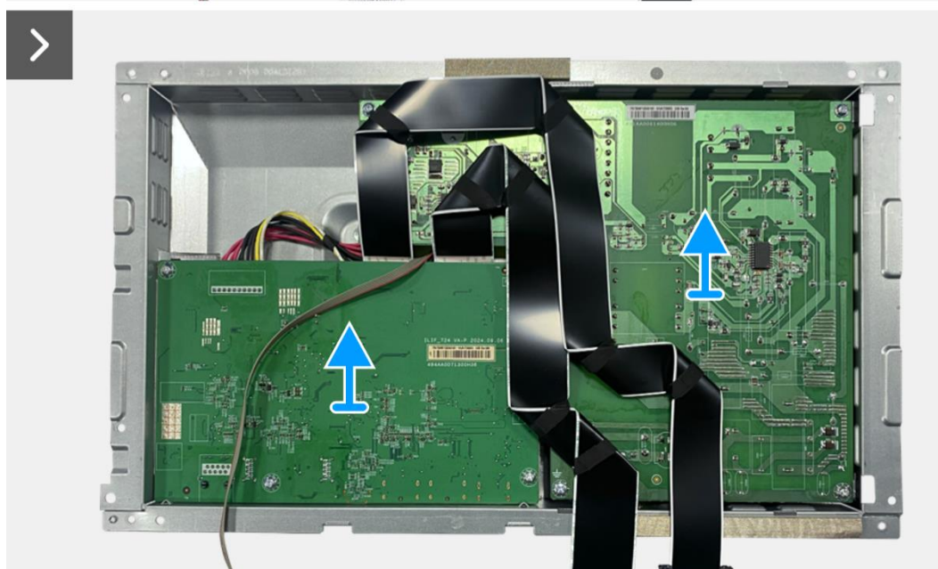
Rysunek 50. Wyjmowanie karty interfejsu
