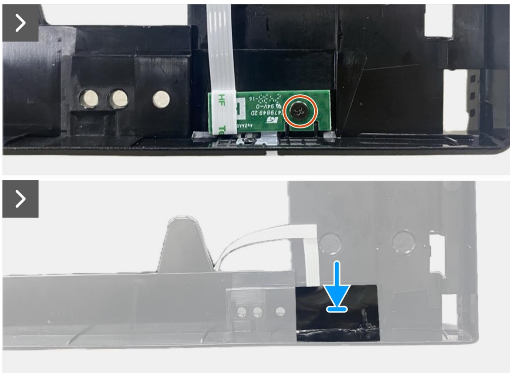
Rysunek 29. Instalowanie płytki LED
