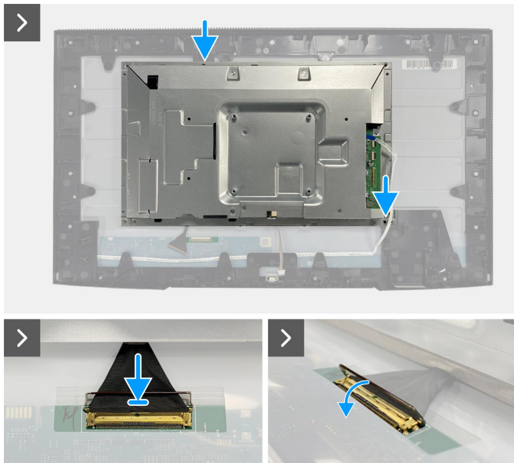
Rysunek 77. Instalowanie zespołu obudowy
