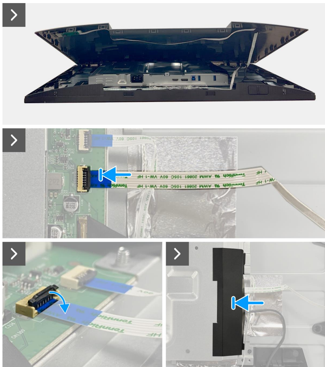
Rysunek 67. Instalowanie tylnej pokrywy
