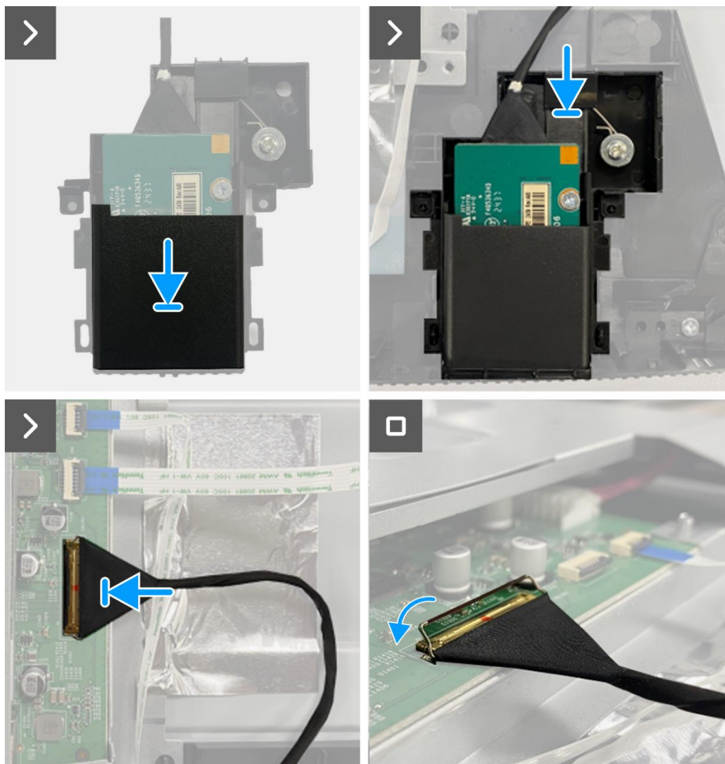
Rysunek 14. Instalowanie płytki QAP
