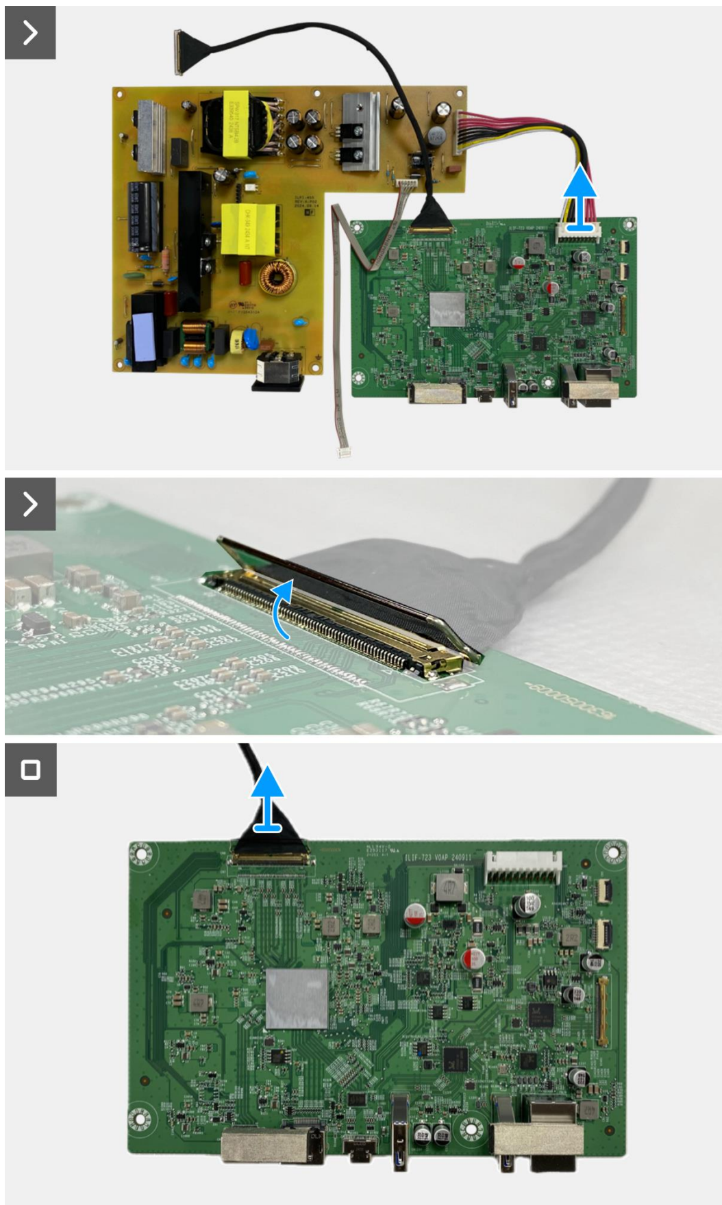
Rysunek 81. Wyjmowanie karty interfejsu
