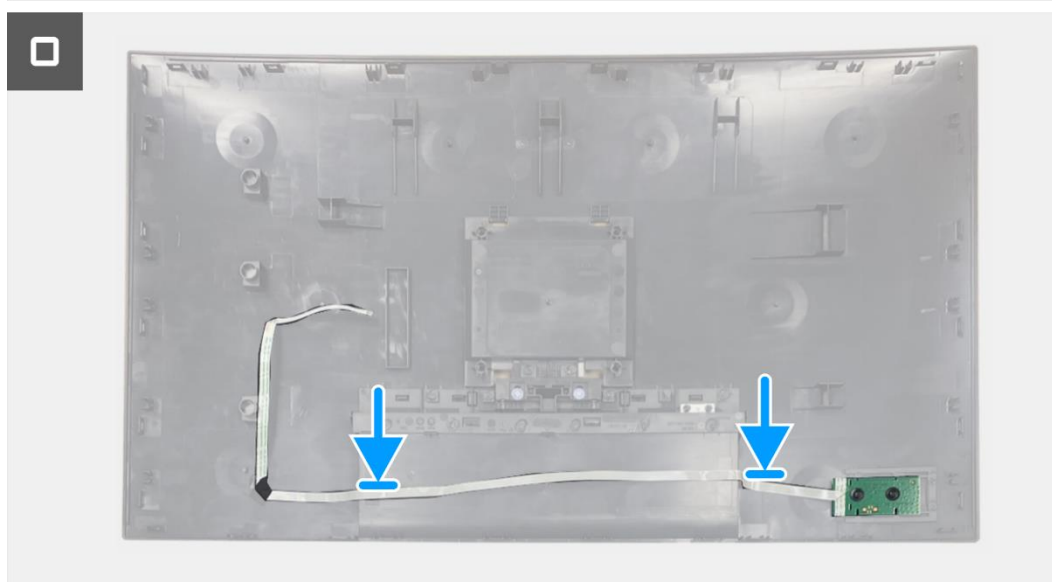
Rysunek 10. Instalowanie płytki klawiatury
