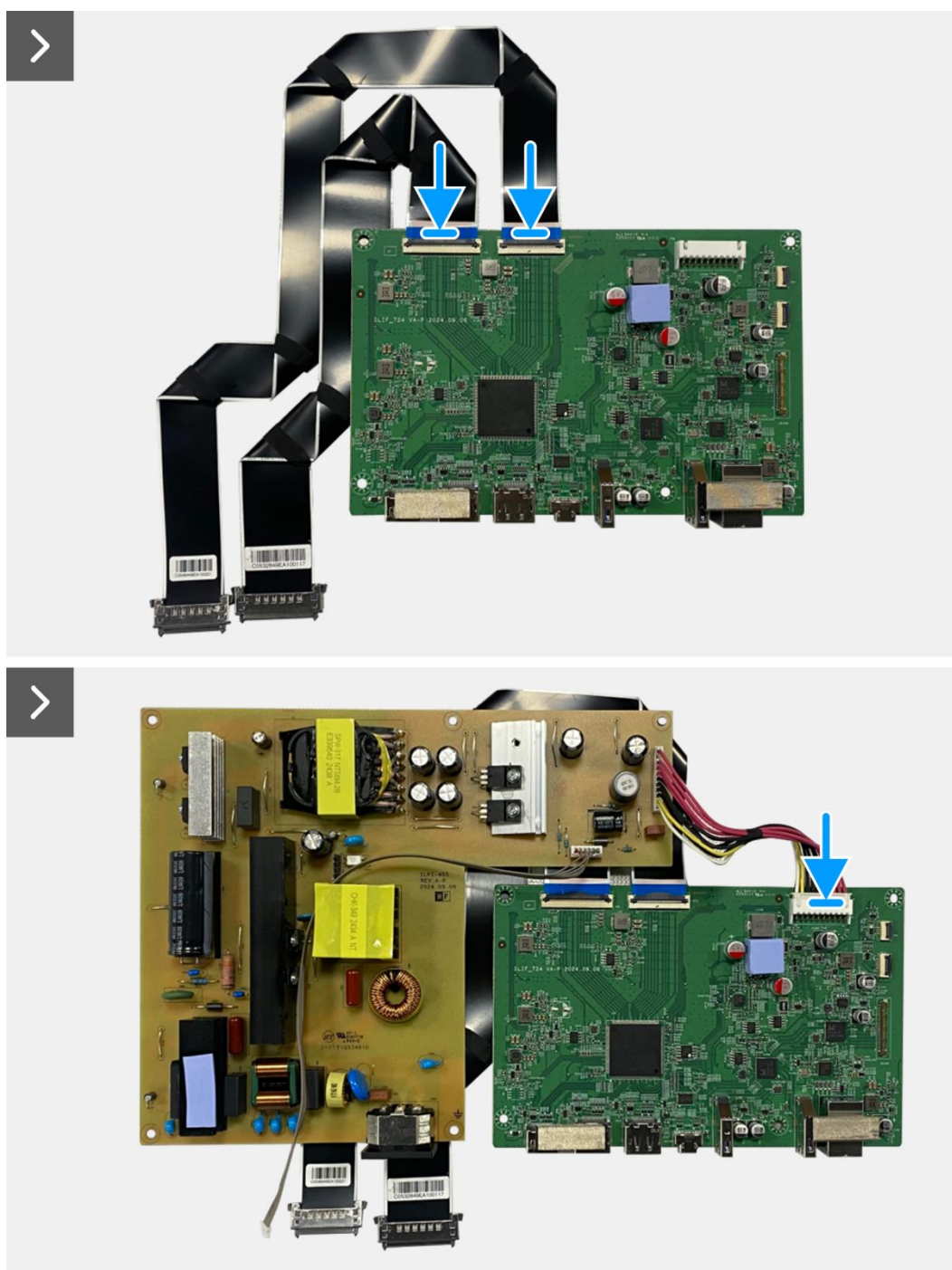
Rysunek 52. Instalacja karty interfejsu
