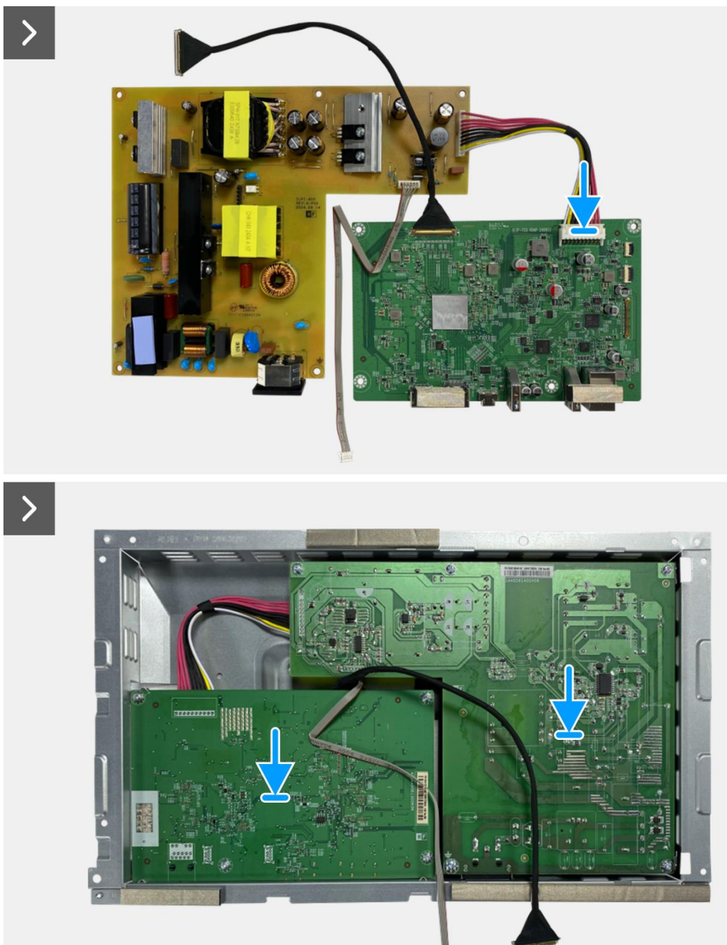
Rysunek 83. Instalacja karty interfejsu
