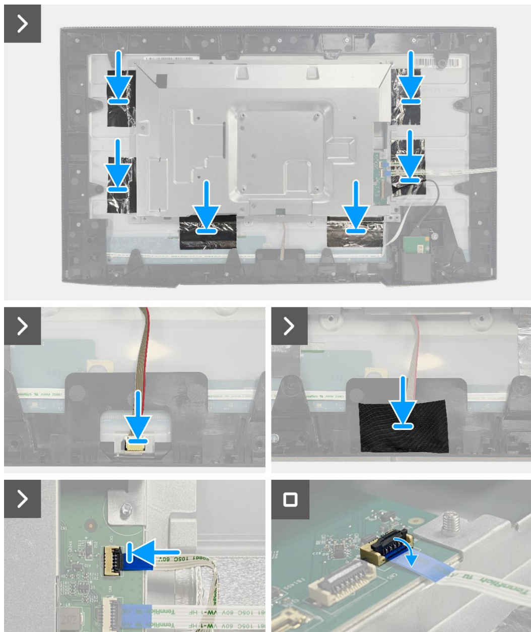
Obrázek 18. Instalace sestavy šasi
