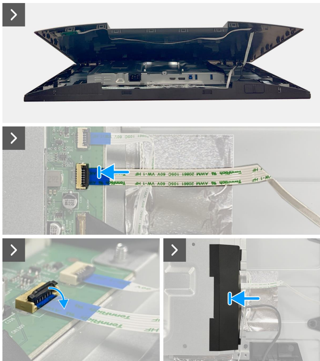
Obrázek 67. Instalace zadního krytu
