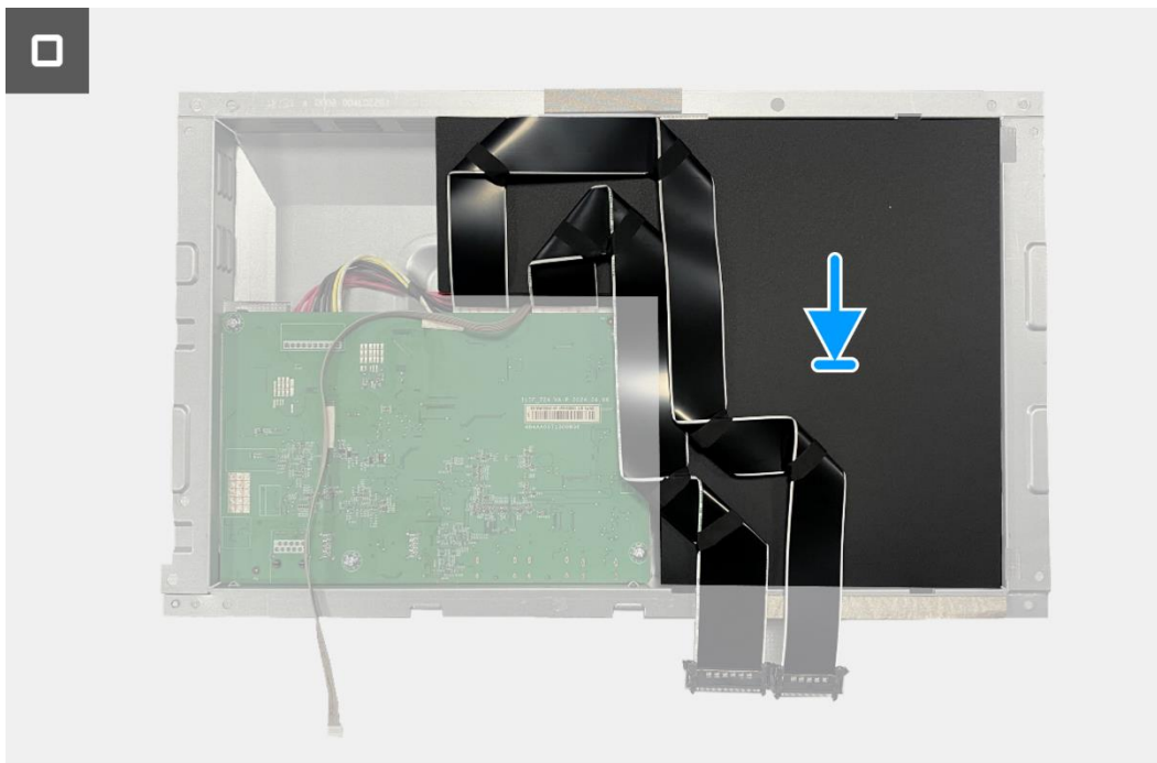
Obrázek 54. Instalace desky rozhraní
