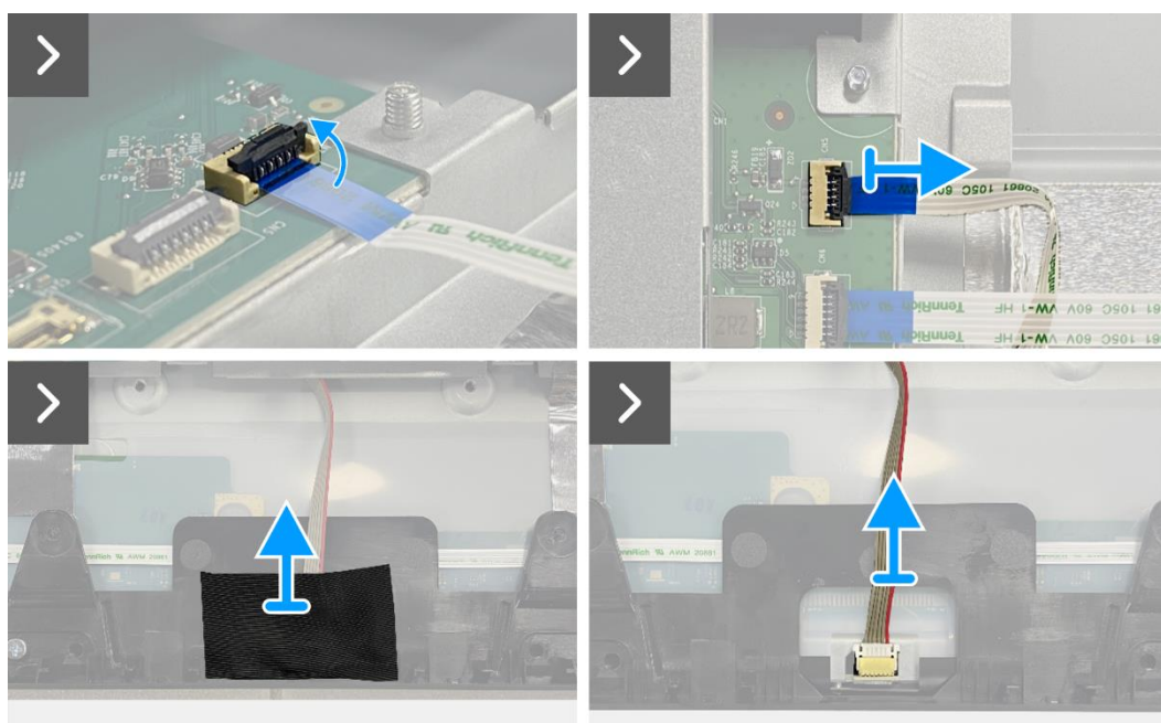
Obrázek 45. Odmontování sestavy šasi
