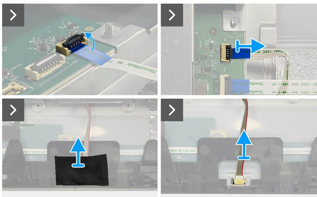
Obrázek 15. Odmontování sestavy šasi
