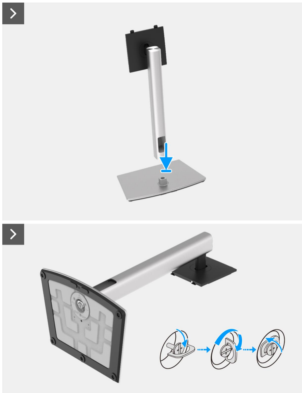
Obrázek 3. Instalace stojanu
