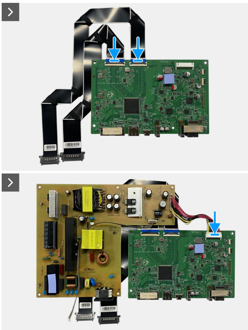
Obrázek 52. Instalace desky rozhraní
