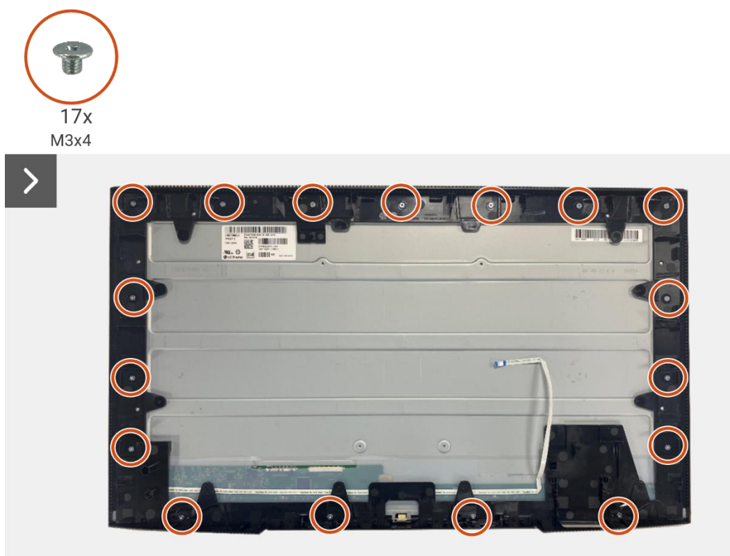
Obrázek 87. Odmontování desky LED
