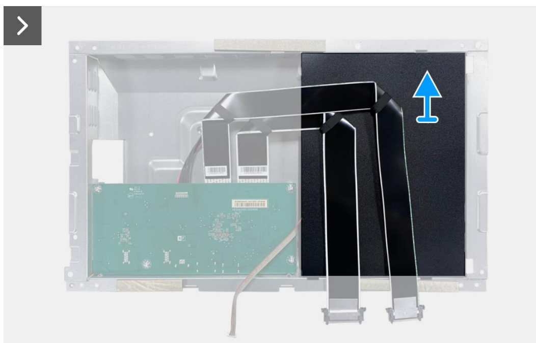
Obrázek 19. Odmontování desky rozhraní
