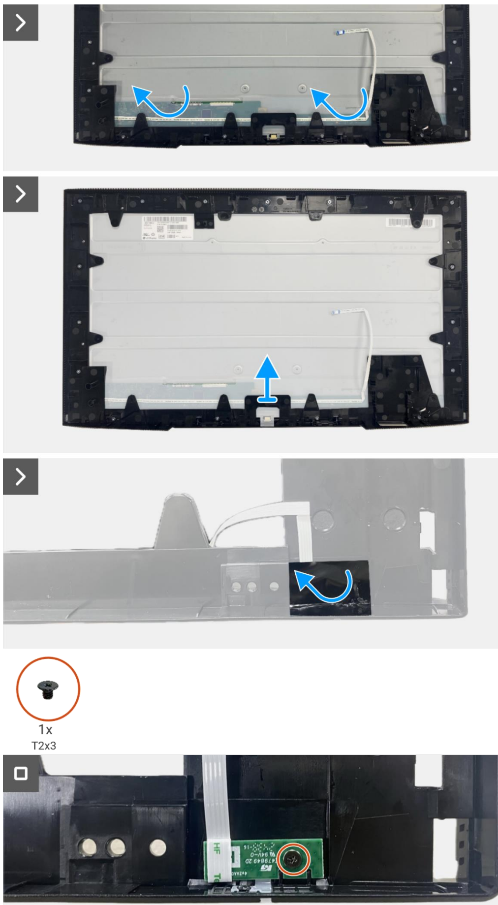
Obrázek 28. Odmontování desky LED
