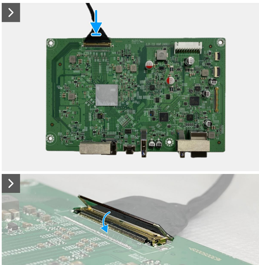
Obrázek 82. Instalace desky rozhraní
