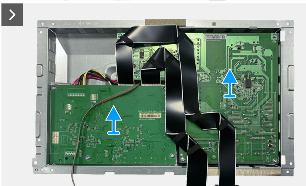
Obrázek 50. Odmontování desky rozhraní
