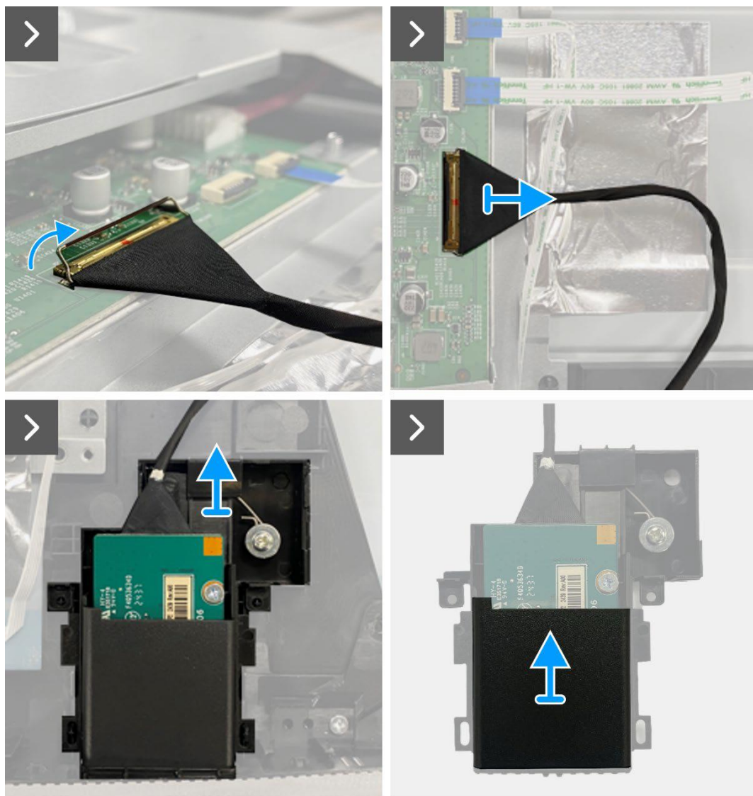
Obrázek 11. Odmontování desky QAP
