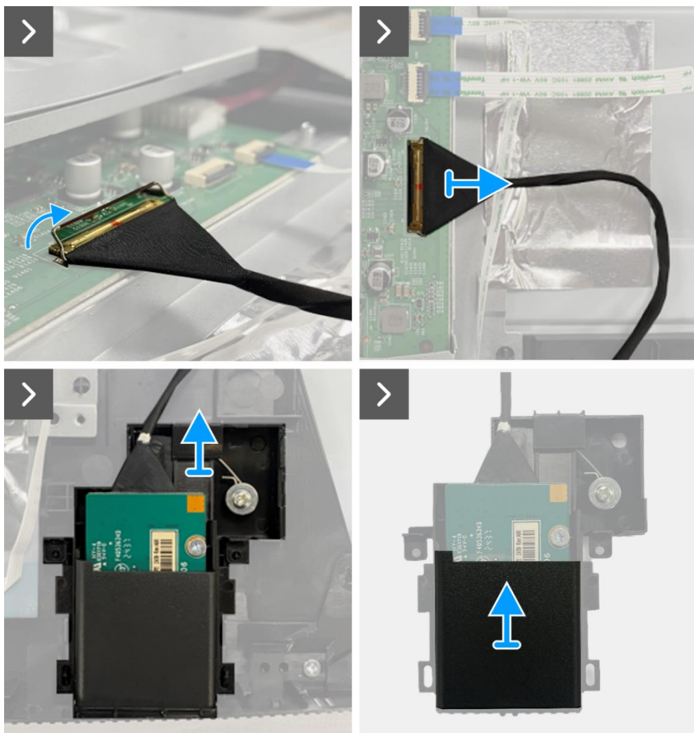
Obrázek 71. Odmontování desky QAP
