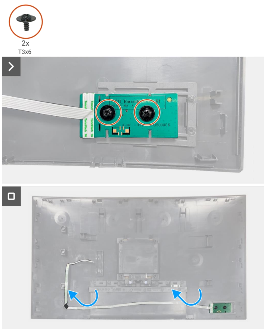
Obrázek 69. Odmontování desky klávesnice
