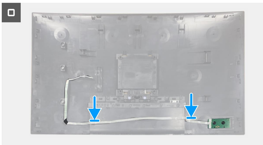
Obrázek 40. Instalace desky klávesnice
