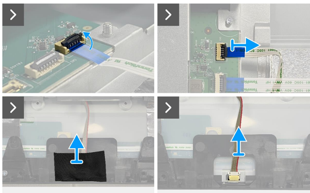
Obrázek 75. Odmontování sestavy šasi
