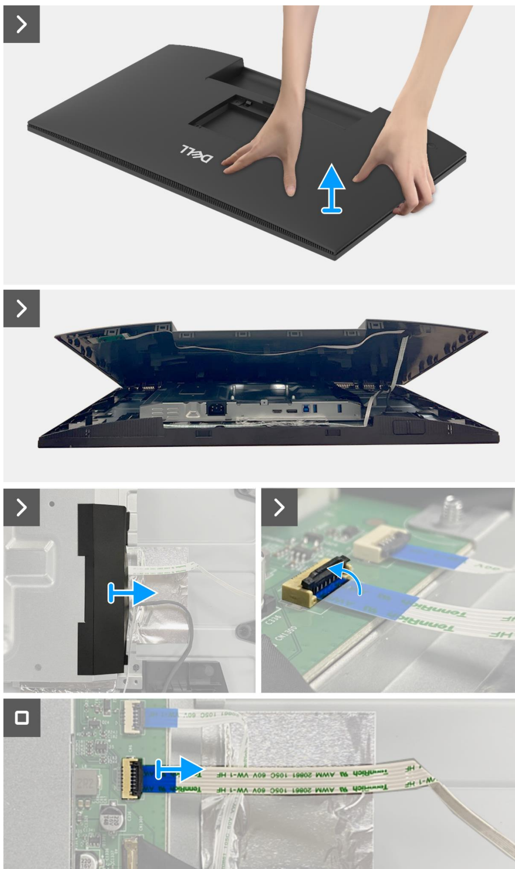
Obrázek 36. Odmontování zadního krytu
