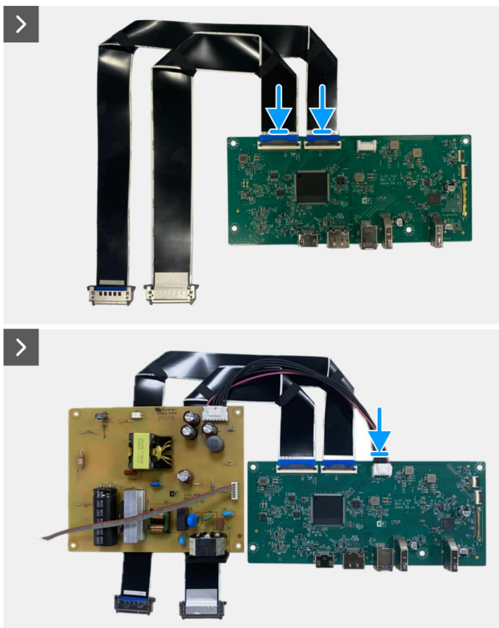
Obrázek 22. Instalace desky rozhraní
