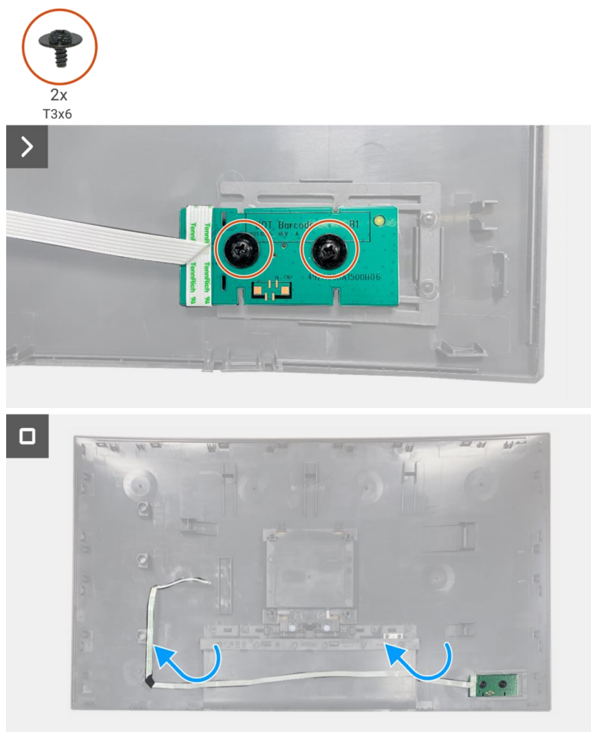
Obrázek 9. Odmontování desky klávesnice
