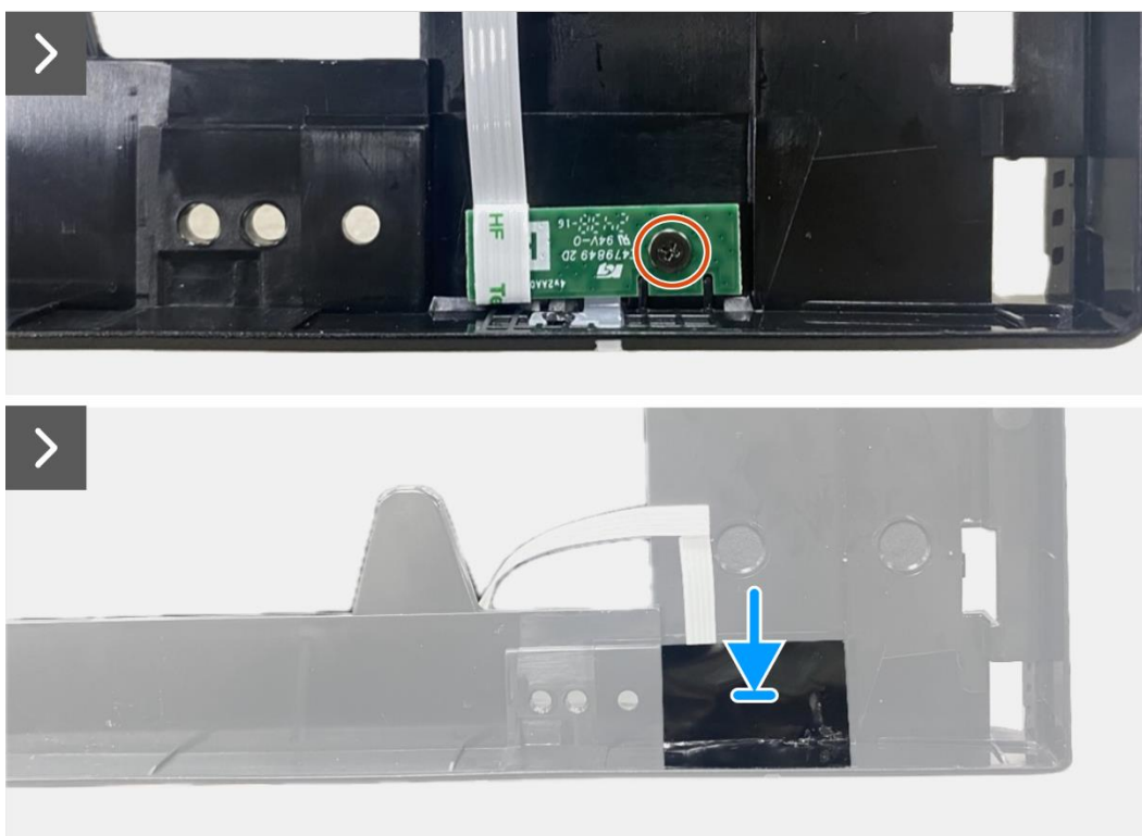
Obrázek 29. Instalace desky LED
