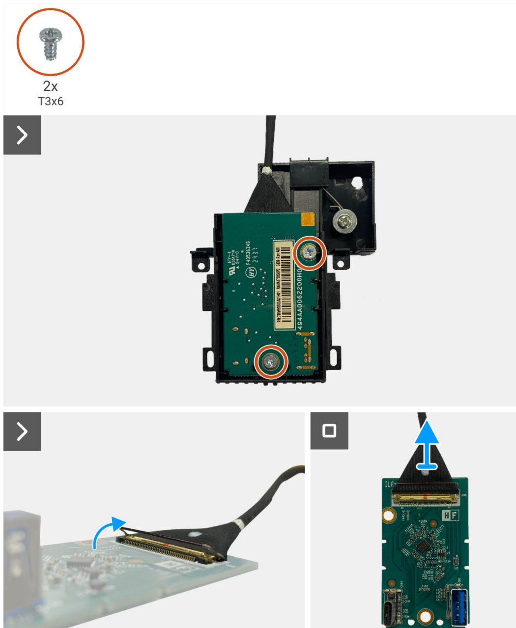
Obrázek 12. Odmontování desky QAP
