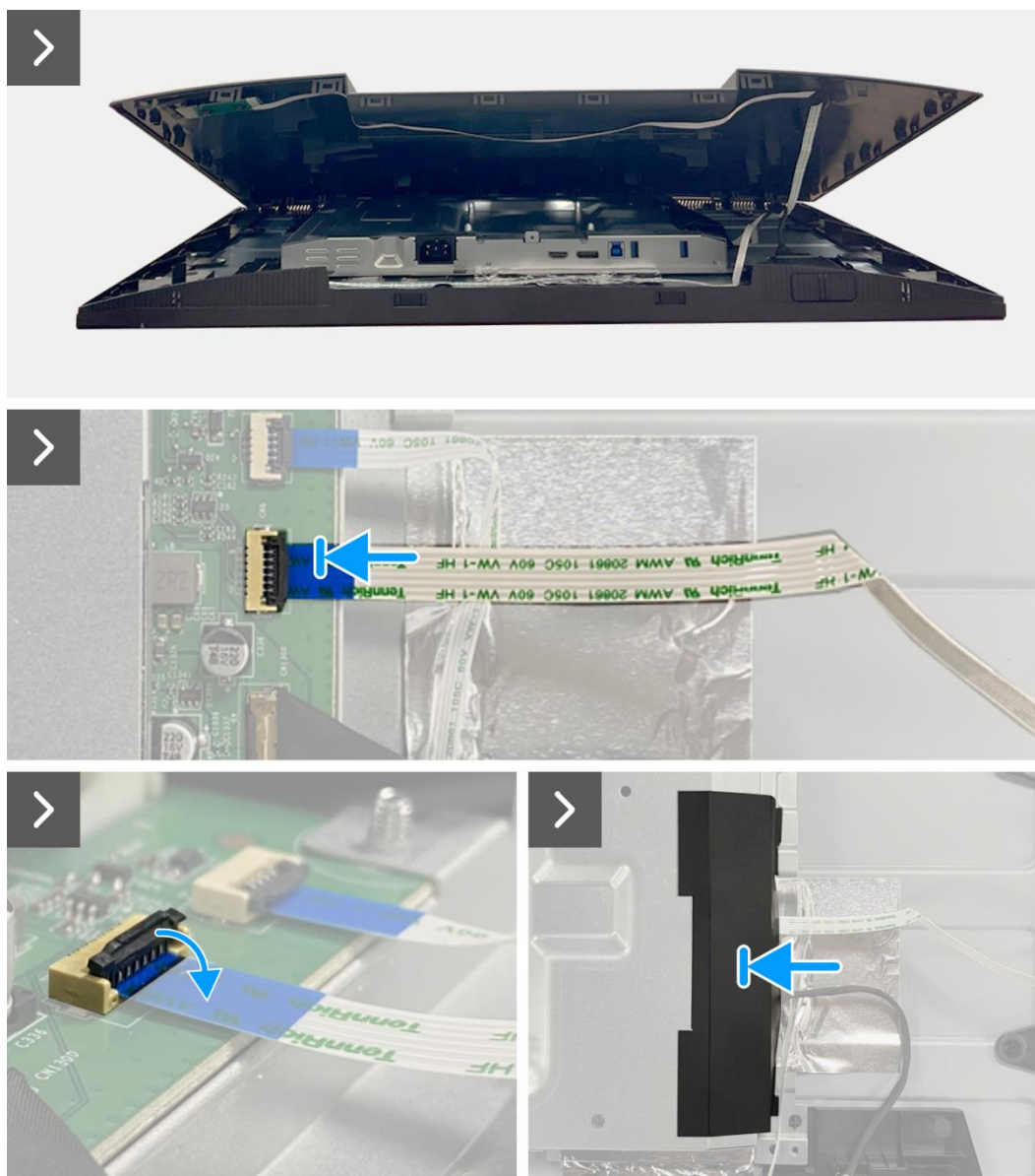
Obrázek 37. Instalace zadního krytu
