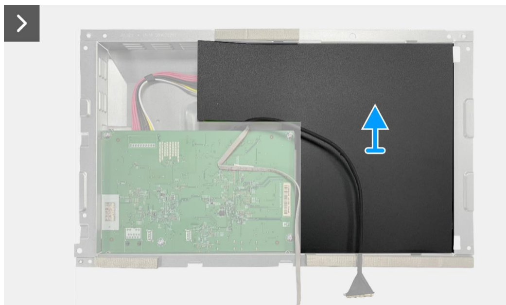
Obrázek 79. Odmontování desky rozhraní
