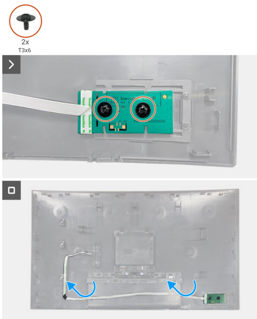
Obrázek 39. Odmontování desky klávesnice
