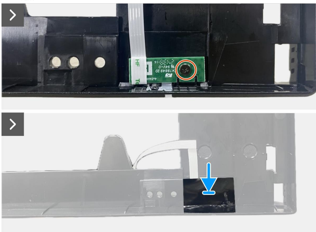
Obrázek 89. Instalace desky LED
