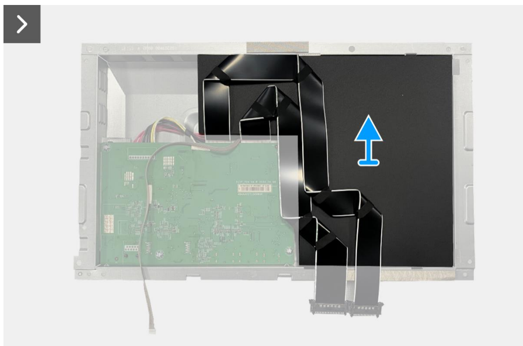
Obrázek 49. Odmontování desky rozhraní
