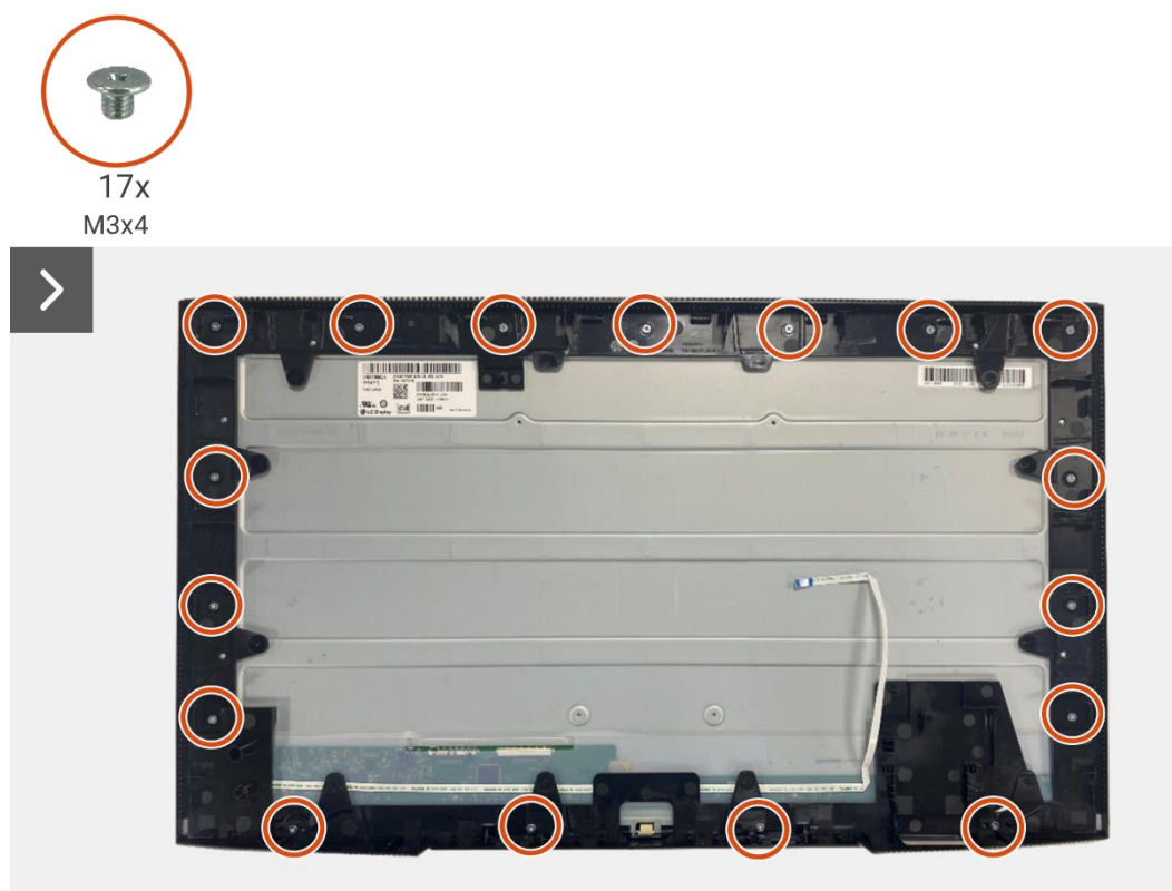
Obrázek 27. Odmontování desky LED
