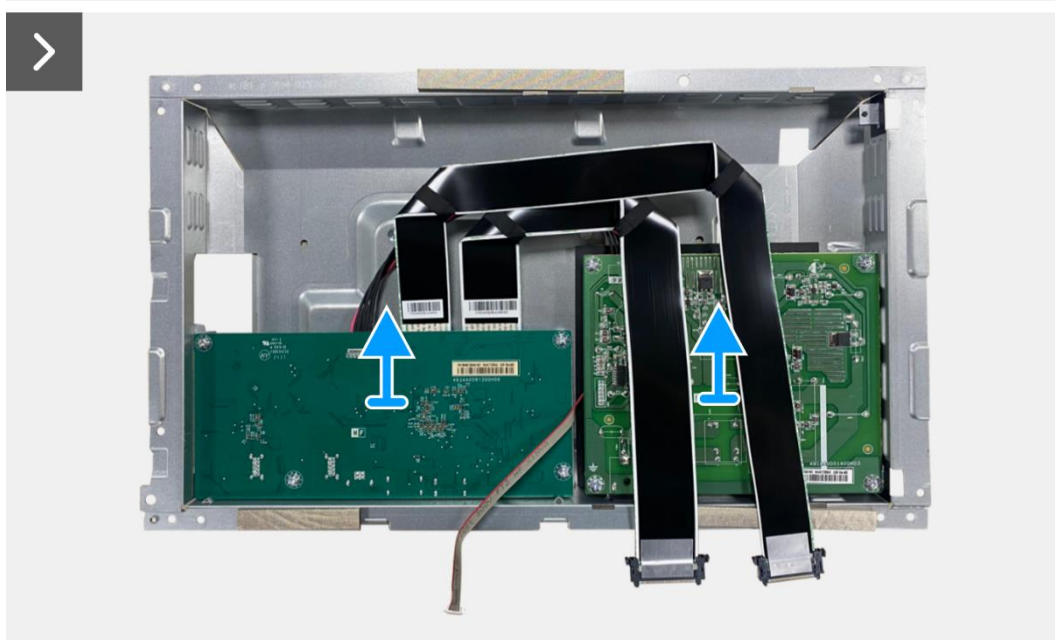
Obrázek 20. Odmontování desky rozhraní
