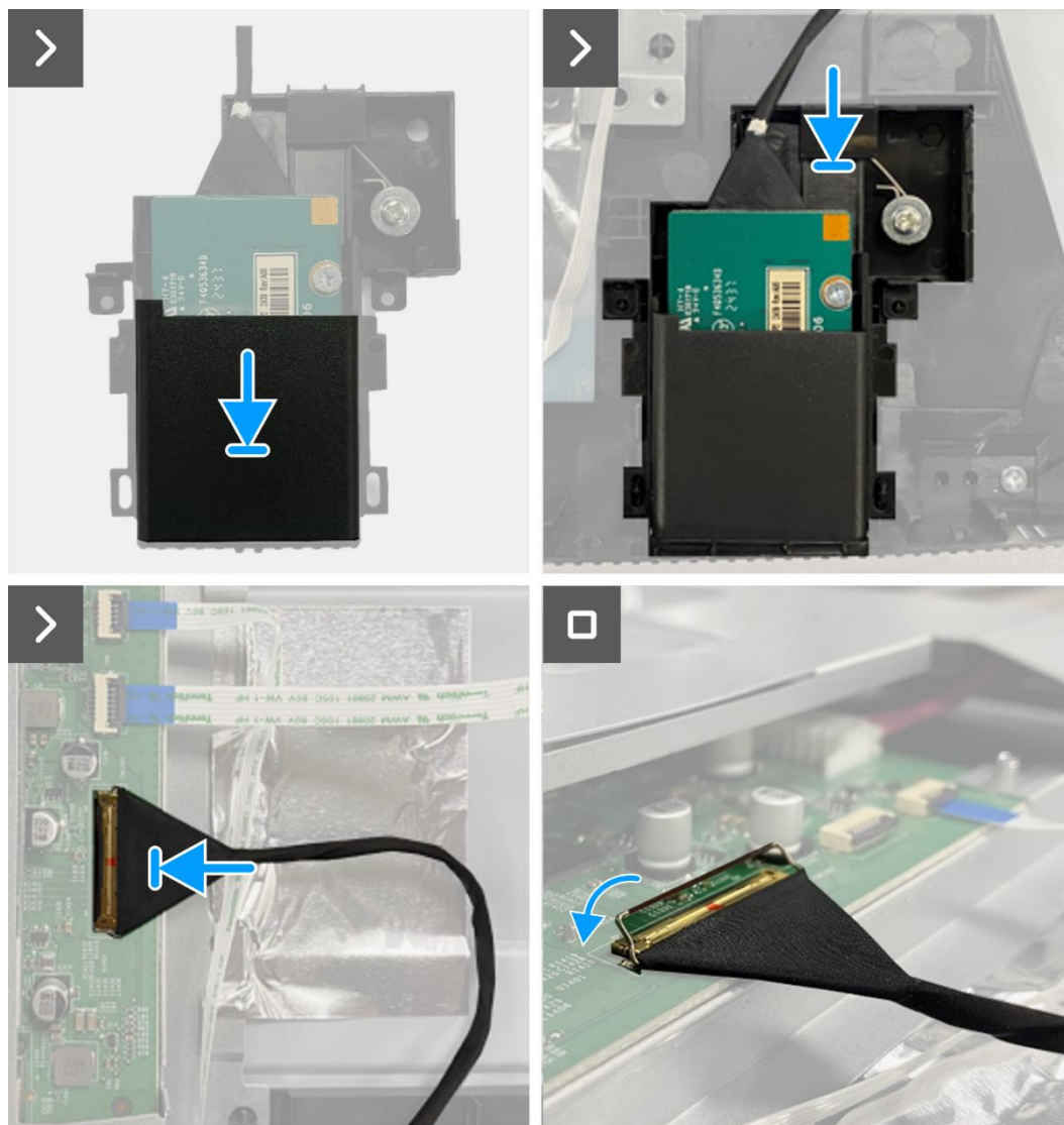
Obrázek 44. Instalace desky QAP
