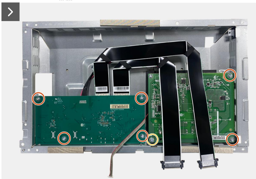
Obrázek 23. Instalace desky rozhraní
