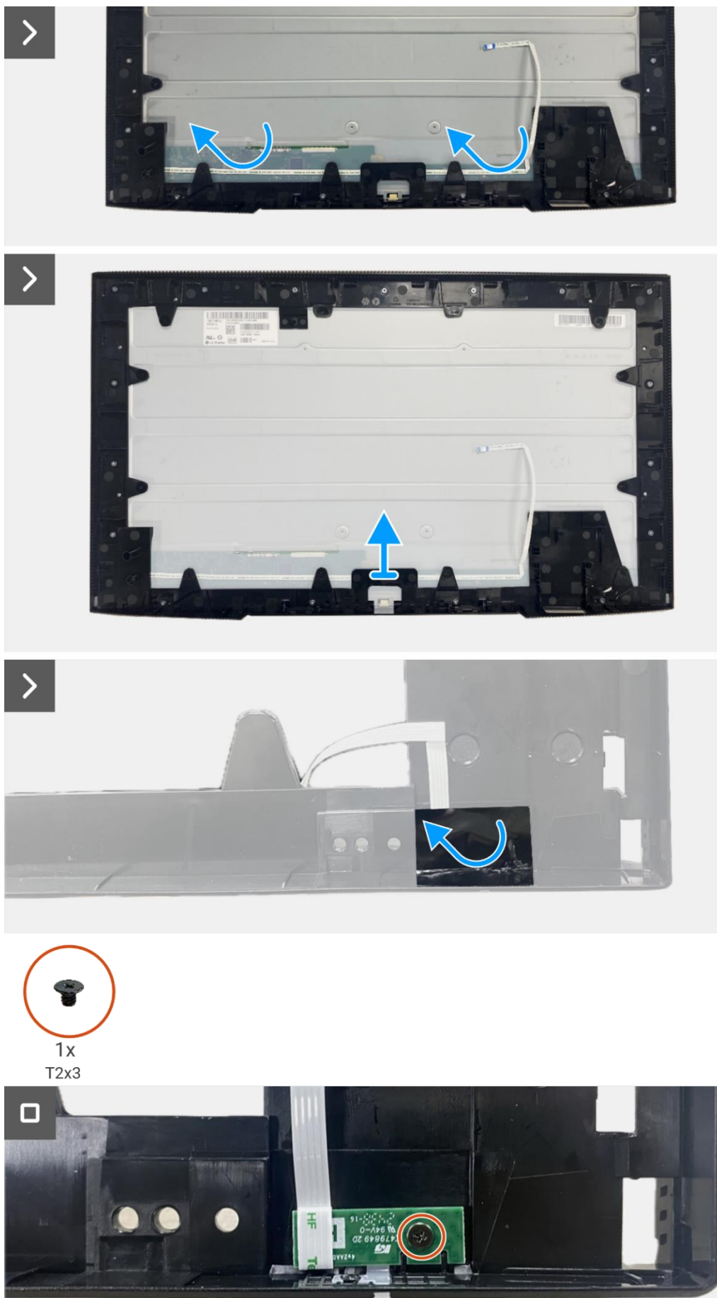
Obrázek 58. Odmontování desky LED
