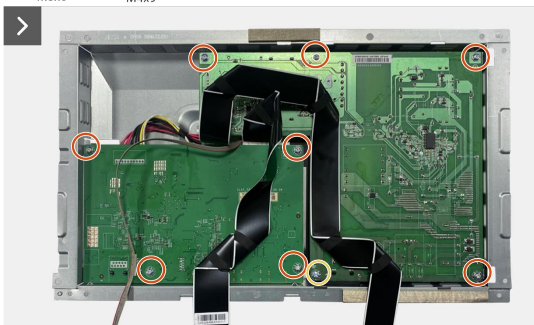
Obrázek 53. Instalace desky rozhraní
