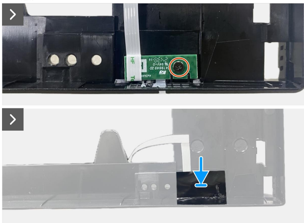
Obrázek 59. Instalace desky LED
