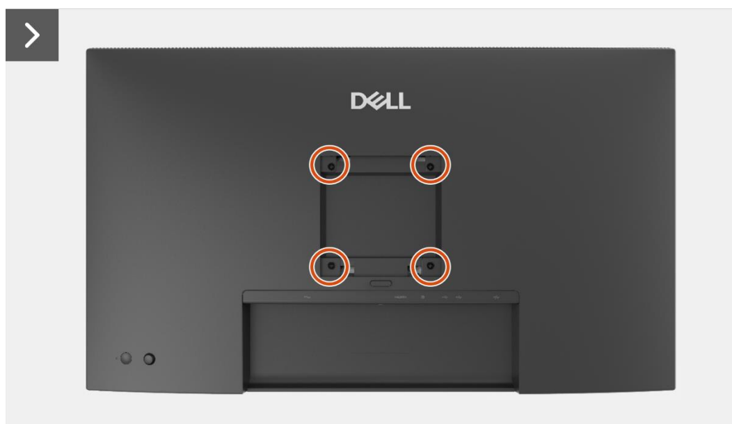
Obrázek 5. Odmontování zadního krytu
