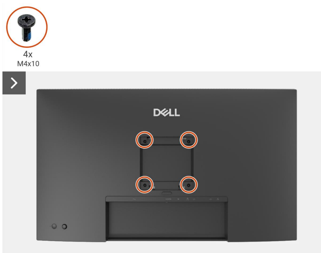
Obrázek 65. Odmontování zadního krytu
