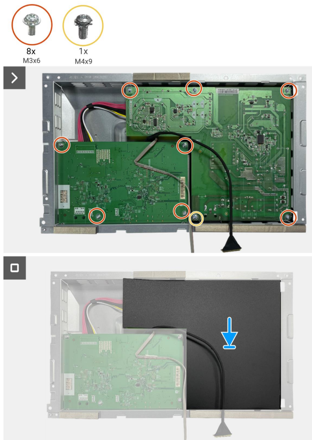
Obrázek 84. Instalace desky rozhraní
