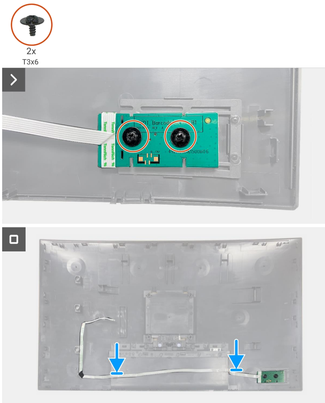
Obrázek 57. Instalace desky klávesnice
