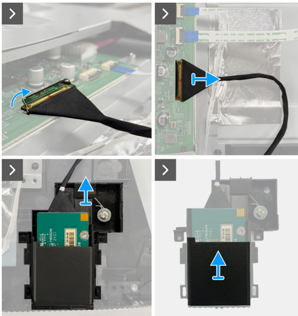
Obrázek 88. Odmontování desky QAP
