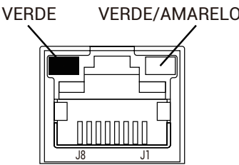
Figura 13. Conector de porta RJ45
