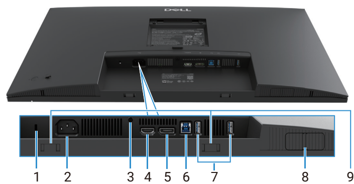
Figura 4. Vista inferior, sem suporte do monitor
