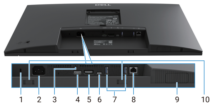
Figura 6. Vista inferior, sem suporte do monitor
