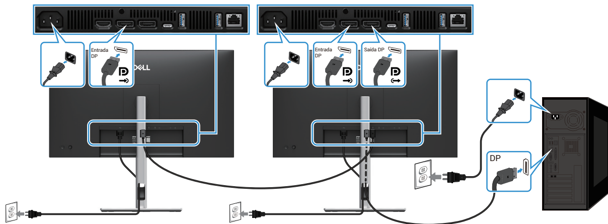
Figura 32. Conexão do monitor para a função DP MST
