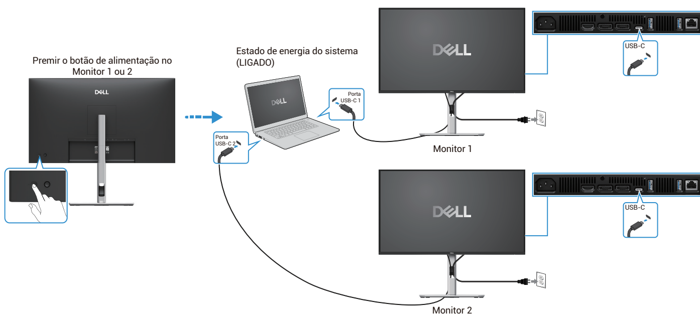
Figura 51. Ao premir o botão de alimentação no Monitor 1 ou no Monitor 2, o computador é ligado
