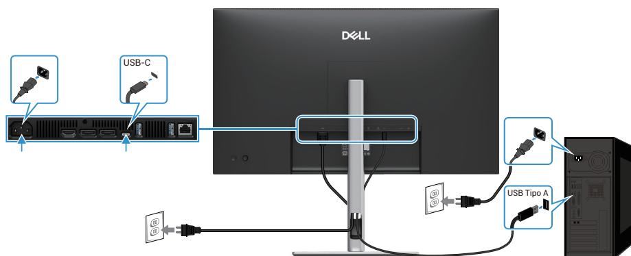
Figura 30. Conexão do cabo USB Tipo C ao Tipo A
