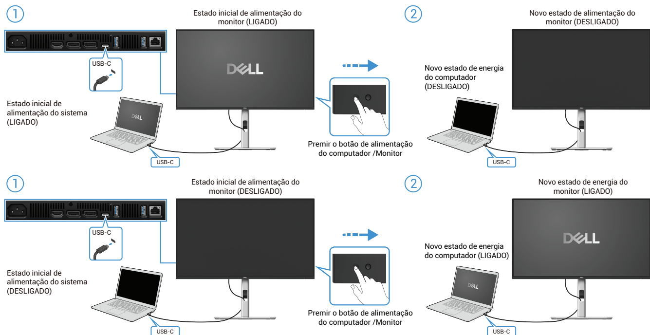
Figura 42. Premir o botão de alimentação do monitor ou o botão de alimentação do computador
