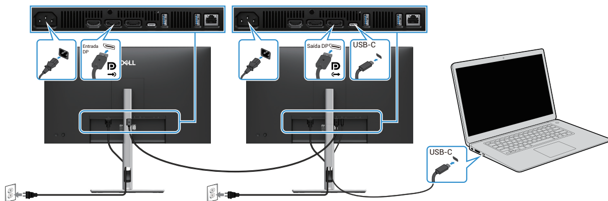
Figura 33. Conexão do monitor para a função USB-C MST
