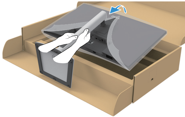
Figura 23. Levantar o monitor
