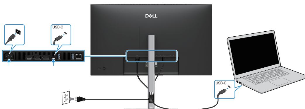
Figura 29. Conexão do cabo USB-C a C
