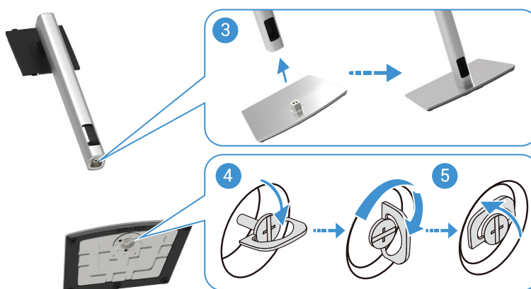
Figura 20. Inserir a base do suporte
