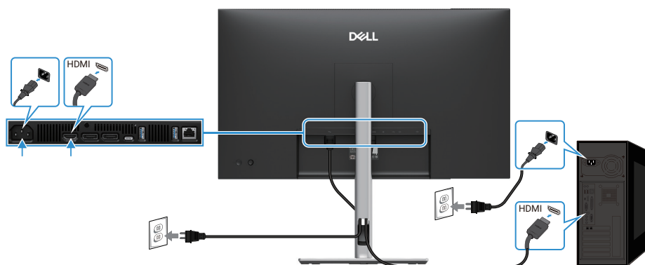
Figura 26. Conexão do cabo HDMI
