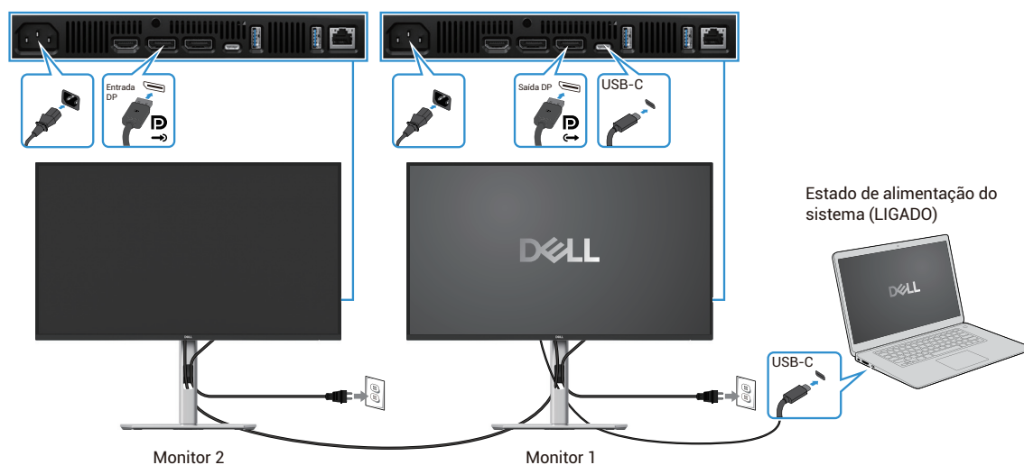
Figura 46. Conexão do monitor para a função USB-C MST
