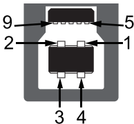
Figura 10. Conector direto USB 5Gbps Tipo B
