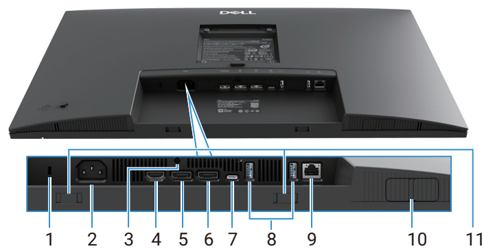
Figura 5. Vista inferior, sem suporte do monitor
