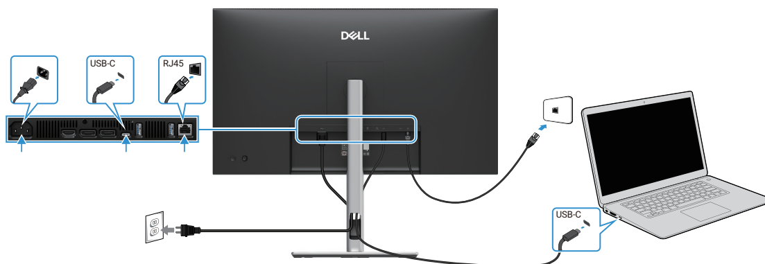
Figura 31. Conexão do cabo RJ45
