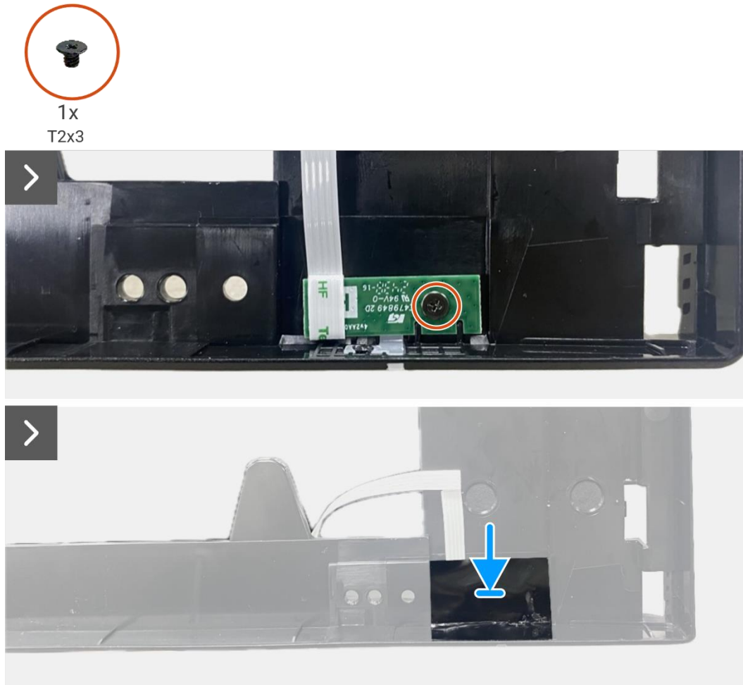
Imagen 106. Instalación de la placa LED
