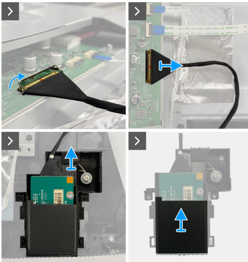
Imagen 88. Extracción de la placa QAP
