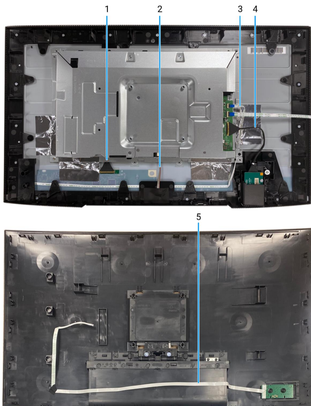
Imagen 9. Diagrama de conectividad de cableado
