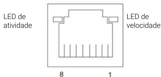
Figura 11. Porta RJ45 (lado do conector)
