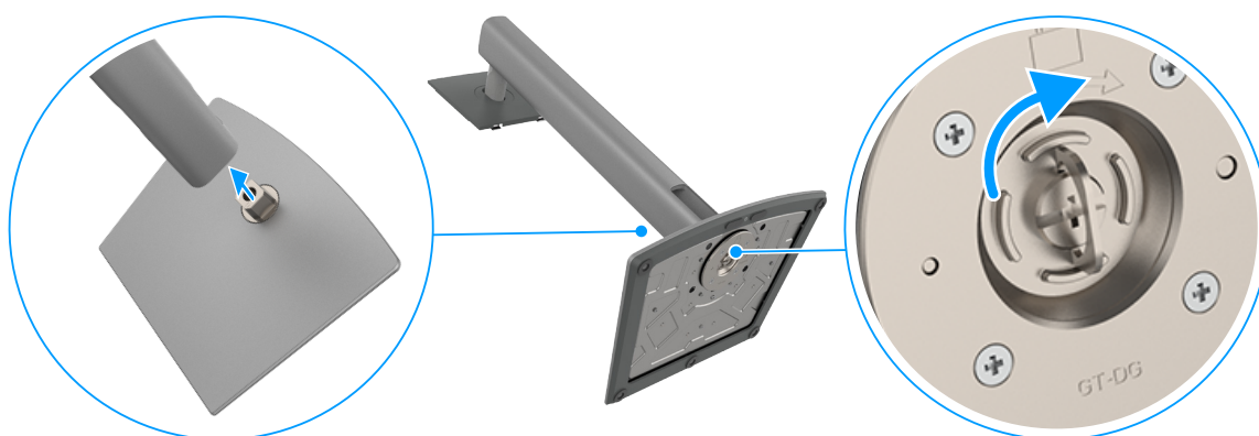
Figura 18. Encaixar o suporte
