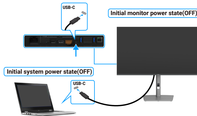
Figura 42. Ligar o monitor para DPBS pela primeira vez
