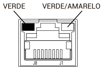
Figura 13. Conector de porta RJ45
