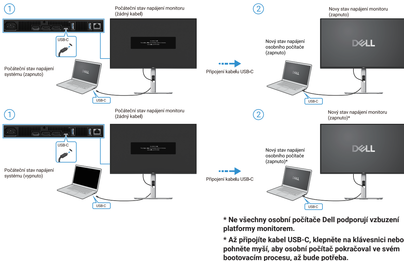
Obrázek 41. Připojení kabelu USB-C
