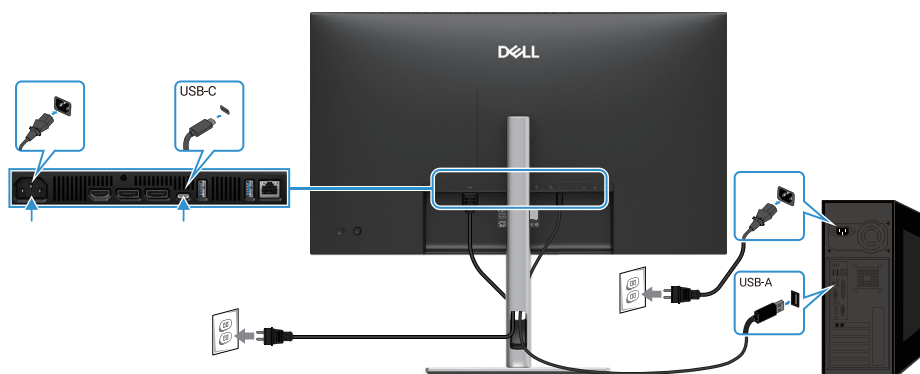
Obrázek 30. Připojení kabelu USB-C na USB-A
