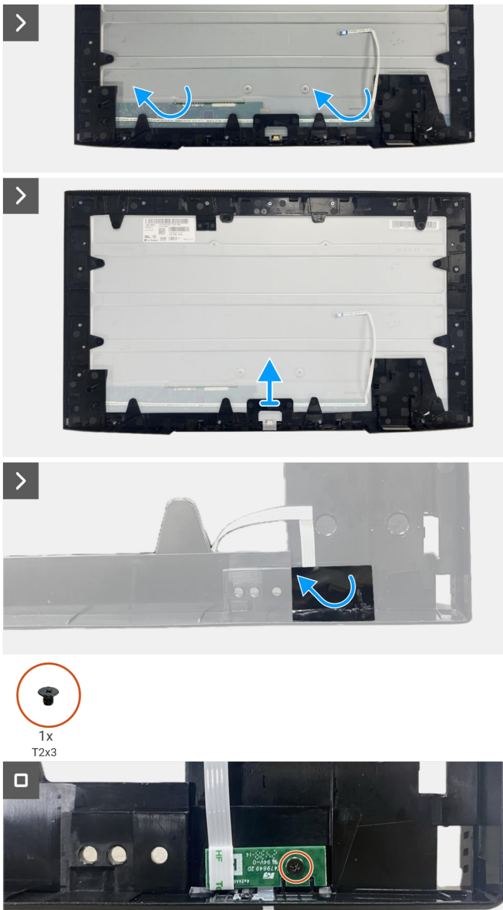
Obrázek 58. Odmontování desky LED
