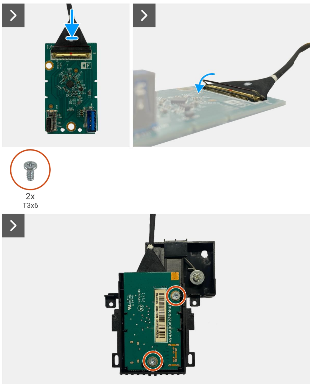
Figure 30. Installation de la carte QAP
