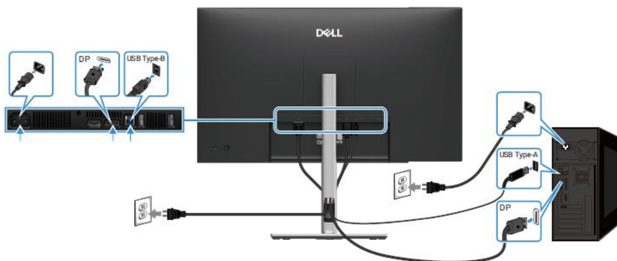
Figure12. Connexion du DisplayPort et le câble USB
