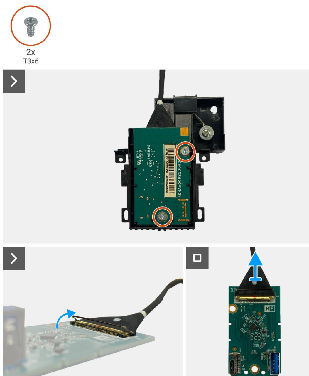
Figure 59. Retrait de la carte QAP
