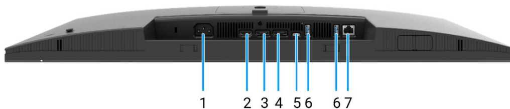
Figure 4. Vue de dessous du moniteur
