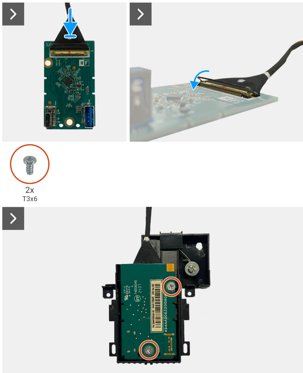
Figure 90. Installation de la carte QAP
