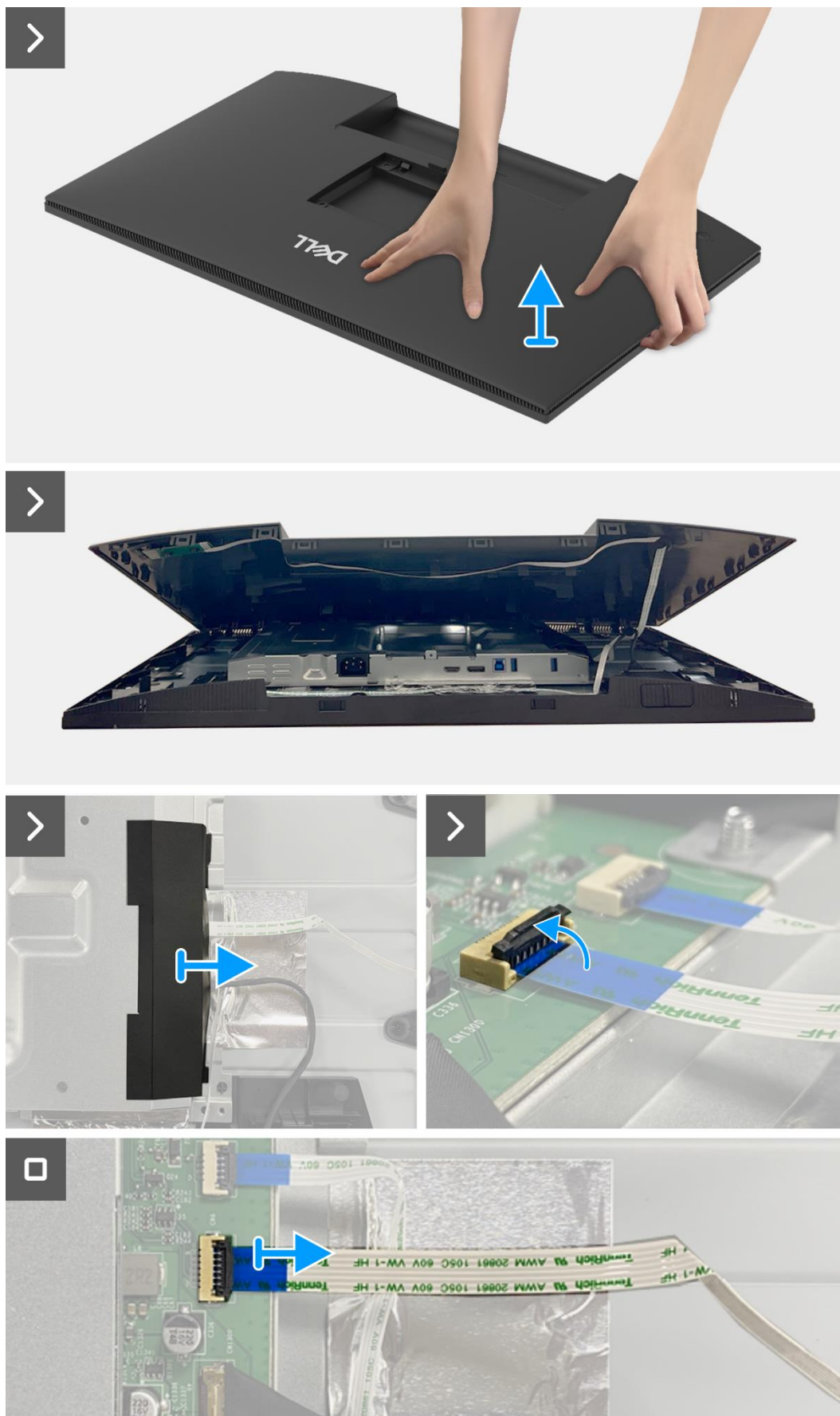
Figure 53. Retrait du couvercle arrière
