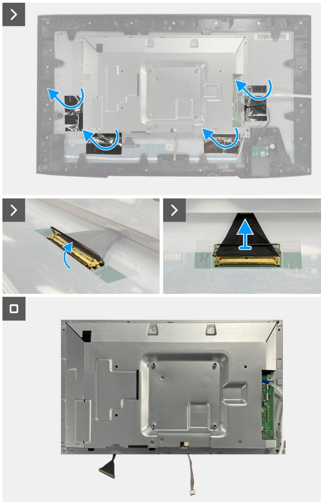
Figure 93. Retrait de l'assemblage du châssis
