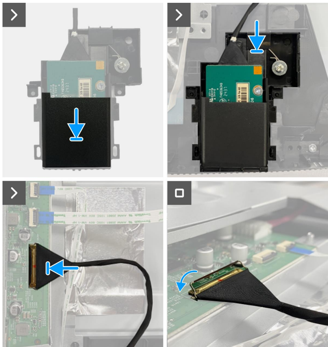
Figure 61. Installation de la carte QAP
