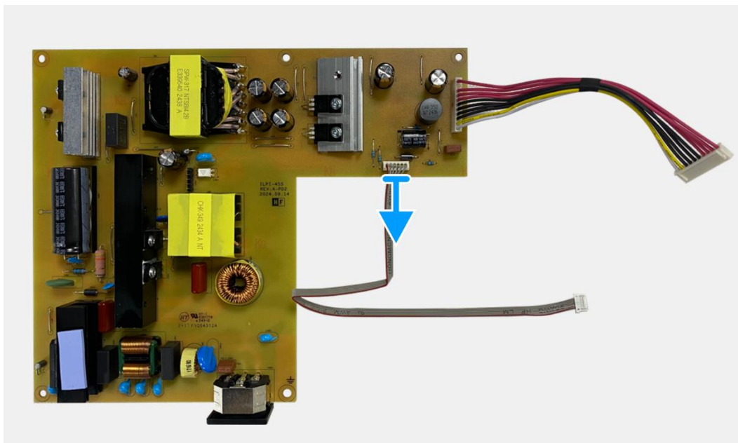
Figure 102. Retrait de la carte d'alimentation
