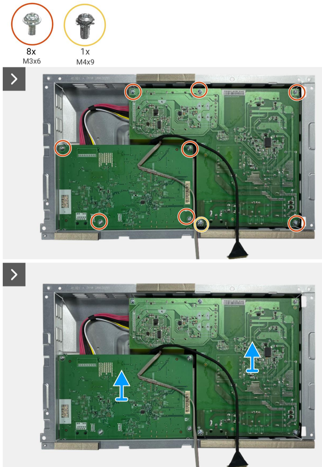
Figure 97. Retrait de la carte interface
