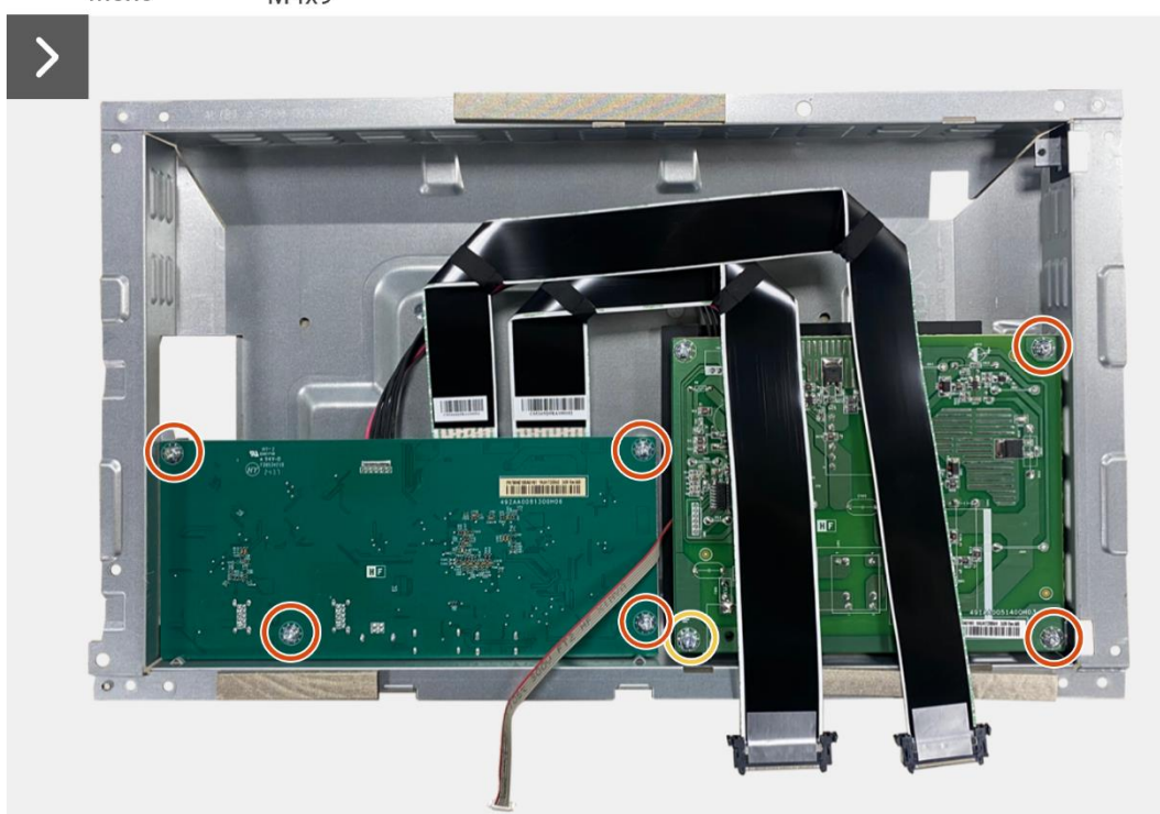
Figure 40. Installation de la carte interface
