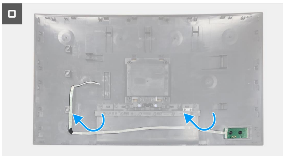
Figure 56. Retrait de la carte clavier
