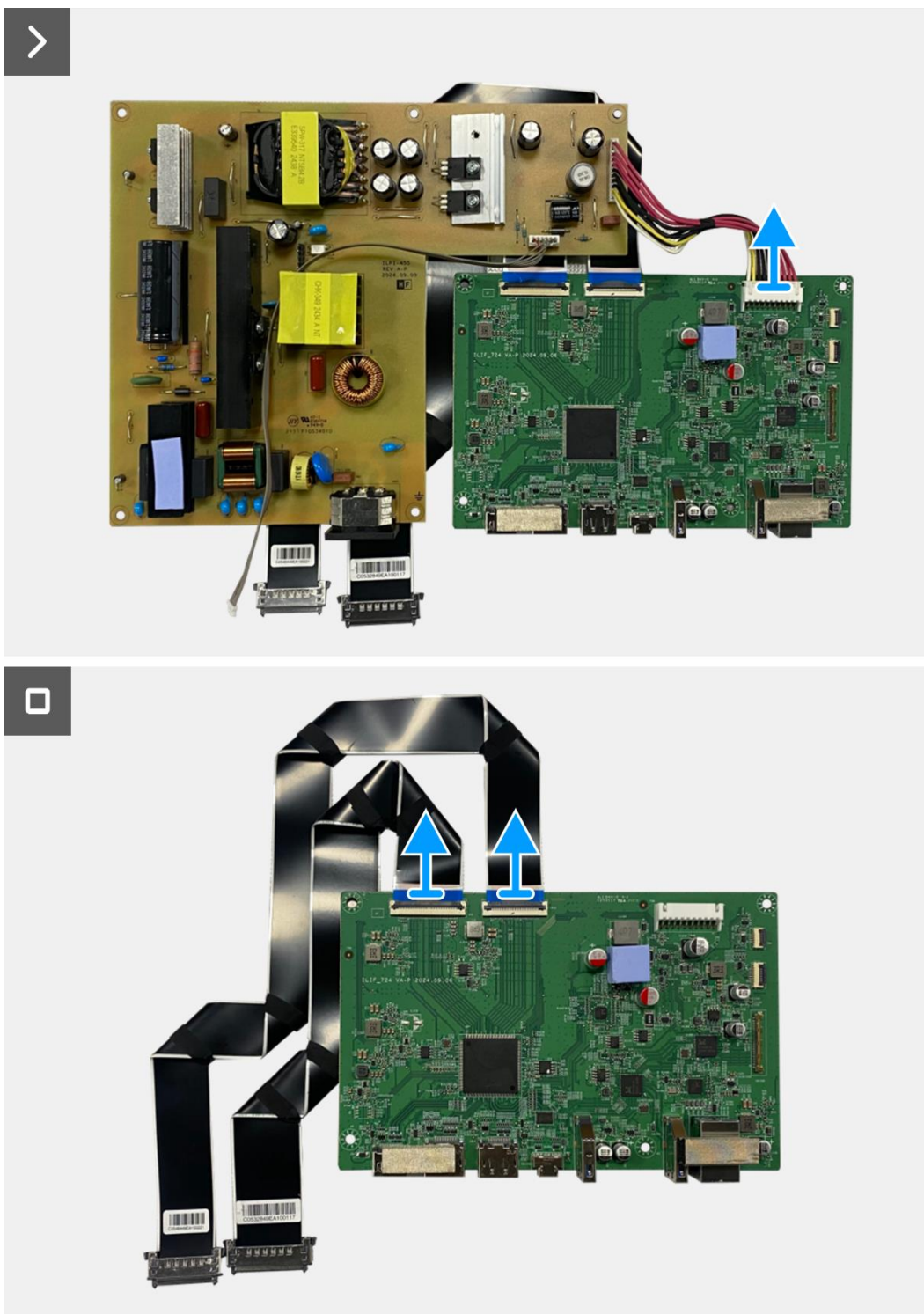
Figure 68. Retrait de la carte interface
