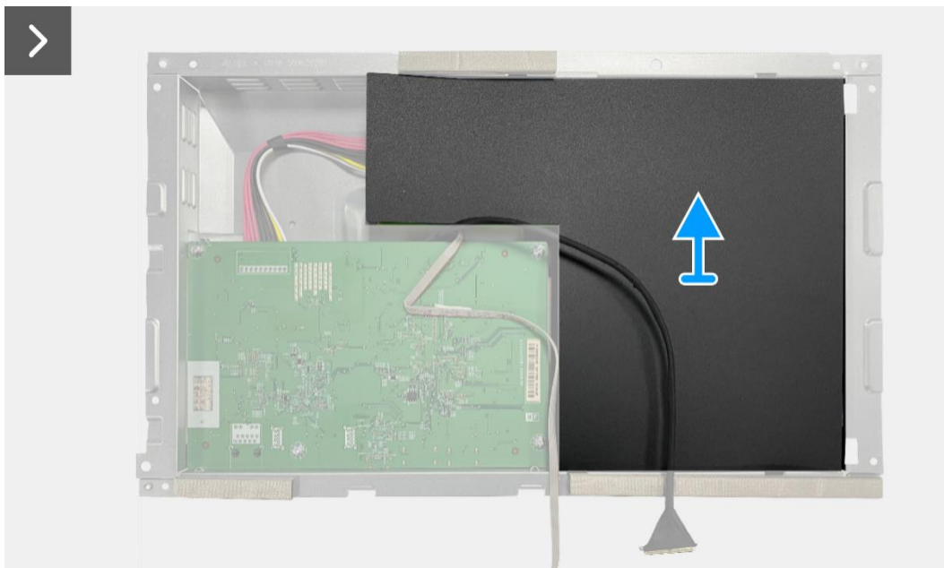
Figure 96. Retrait de la carte interface
