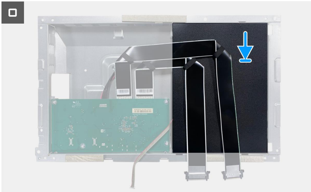
Figure 41. Installation de la carte interface
