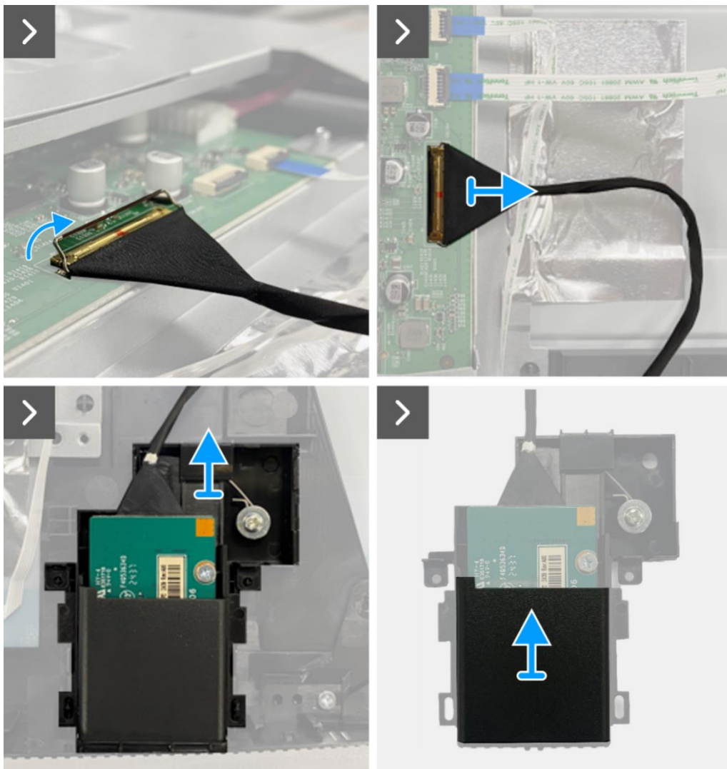
Figure 28. Retrait de la carte QAP
