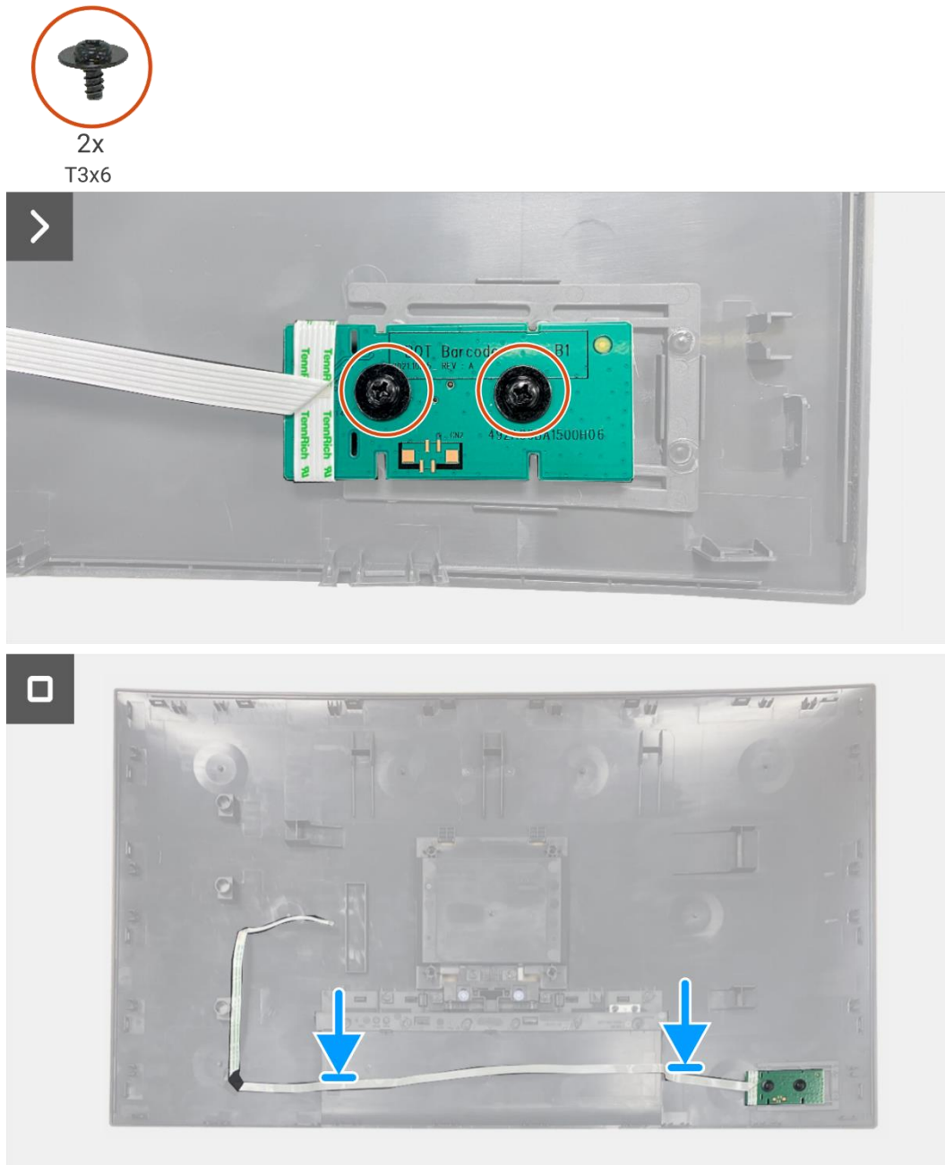
Figure 57. Installation de la carte clavier
