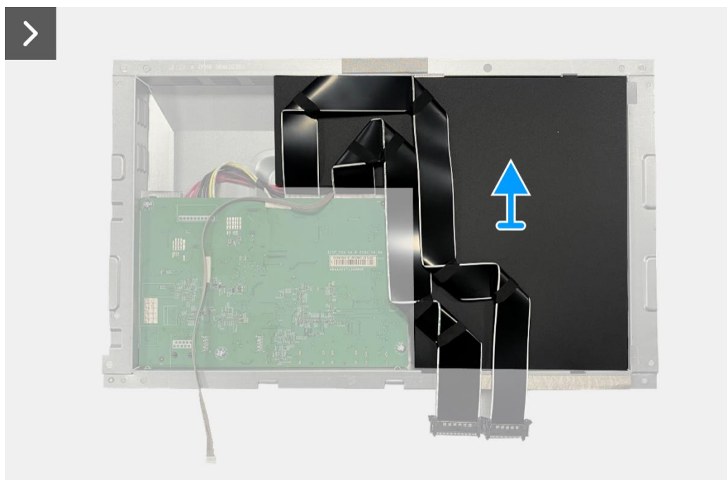
Figure 66. Retrait de la carte interface
