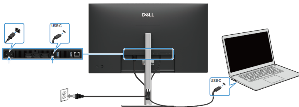
Figure 13. Connexion du câble USB-C vers C
