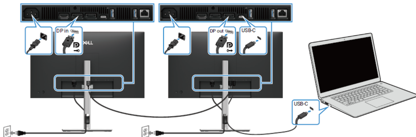
Figure 17. Connexion du moniteur pour la fonction MST pour USB-C
