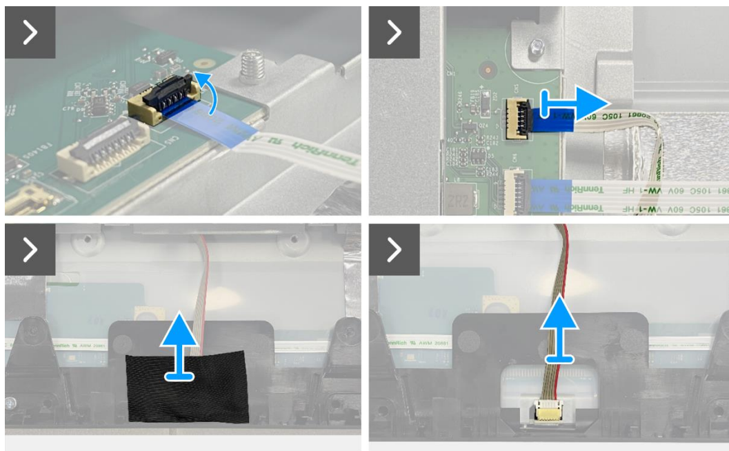
Figure 92. Retrait de l'assemblage du châssis
