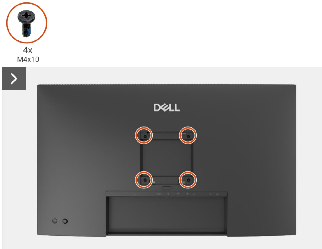
Figure 52. Retrait du couvercle arrière
