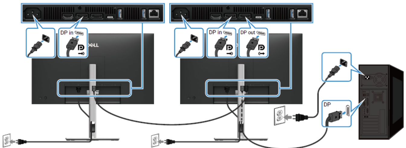
Figure 16. Connexion du moniteur pour la fonction MST DP
