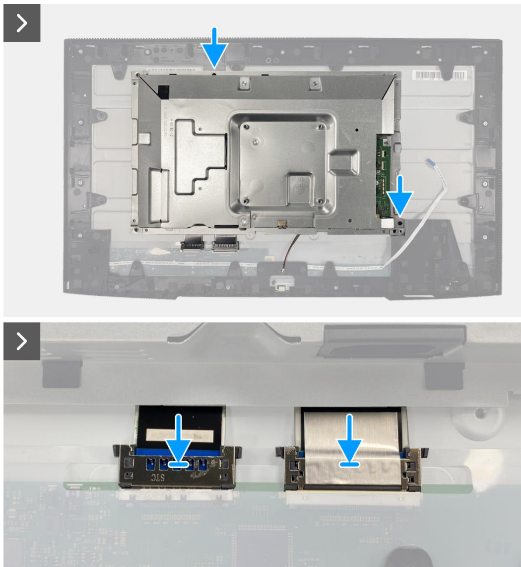
Figure 64. Installation de l'assemblage du châssis
