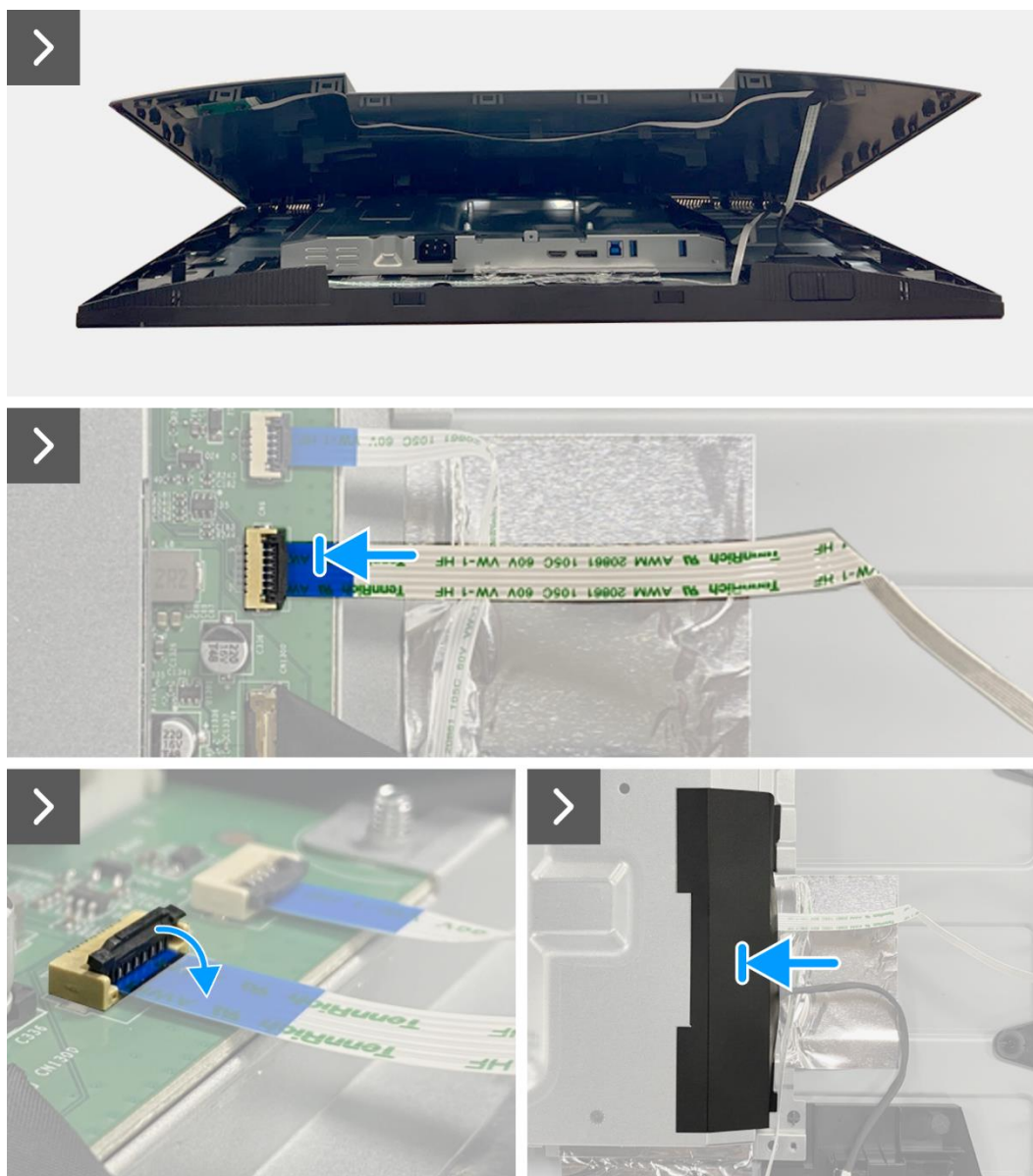
Figure 24. Installation du couvercle arrière
