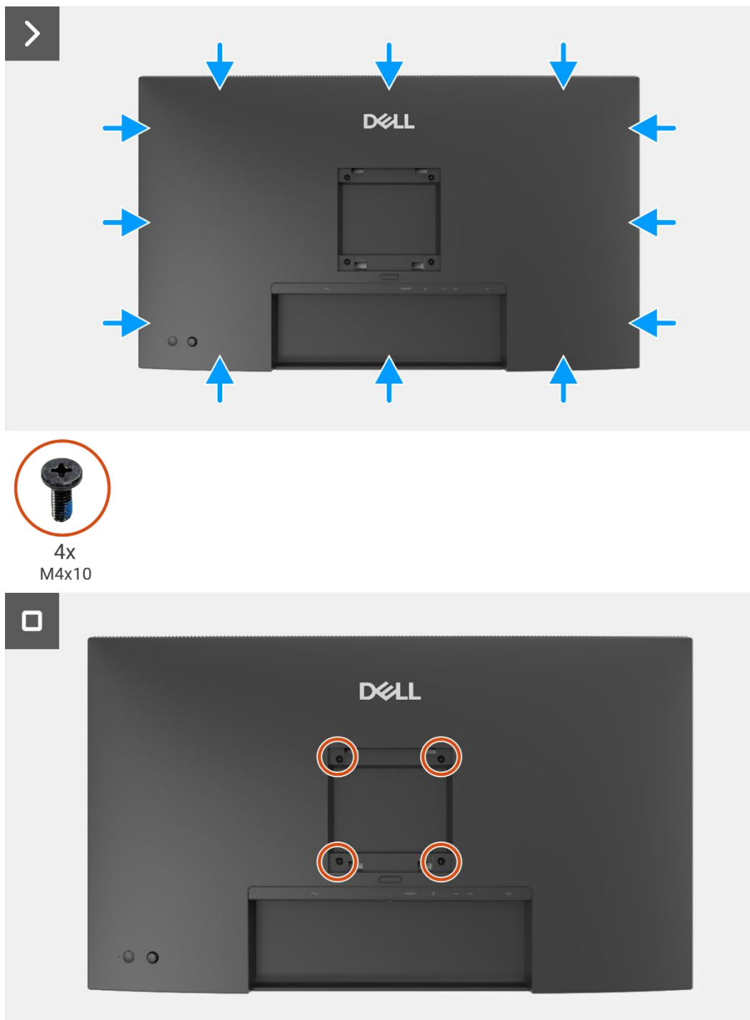
Figure 25. Installation du couvercle arrière
