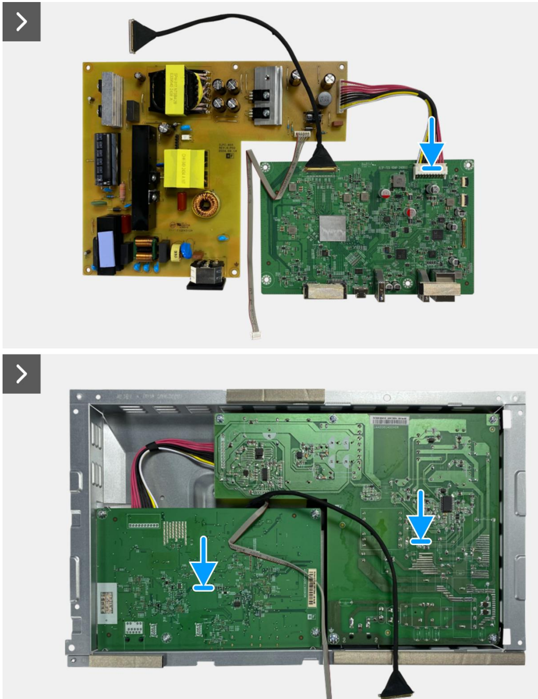
Figure 100. Installation de la carte interface
