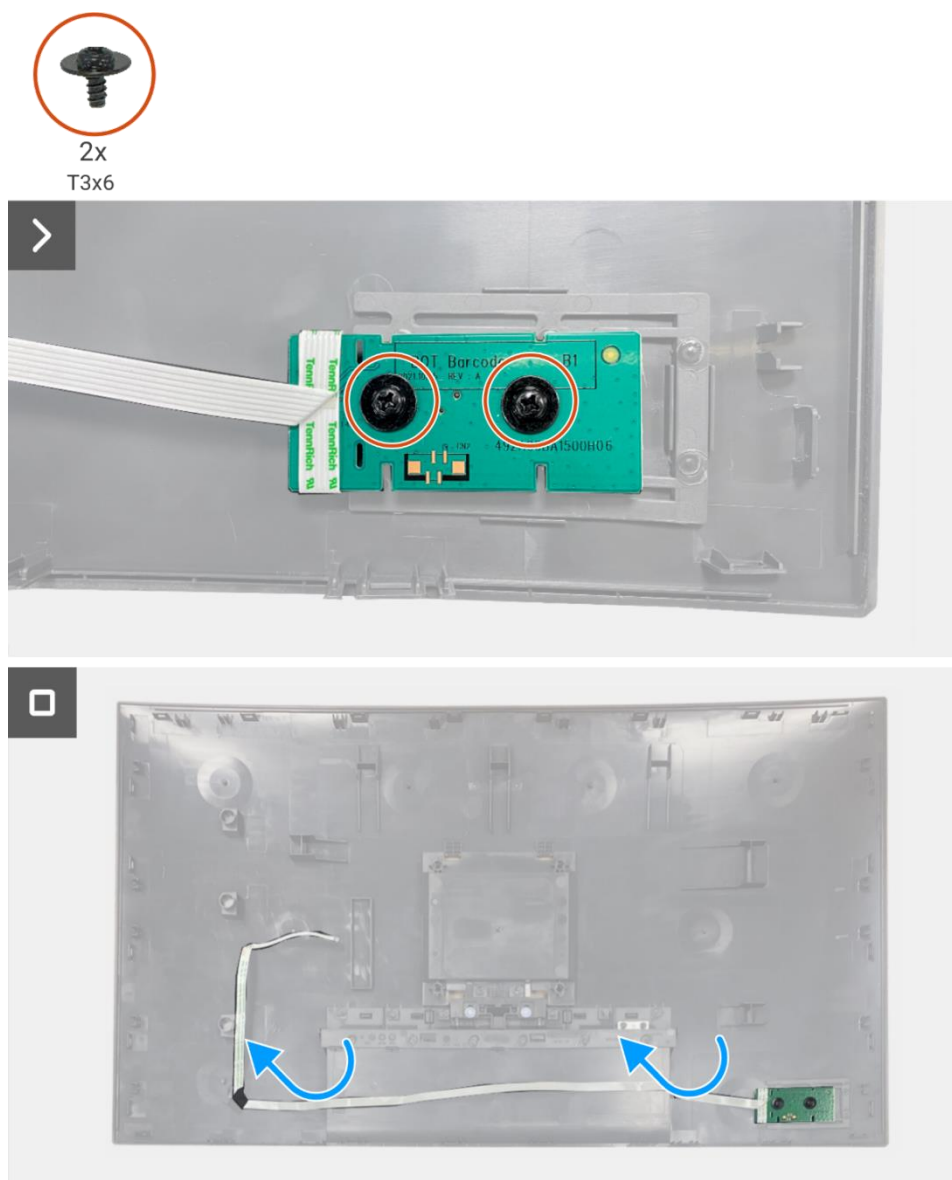
Figure 26. Retrait de la carte clavier
