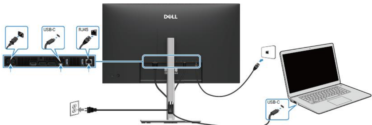
Figure 15. Connexion du câble RJ45
