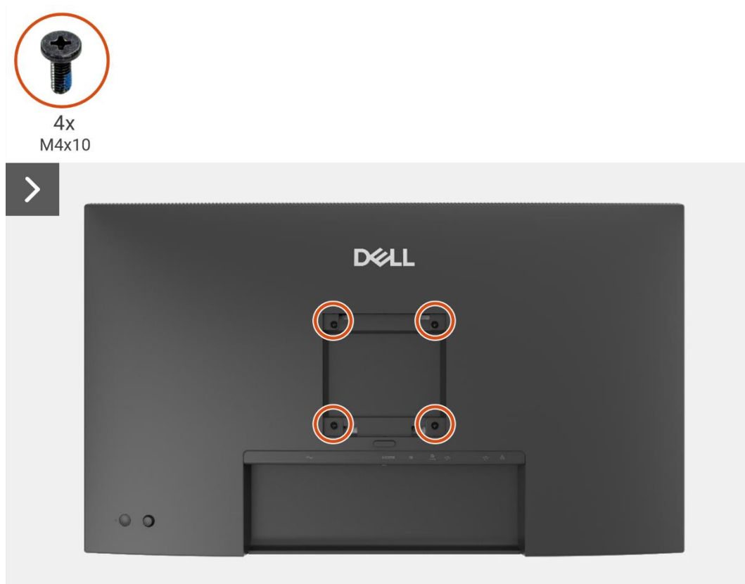
Figure 82. Retrait du couvercle arrière
