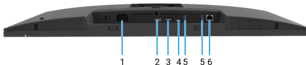
Figure 5. Vue de dessous du moniteur
