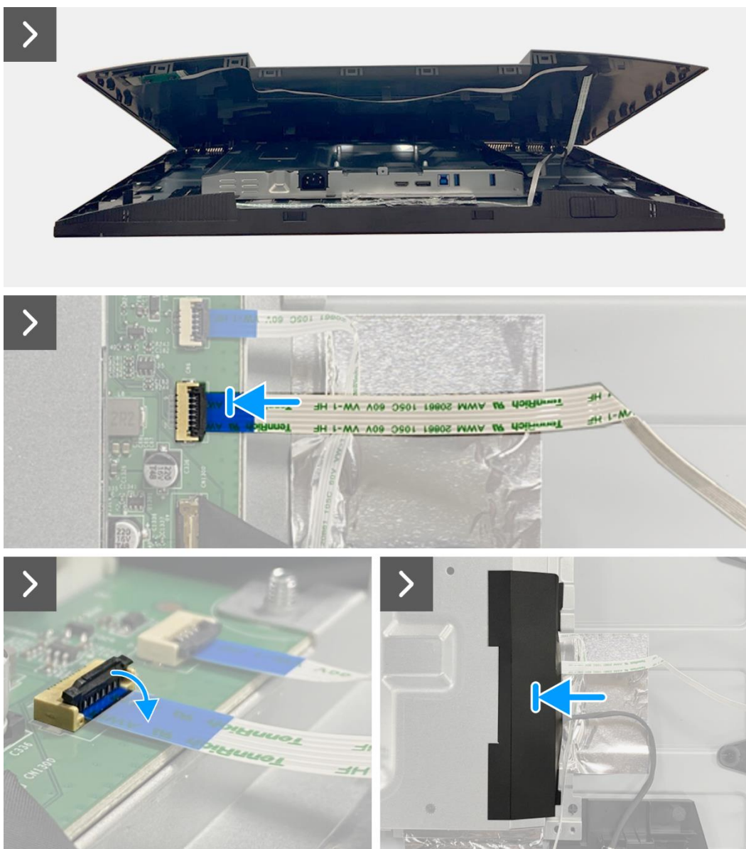
Figure 54. Installation du couvercle arrière
