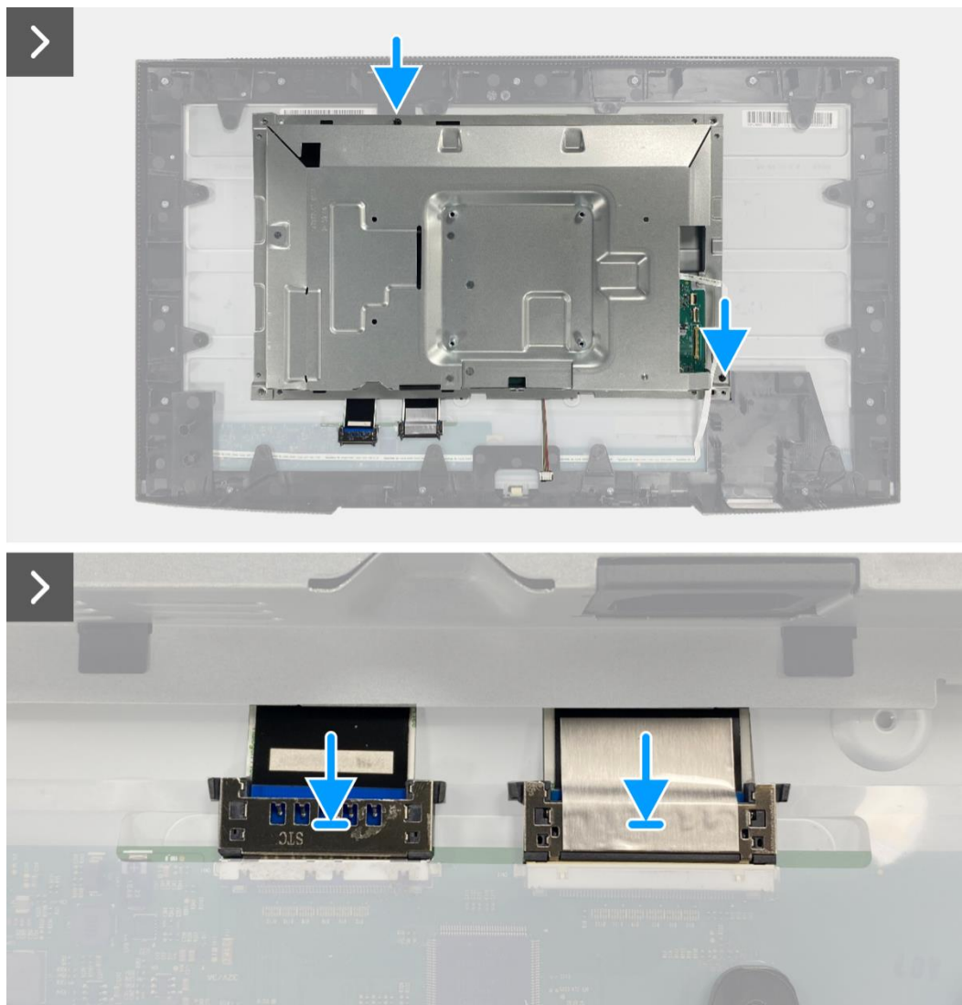
Figure 34. Installation de l'assemblage du châssis
