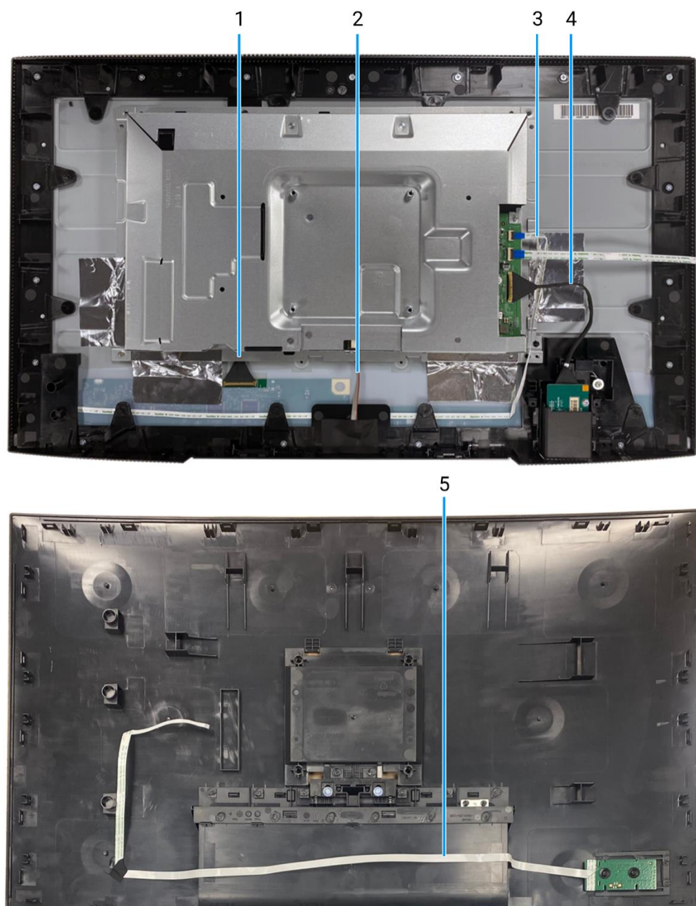
Figure 9. Schéma de connectivité des câblages
