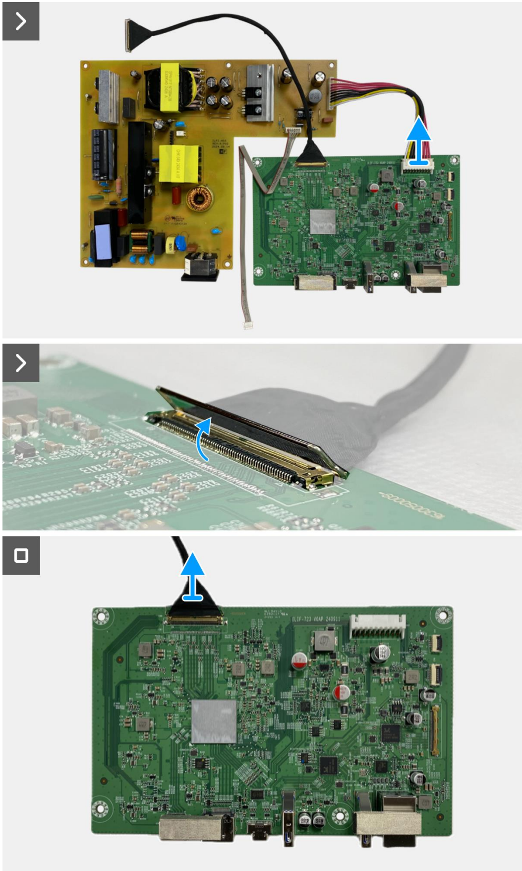
Figure 98. Retrait de la carte interface
