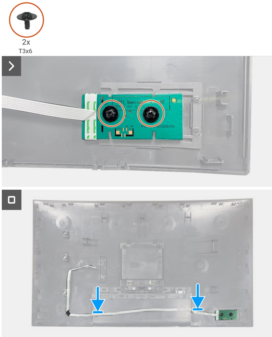
Rysunek 40. Instalowanie płytki klawiatury
