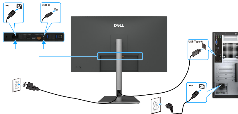
Figura 33. Conectar el cable USB Tipo-C a Tipo A
