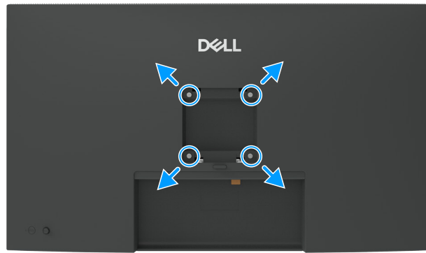
Figura 56. Instalación en pared VESA
