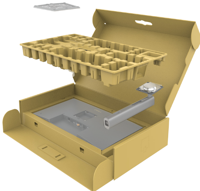
Figura 17. Desembalaje
