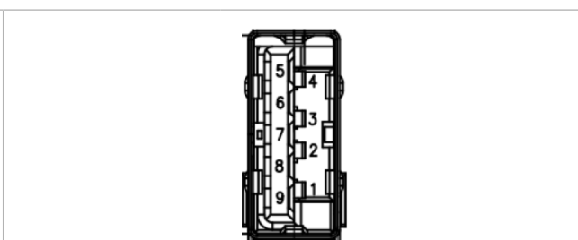
Figura 10. Puerto USB Tipo-A de 5 Gbps de bajada (parte trasera)
