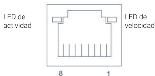
Figura 11. Puerto RJ45 (lado del conector)
