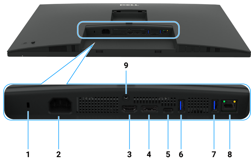
Figura 4. Vista inferior del monitor
