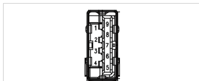
Figura 9. Puerto USB Tipo-A de 5 Gbps de bajada (parte inferior)
