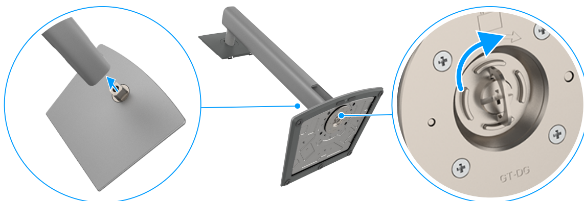
Figura 18. Conectar el pedestal
