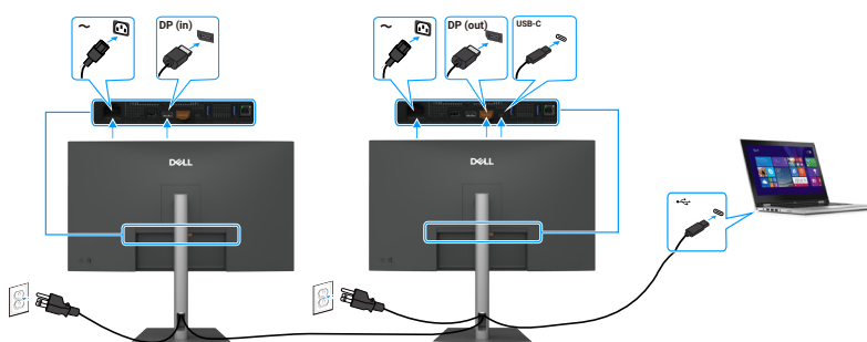
Figura 32. Conectar el monitor para la función USB-C MST (Multi-Stream Transport)
