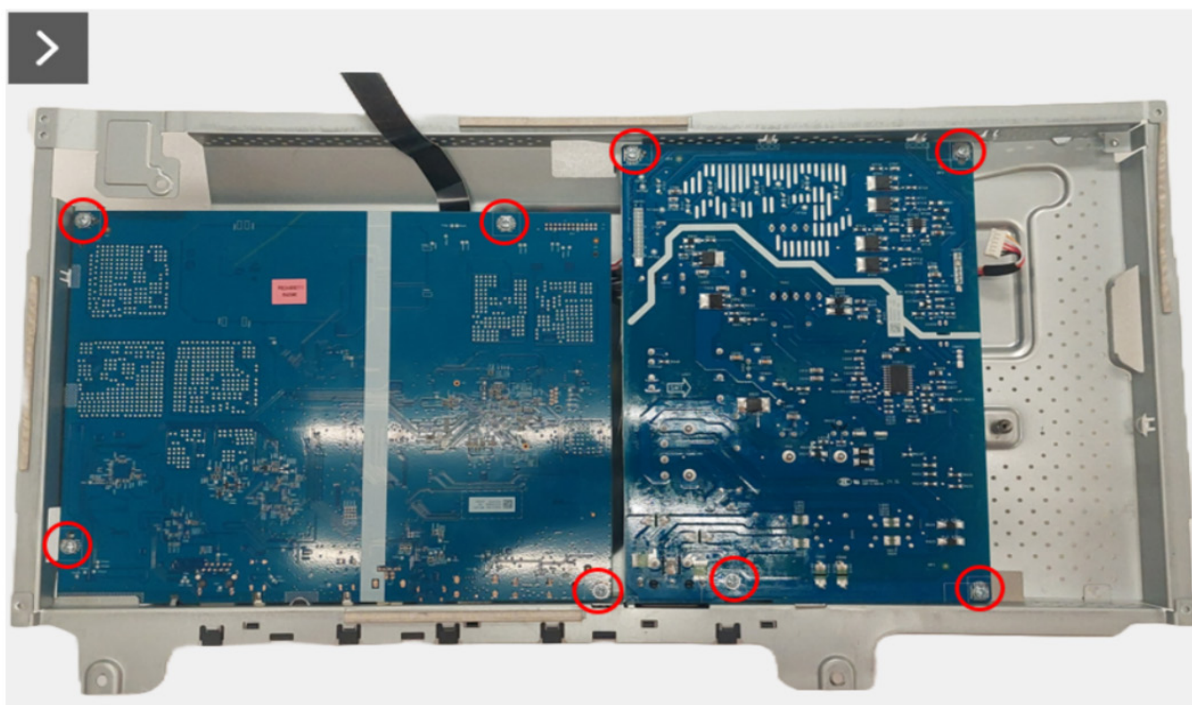
Obrázek 15. Demontáž desky rozhraní
