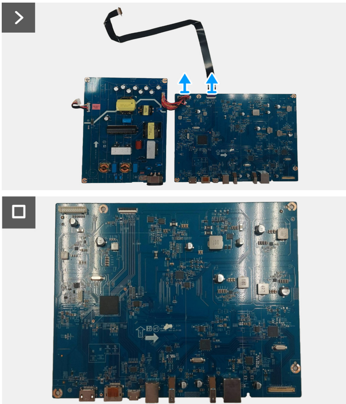
Obrázek 16. Demontáž desky rozhraní
