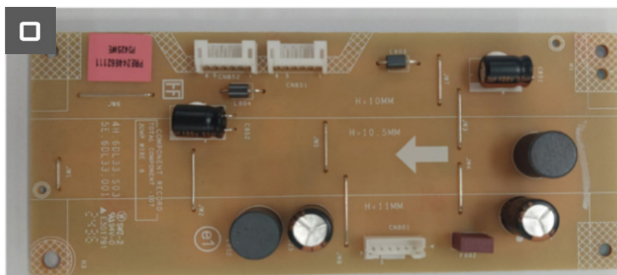
Obrázek 12. Demontáž desky se zdrojem LED
