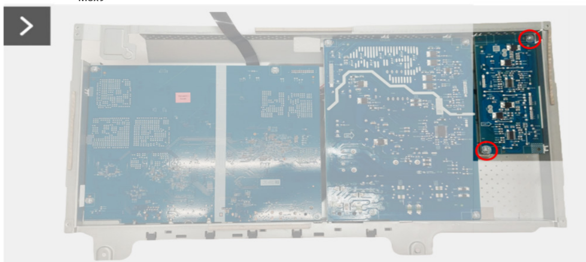
Obrázek 11. Demontáž desky se zdrojem LED
