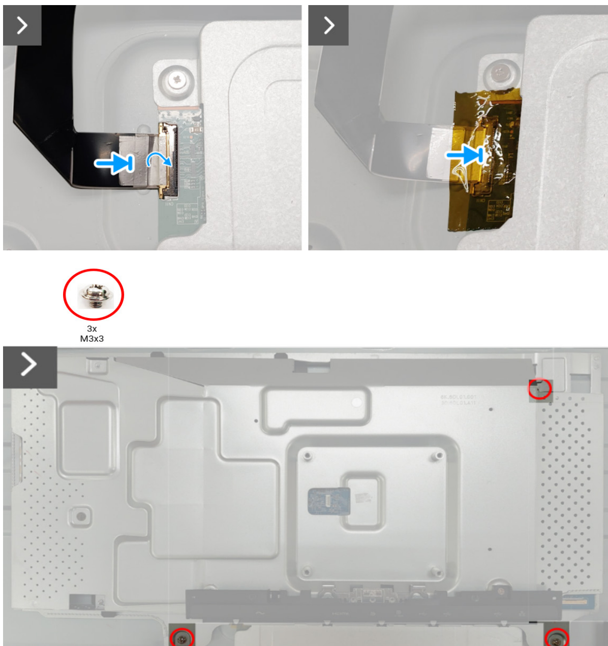
Obrázek 9. Instalace sestavy šasi
