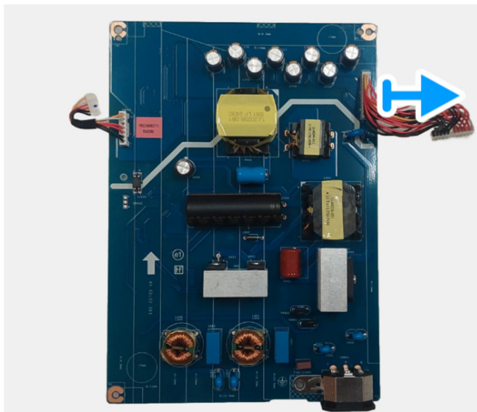
Obrázek 18. Demontáž napájecí desky
