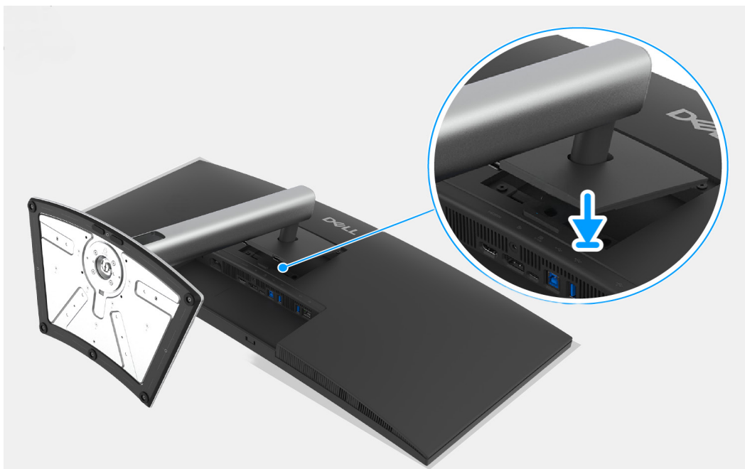
Obrázek 2. Instalace podstavce
