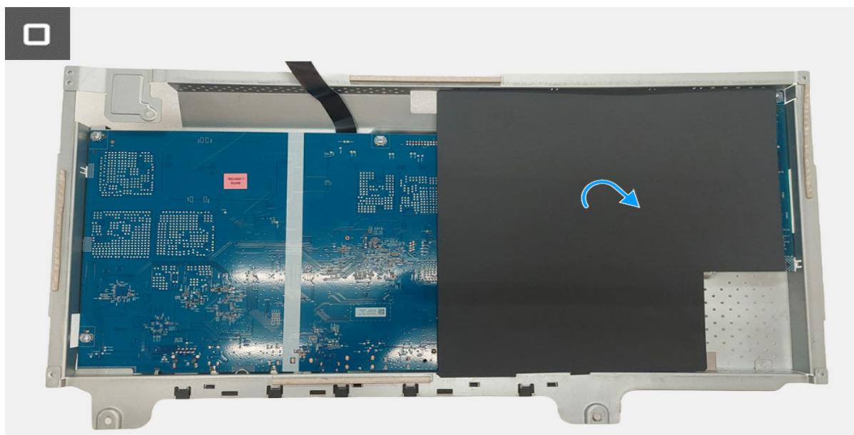
Obrázek 8. Demontáž sestavy šasi
