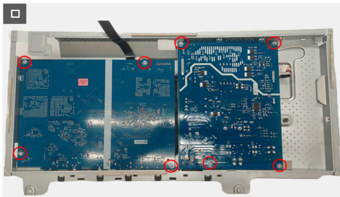
Obrázek 17. Instalace desky rozhraní
