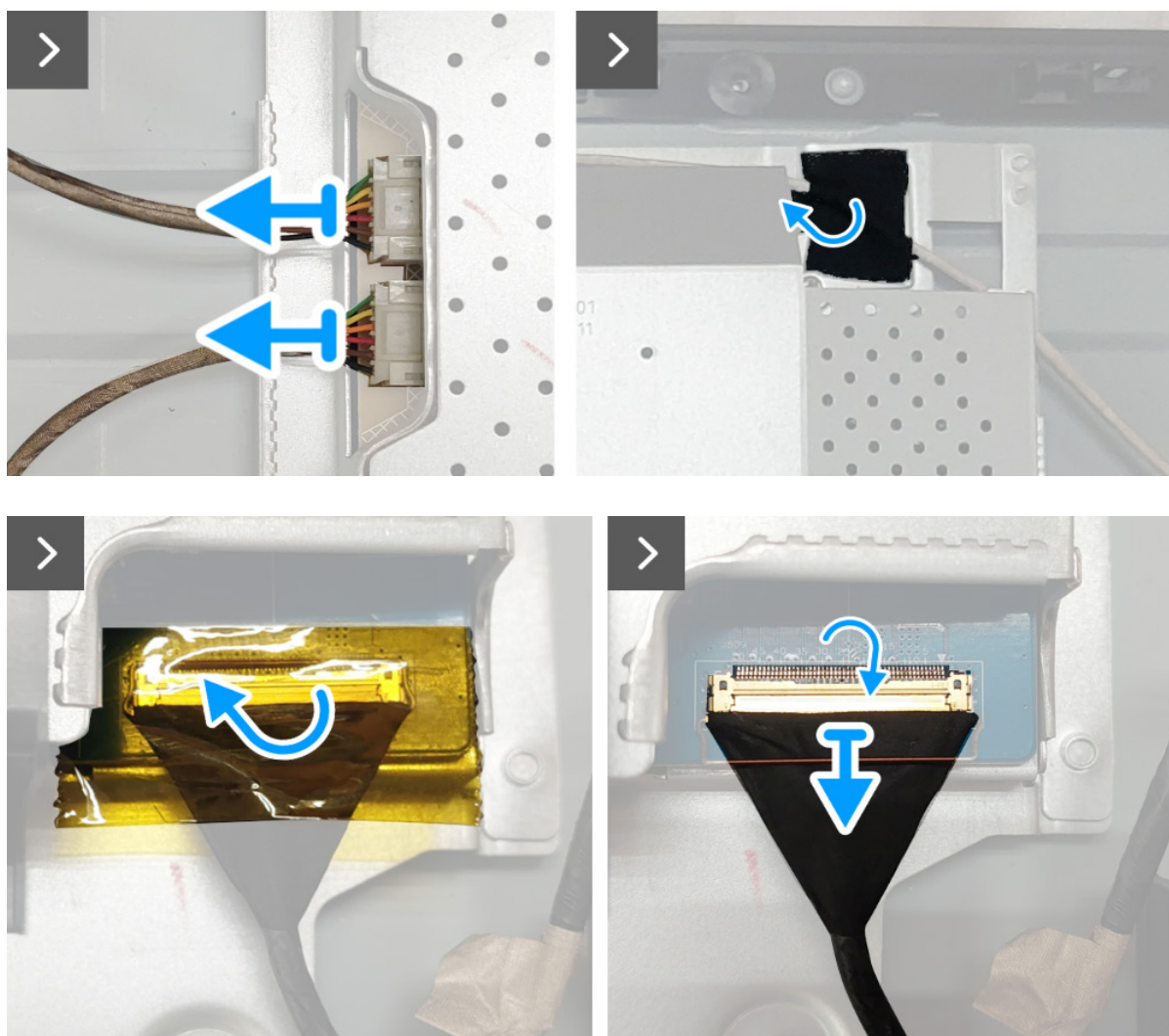
Obrázek 7. Demontáž sestavy šasi
