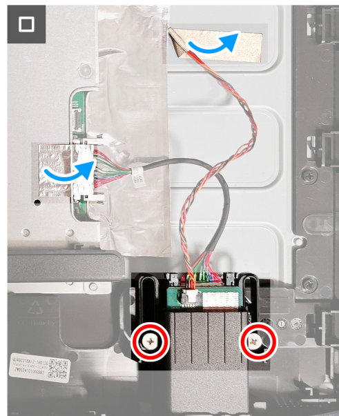
Rysunek 12. Instalacja koncentratora USB
