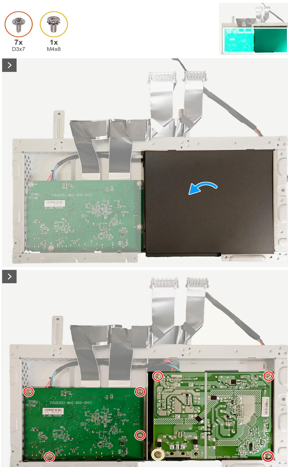
Rysunek 18. Zdejmowanie płyty systemowej i płyty zasilania
