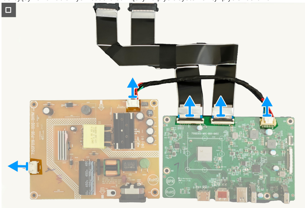
Rysunek 19. Zdejmowanie płyty systemowej i płyty zasilania
