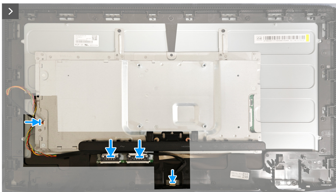
Rysunek 16. Instalacja metalowej ramki
