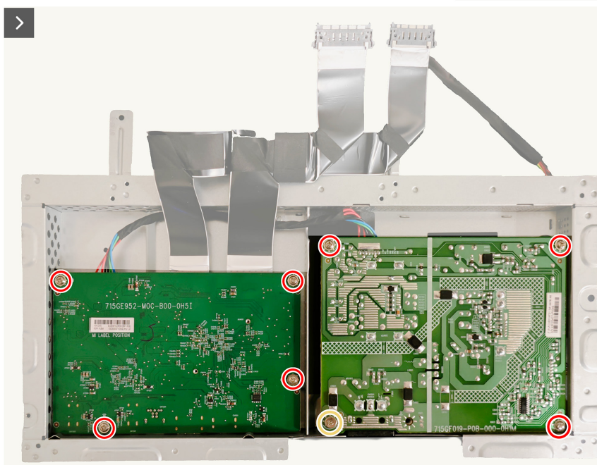
Rysunek 21. Instalacja płyty systemowej i płyty zasilania
