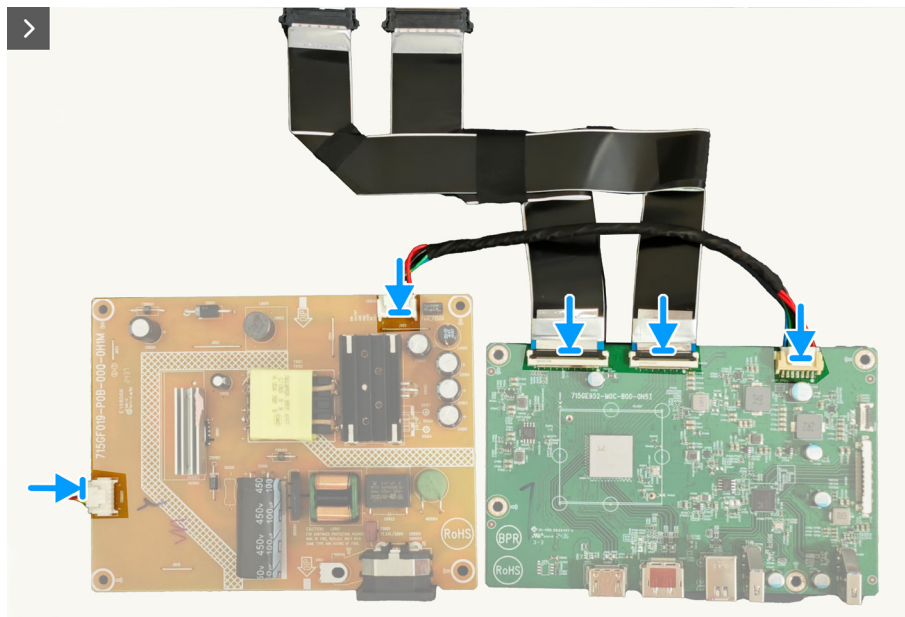
Rysunek 20. Instalacja płyty systemowej i płyty zasilania
