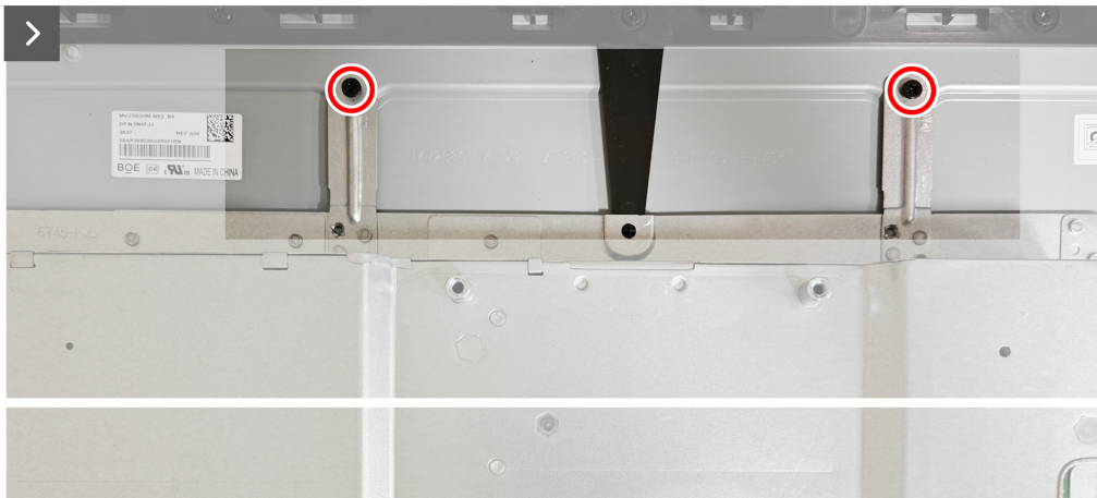
Rysunek 14. Zdejmowanie metalowej ramy
