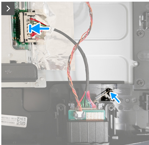
Rysunek 12. Instalacja koncentratora USB
