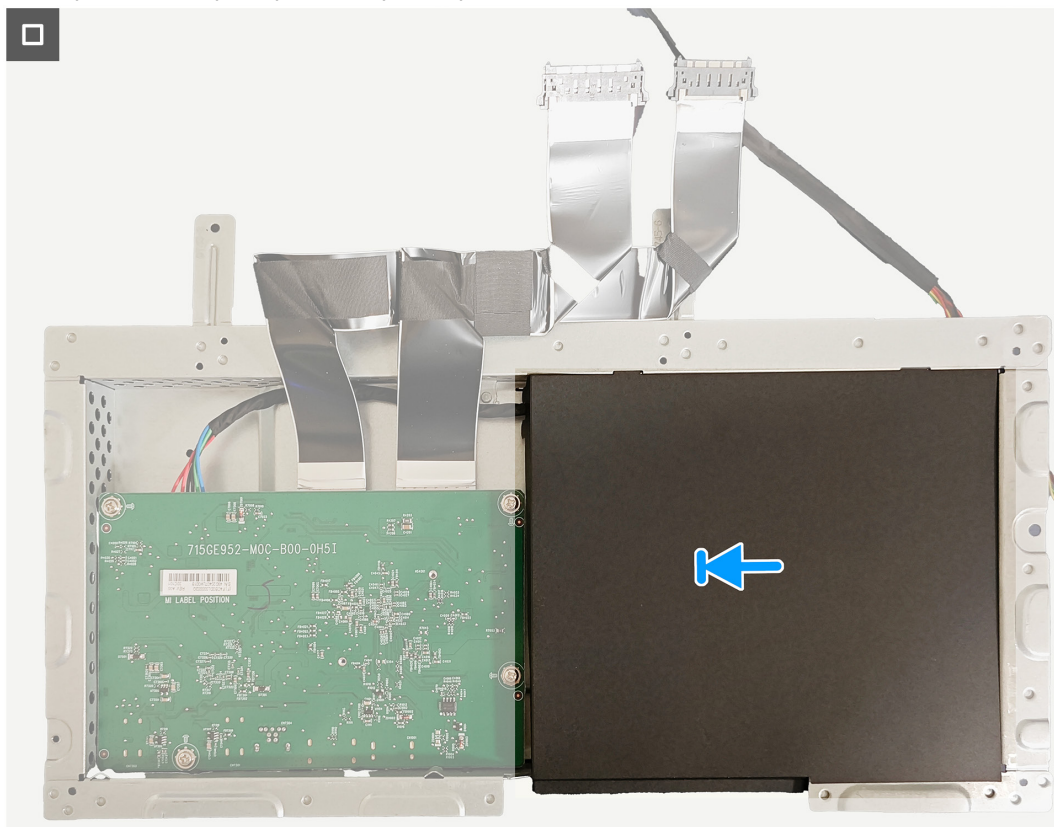
Rysunek 22. Instalacja płyty systemowej i płyty zasilania
