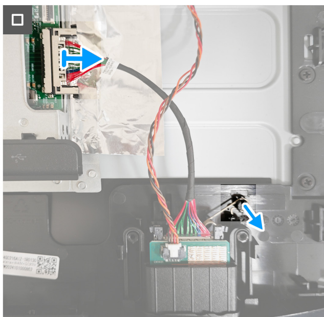
Rysunek 11. Zdejmowanie koncentratora USB
