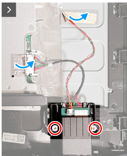
Rysunek 11. Zdejmowanie koncentratora USB
