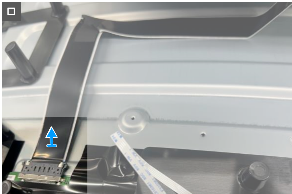
Figure 14. Enlever le blindage métallique
