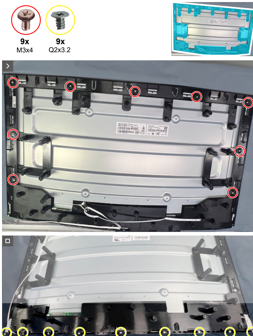
Figure 27. Installer le cadre central
