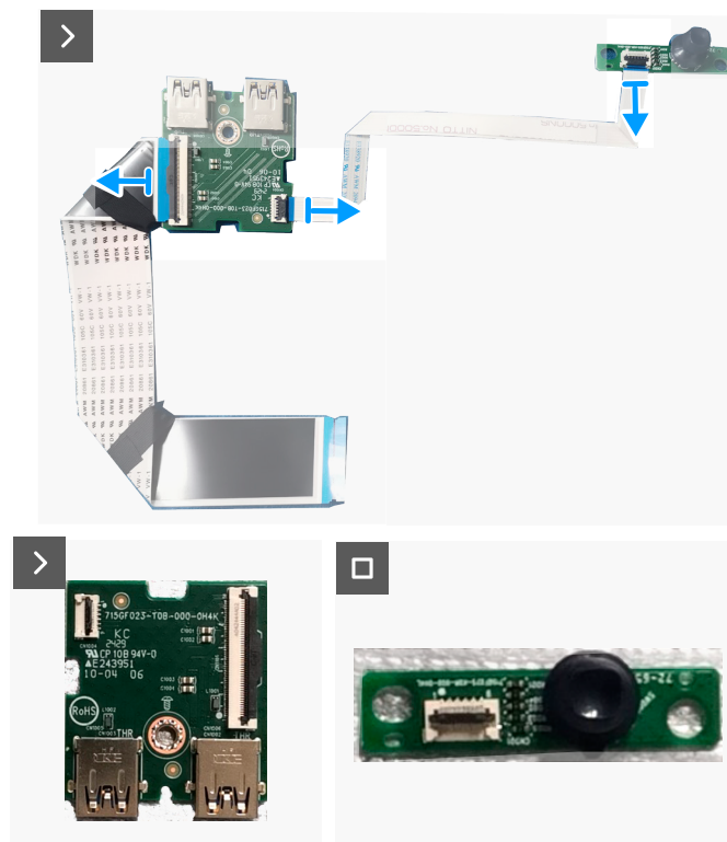
Figure 32. Enlever la carte d'E/S et la carte du bouton-joystick
