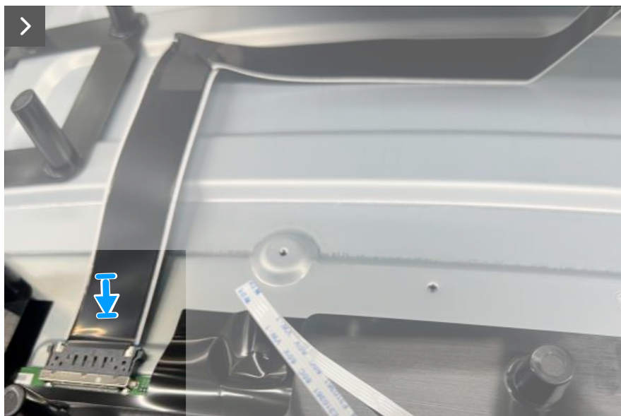
Figure 15. Installer le blindage métallique
