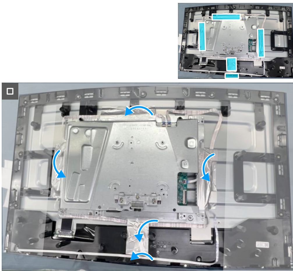
Figure 19. Installer le blindage métallique
