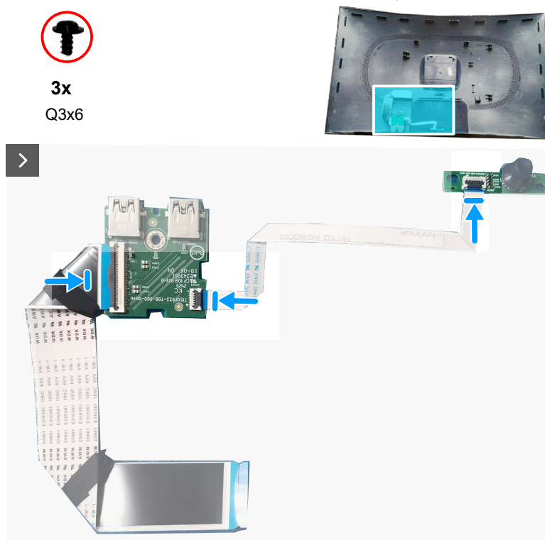
Figure 33. Installer la carte d'E/S et la carte du bouton-joystick
