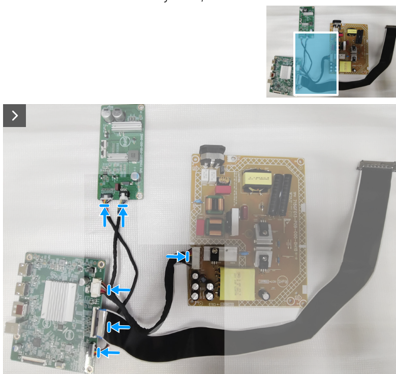
Figure 23. Installer la carte du système et la carte d'alimentation
