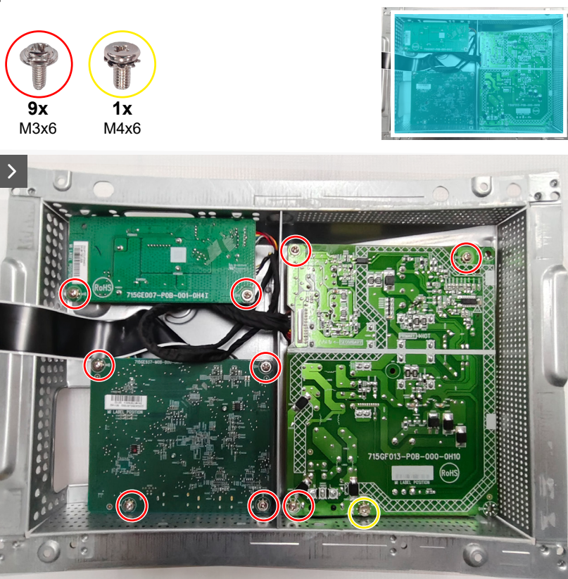
Figure 24. Installer la carte du système et la carte d'alimentation
