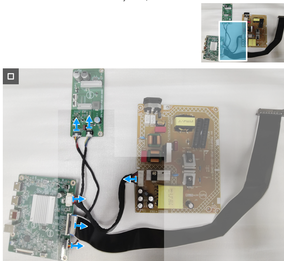
Figure 22. Enlever la carte du système et la carte d'alimentation
