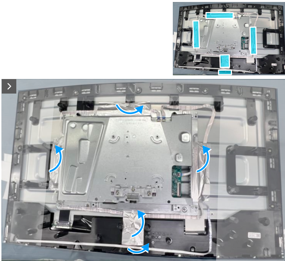
Figure 10. Enlever le blindage métallique
