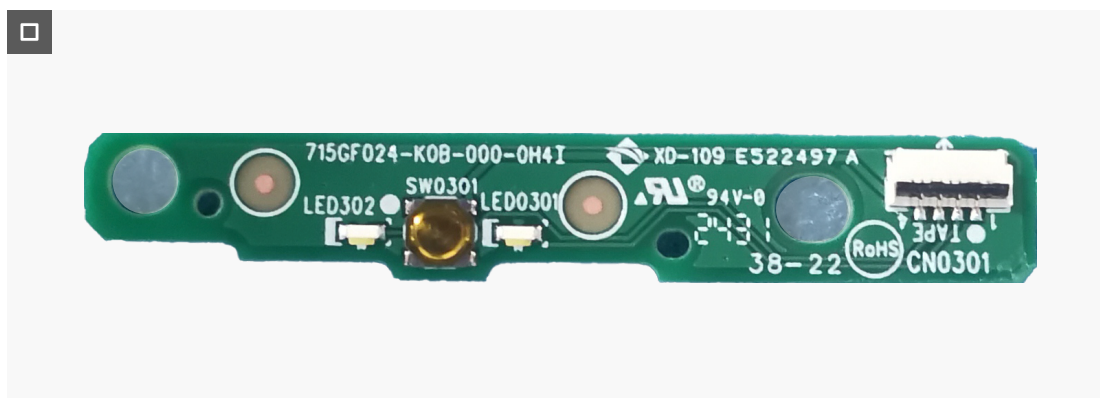
Figure 29. Enlever la carte du bouton-alimentation
