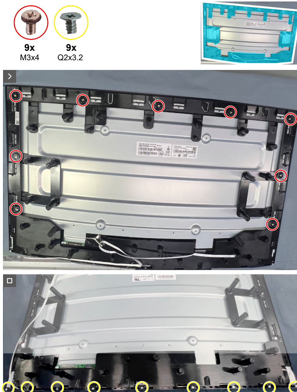
Figure 26. Enlever le cadre central
