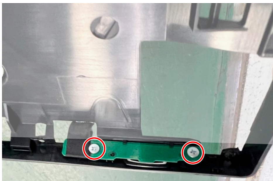
Figure 30. Installer la carte du bouton-alimentation
