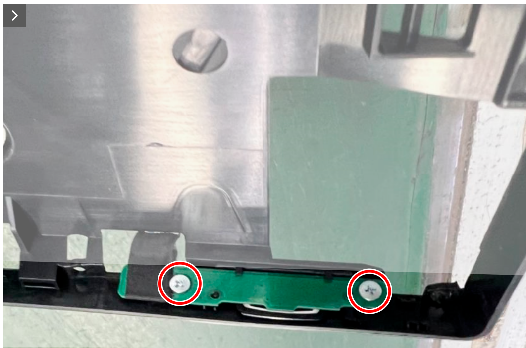
Figure 28. Enlever la carte du bouton-alimentation
