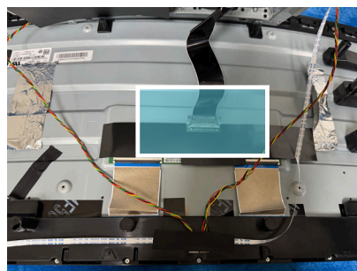
Figure 13. Enlever le blindage métallique
