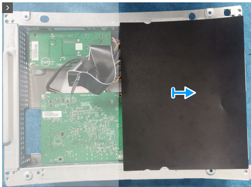
Figure 20. Enlever la carte du système et la carte d'alimentation
