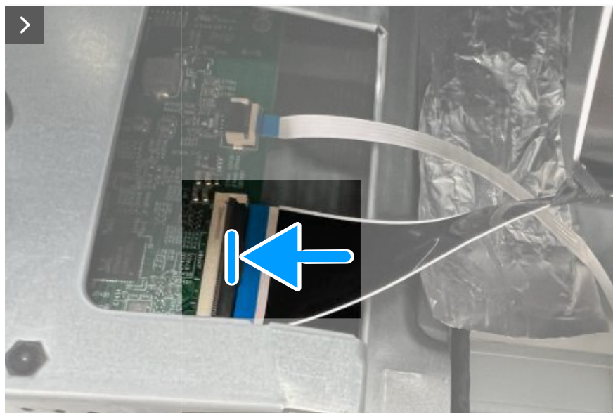
Figure 7. Installer le couvercle arrière
