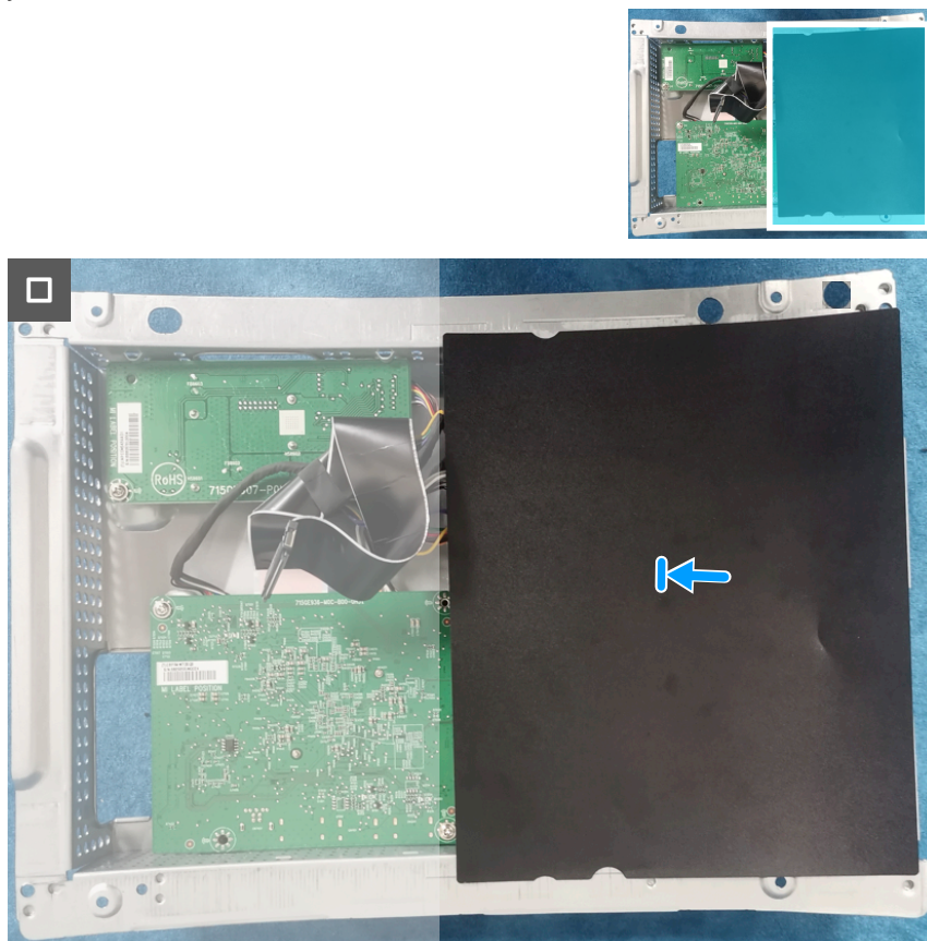
Figure 25. Installer la carte du système et la carte d'alimentation
