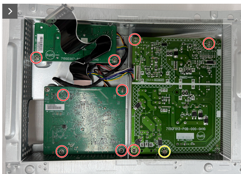
Figure 24. Installer la carte du système et la carte d'alimentation
