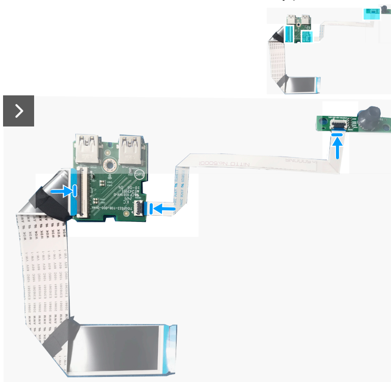
Figure 33. Installer la carte d'E/S et la carte du bouton-joystick
