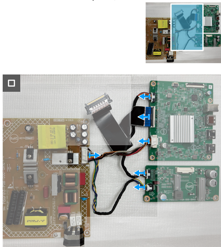
Figure 22. Enlever la carte du système et la carte d'alimentation
