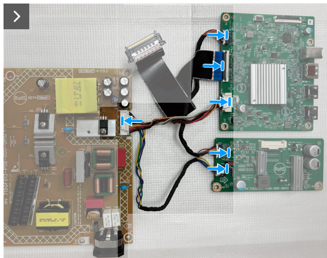
Figure 23. Installer la carte du système et la carte d'alimentation
