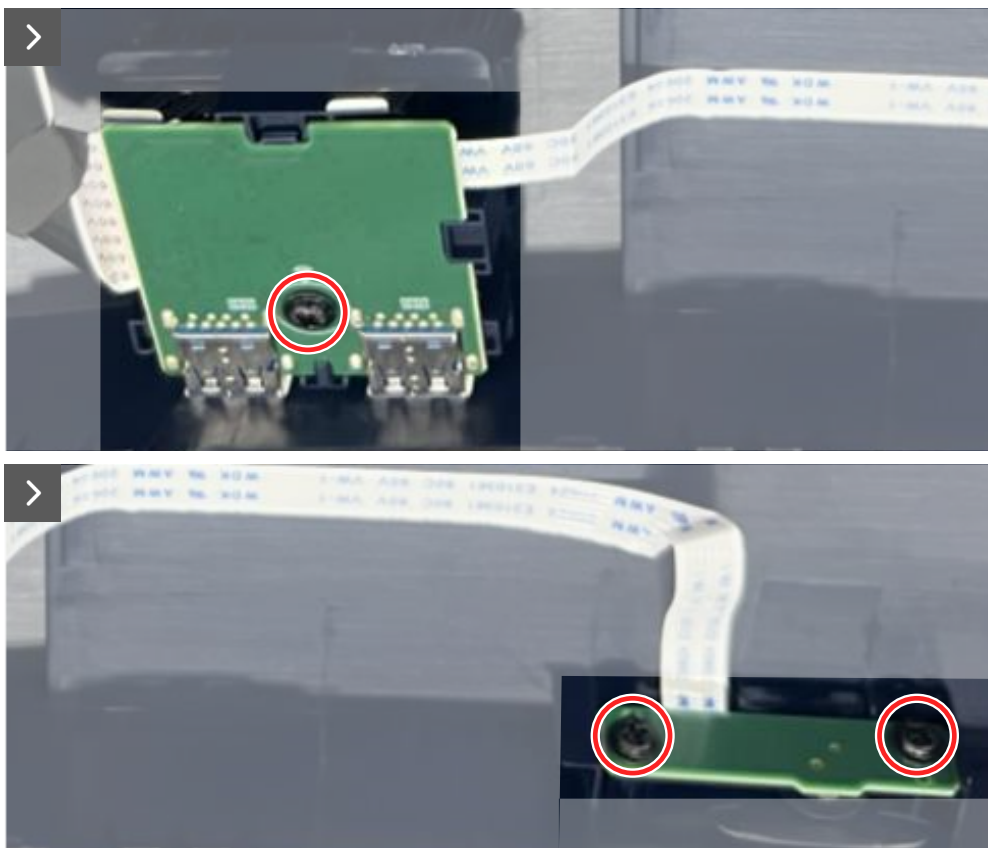
Figure 31. Enlever la carte d'E/S et la carte du bouton-joystick
