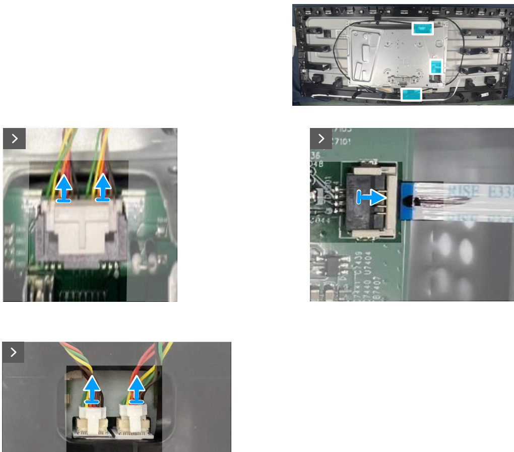
Figure 11. Enlever le blindage métallique
