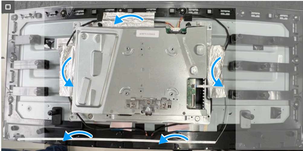
Figure 19. Installer le blindage métallique
