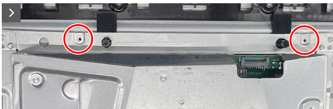
Figure 12. Enlever le blindage métallique
