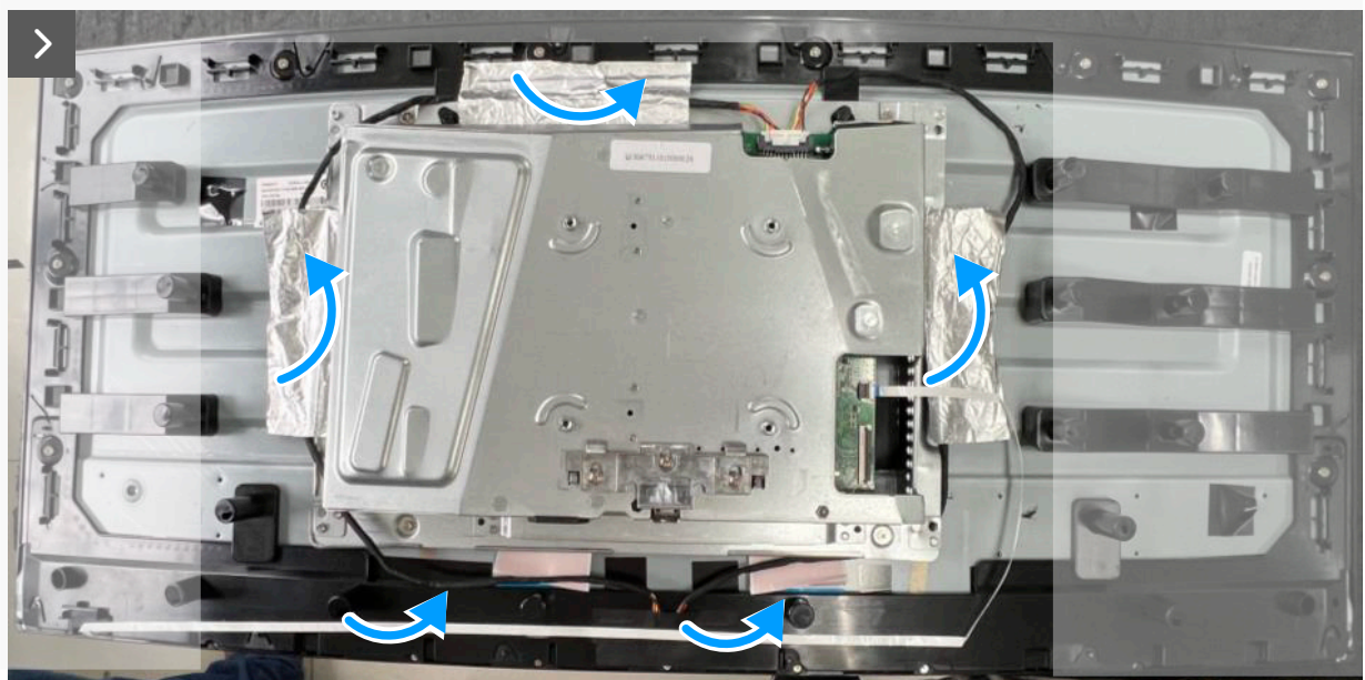
Figure 10. Enlever le blindage métallique
