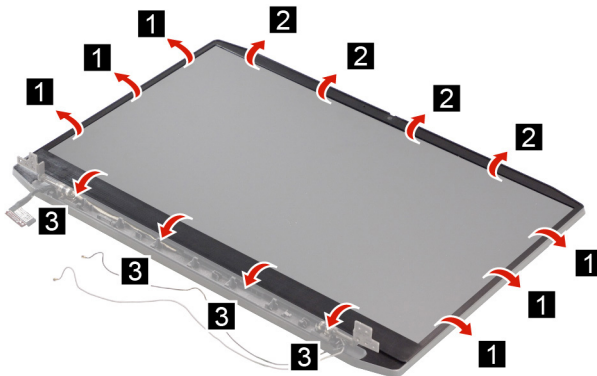
Figure 29. Remove the LCD bezel
