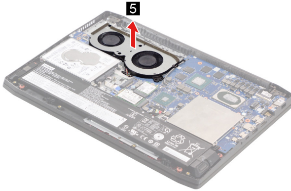
Figure 17. Remove the fan
