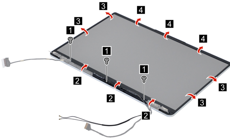
Figure 25. Remove the LCD bezel
