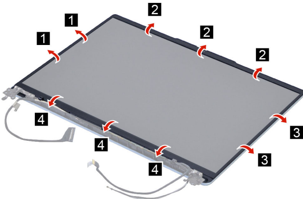
Figure 29. Remove the LCD bezel
