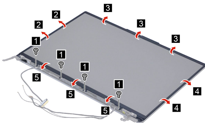
Figure 27. Remove the LCD bezel
