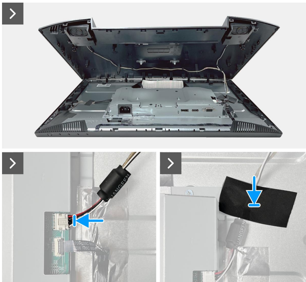
Rysunek 5. Instalowanie tylnej pokrywy
