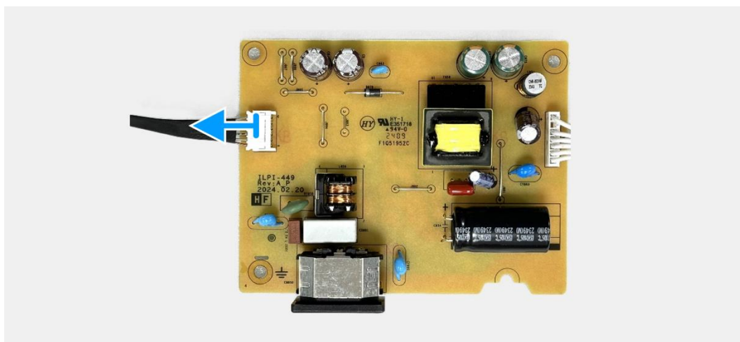
Rysunek 43. Wyjmowanie płyty zasilania
