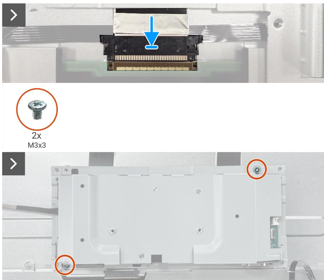
Rysunek 11. Instalowanie zespołu obudowy
