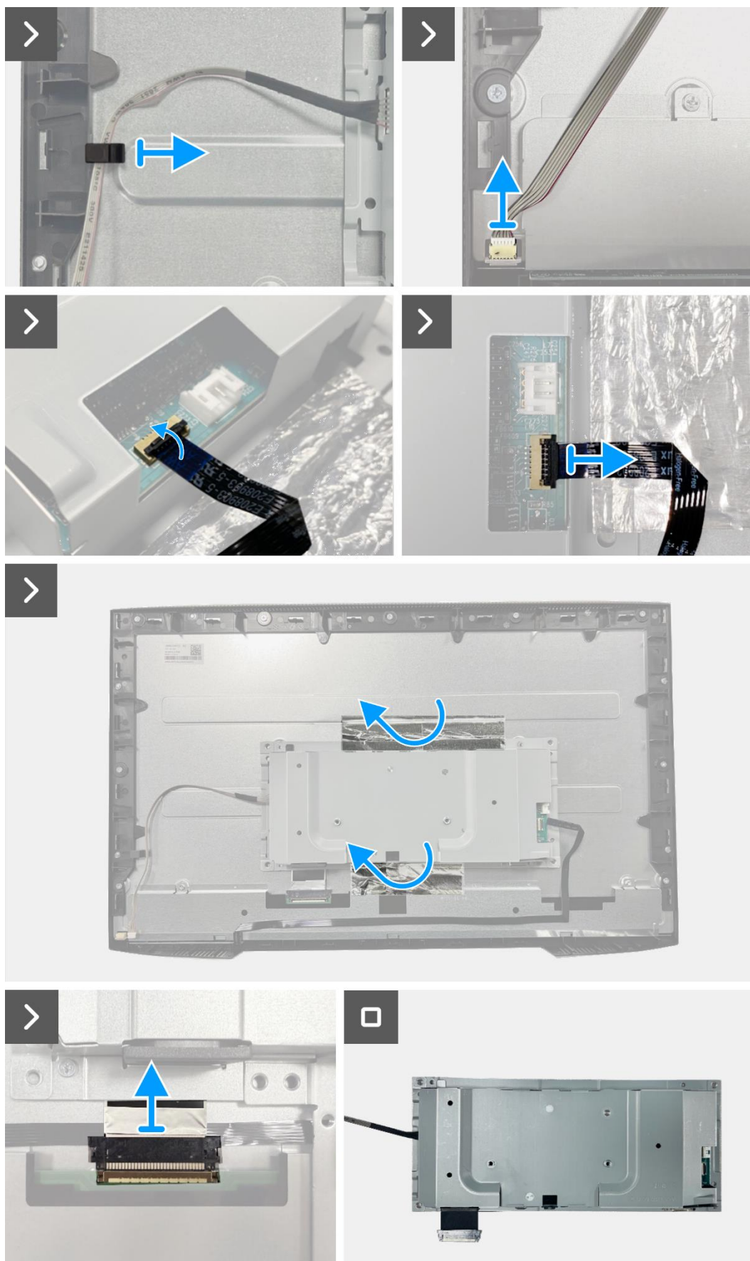
Rysunek 32. Demontaż zespołu obudowy
