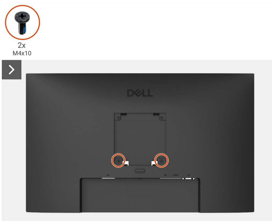
Rysunek 3. Zdejmowanie tylnej pokrywy
