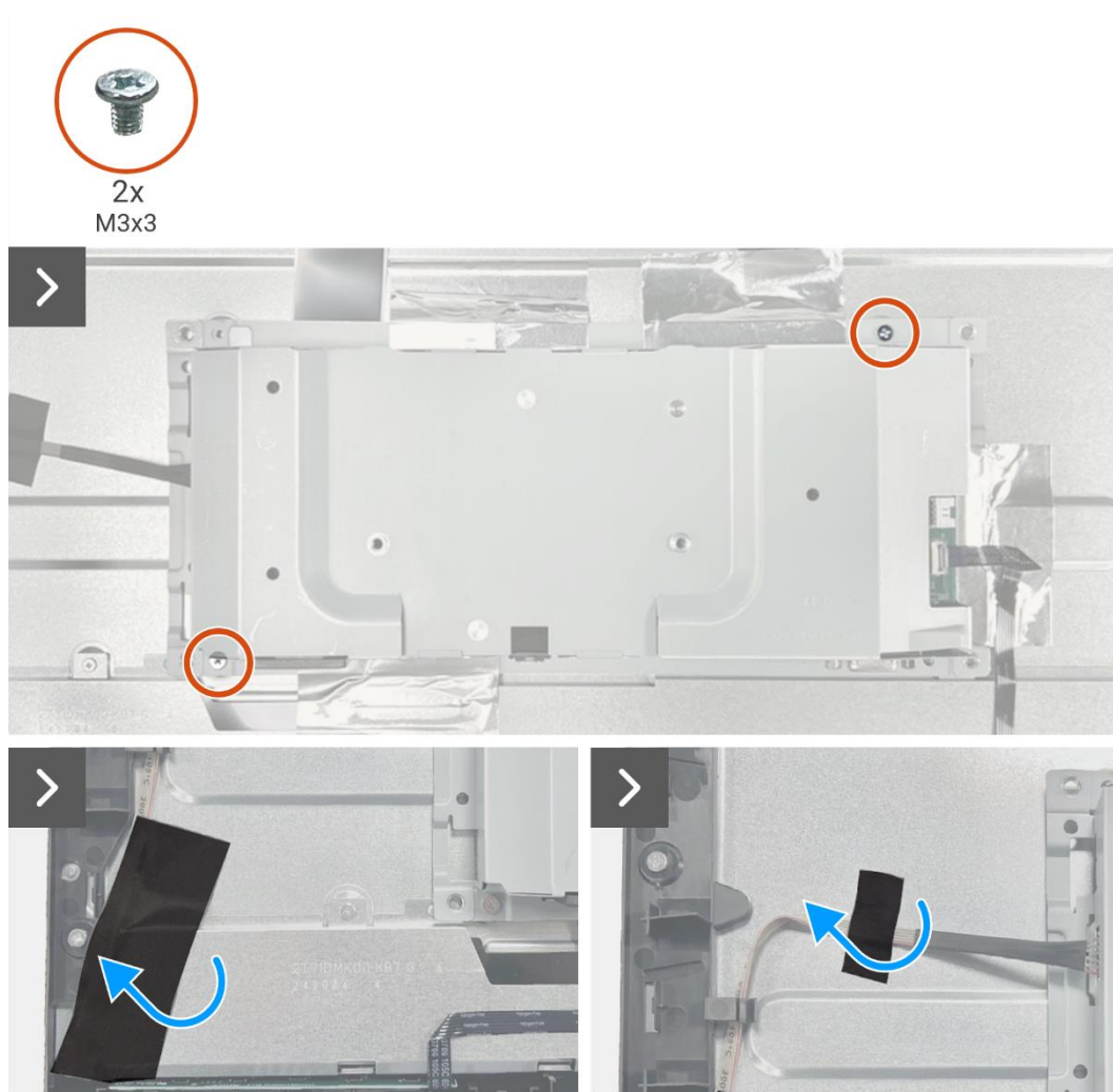
Rysunek 9. Demontaż zespołu obudowy
