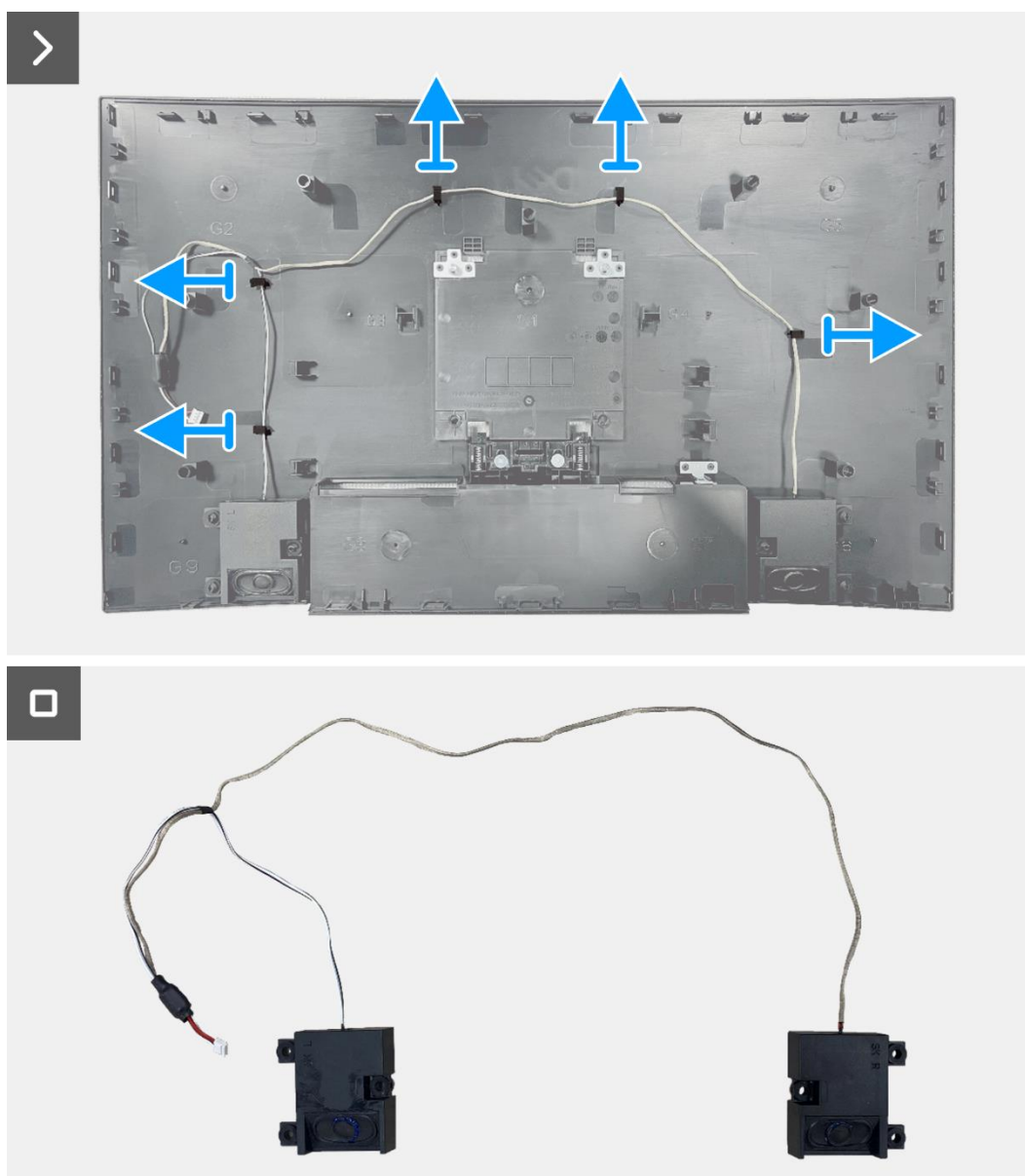
Rysunek 29. Demontaż głośników
