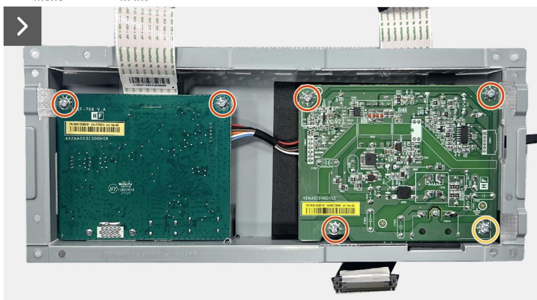
Rysunek 16. Wyjmowanie karty interfejsu
