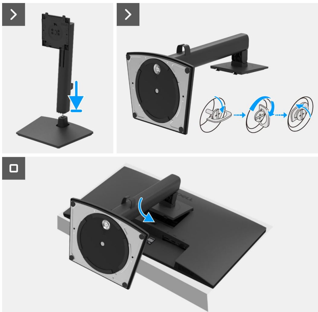
Rysunek 2. Montaż podstawy
