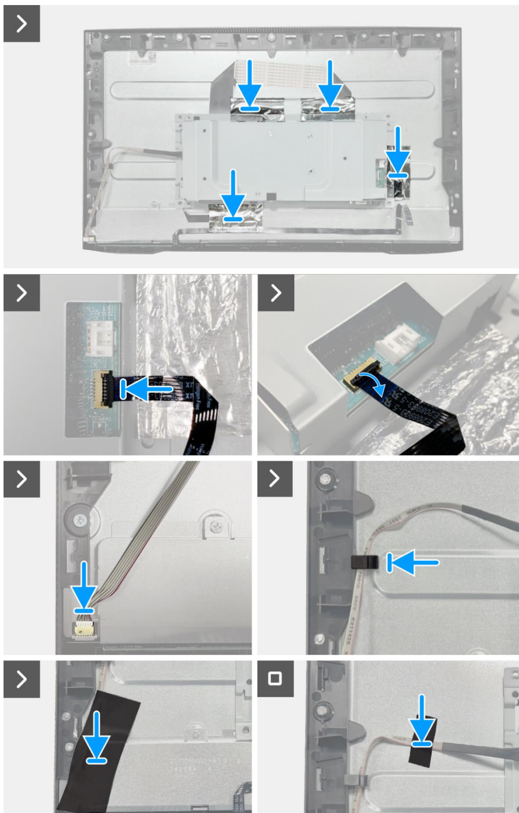
Rysunek 12. Instalowanie zespołu obudowy
