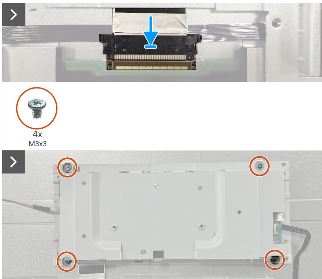
Obrázek 33. Instalace sestavy šasi
