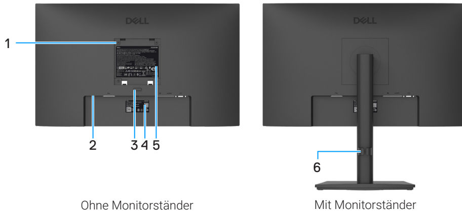
Abbildung 2. Rückansicht
