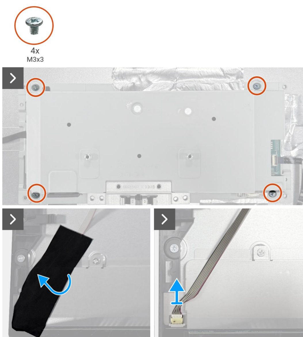
Obrázek 6. Odmontování sestavy šasi
