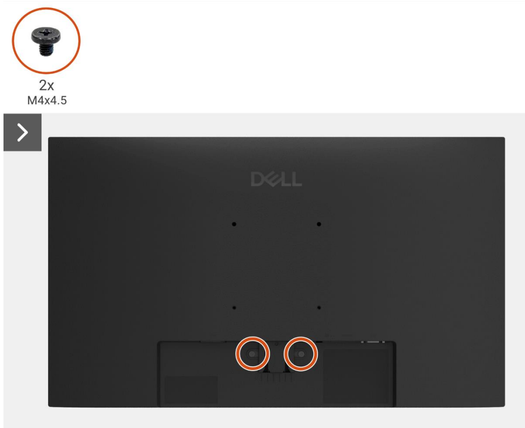
Obrázek 3. Odmontování zadního krytu
