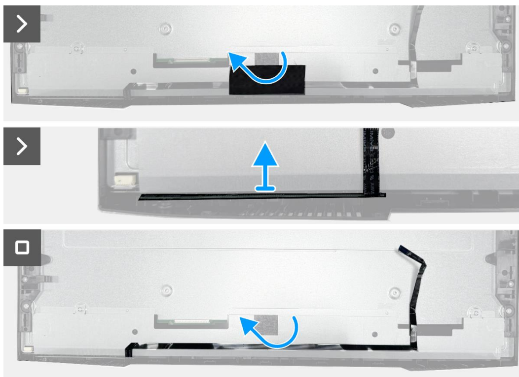
Obrázek 10. Odmontování desky klávesnice
