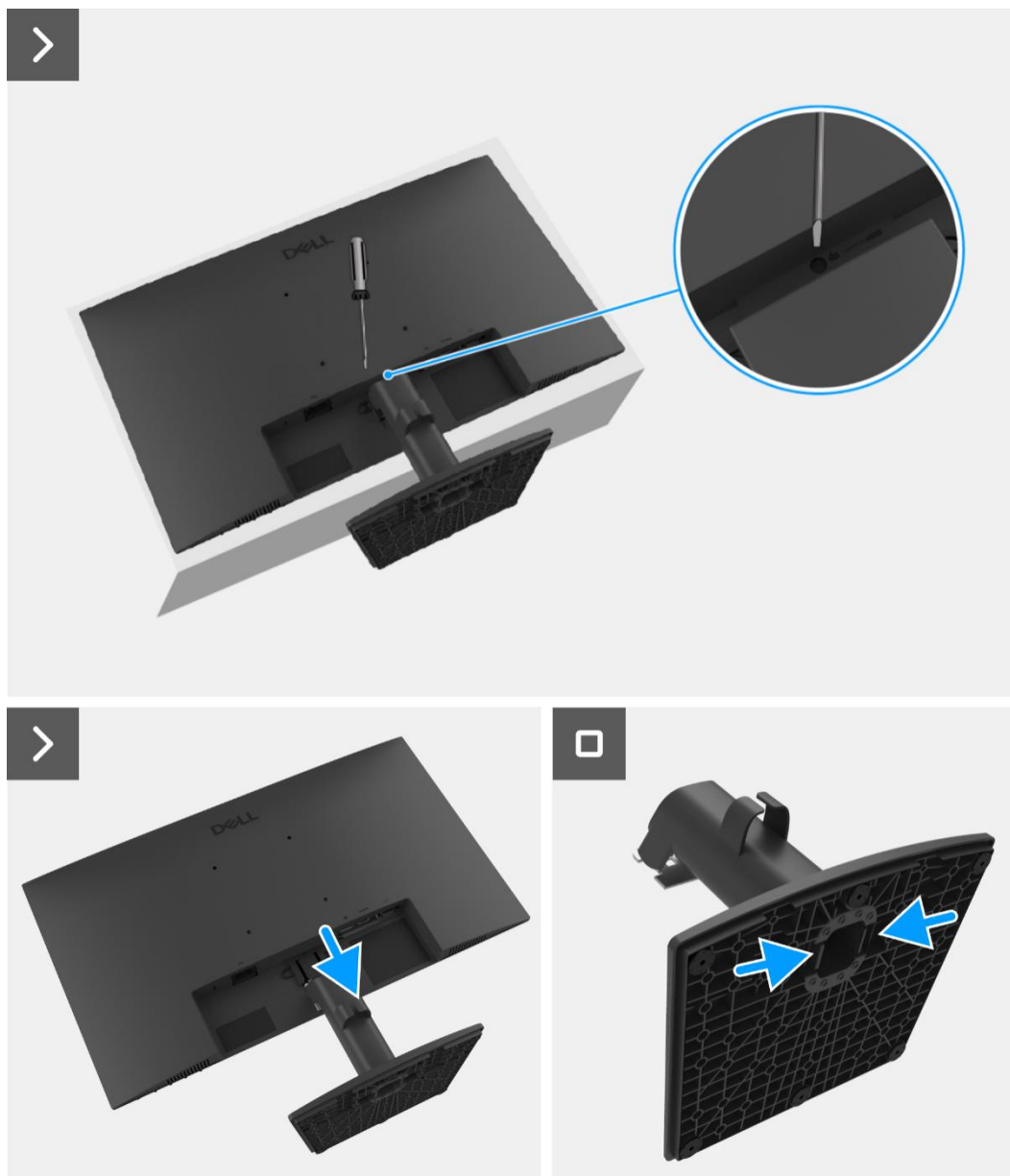
Obrázek 1. Odmontování stojanu
