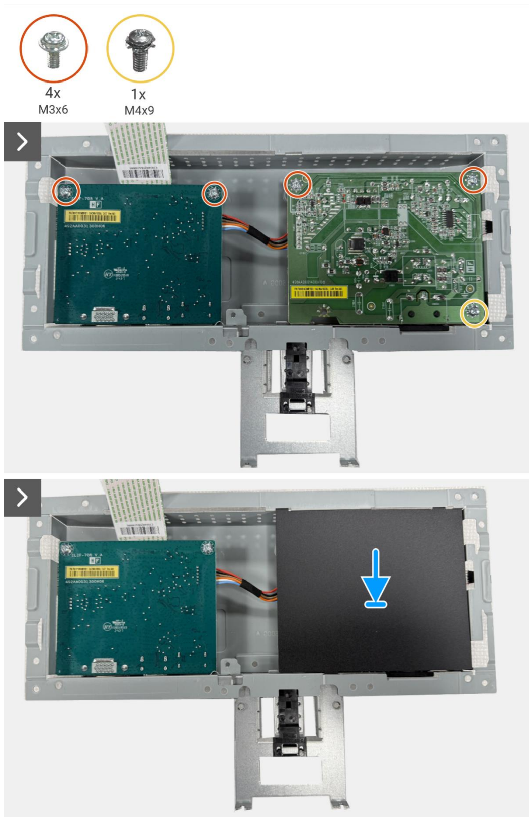
Obrázek 16. Instalace desky rozhraní
