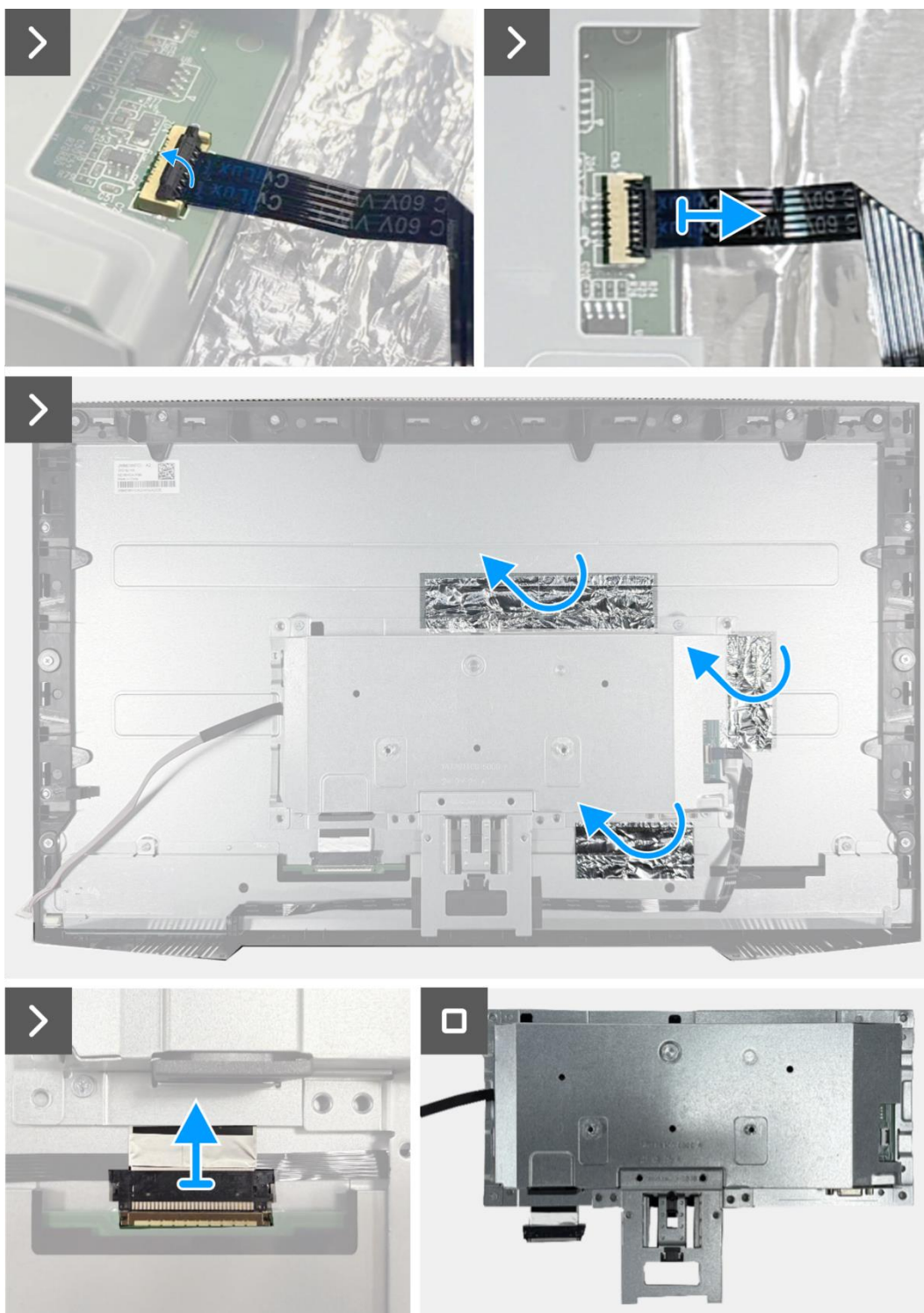
Obrázek 7. Odmontování sestavy šasi
