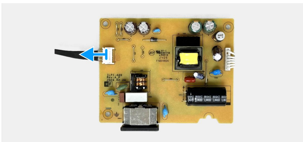
Obrázek 18. Odmontování napájecí desky
