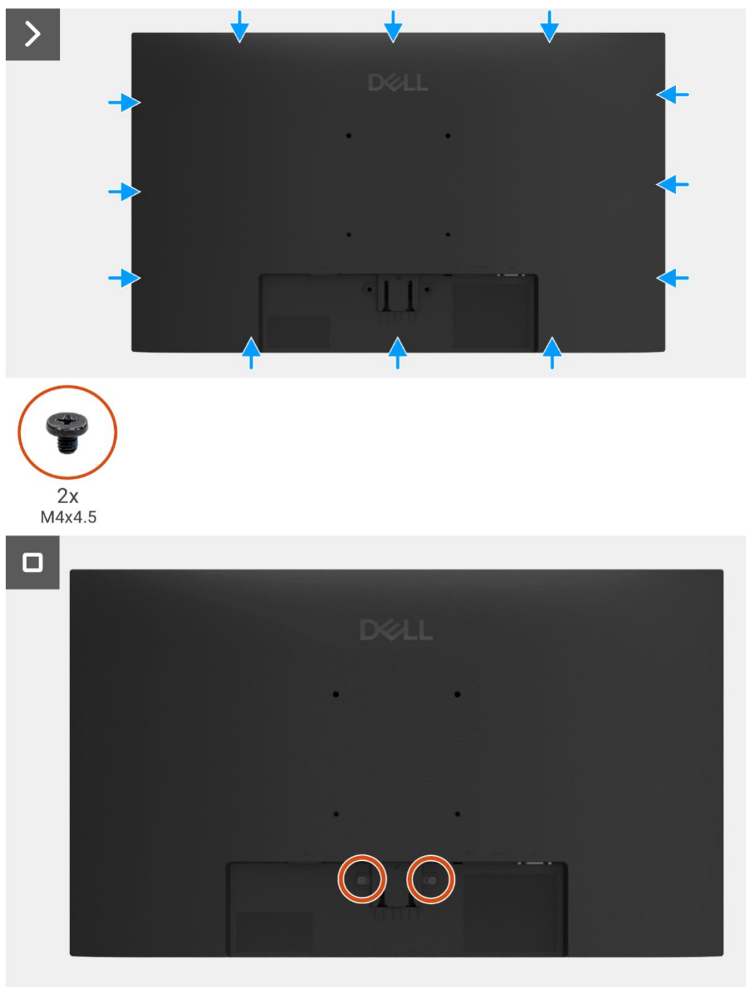
Obrázek 5. Instalace zadního krytu
