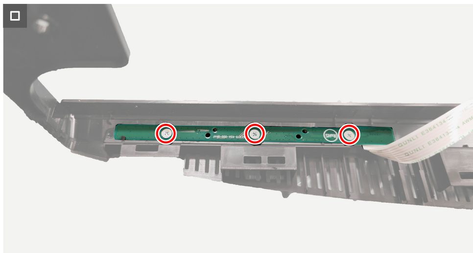
Obrázek 11. Instalace tlačítkové desky
