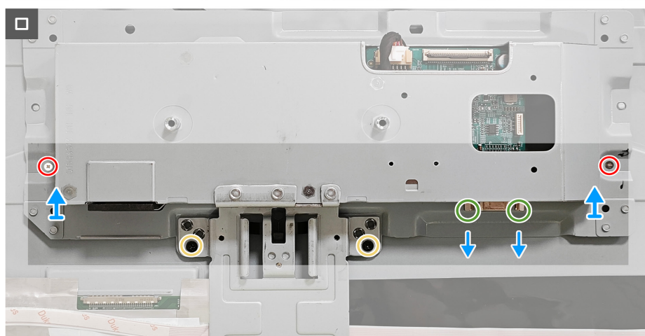
Obrázek 7. Demontáž kovového krytu
