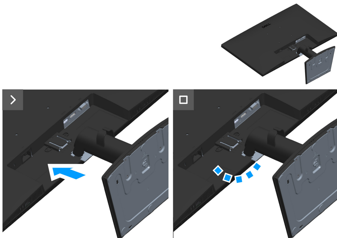
Obrázek 2. Instalace stojánu
