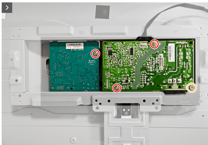
Obrázek 12. Demontáž systémové desky a napájecí desky
