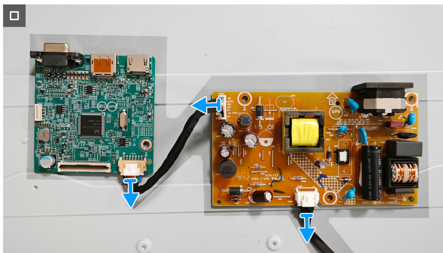
Obrázek 13. Demontáž systémové desky a napájecí desky
