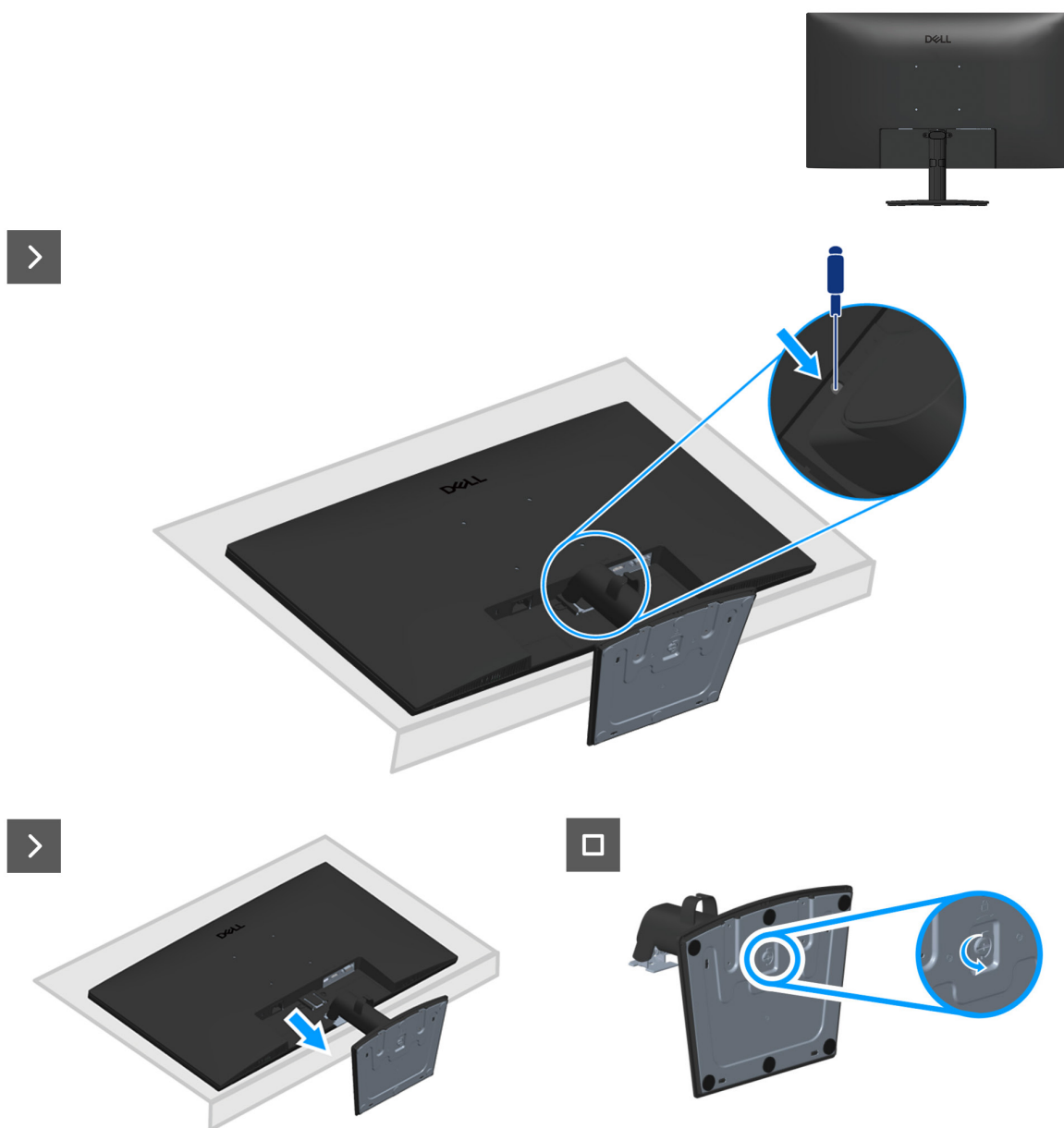
Obrázek 1. Demontáž stojánku
