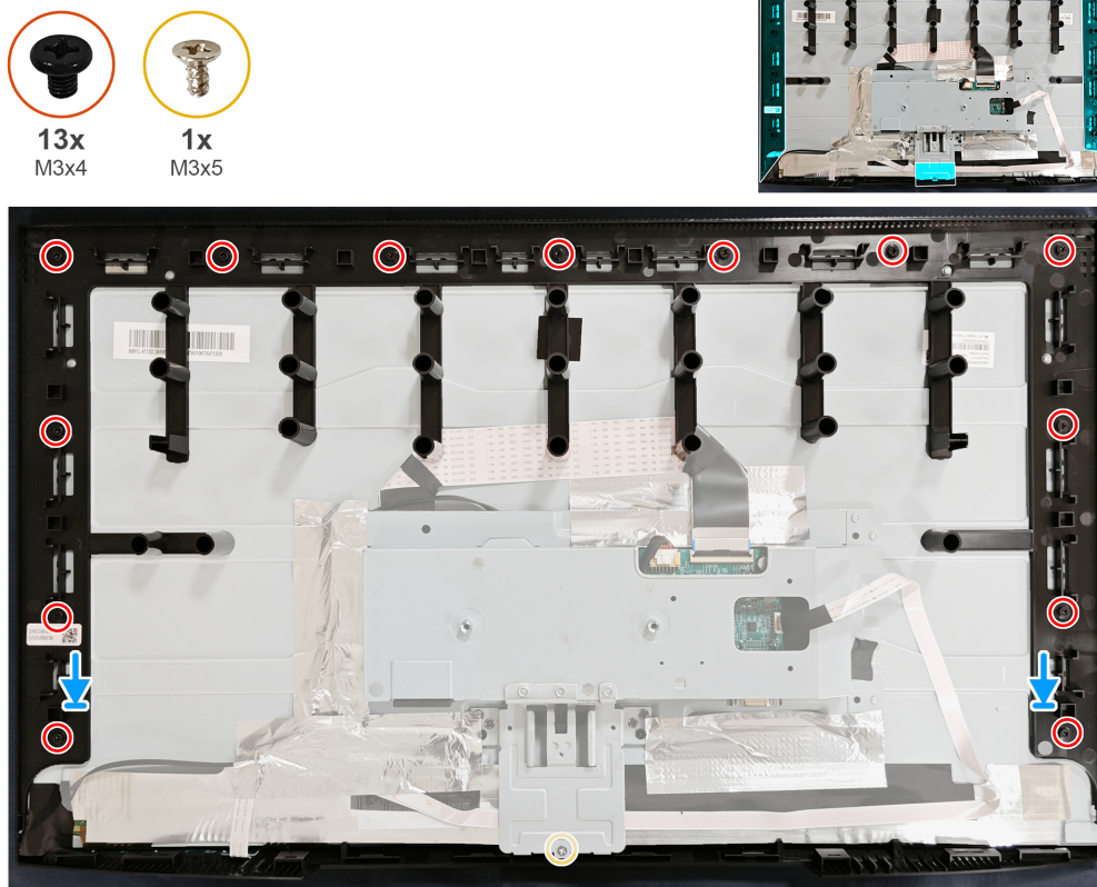
Obrázek 6. Instalace středního rámu
