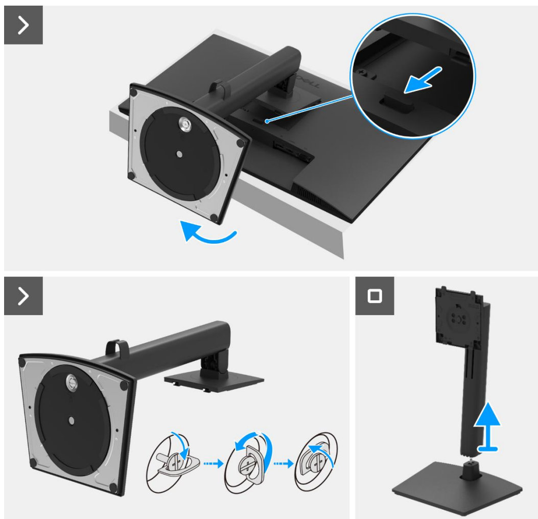
Rysunek 1. Demontaż podstawy
