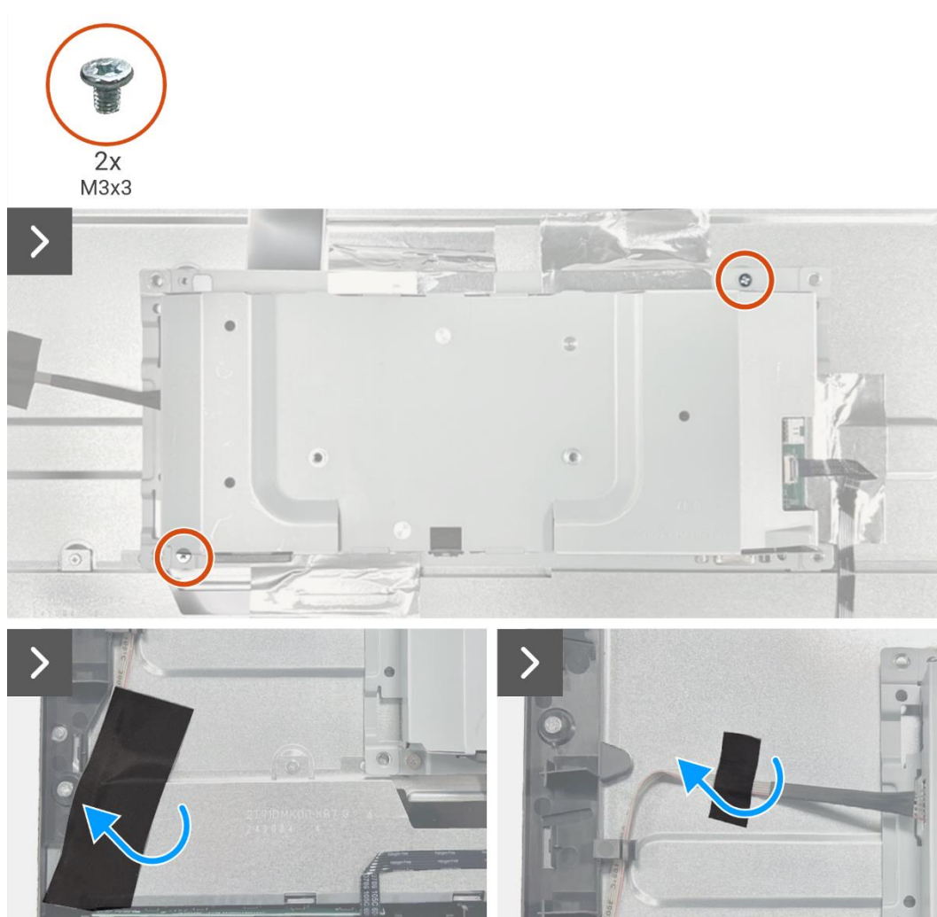
Rysunek 9. Demontaż zespołu obudowy
