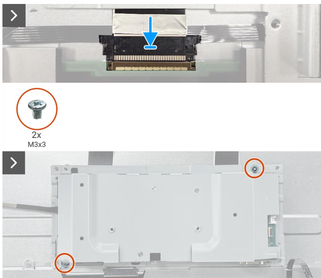
Obrázek 11. Instalace sestavy šasi
