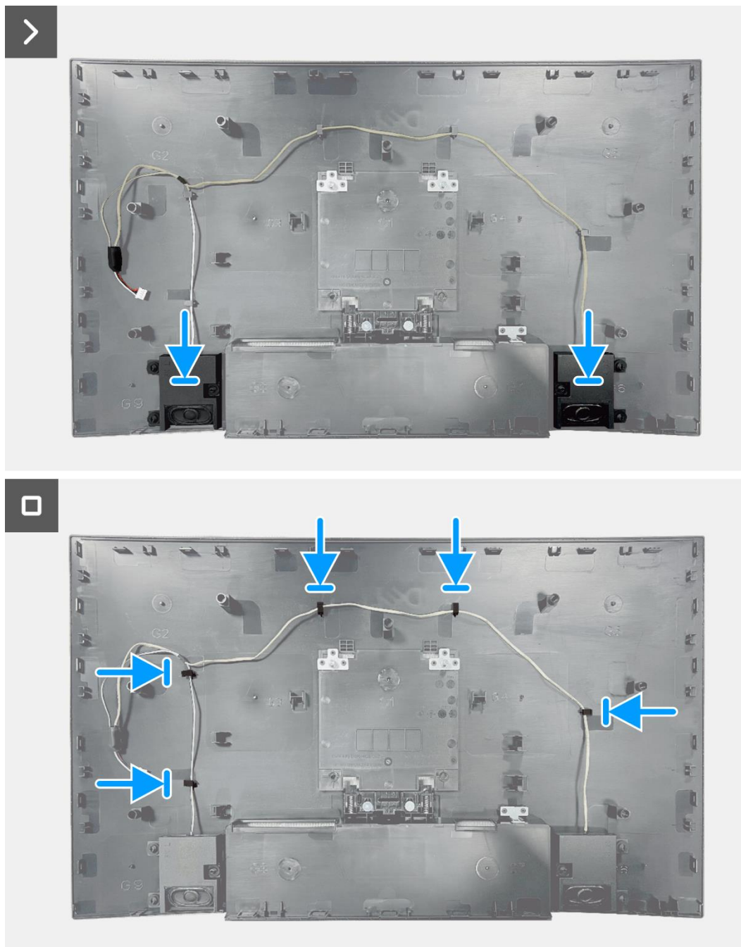
Obrázek 8. Instalace reproduktorů
