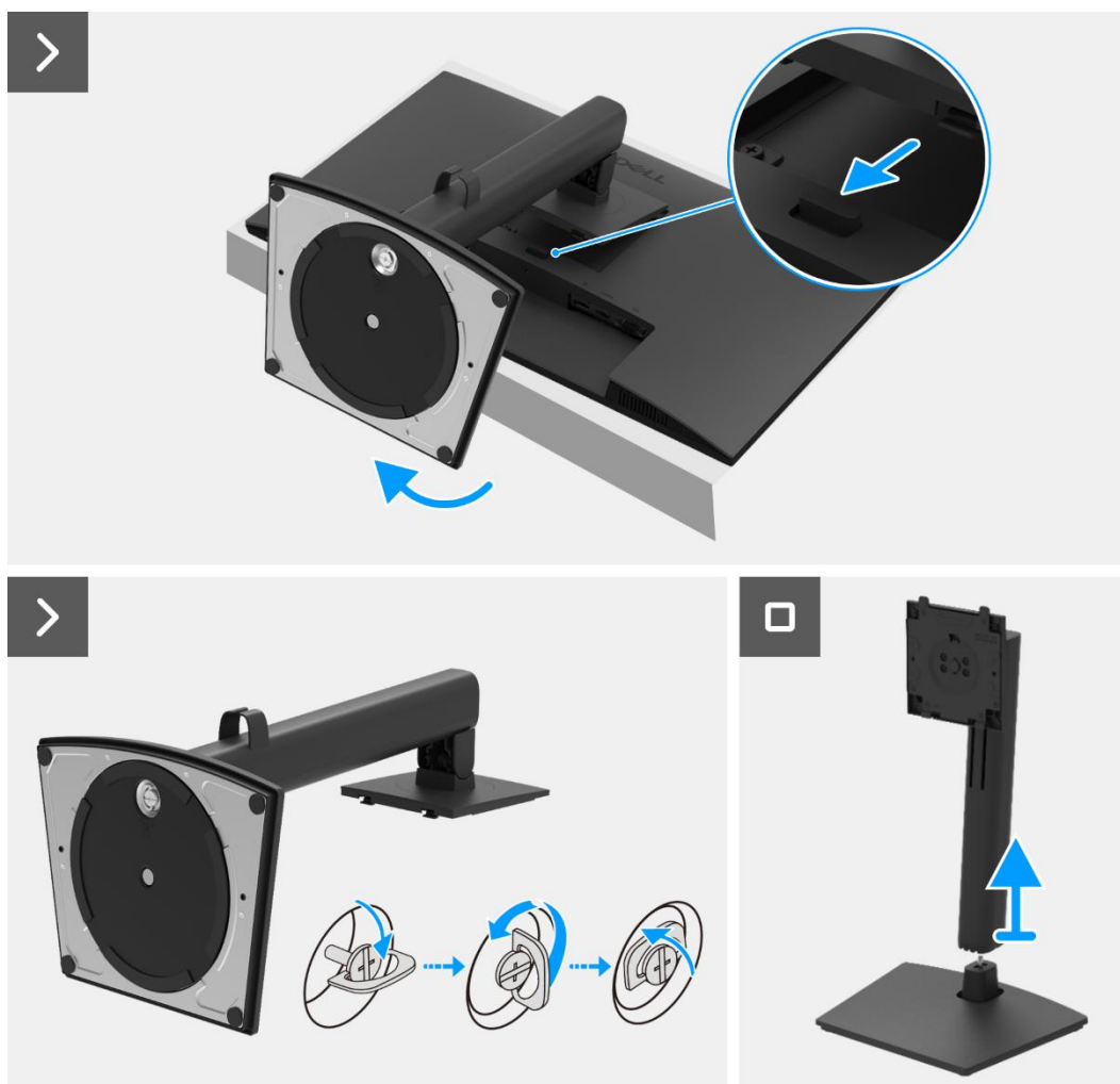
Obrázek 23. Odmontování stojanu
