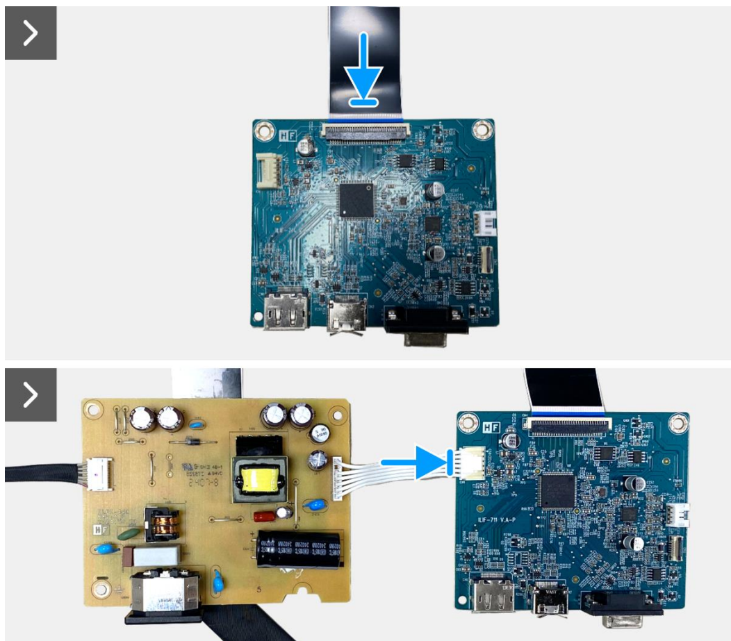
Obrázek 40. Instalace desky rozhraní
