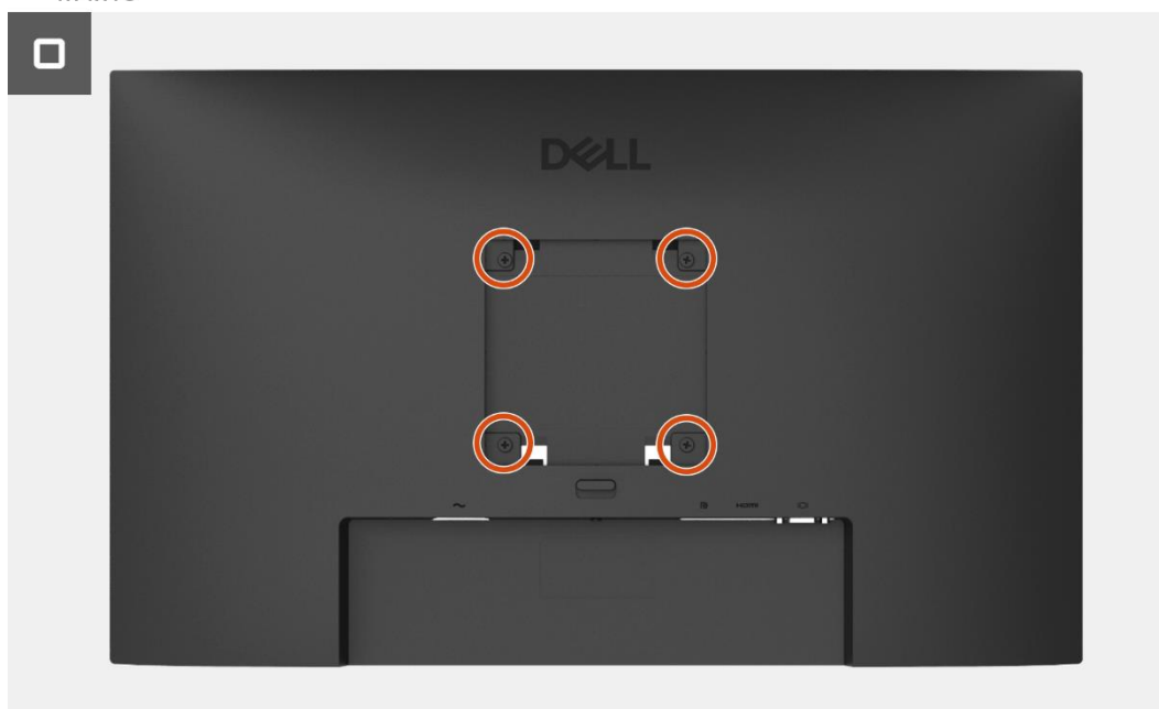
Obrázek 28. Instalace zadního krytu
