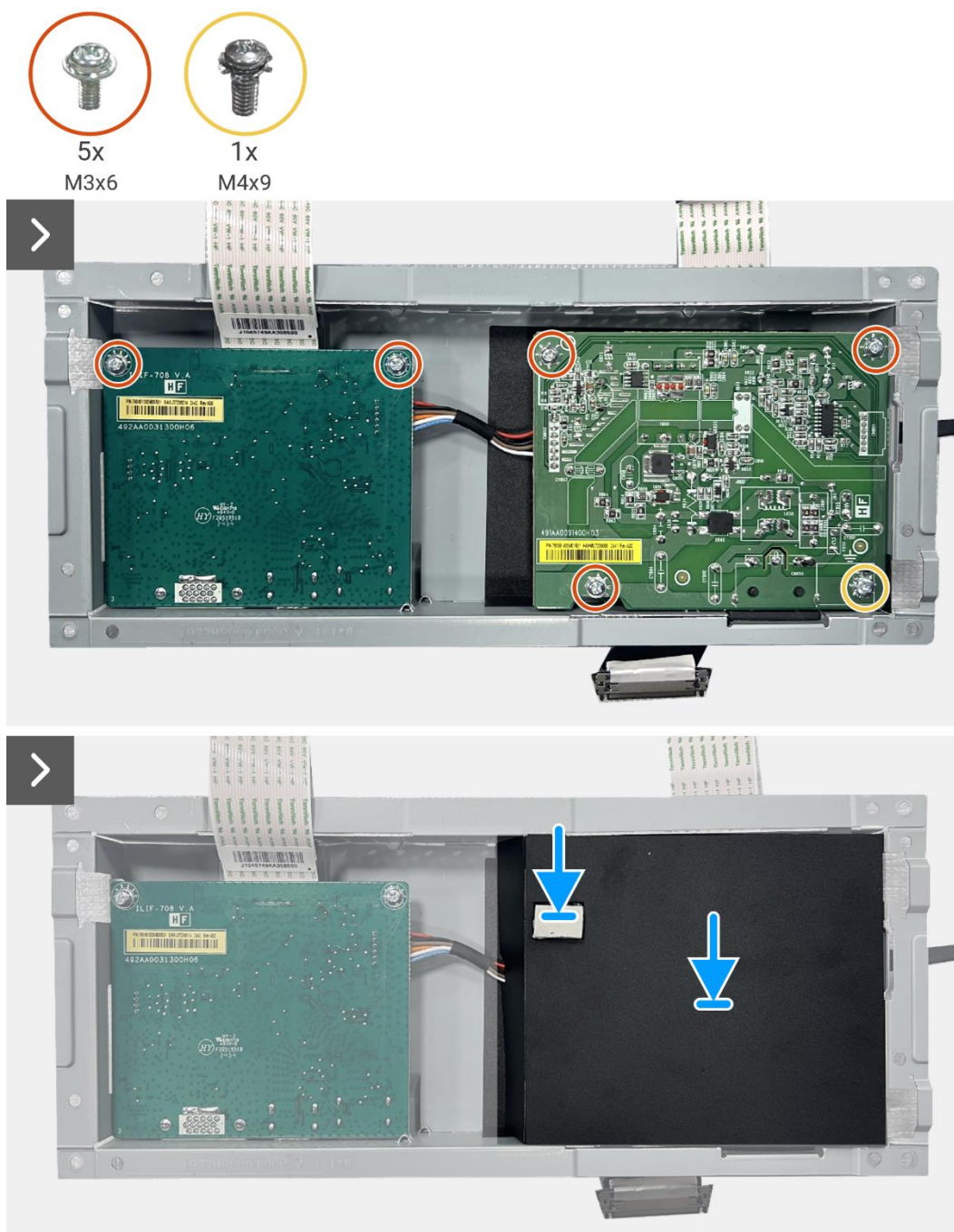
Obrázek 41. Instalace desky rozhraní
