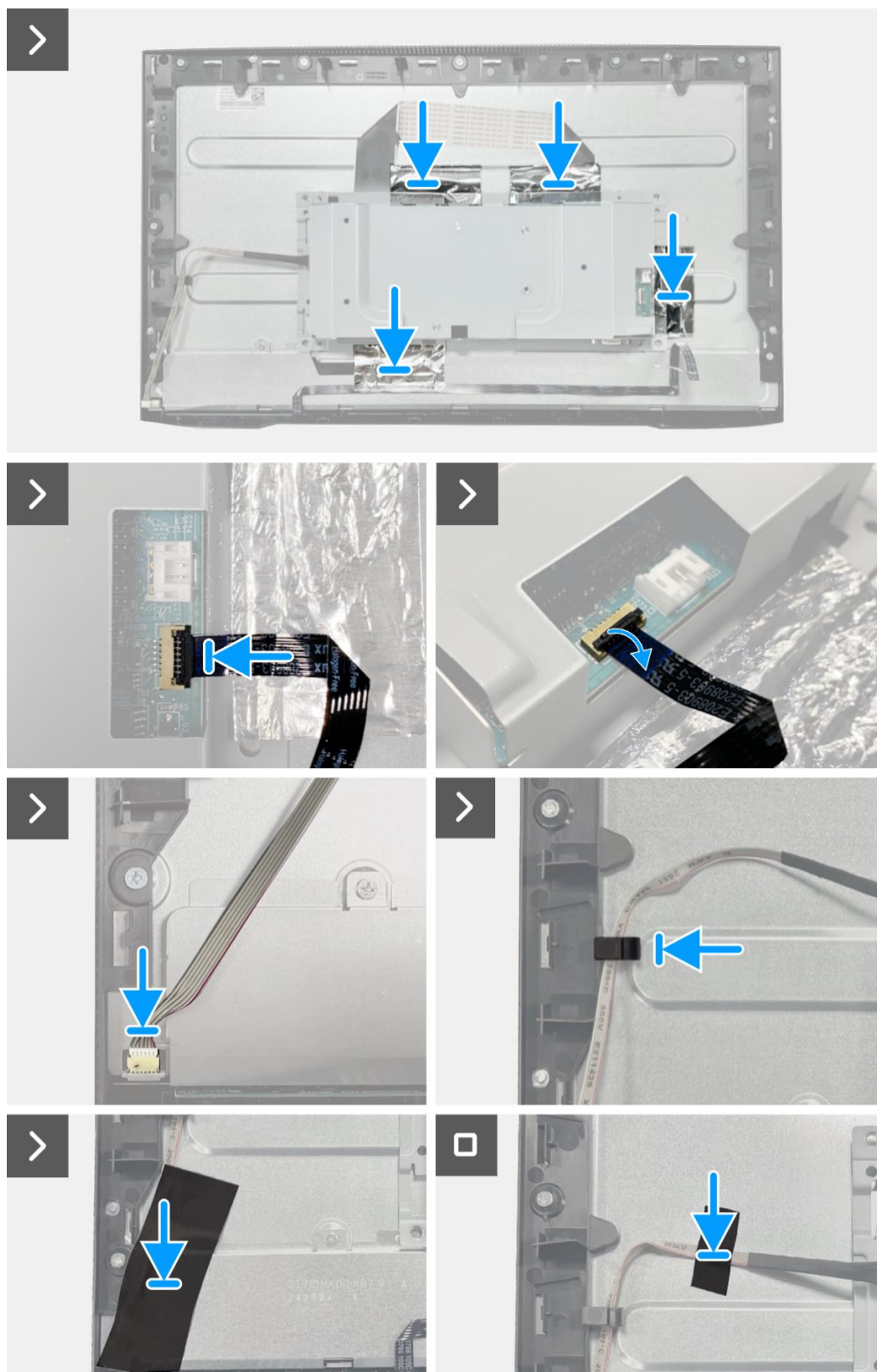
Obrázek 12. Instalace sestavy šasi
