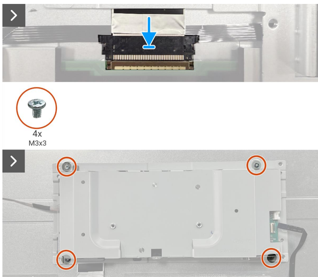
Obrázek 33. Instalace sestavy šasi
