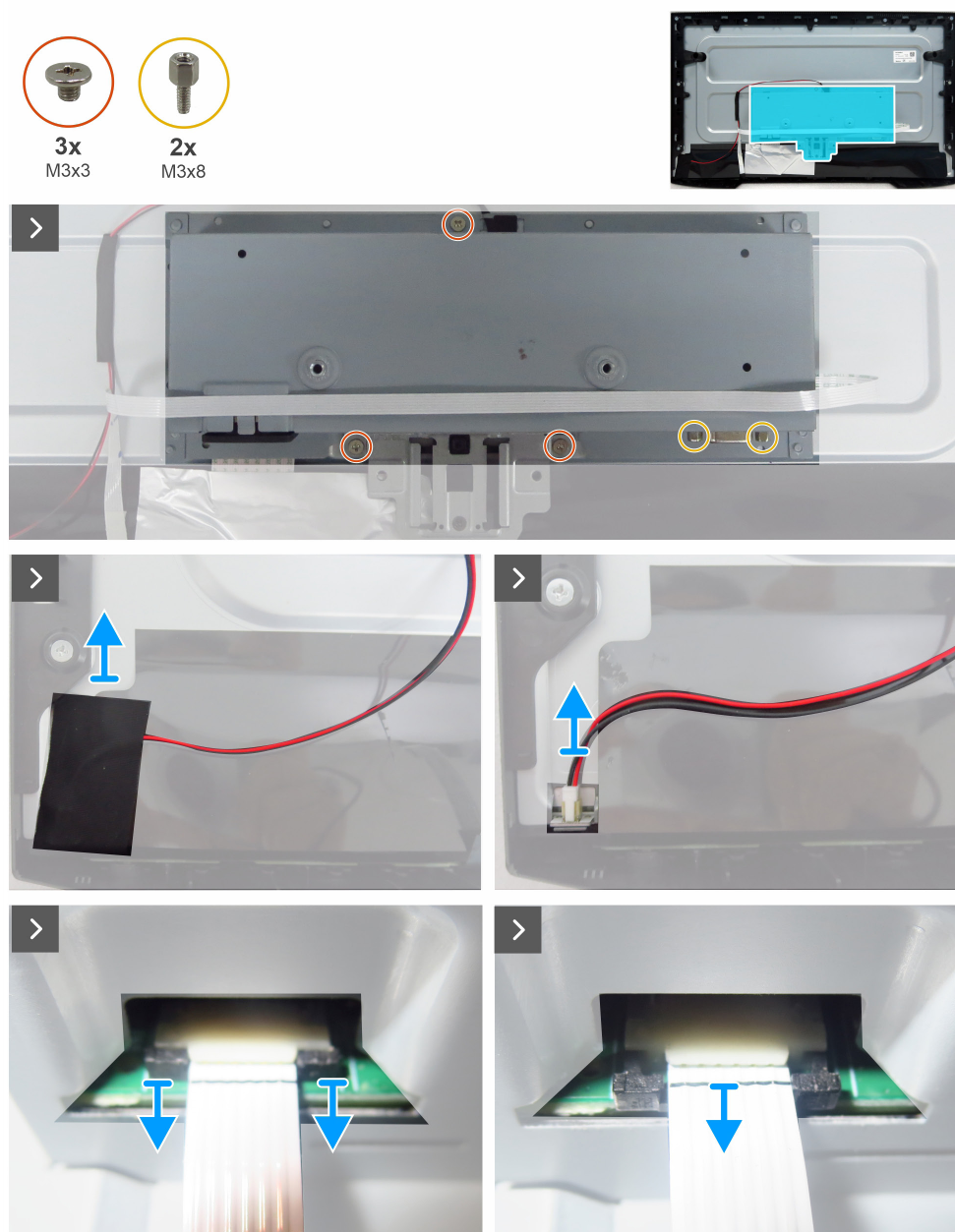
Obrázek 5. Demontáž hlavního šasi
