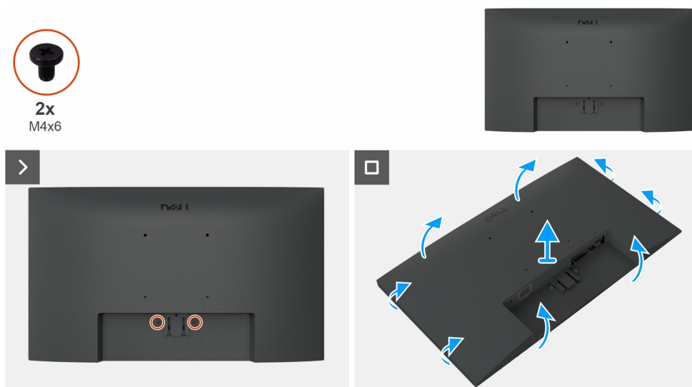
Obrázek 3. Sejmutí zadního krytu
