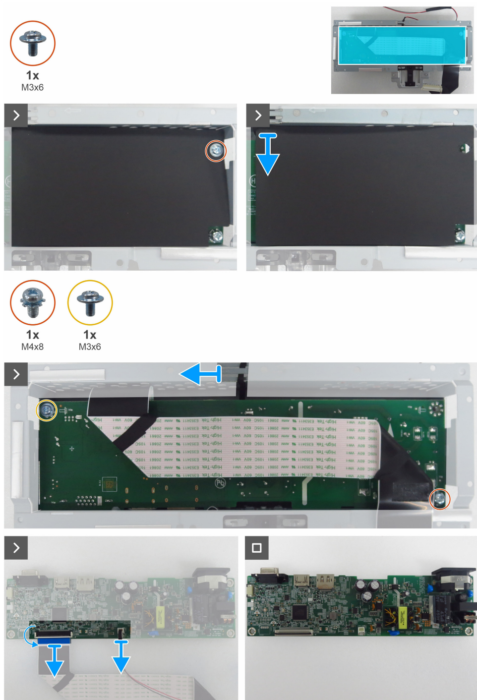
Obrázek 13. Odstranění hlavní desky
