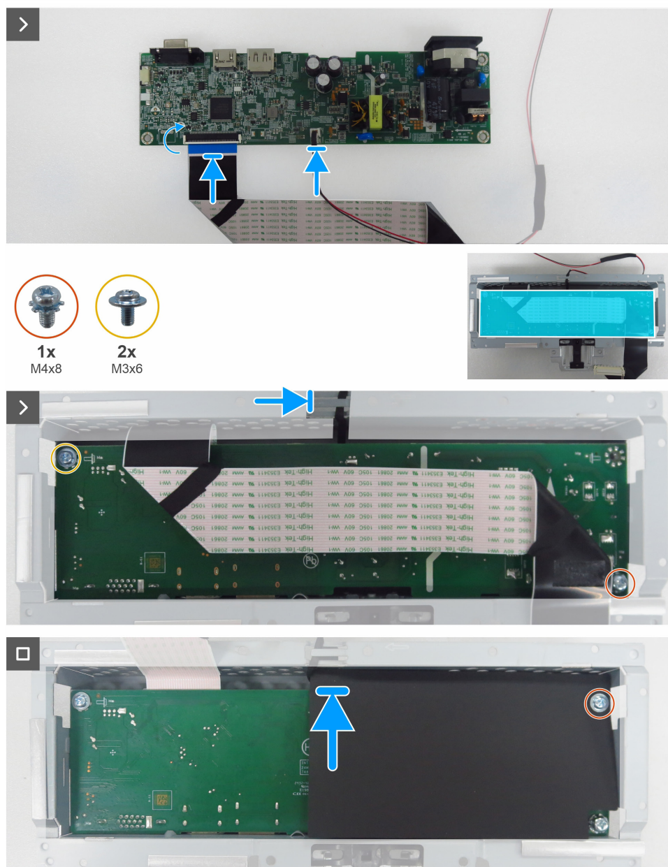
Obrázek 14. Instalace hlavní desky
