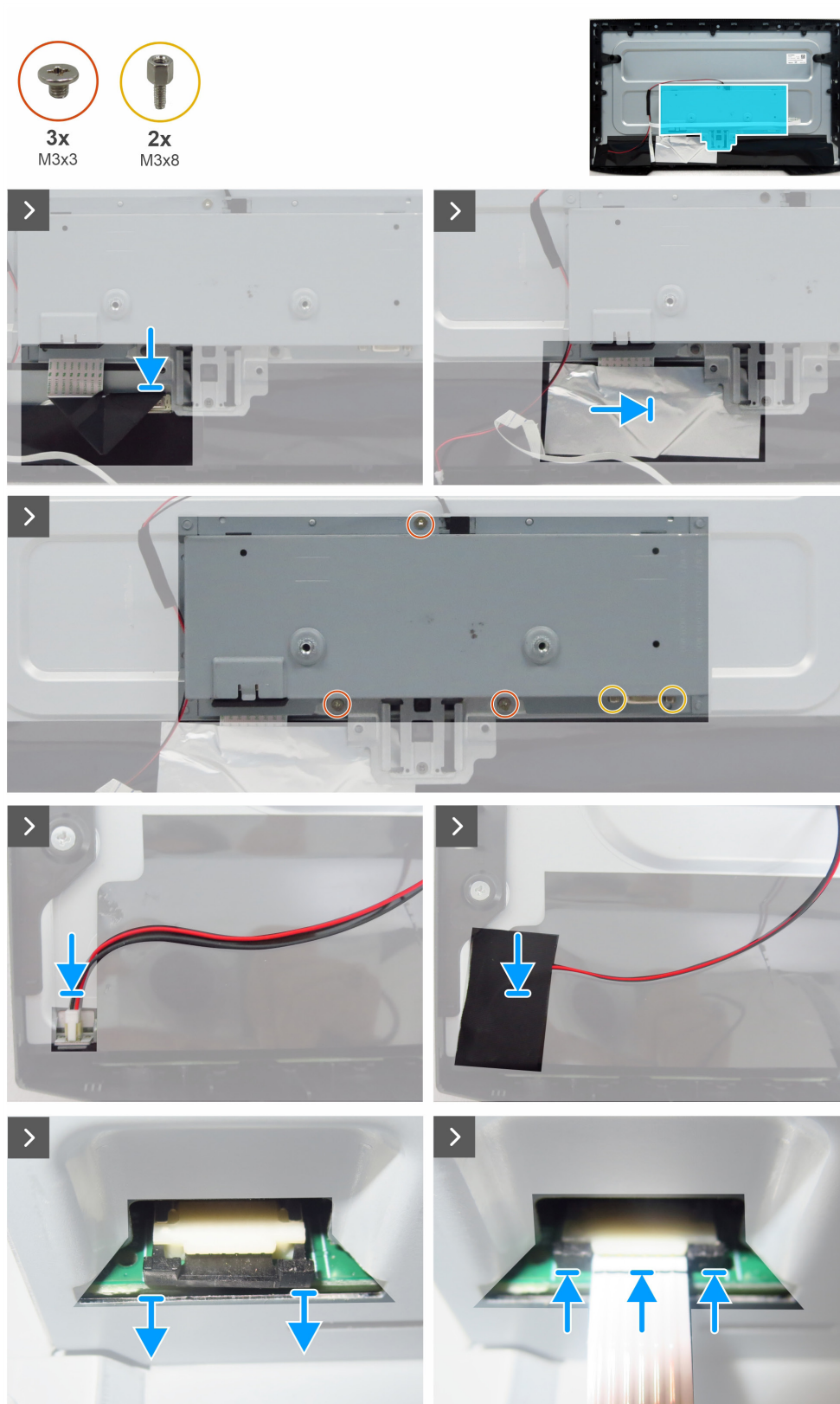
Obrázek 7. Instalace hlavního šasi
