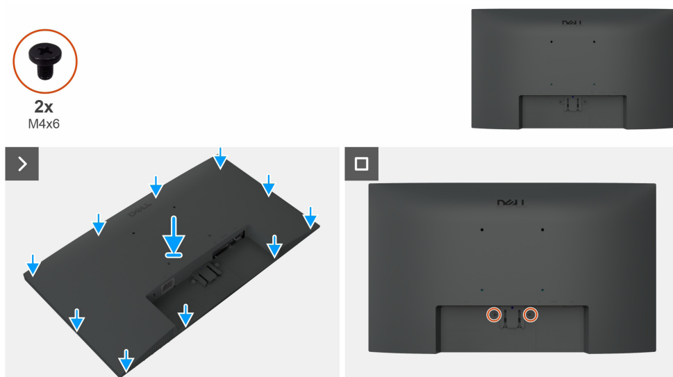
Obrázek 4. Instalace zadního krytu
