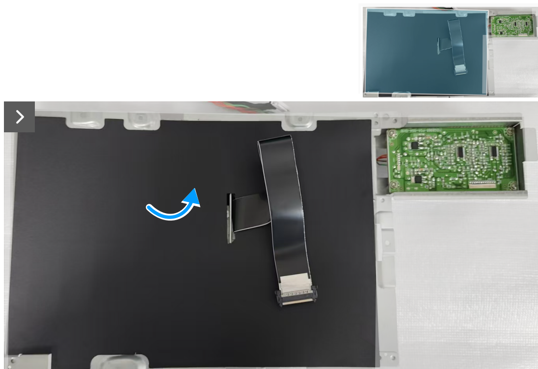
Rysunek 15. Zdejmowanie mylara
