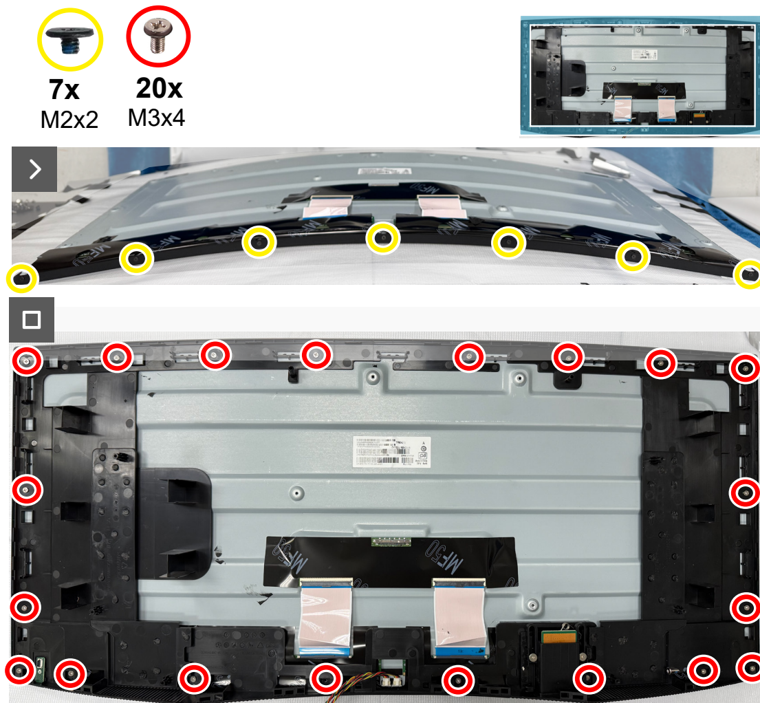
Rysunek 24. Przykręć ponownie śruby
