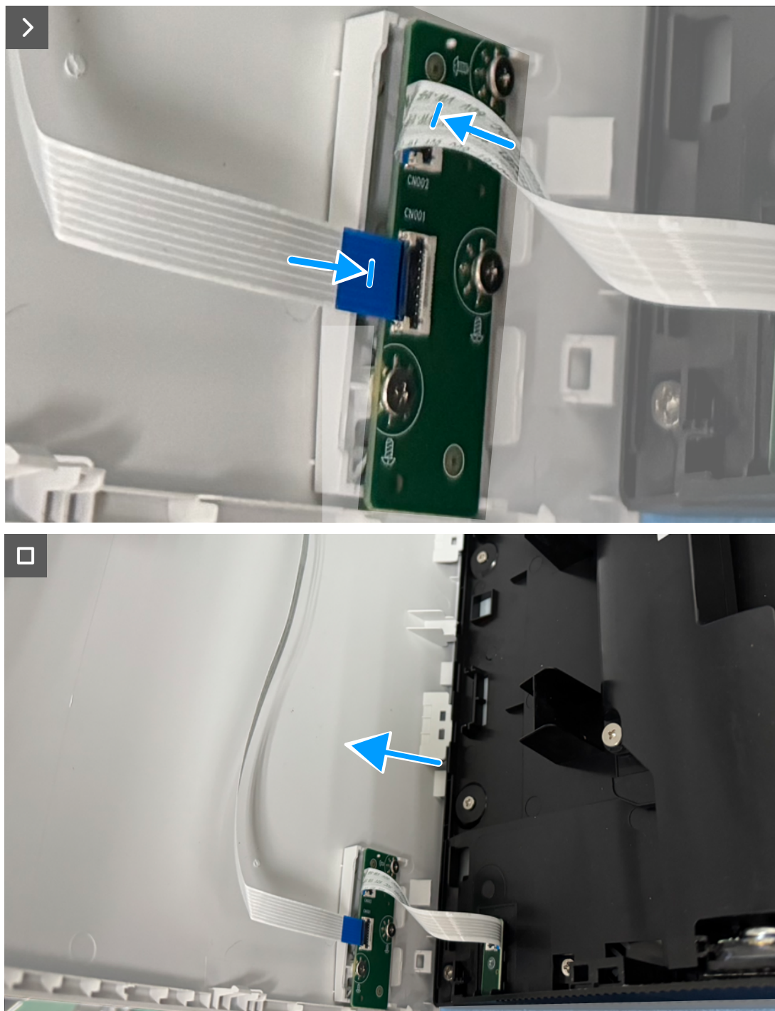
Rysunek 5. Podłącz kable płyty klawiatury i płyty obiektywu
