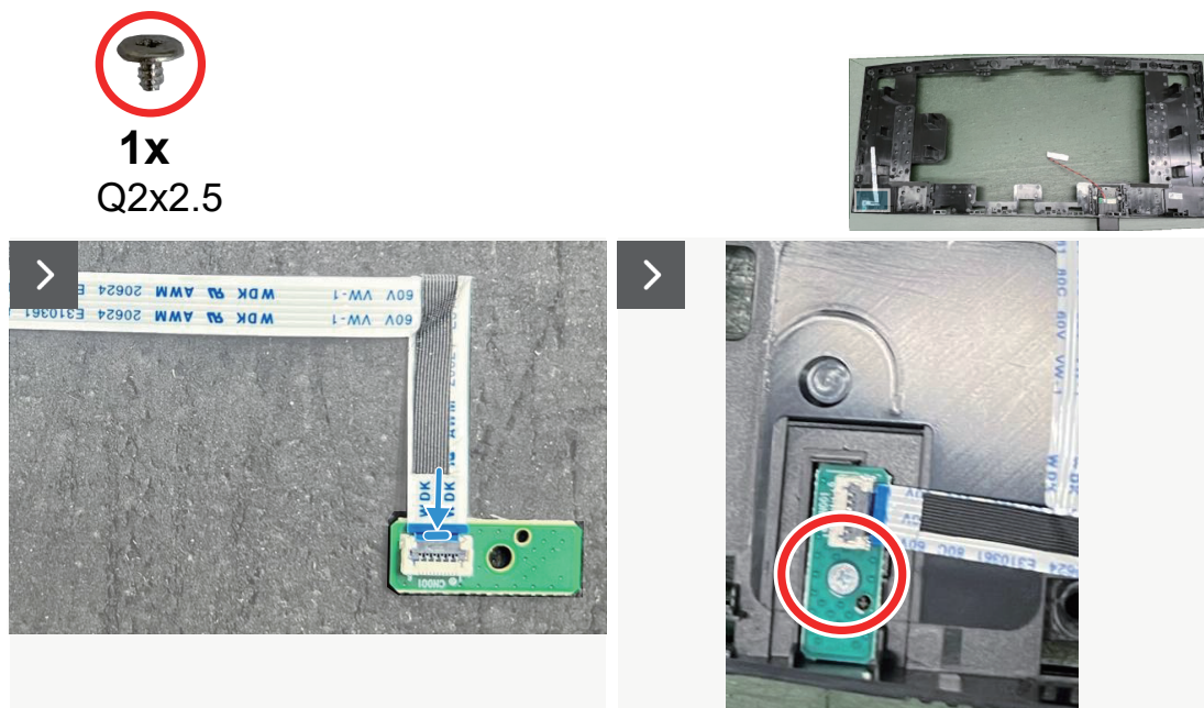
Rysunek 26. Instalacja płyty obiektywu
