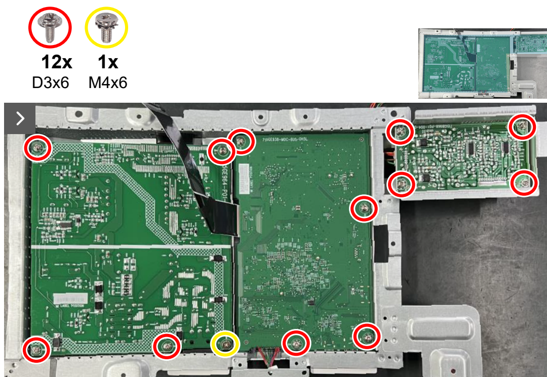
Rysunek 20. Przykręć ponownie śruby
