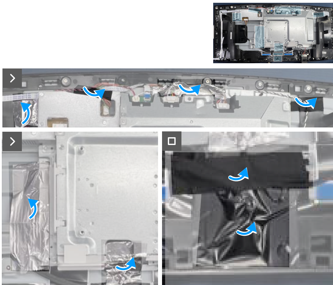
Rysunek 7. Przyklej taśmy, aby przymocować kable i metalową osłonę
