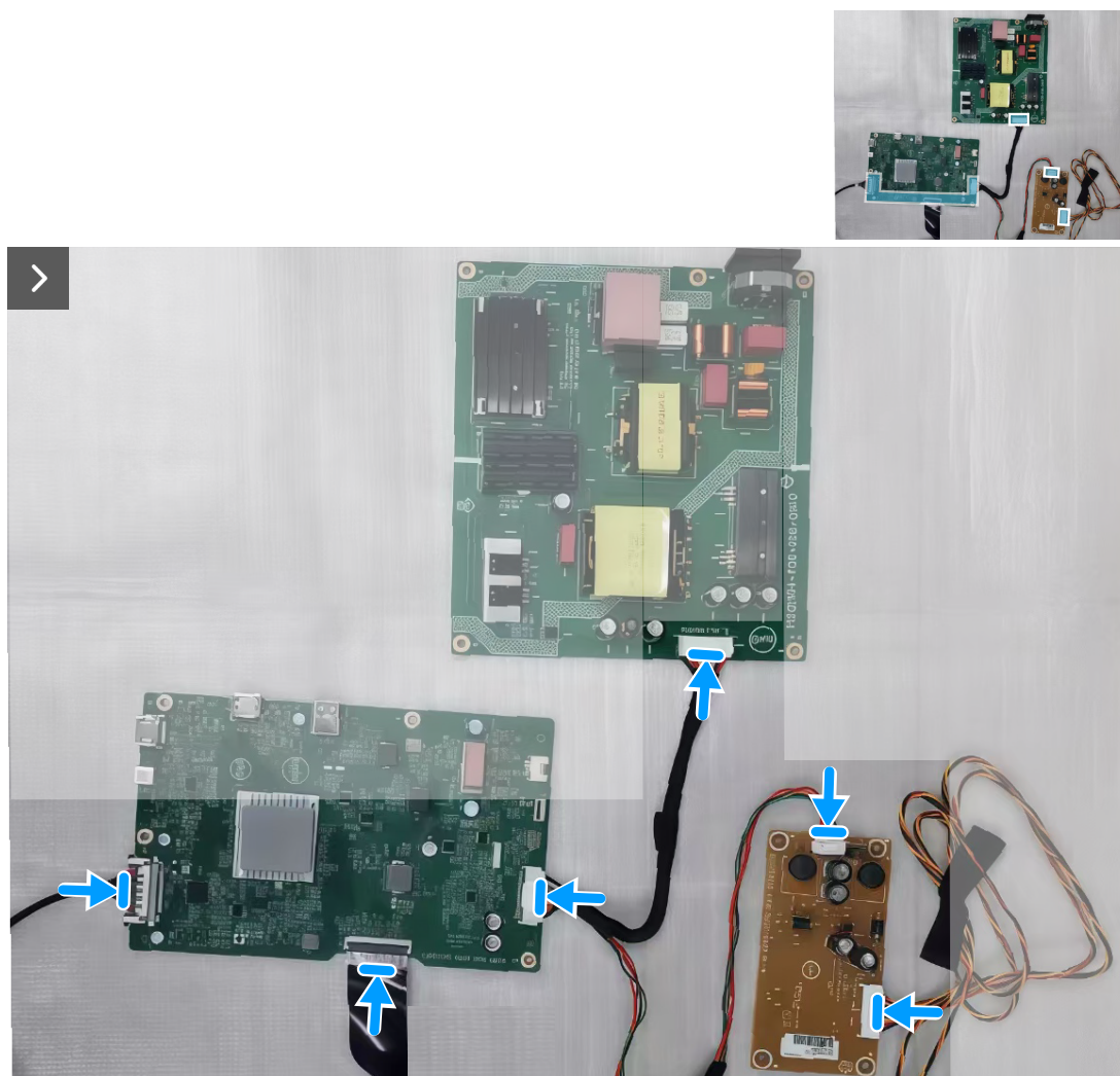
Rysunek 19. Podłączenie kabli
