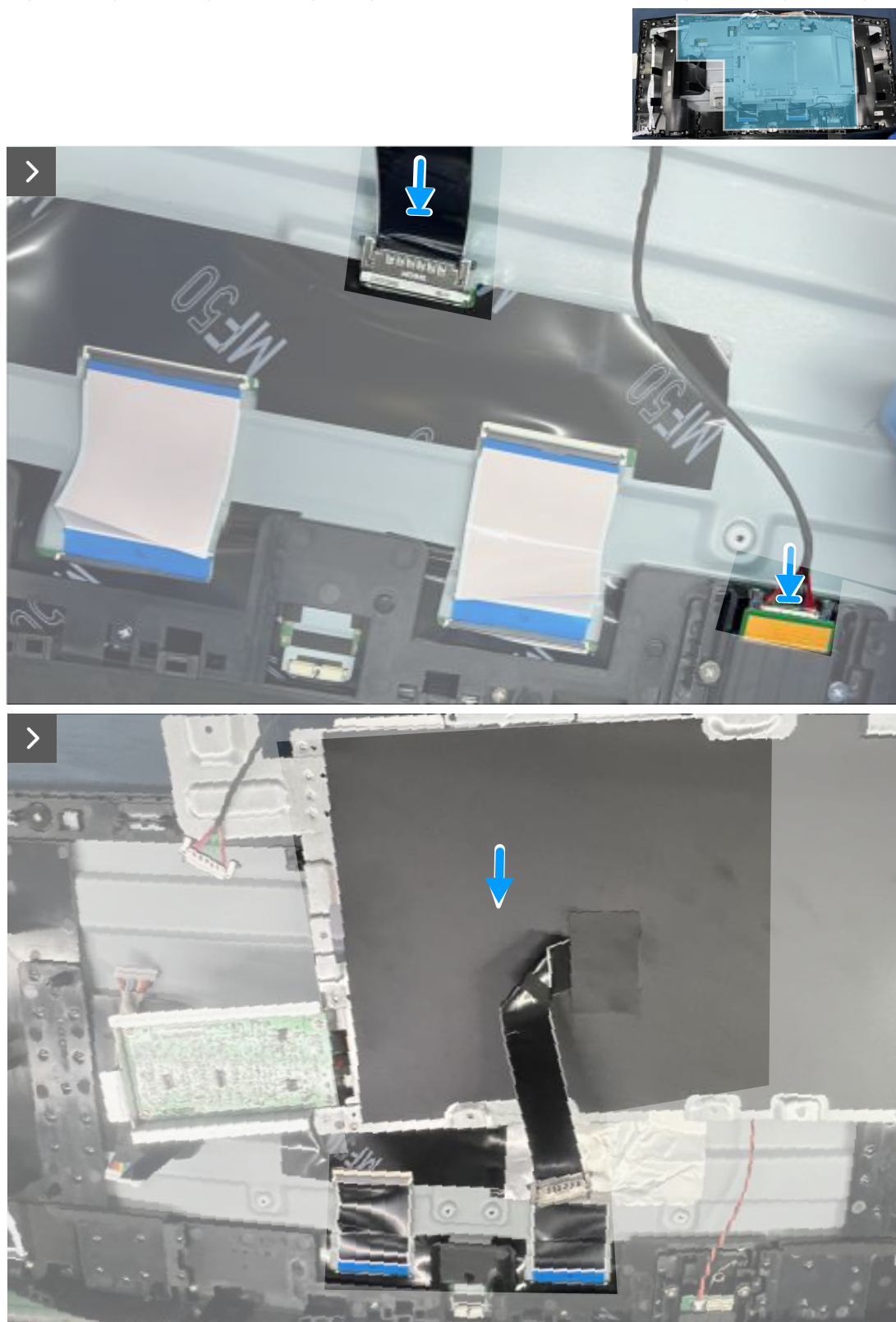
Rysunek 13. Podłączenie kabli wyświetlacza
