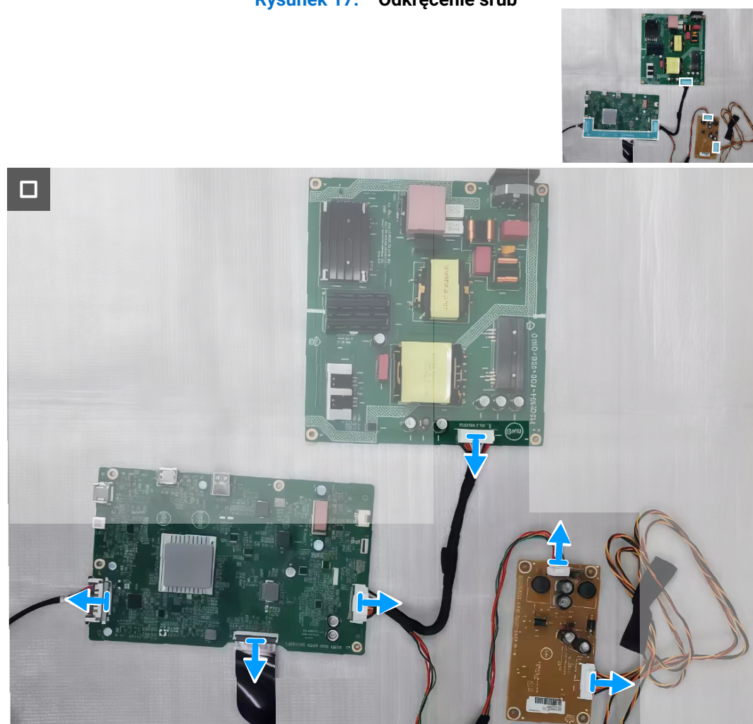
Rysunek 18. Odłączenie kabli
