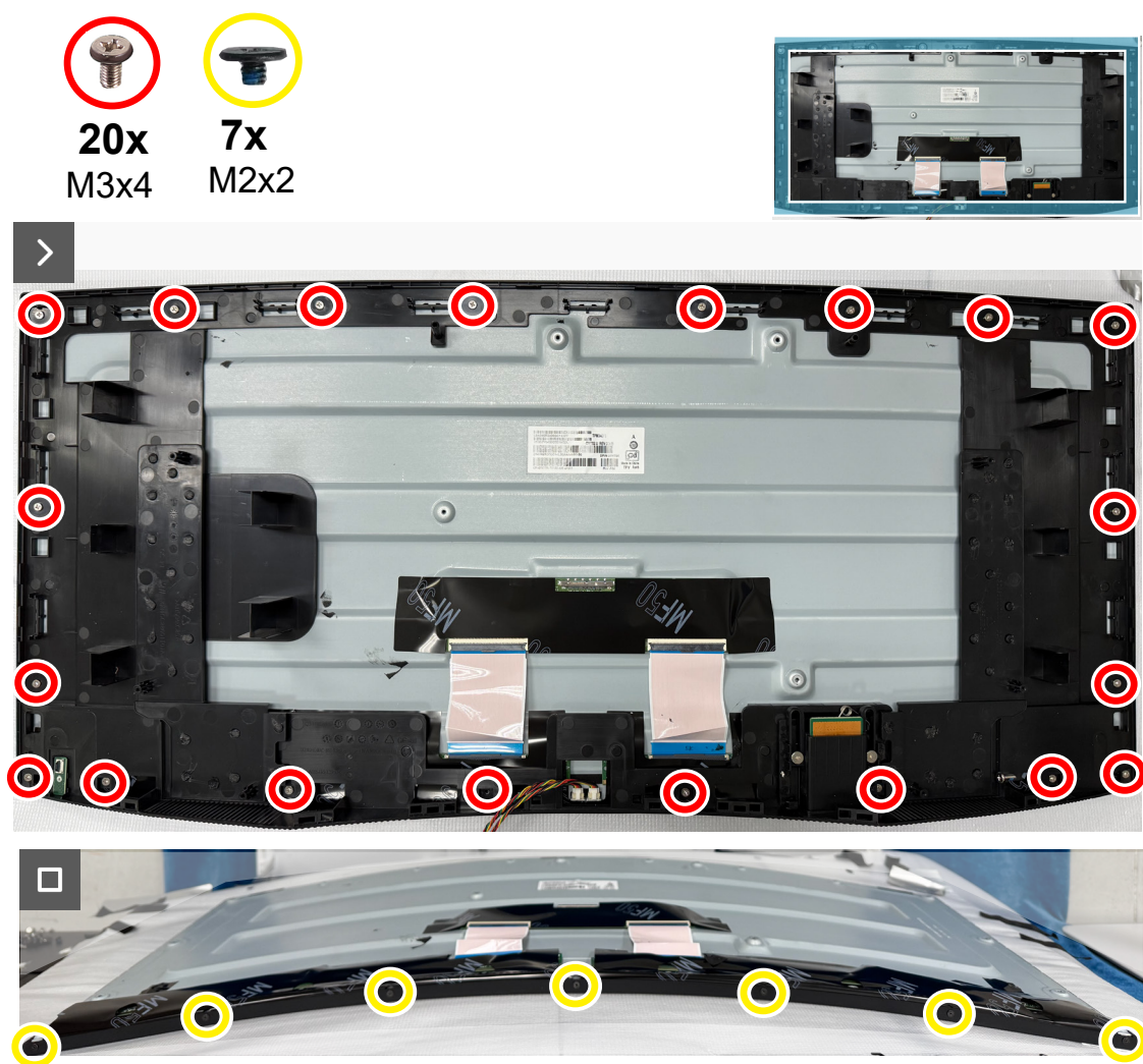
Rysunek 23. Odkręcenie śrub
