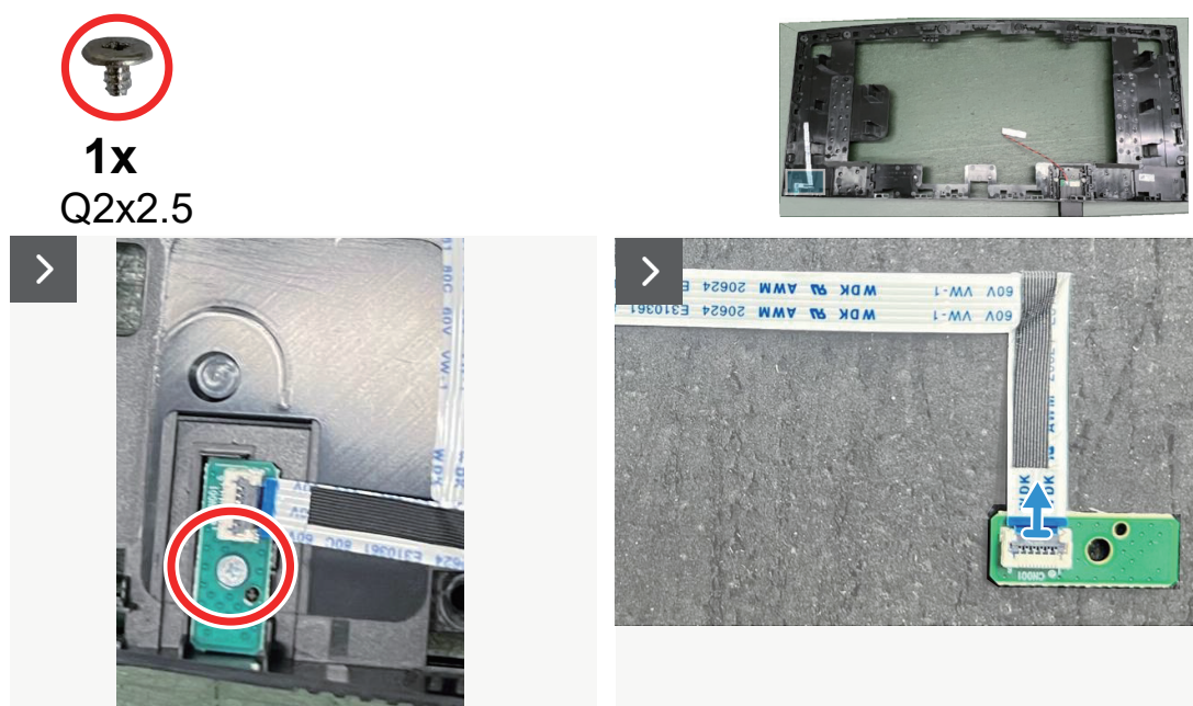
Rysunek 25. Zdejmowanie płyty obiektywu
