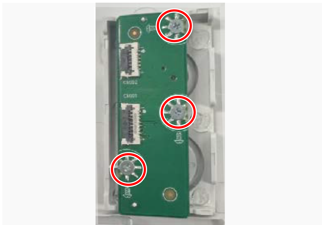
Rysunek 29. Zdejmowanie płyty klawiatury
