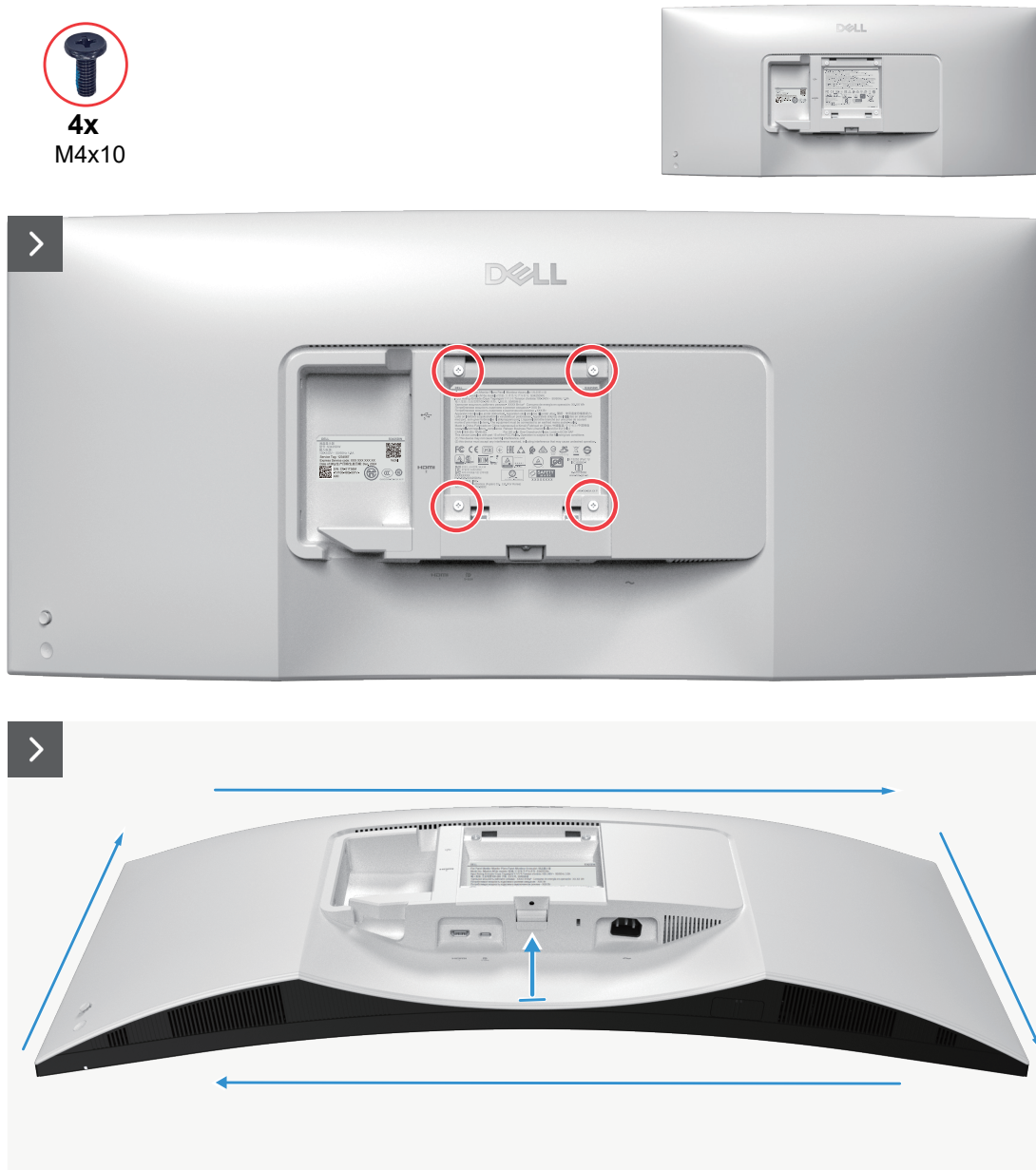
Rysunek 3. Odkręcanie śrub i podważanie pokrywy tylnej
