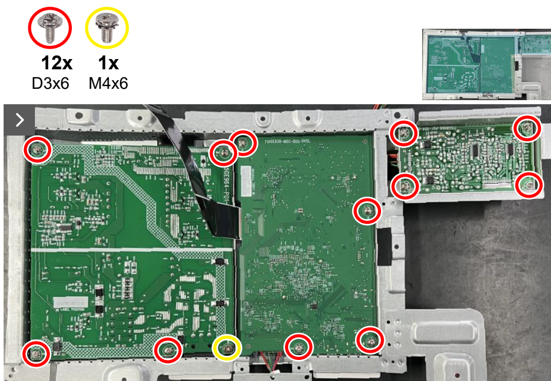
Rysunek 17. Odkręcenie śrub
