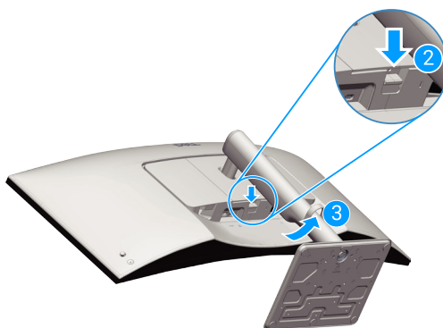
Abbildung 25. Monitorständer abnehmen
