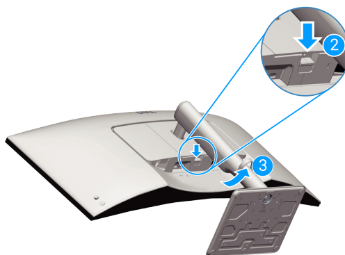
Figure 25. Retrait du support du moniteur
