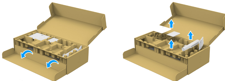
Figure 11. Enlevez la colonne de support et le socle
