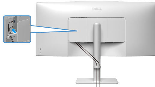
Figure 22. Fixation du couvercle des E/S latérales
