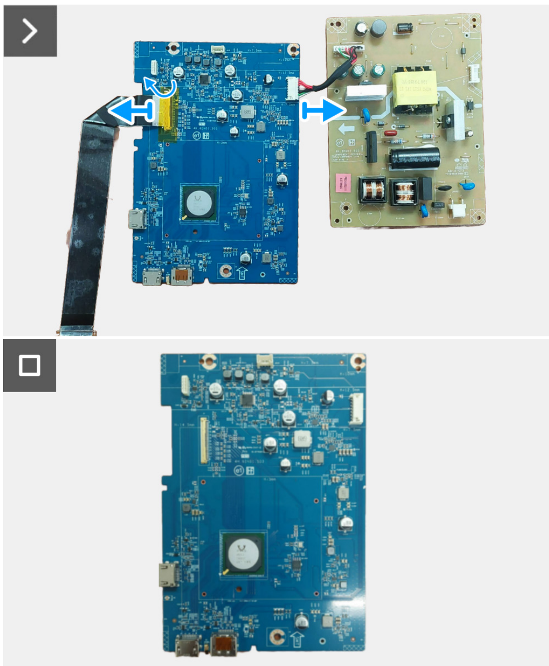
Obrázek 12. Demontáž desky rozhraní
