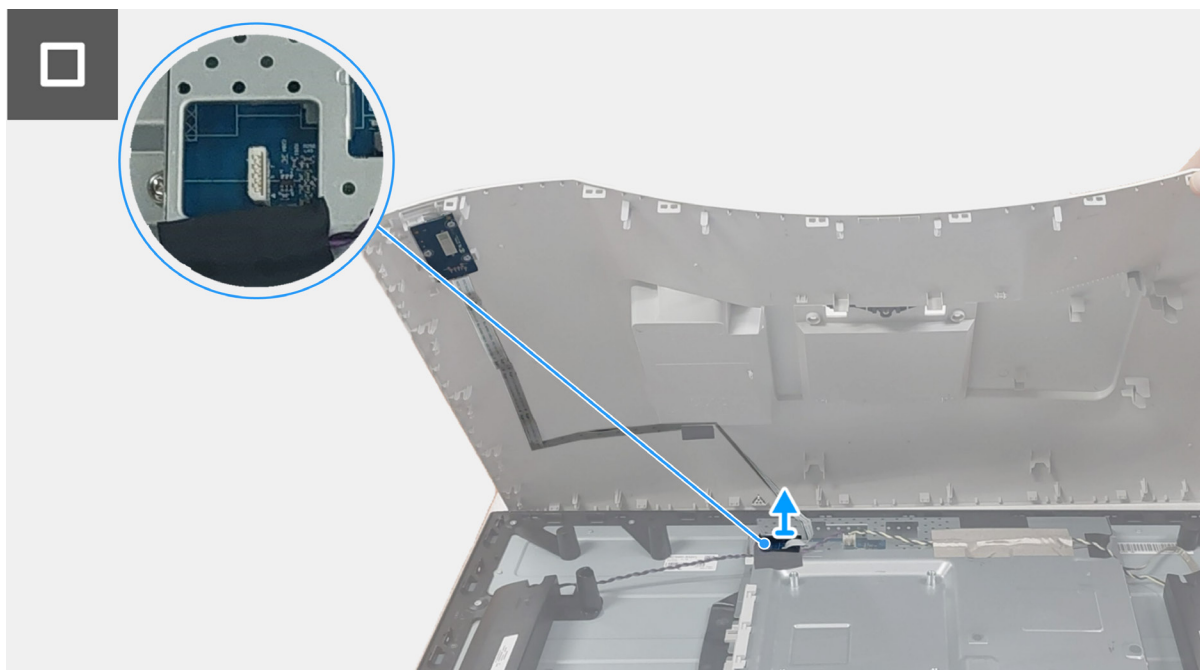
Obrázek 4. Sejmутí zadního krytu
