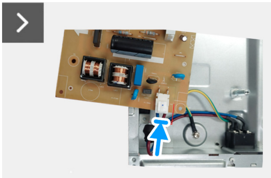
Obrázek 16. Instalace napájecí desky
