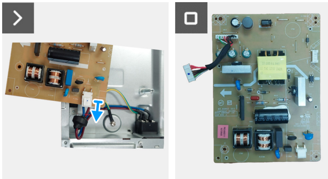
Obrázek 15. Demontáž napájecí desky
