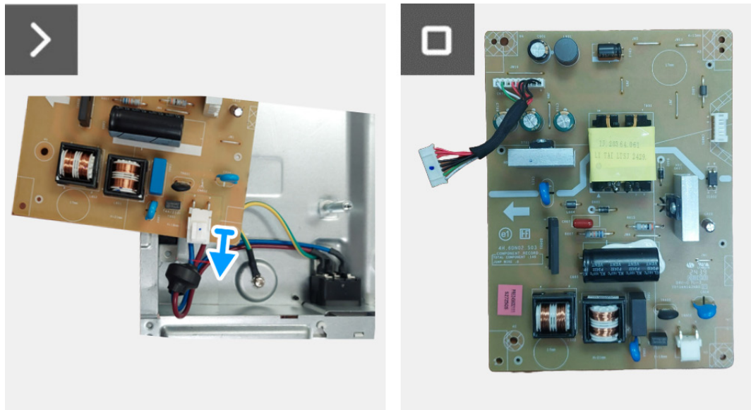
Figure 23. Retirer la carte d'alimentation
