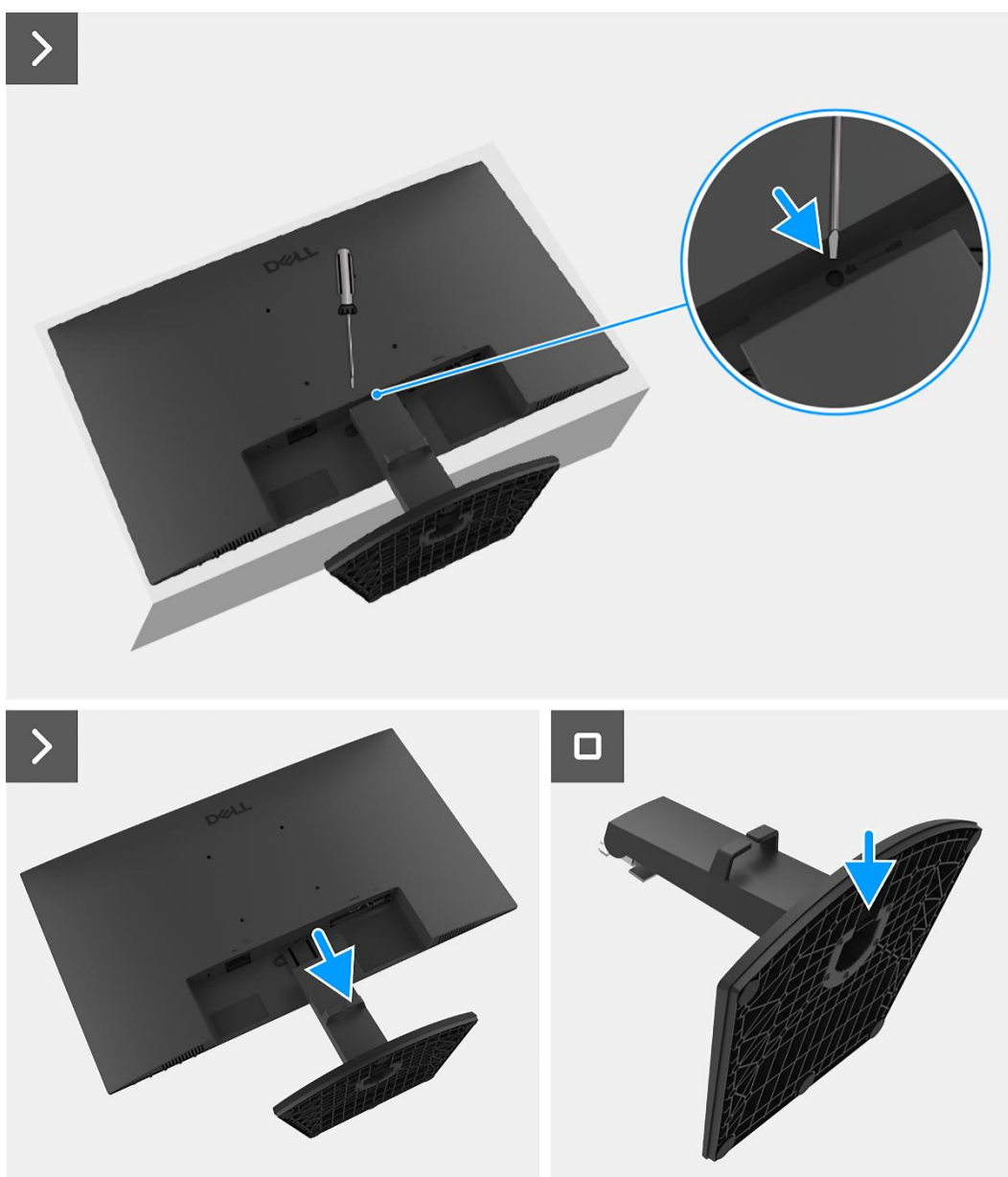
Obrázek 1. Odmontování stojanu
