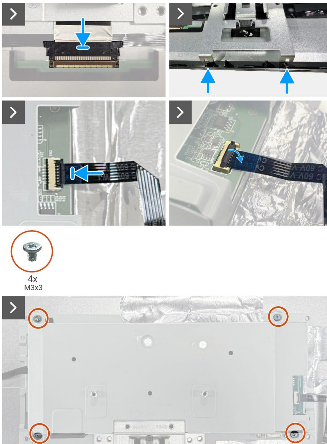
Obrázek 8. Instalace sestavy šasi
