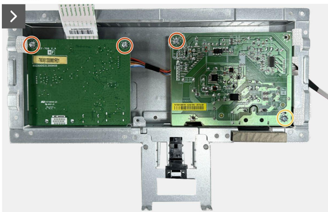
Obrázek 13. Odmontování desky rozhraní
