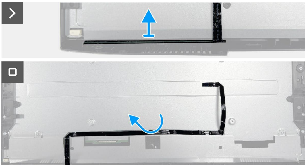
Obrázek 10. Odmontování desky klávesnice
