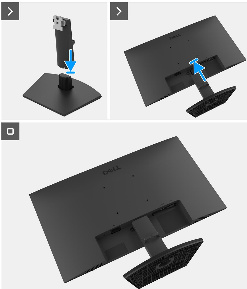
Obrázek 2. Instalace stojanu
