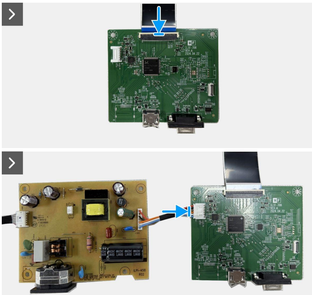
Obrázek 15. Instalace desky rozhraní
