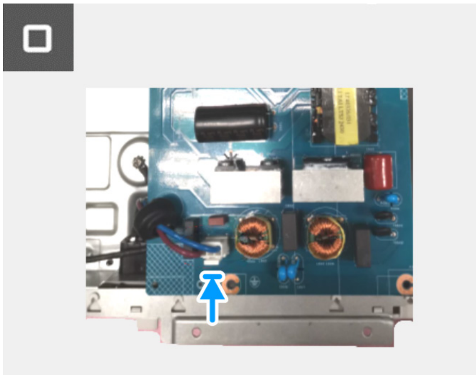
Obrázek 16. Instalace napájecí desky
