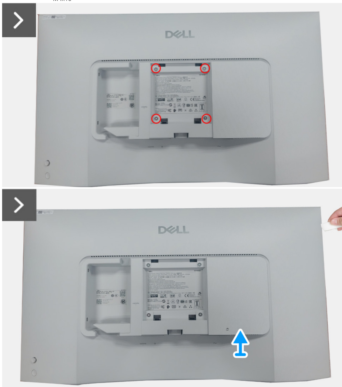
Obrázek 3. Sejmutí zadního krytu
