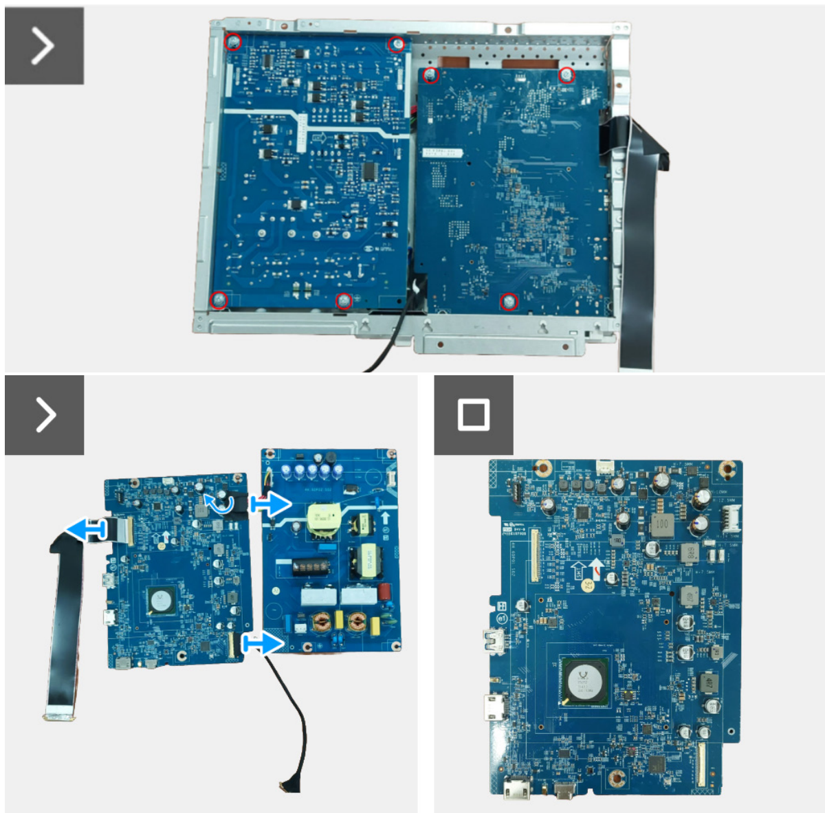
Obrázek 12. Demontáž desky rozhraní
