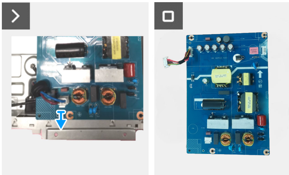
Obrázek 15. Demontáž napájecí desky
