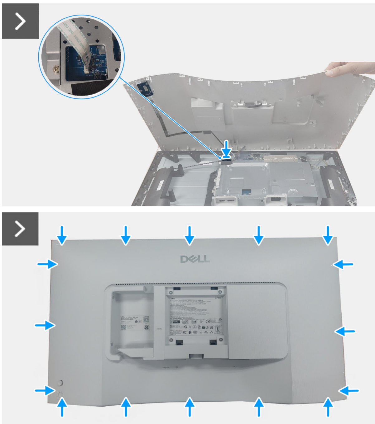
Obrázek 5. Instalace zadního krytu
