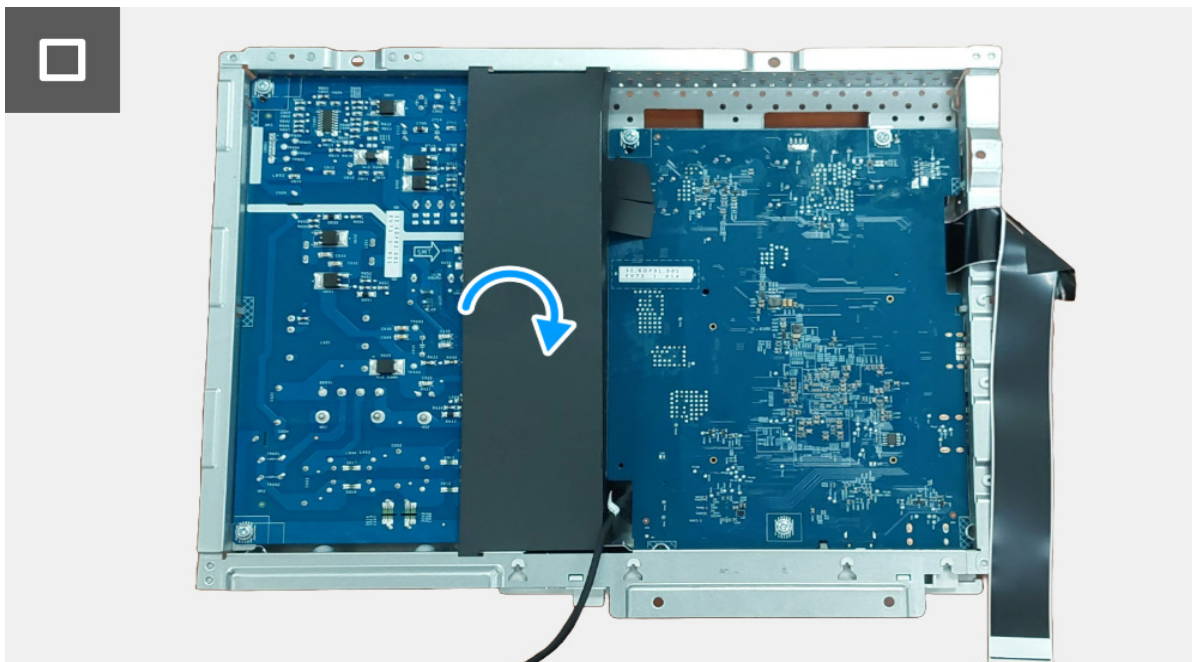
Obrázek 14. Instalace desky rozhraní
