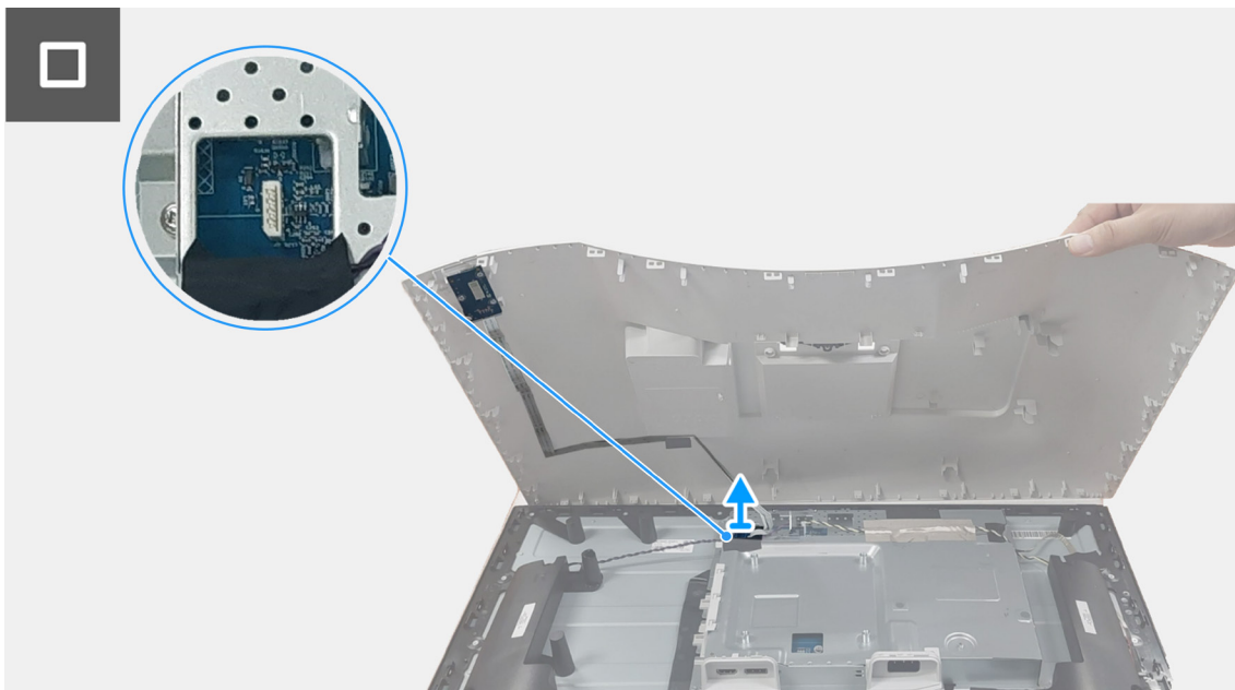
Obrázek 4. Sejmutí zadního krytu
