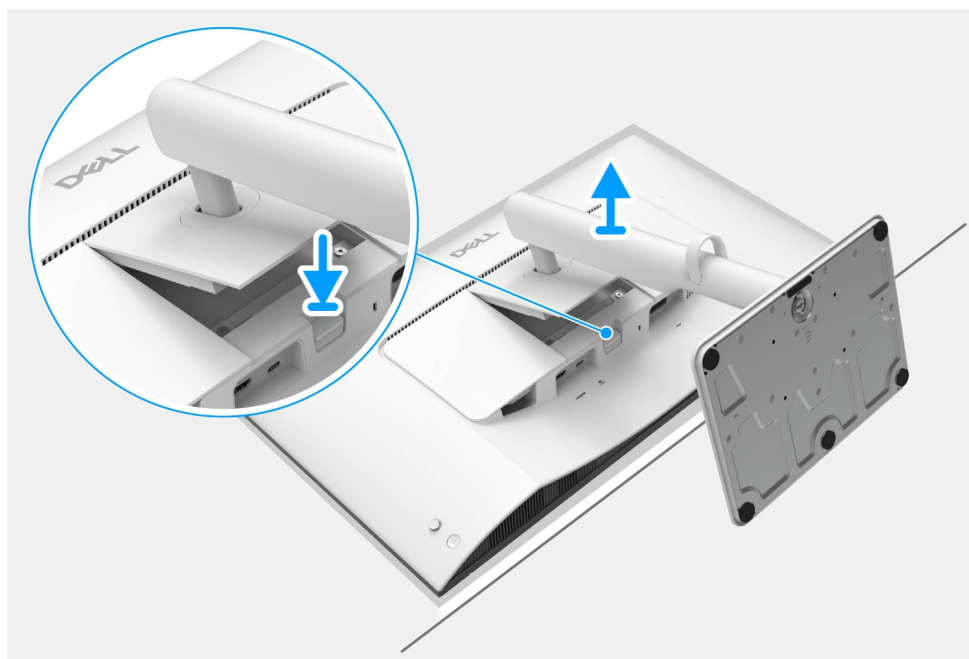
Obrázek 1. Demontáž podstavce
