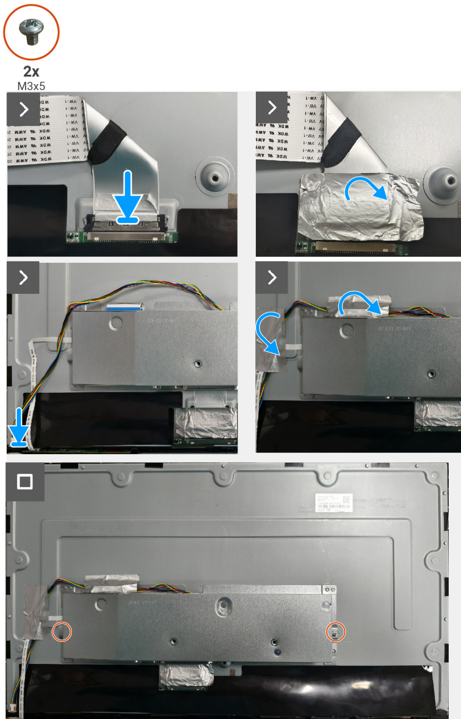
Obrázek 8. Instalace sestavy desky rozhraní
