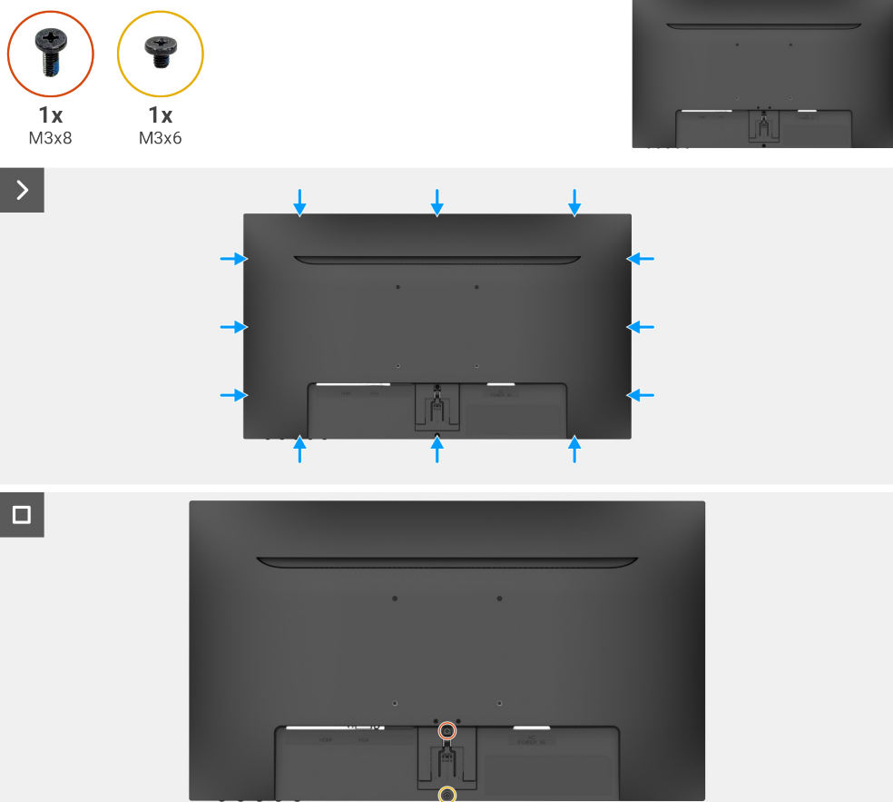
Obrázek 4. Instalace zadního krytu
