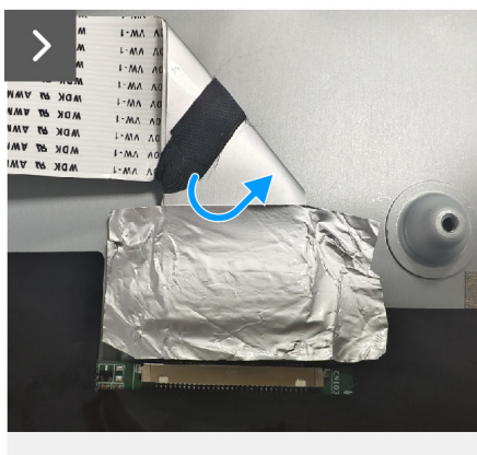
Obrázek 7. Demontáž sestavy desky rozhraní
