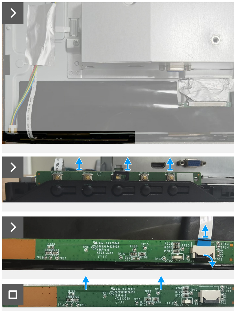
Obrázek 5. Odpojení desky klávesnice
