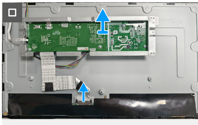
Obrázek 7. Demontáž sestavy desky rozhraní
