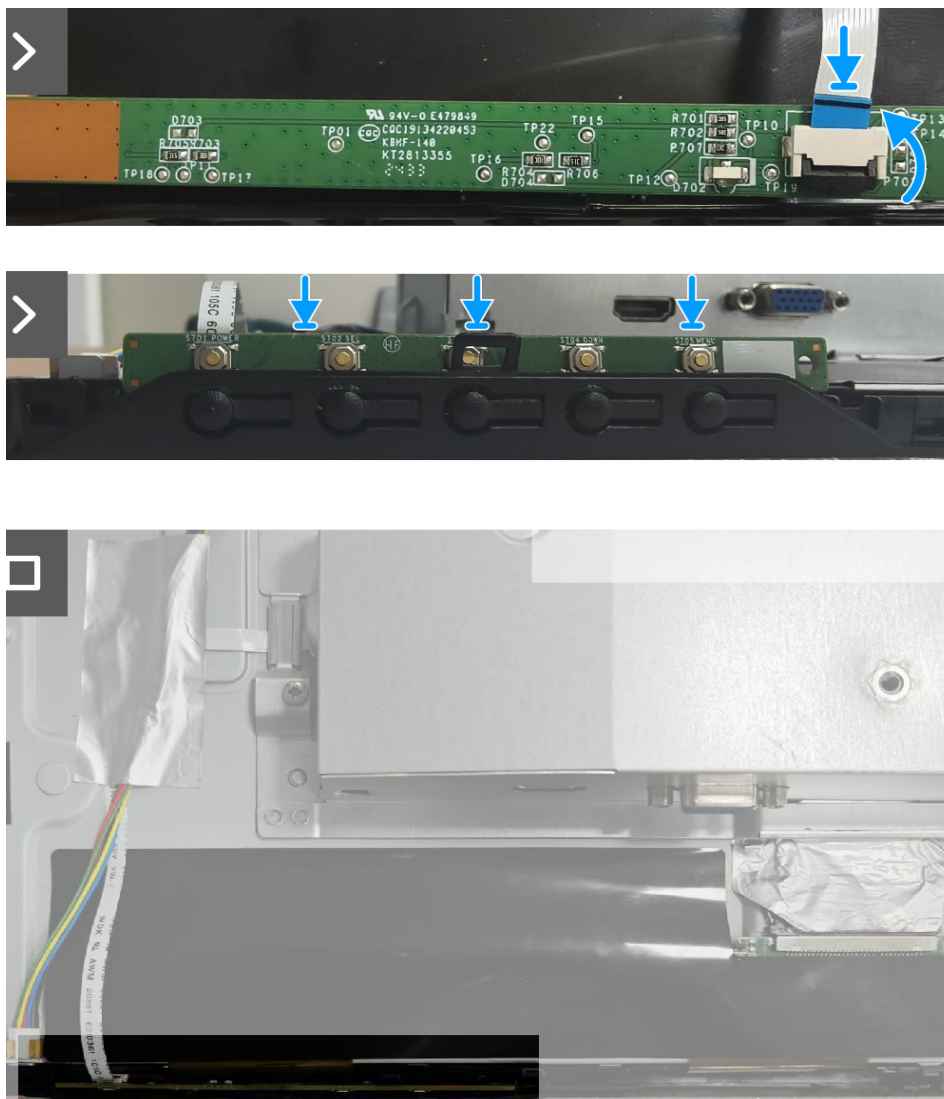
Obrázek 6. Instalace desky klávesnice
