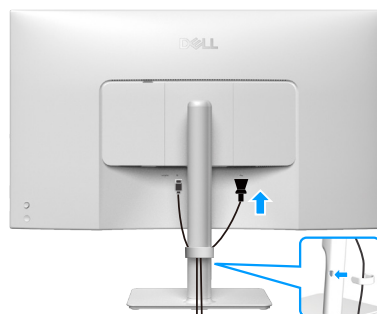
Figure 21. Gestion de vos câbles
