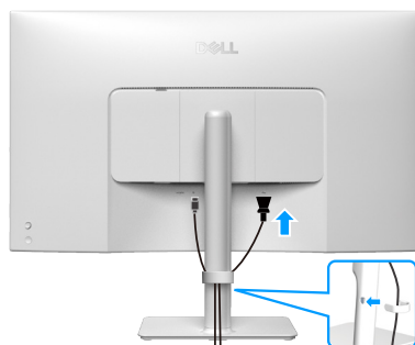
Figura 21. Organizar los cables
