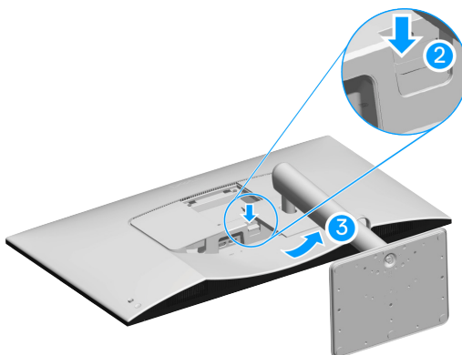
Figura 23. Desmontar el pedestal del monitor
