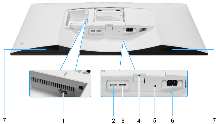
Figura 3. Vista inferior del monitor
