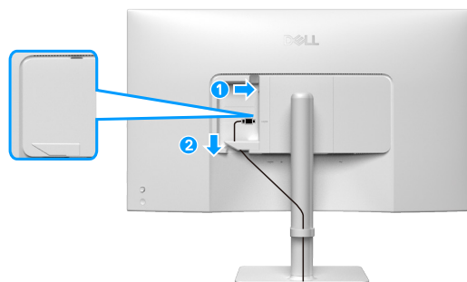
Figura 19. Enrutamiento del cable hacia el lado de E/S
