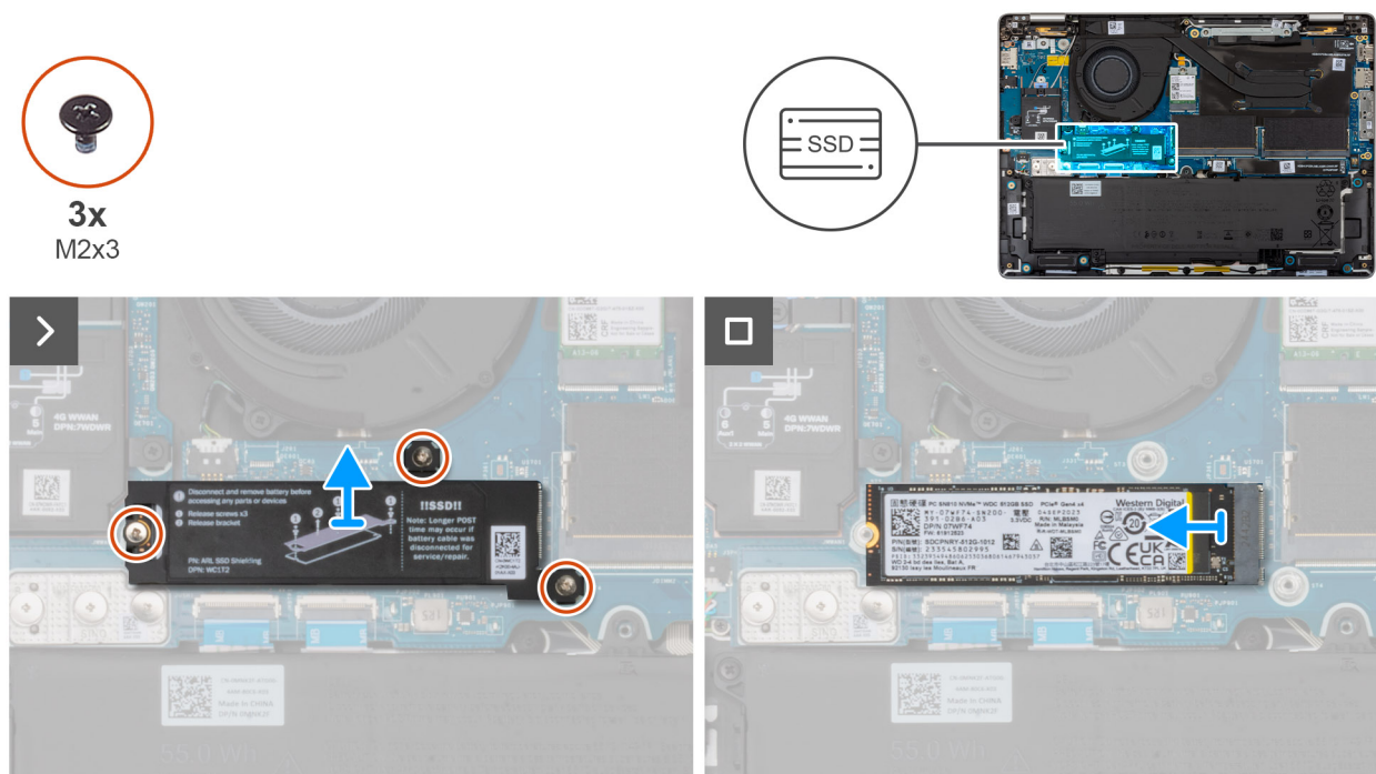
Figura 37. Rimozione dell'SSD M.2 2280
