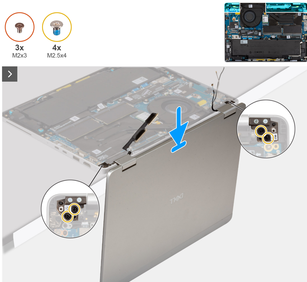
Figura 65. Installazione del gruppo del display
