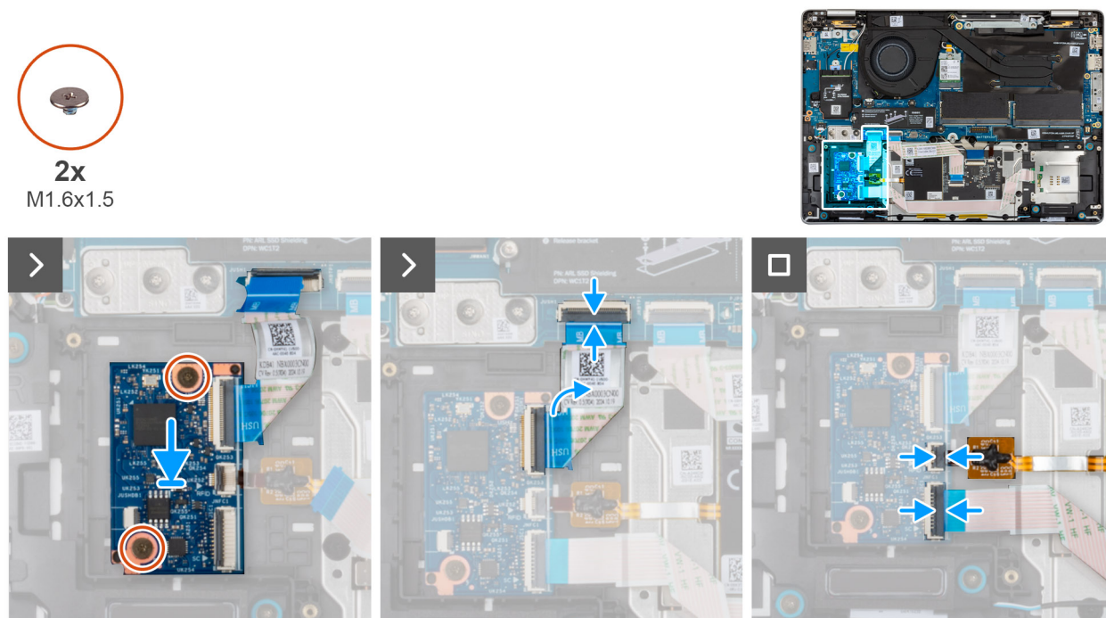
Figura 46. Installazione della scheda figlia USH
