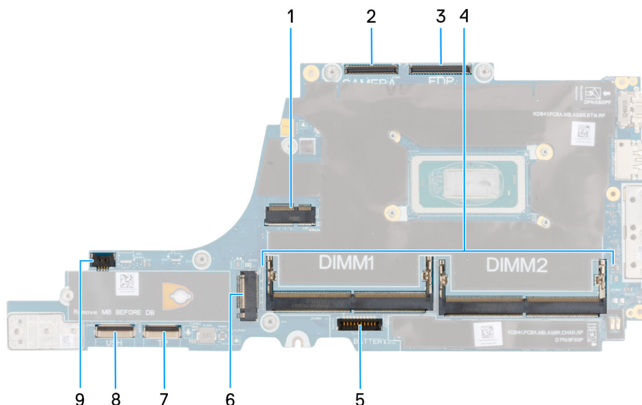
Figura 49. Connettori della scheda di sistema
