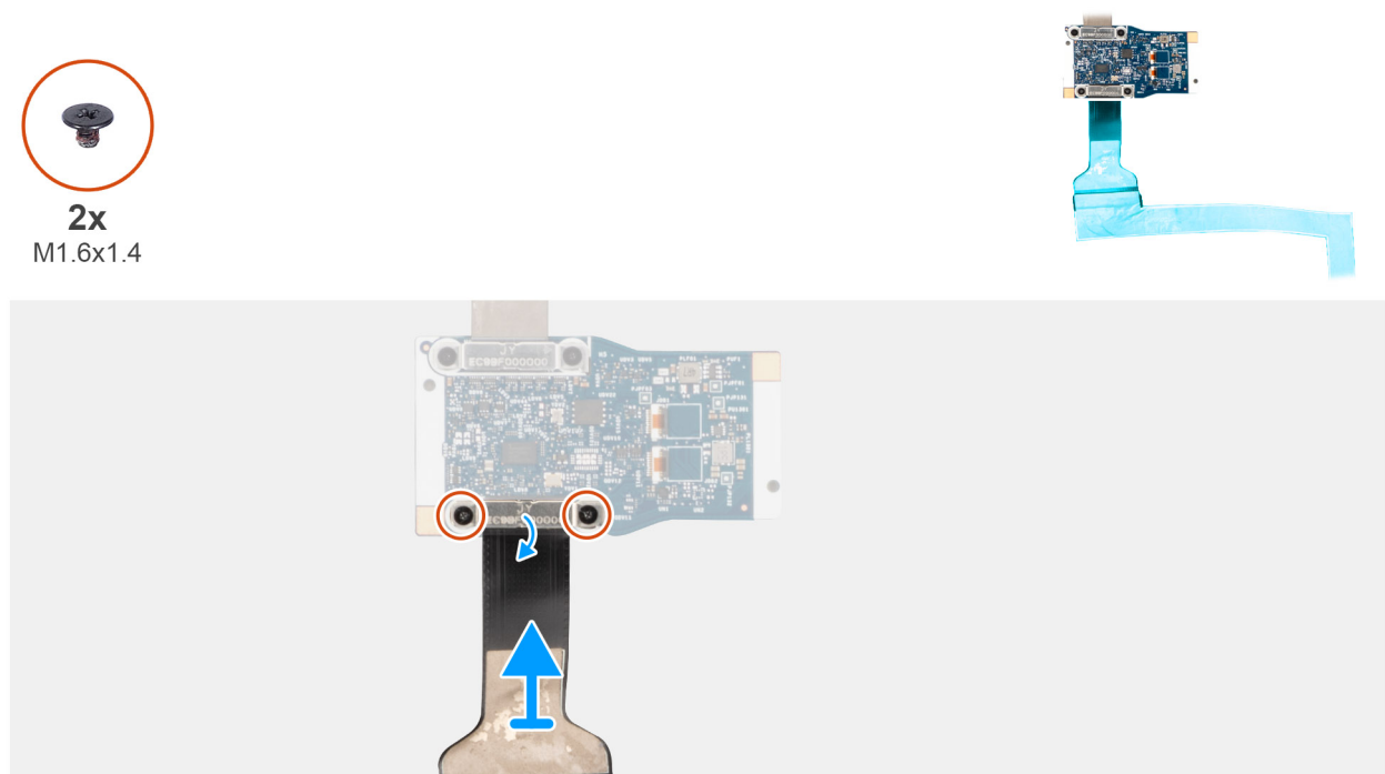
Figura 89. Rimozione del cavo del display per la fotocamera MIPI
