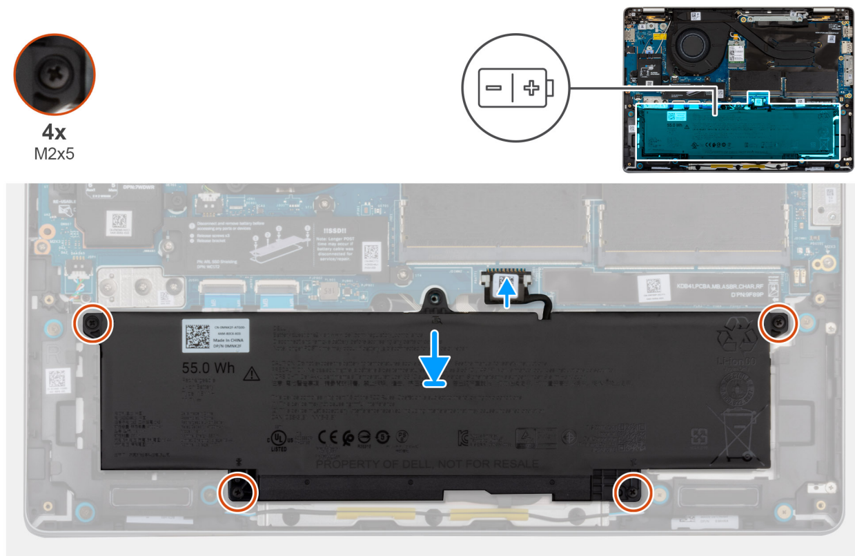
Figura 28. Installazione della batteria
