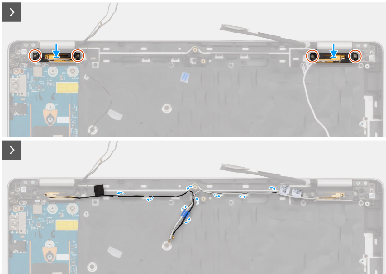
Figura 55. Installazione del modulo dell'antenna WLAN
