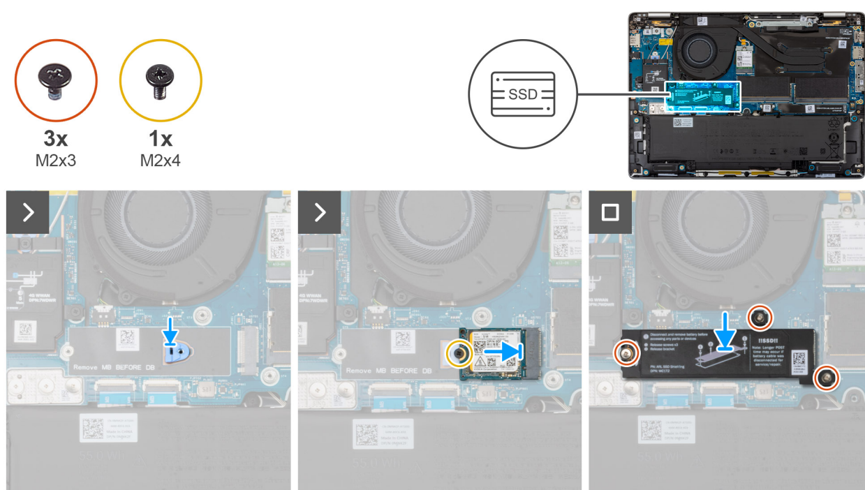
Figura 36. Installazione dell'SSD M.2 2230
