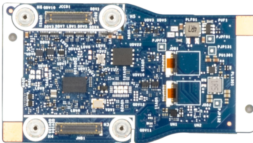
Figura 93. Scheda figlia centrale
