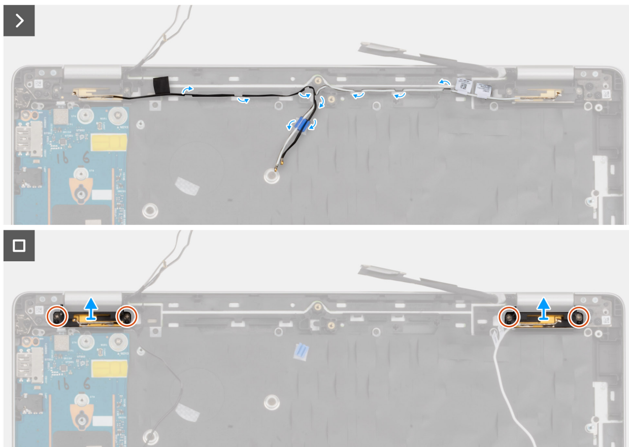
Figura 54. Rimozione del modulo dell'antenna WLAN
