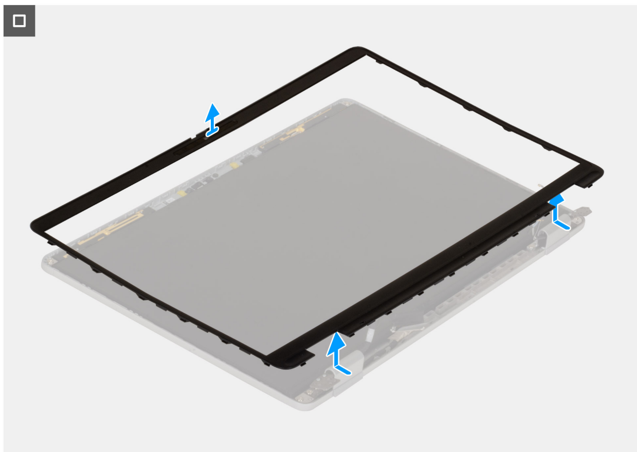
Figura 71. Rimozione della cornice del display
