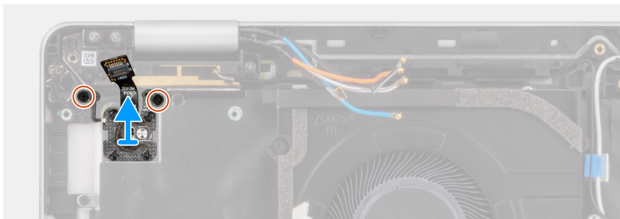
Figura 61. Rimozione del pulsante di accensione con lettore di impronte digitali opzionale
