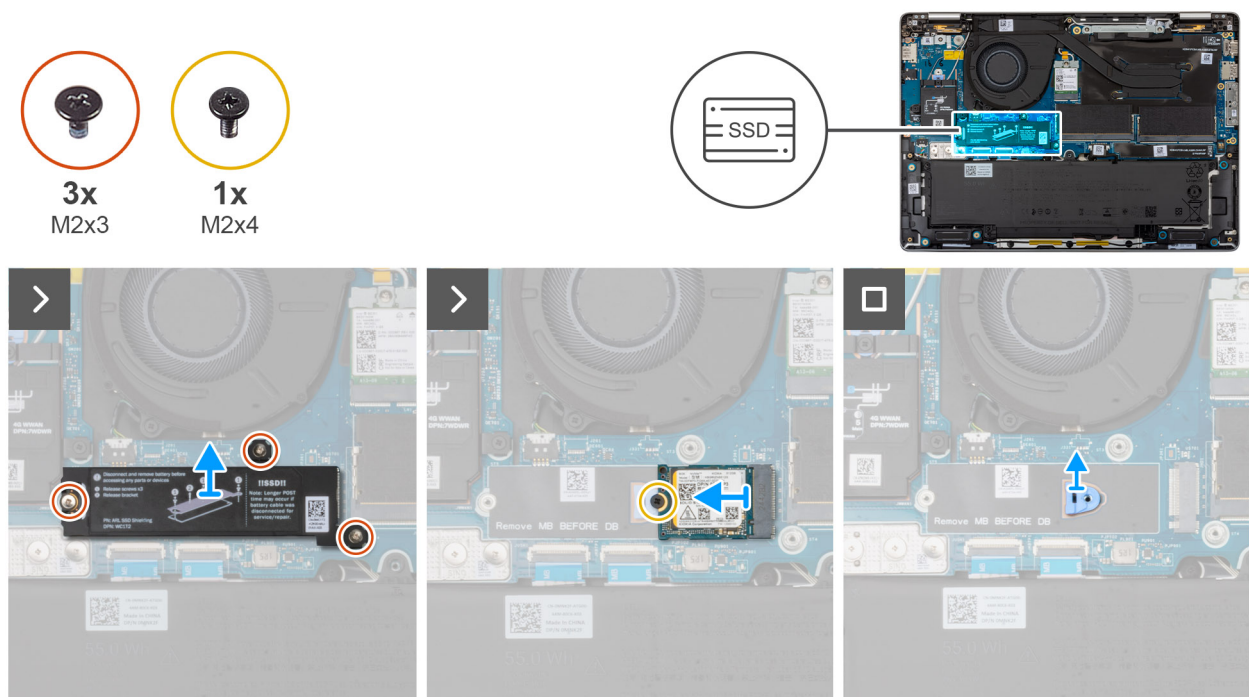
Figura 35. Rimozione dell'SSD M.2 2230
