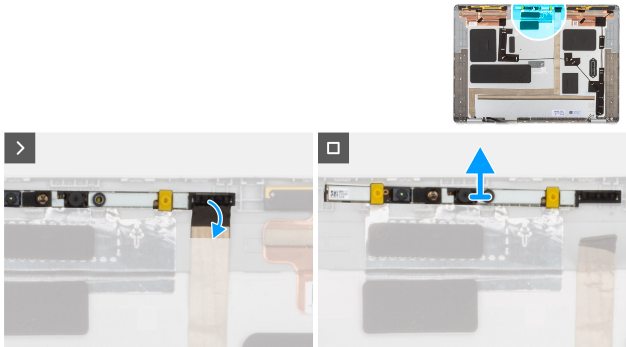
Figura 81. Rimozione della fotocamera RGB/IR
