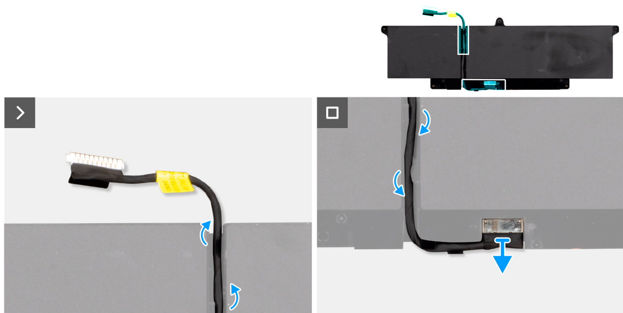
Figura 29. Rimozione del cavo della batteria
