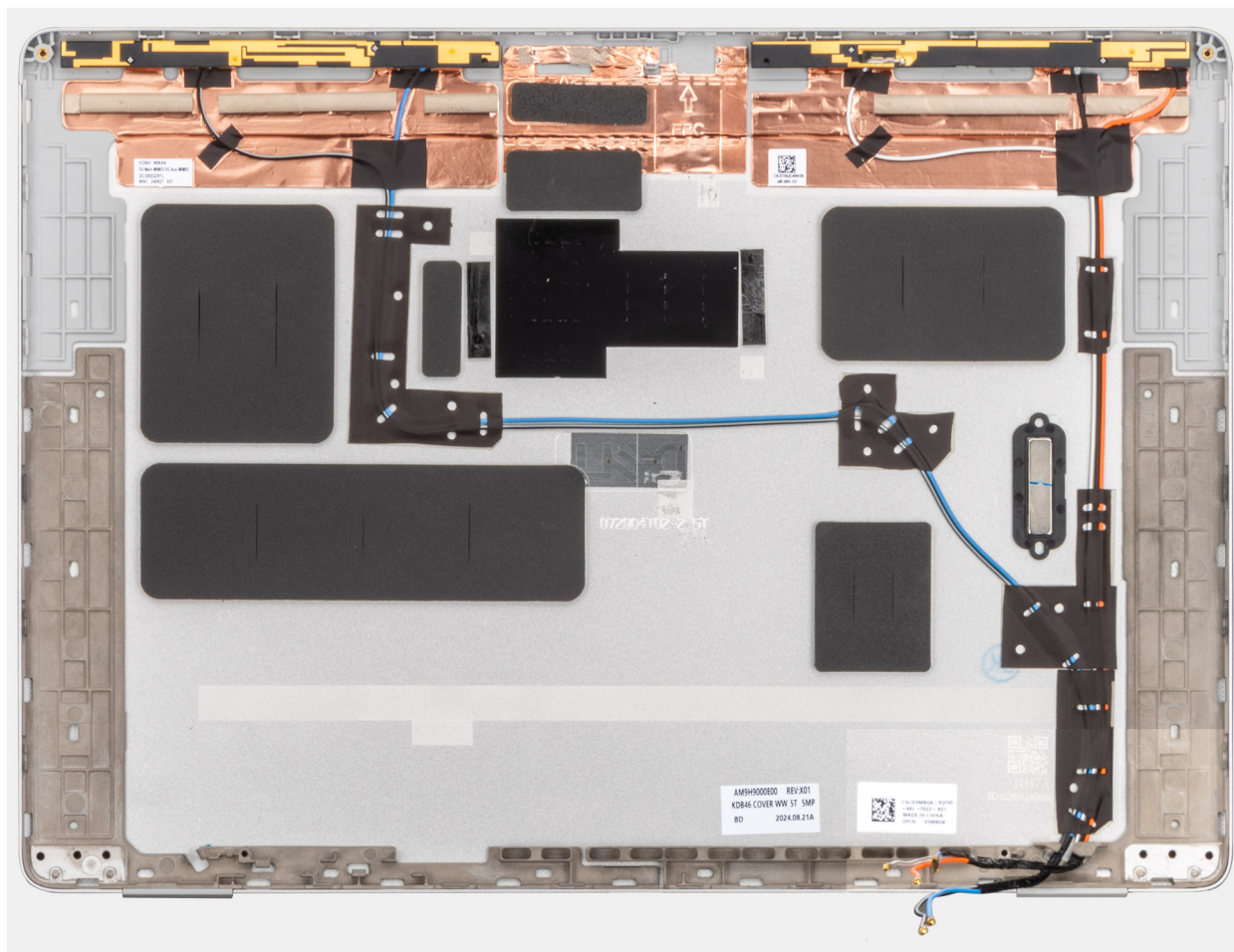
Figura 95. Gruppo del coperchio posteriore del display e antenna
