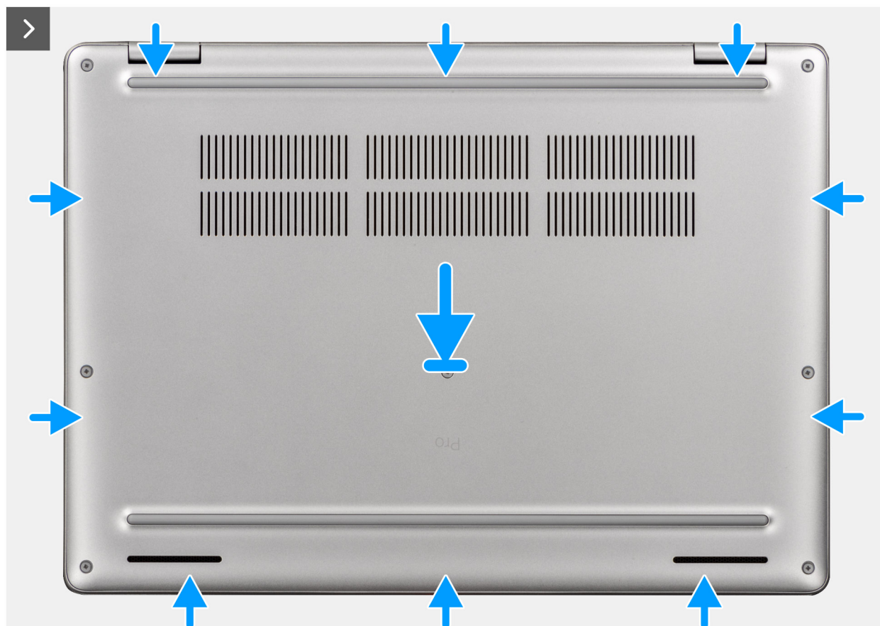
Figura 25. Installazione del coperchio della base
