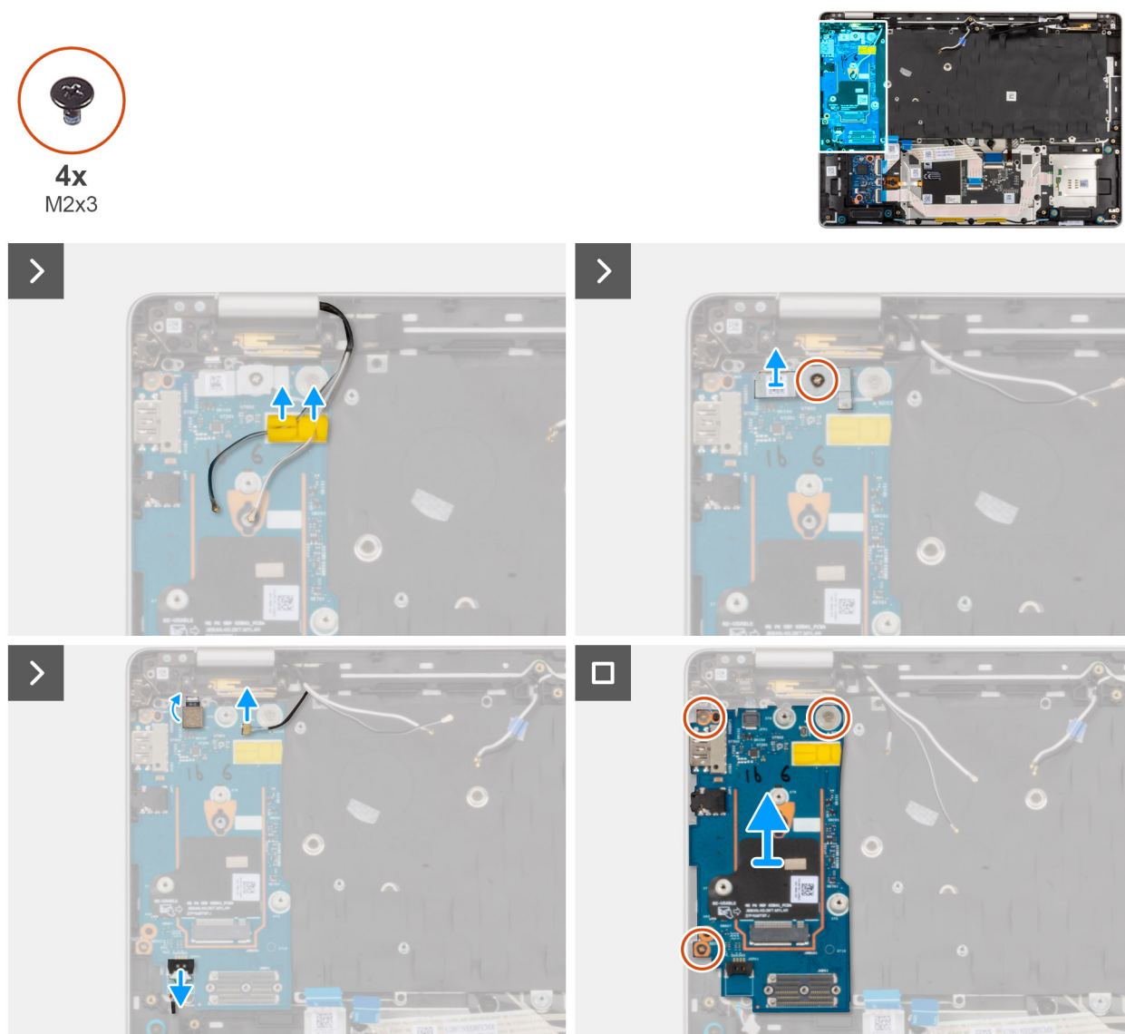
Figura 59. Rimozione della scheda di I/O
