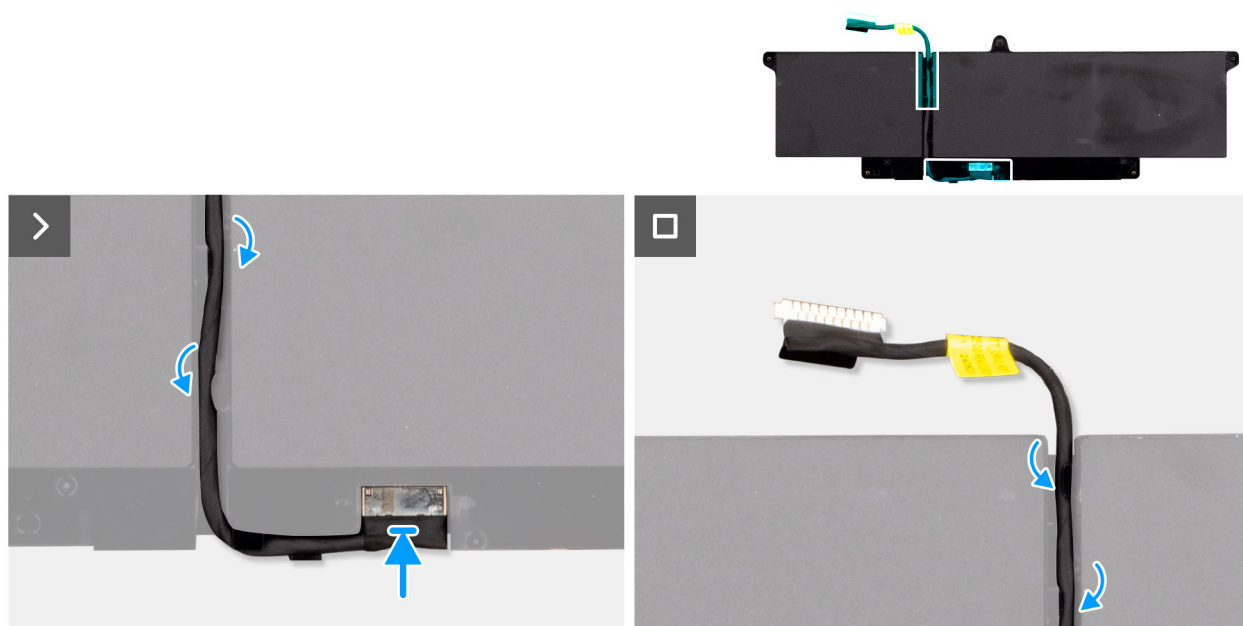
Figura 30. Installazione del cavo della batteria
