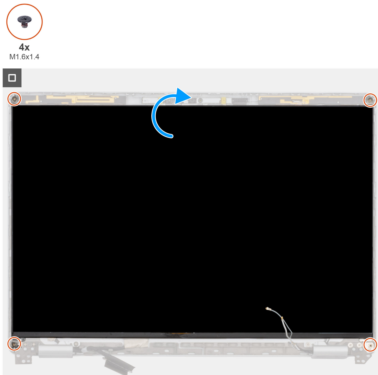
Figura 78. Installazione del pannello del display
