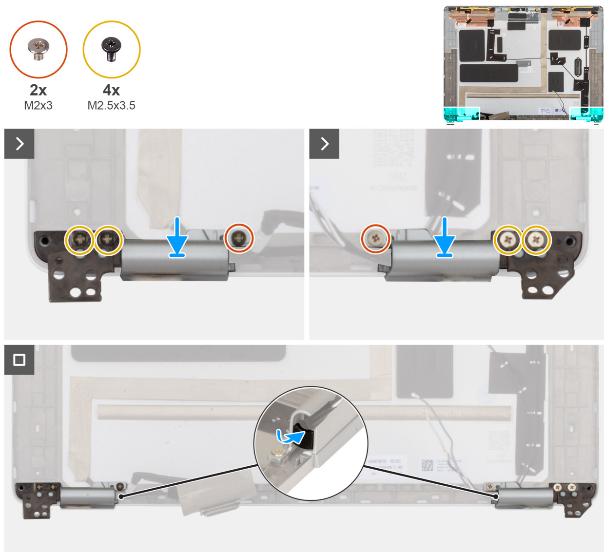
Figura 80. Installazione dei cappucci delle cerniere del display
