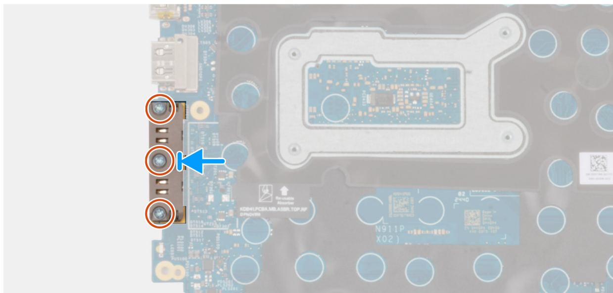
Figura 58. Installazione del modulo del connettore USB Type-C
