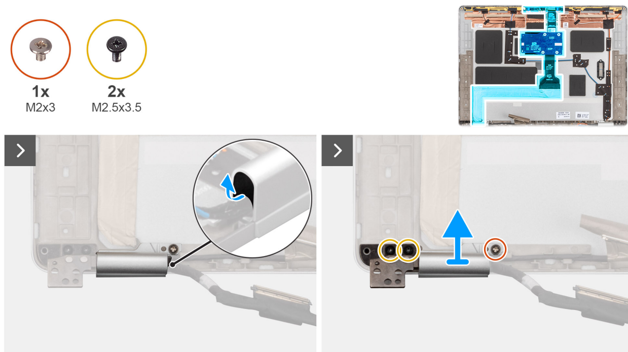
Figura 83. Rimozione del cavo del display
