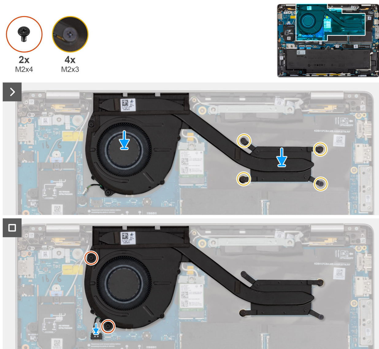
Figura 44. Installazione del gruppo ventola e dissipatore di calore
