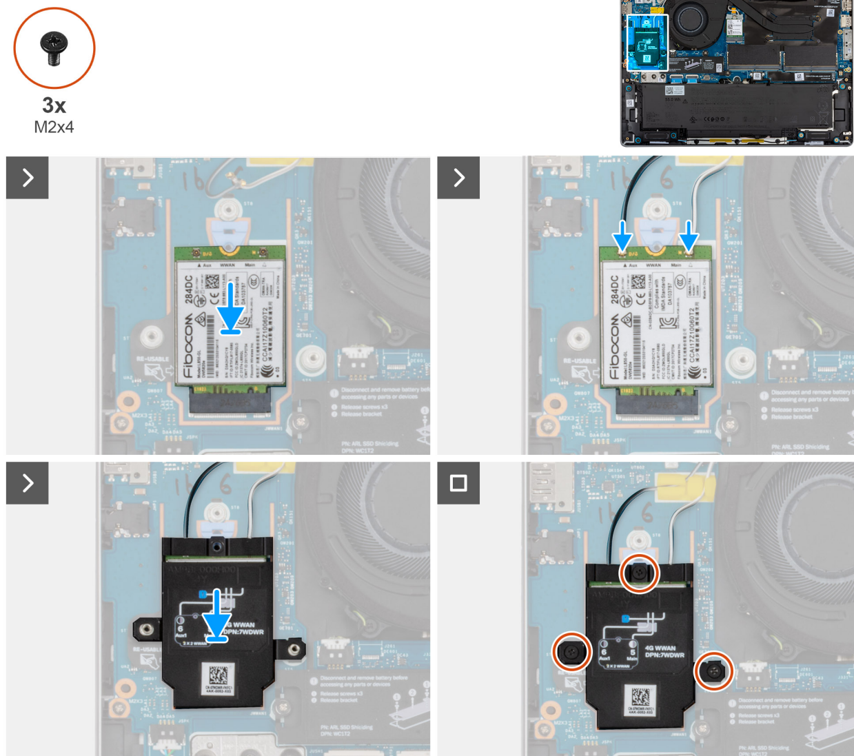
Figura 34. Installazione della scheda WWAN
