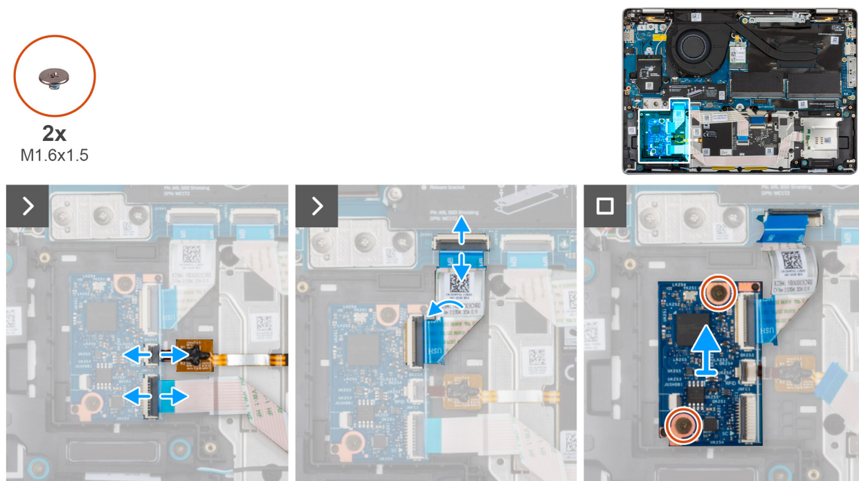
Figura 45. Rimozione della scheda figlia USH
