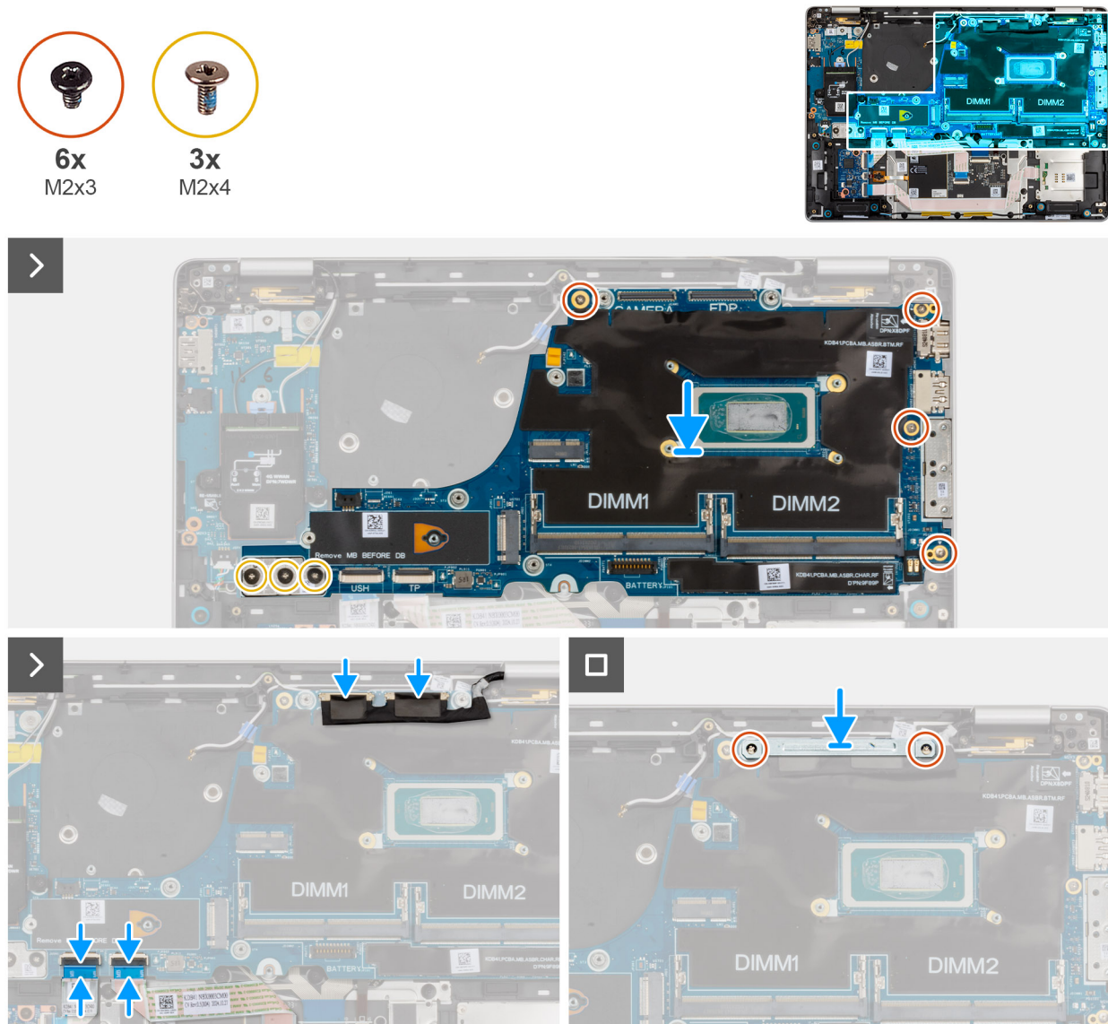
Figura 52. Installazione della scheda di sistema
