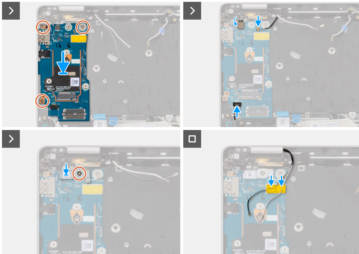
Figura 60. Installazione della scheda di I/O
