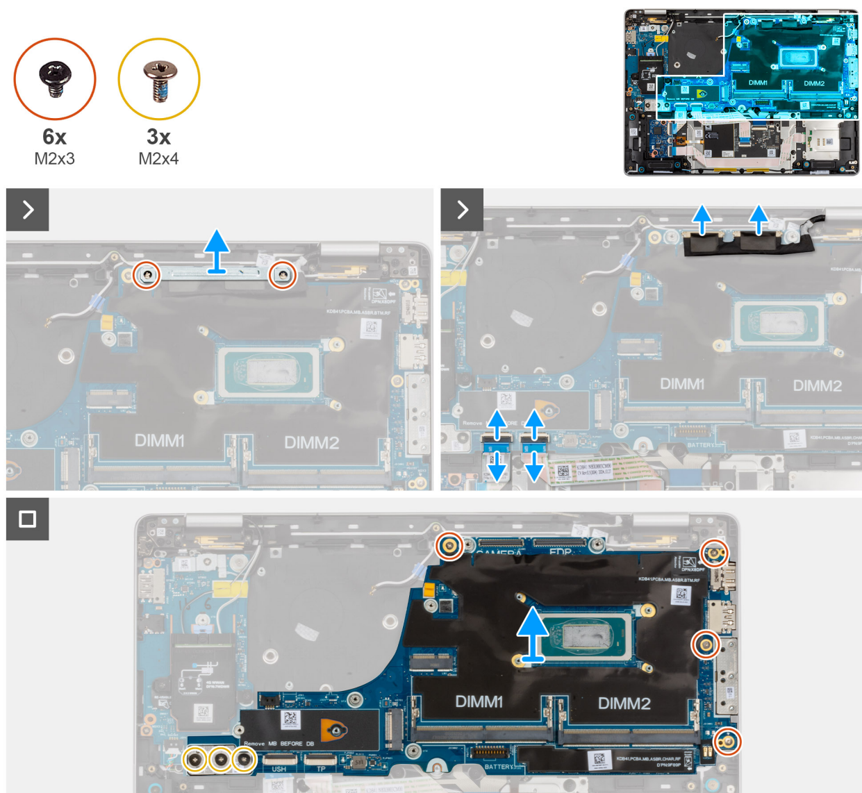
Figura 50. Rimozione della scheda di sistema
