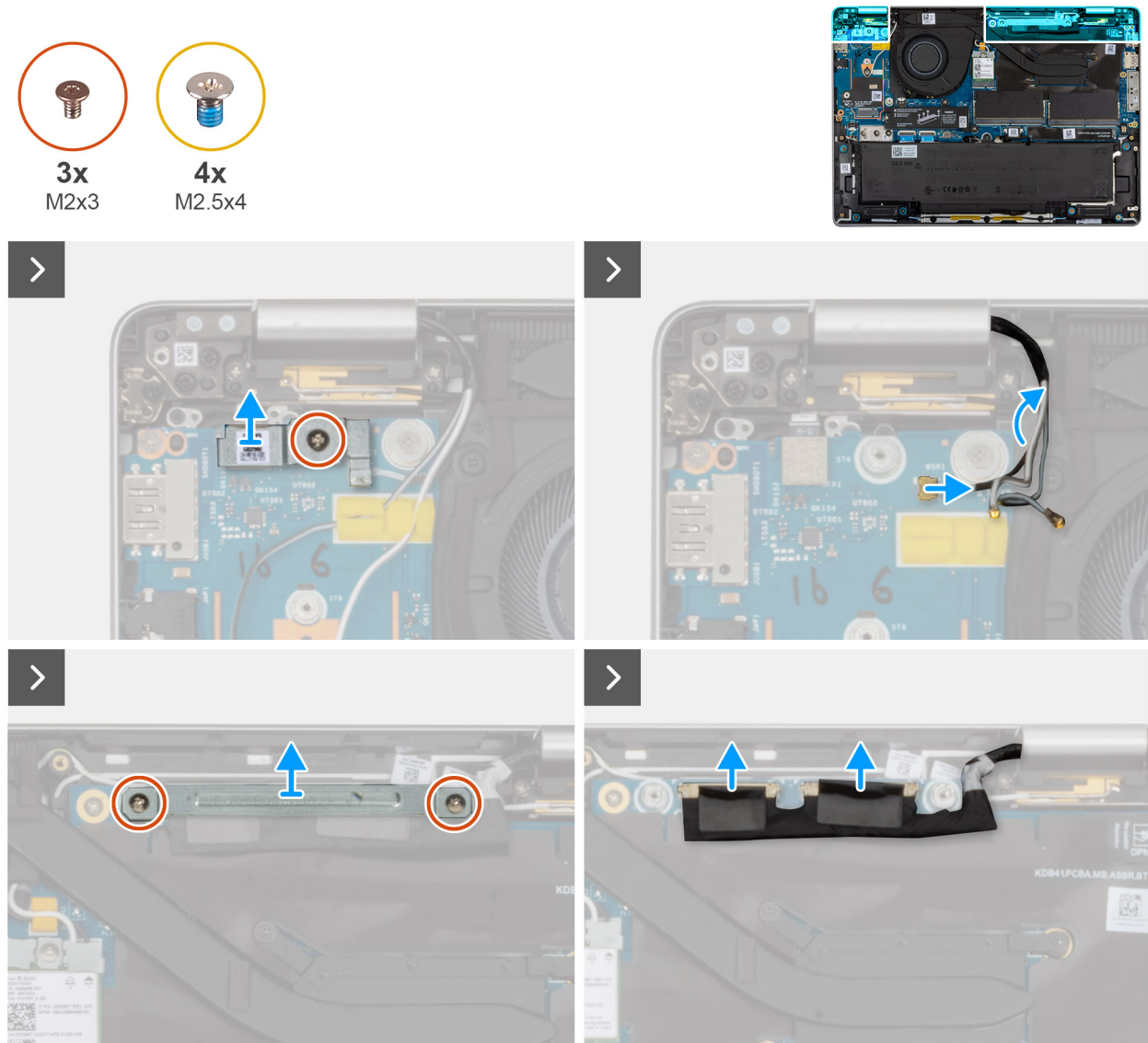
Figura 63. Rimozione del gruppo del display
