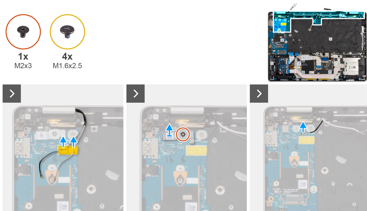
Figura 53. Rimozione del modulo dell'antenna WLAN
