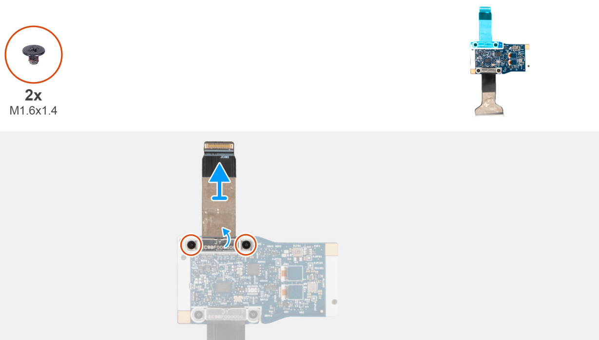
Figura 91. Rimozione del cavo della scheda figlia centrale
