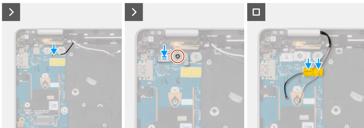
Figura 56. Installazione del modulo dell'antenna WLAN
