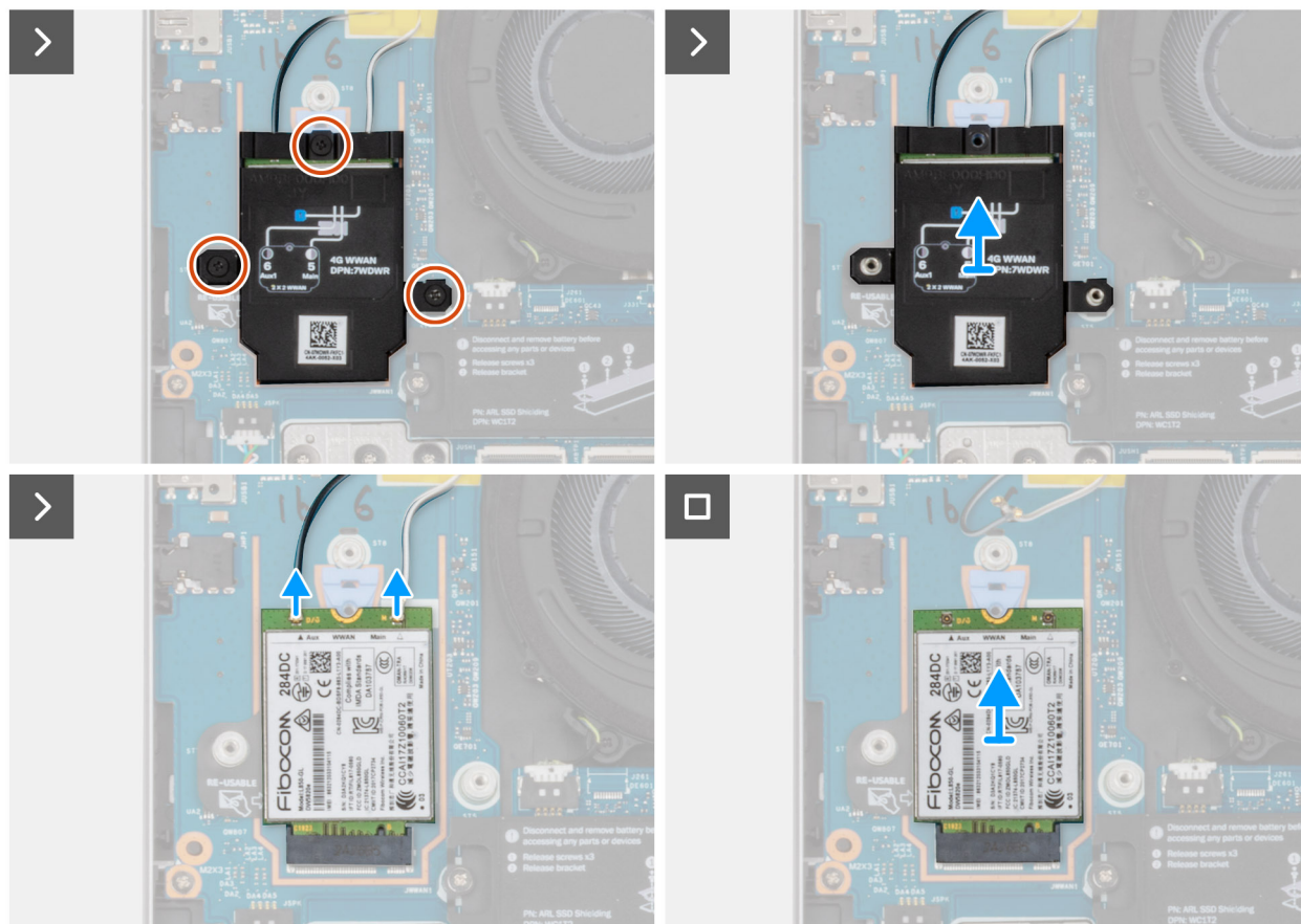
Figura 33. Rimozione della scheda WWAN
