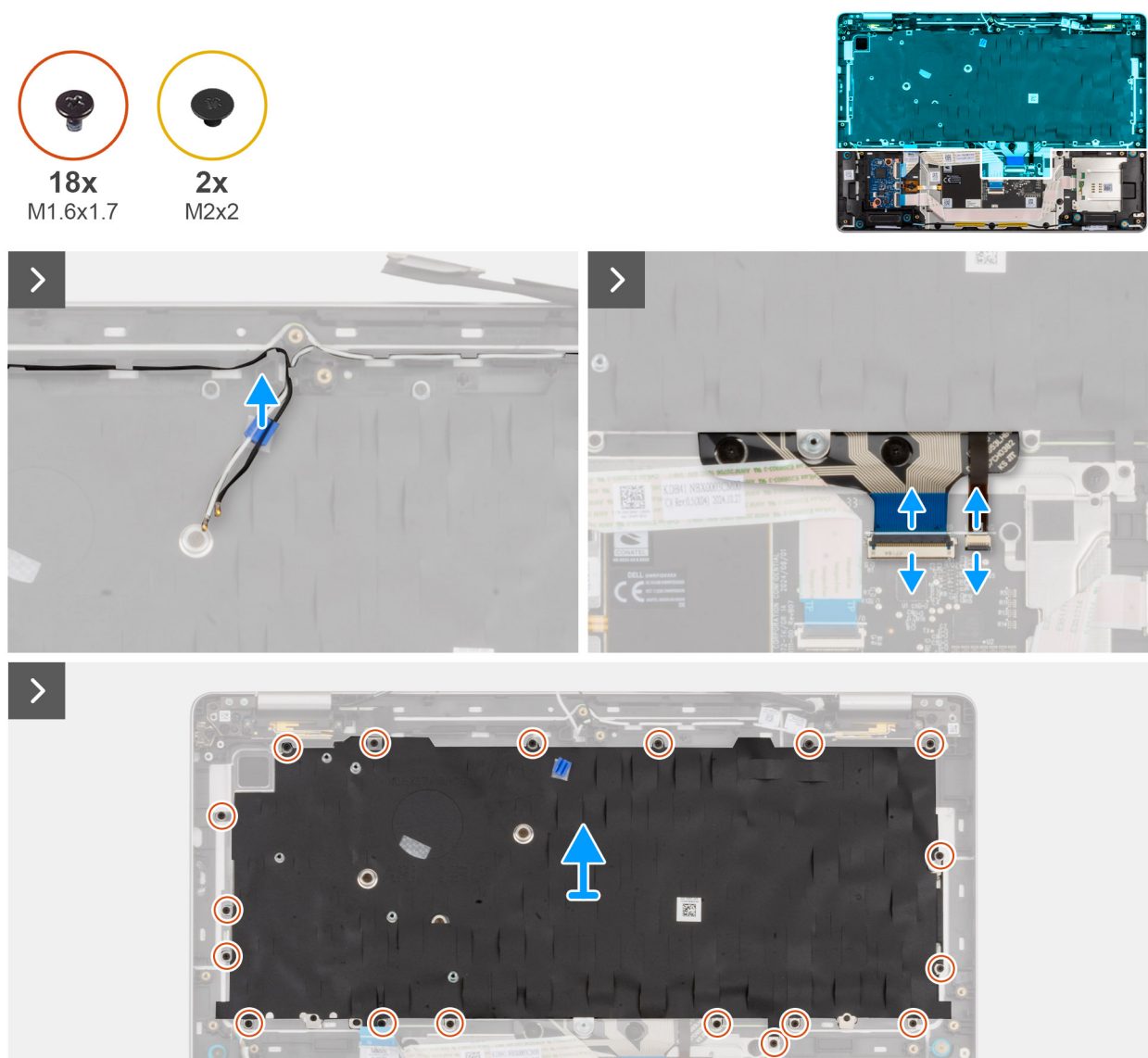
Figura 97. Rimozione della tastiera
