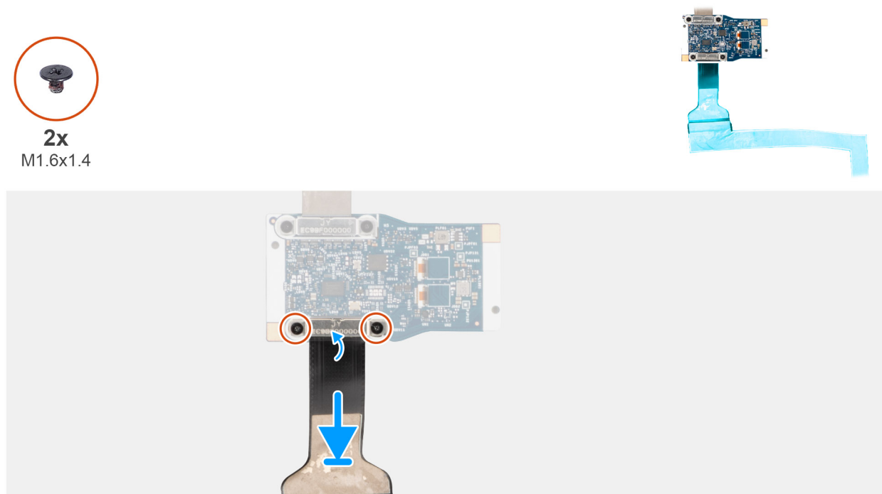
Figura 90. Installazione della cavo del display per la fotocamera MIPI
