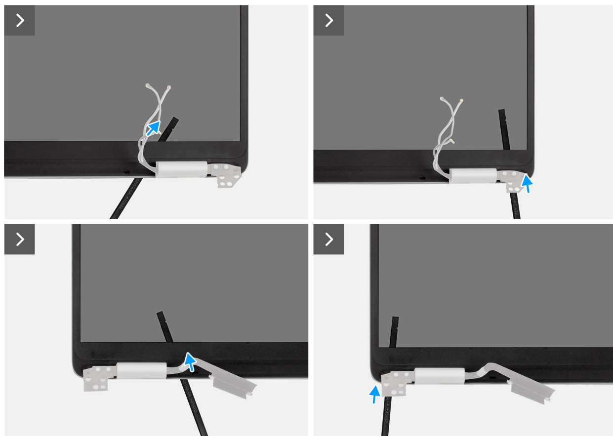
Figura 69. Rimozione della cornice del display
