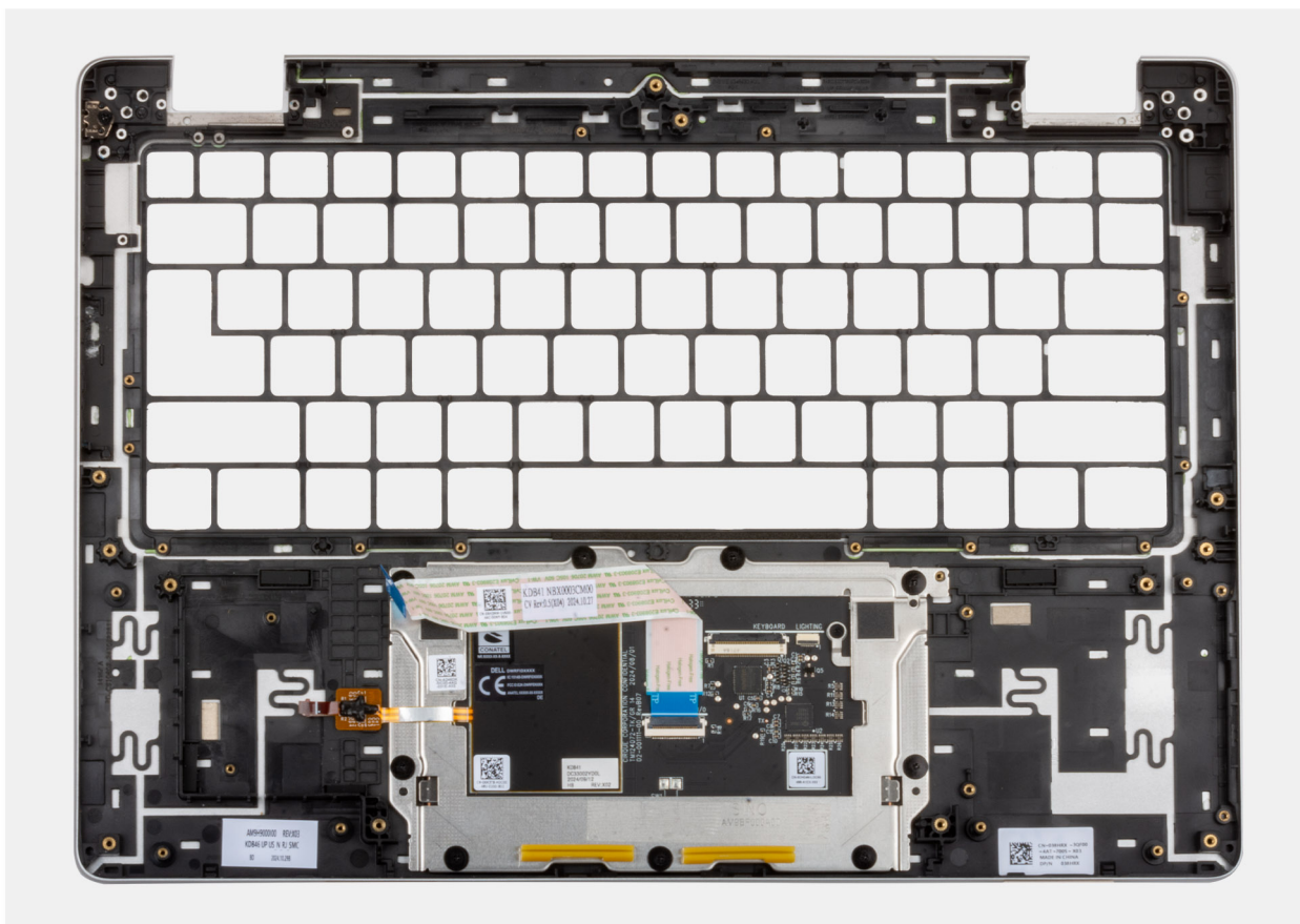
Figura 101. Gruppo del poggiapolsi
