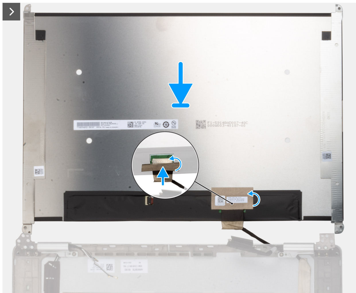
Figura 77. Installazione del pannello del display
