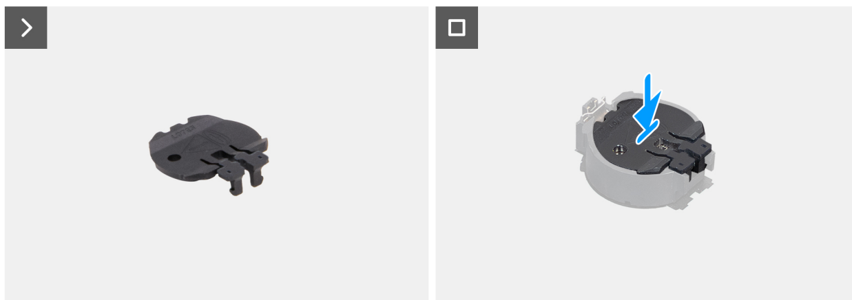
Rysunek 11. Instalowanie pokrywki baterii pastylkowej
