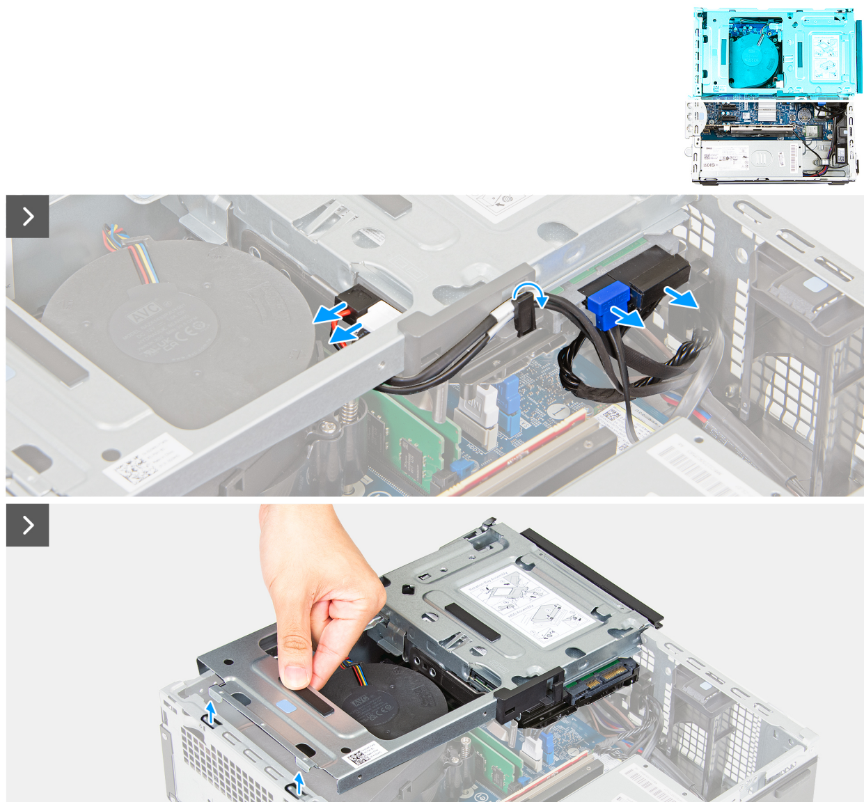
Rysunek 35. Wymontowywanie wnęki na dyski
