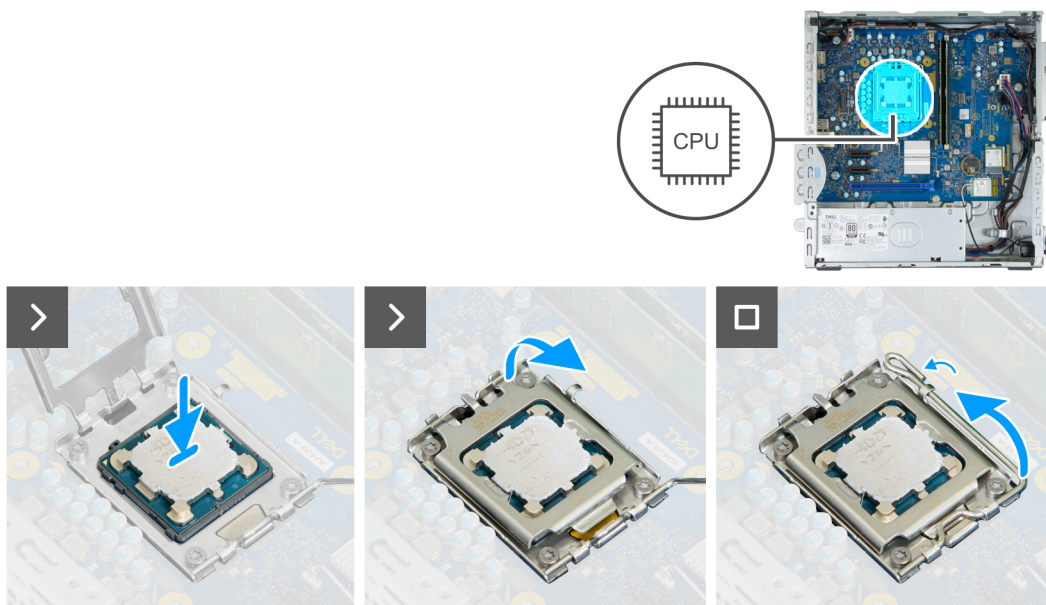
Rysunek 60. Instalowanie procesora
