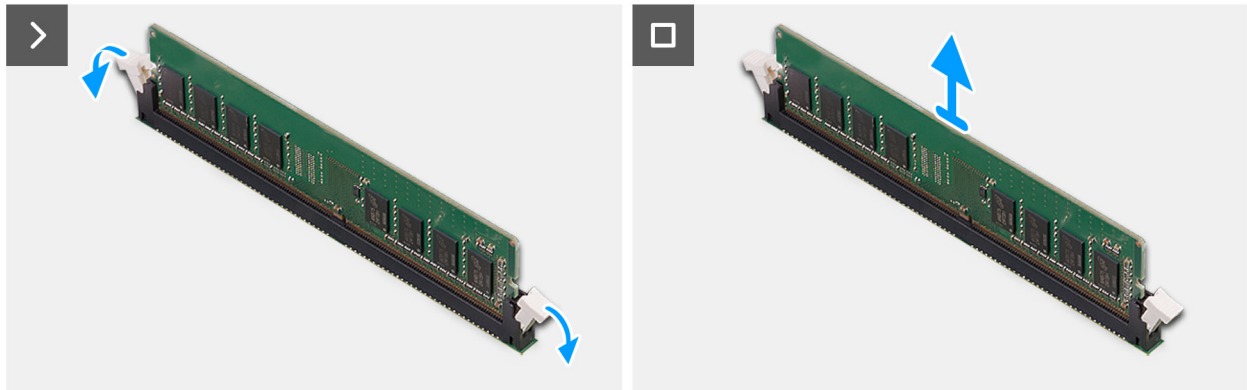
Afbeelding 27. Een geheugenmodule verwijderen
