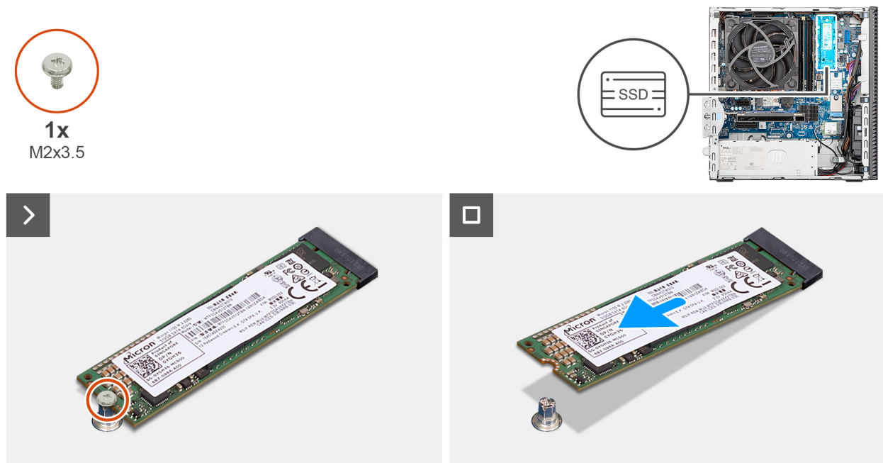
Afbeelding 35. De M.2 2280 SSD verwijderen
