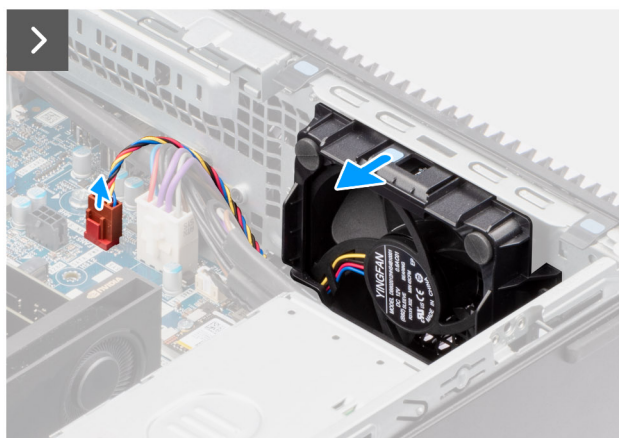
Afbeelding 47. De chassisventilator verwijderen
