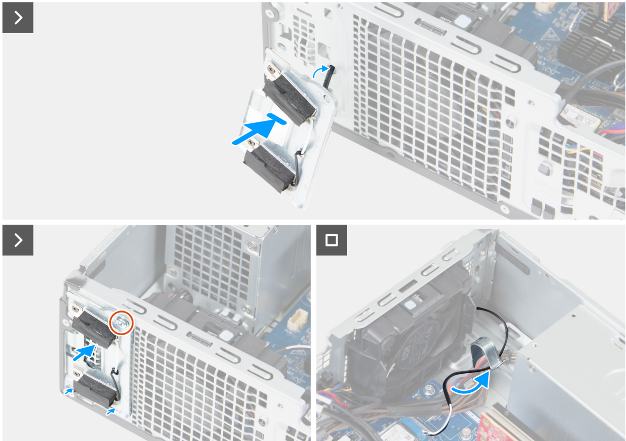
Afbeelding 50. De antennemodule plaatsen
