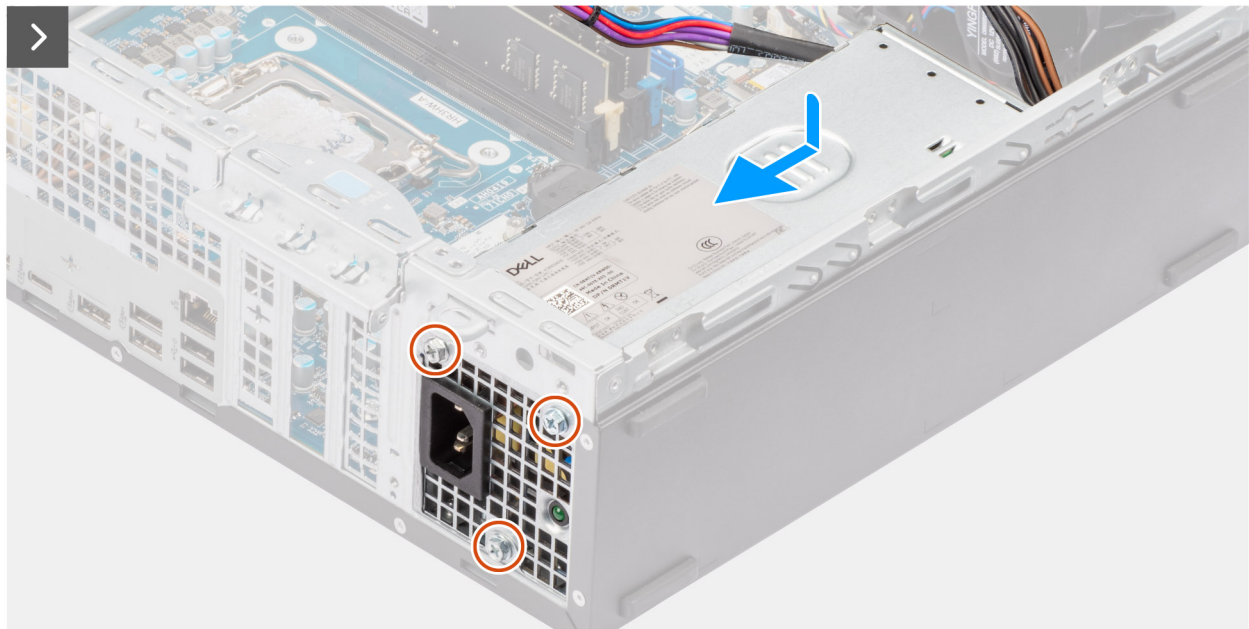
Afbeelding 59. De voedingseenheid plaatsen
