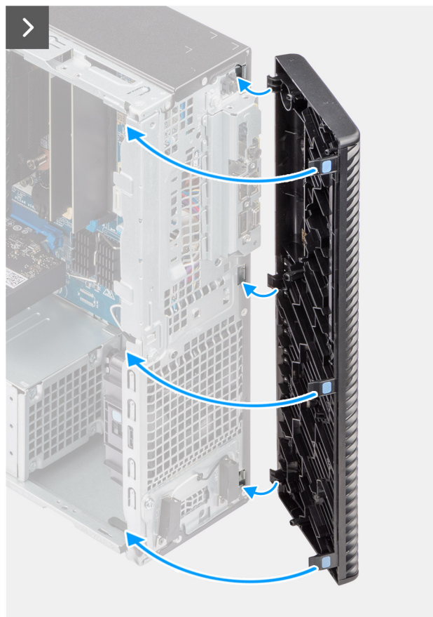
Afbeelding 16. Het voorpaneel plaatsen
