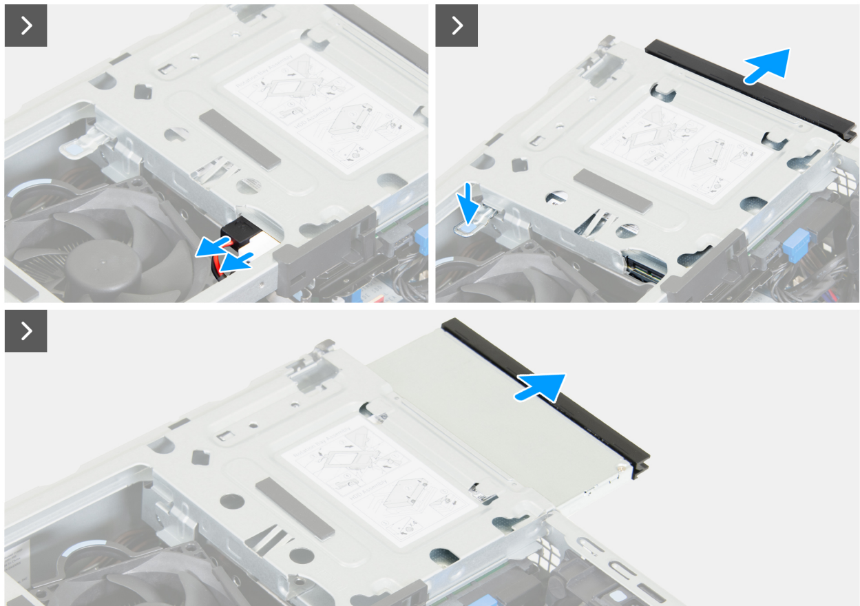
Afbeelding 17. Het optische station verwijderen
