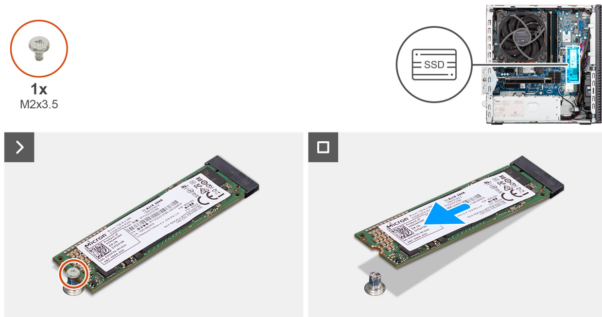
Afbeelding 37. De M.2 2280 SSD verwijderen
