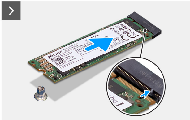
Afbeelding 36. De M.2 2280 SSD installeren
