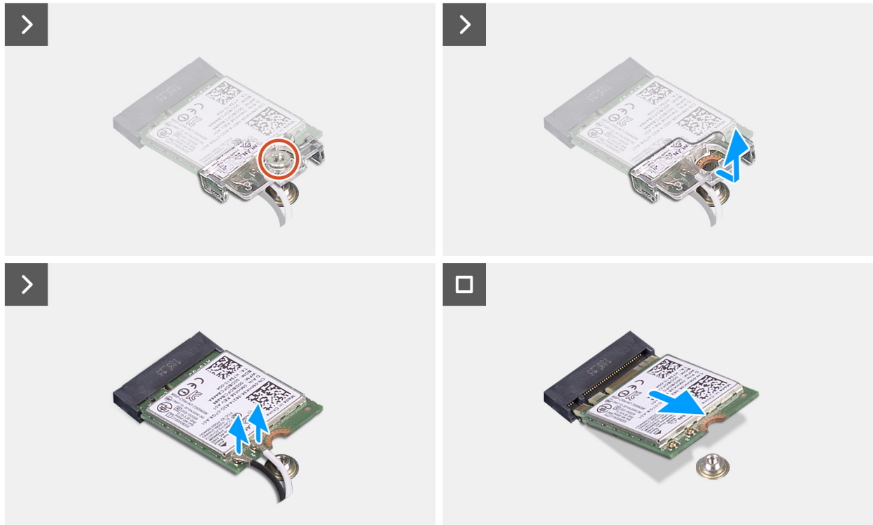
Afbeelding 41. De draadloze kaart verwijderen
