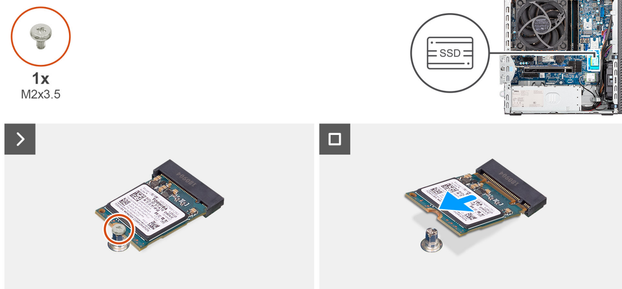
Afbeelding 31. De M.2 2230 SSD verwijderen
