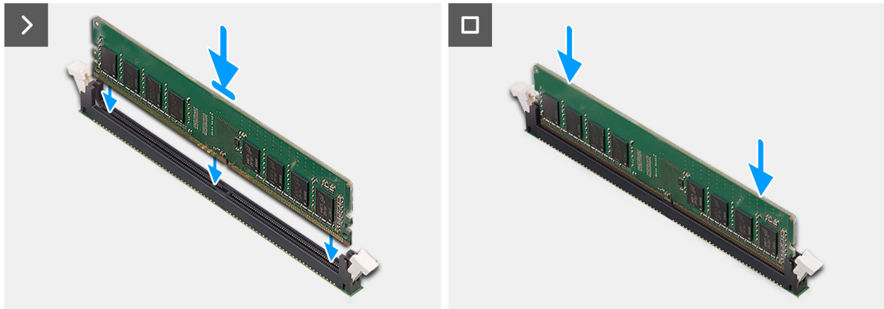
Afbeelding 28. De geheugenmodule plaatsen
