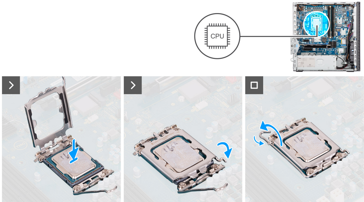
Afbeelding 56. De processor plaatsen
