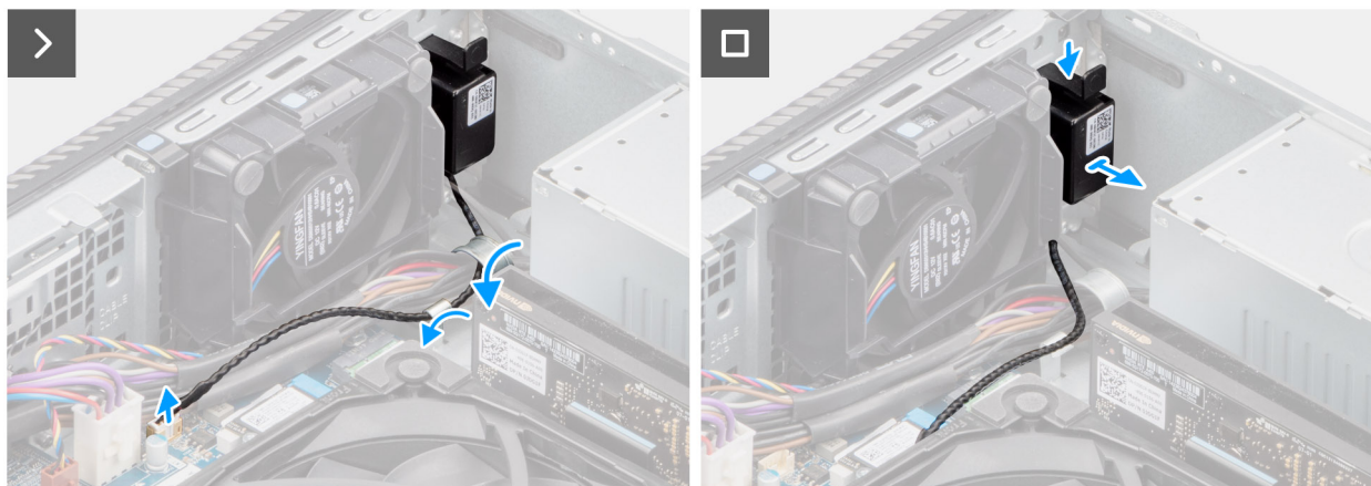
Afbeelding 25. De interne luidspreker verwijderen
