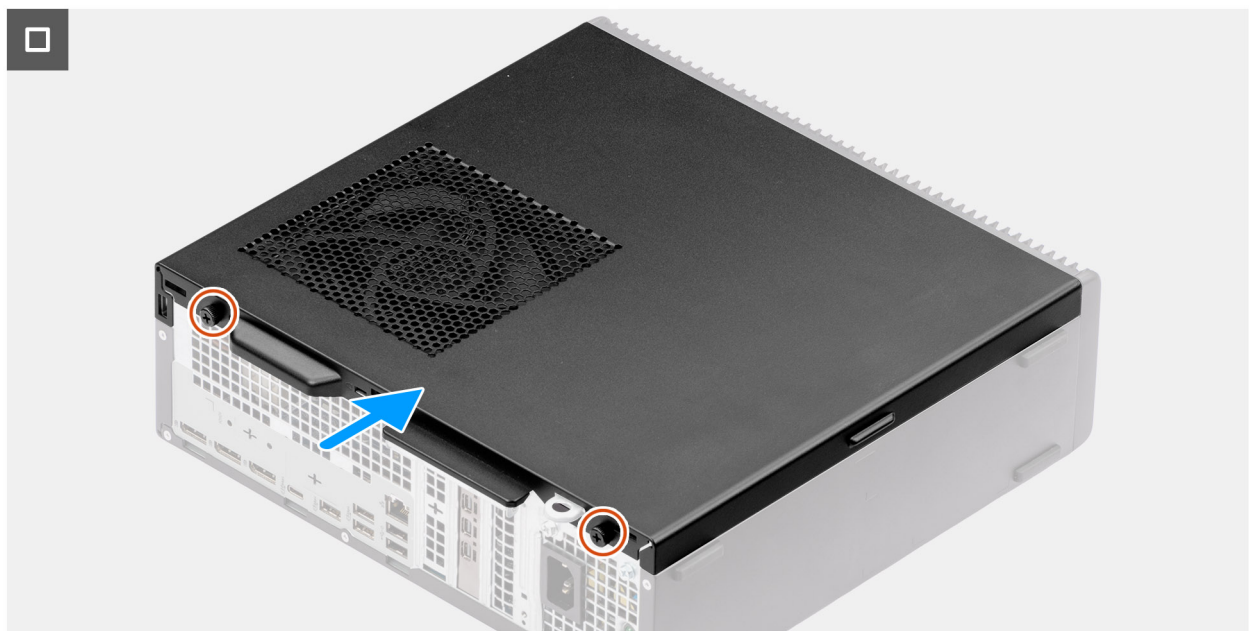
Afbeelding 12. De zijplaat plaatsen
