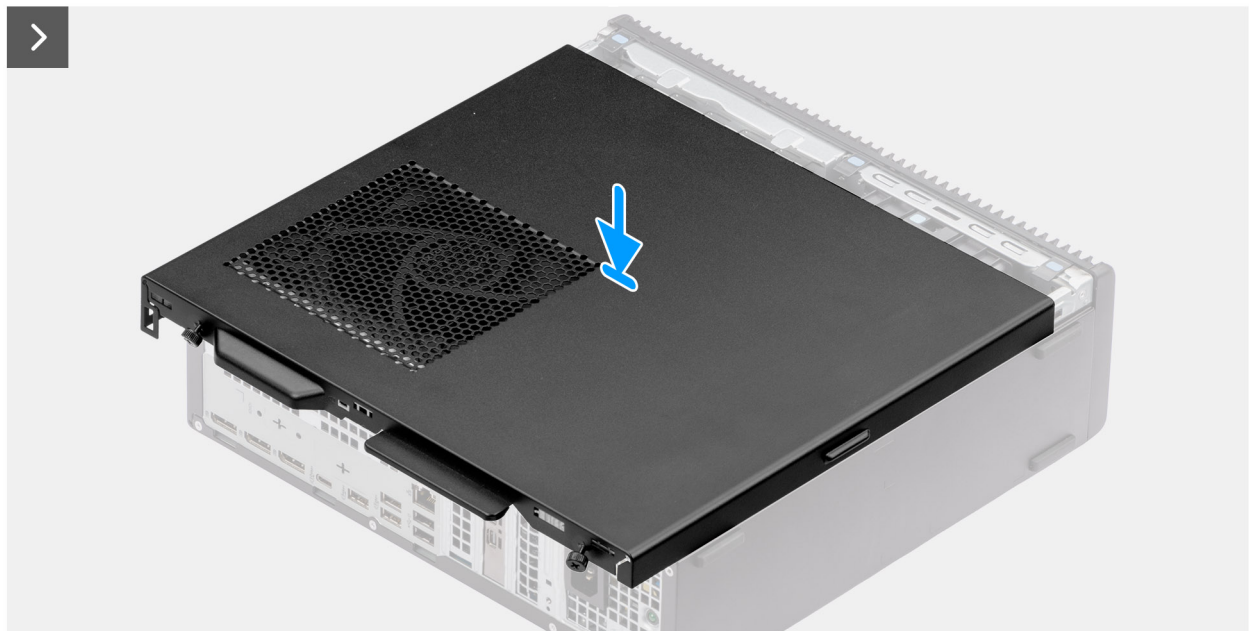
Afbeelding 11. De zijplaat plaatsen
