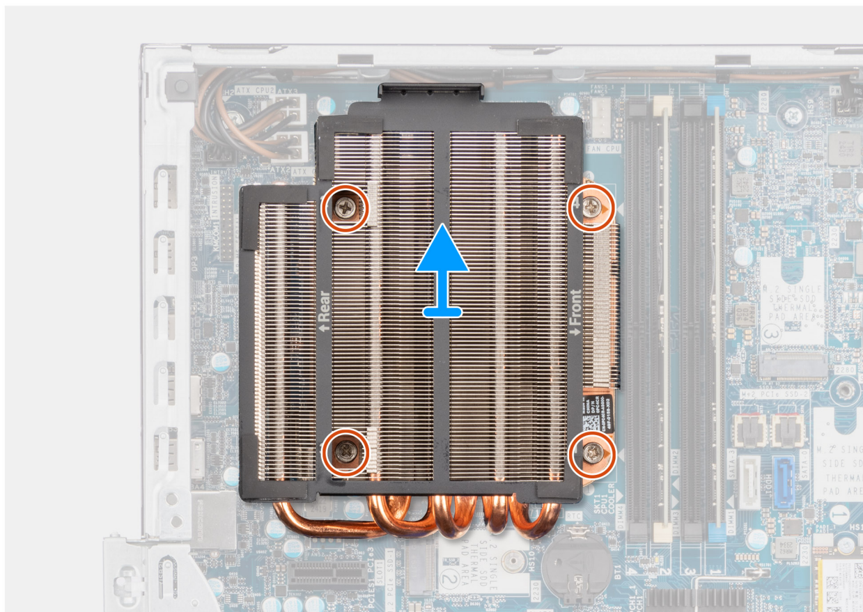
Afbeelding 53. De koelplaatteenheid van de processor verwijderen
