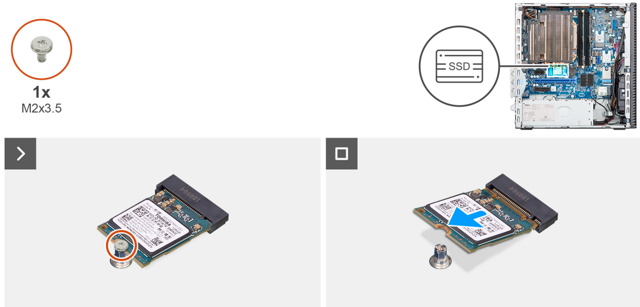
Afbeelding 33. De M.2 2230 SSD verwijderen
