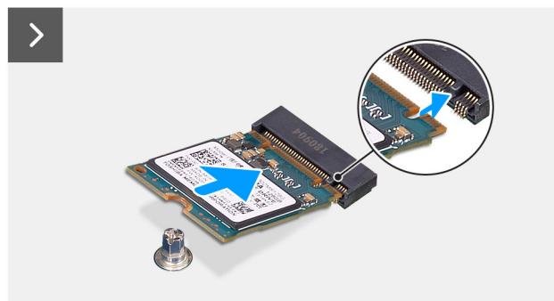
Afbeelding 32. De M.2 2230 SSD in slot 0 installeren
