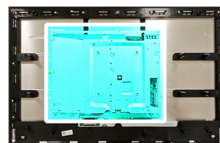
Figura 21. Rimozione della schermatura metallica
