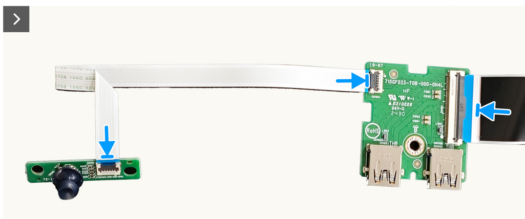
Figura 43. Installazione della scheda I/O e della scheda del tasto del joystick
