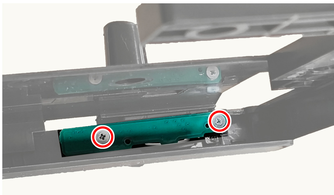
Figura 40. Installazione della scheda del tasto di alimentazione
