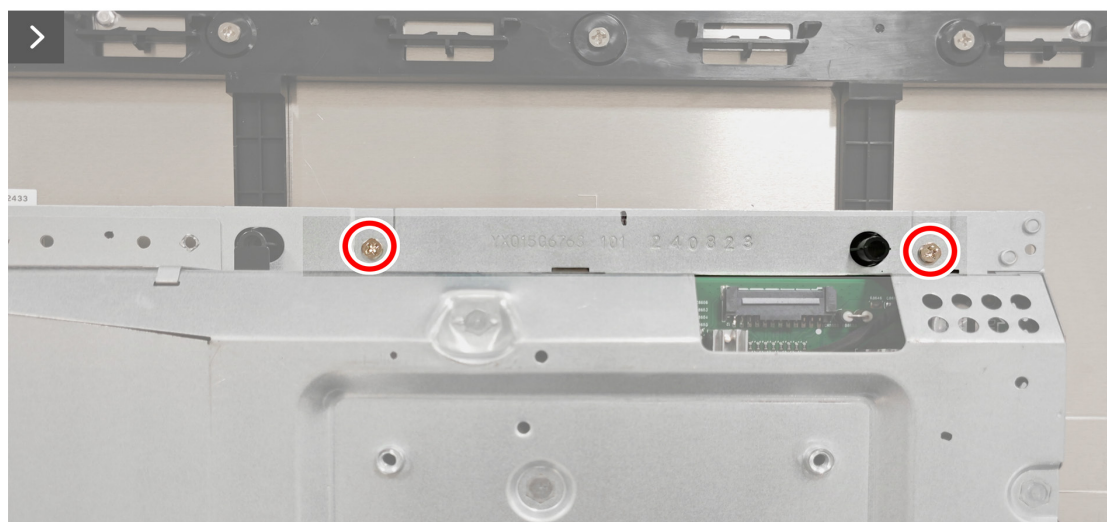
Figura 26. Installazione della schermatura metallica
