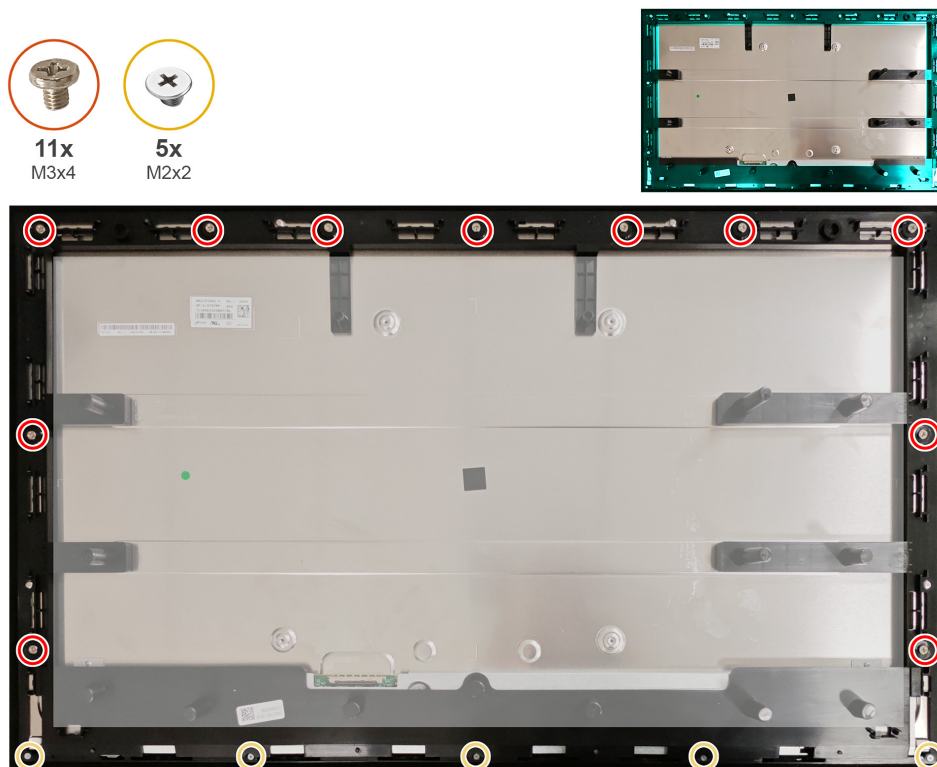
Figura 36. Rimozione della struttura centrale
