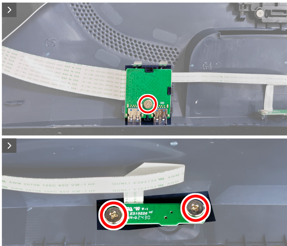
Figura 41. Rimozione della scheda I/O e della scheda del tasto del joystick
