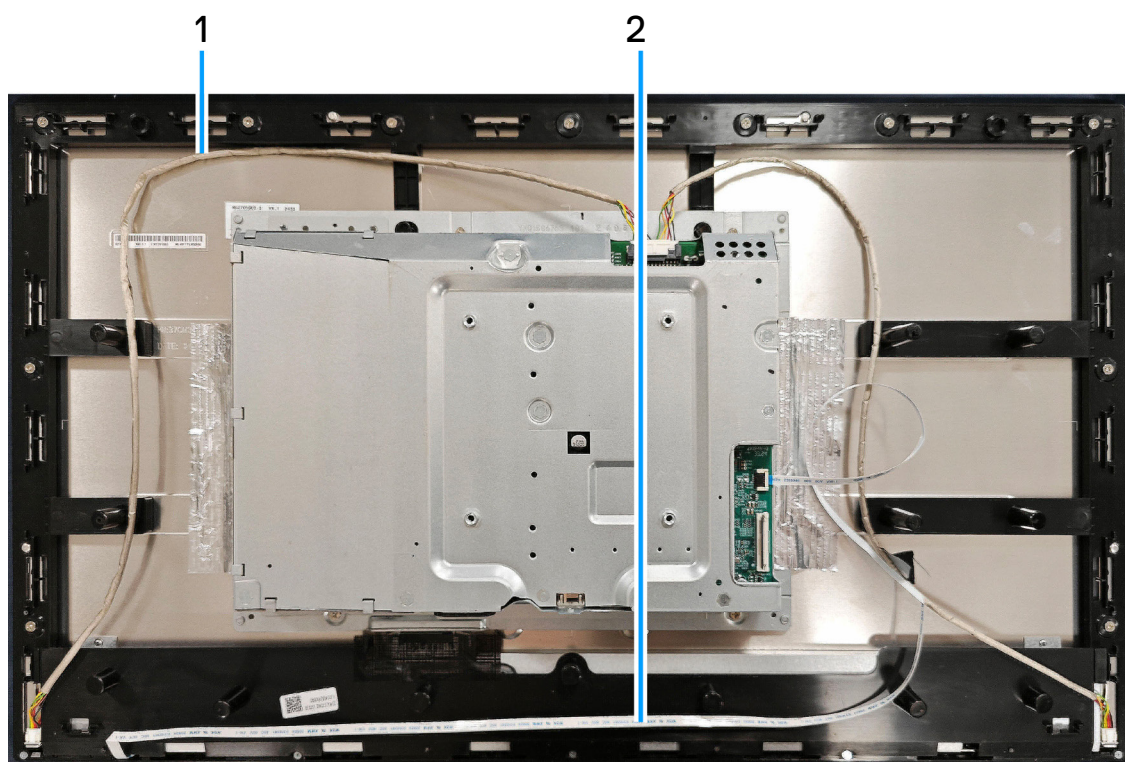
Figura 6. Schema di connettività elettrica
