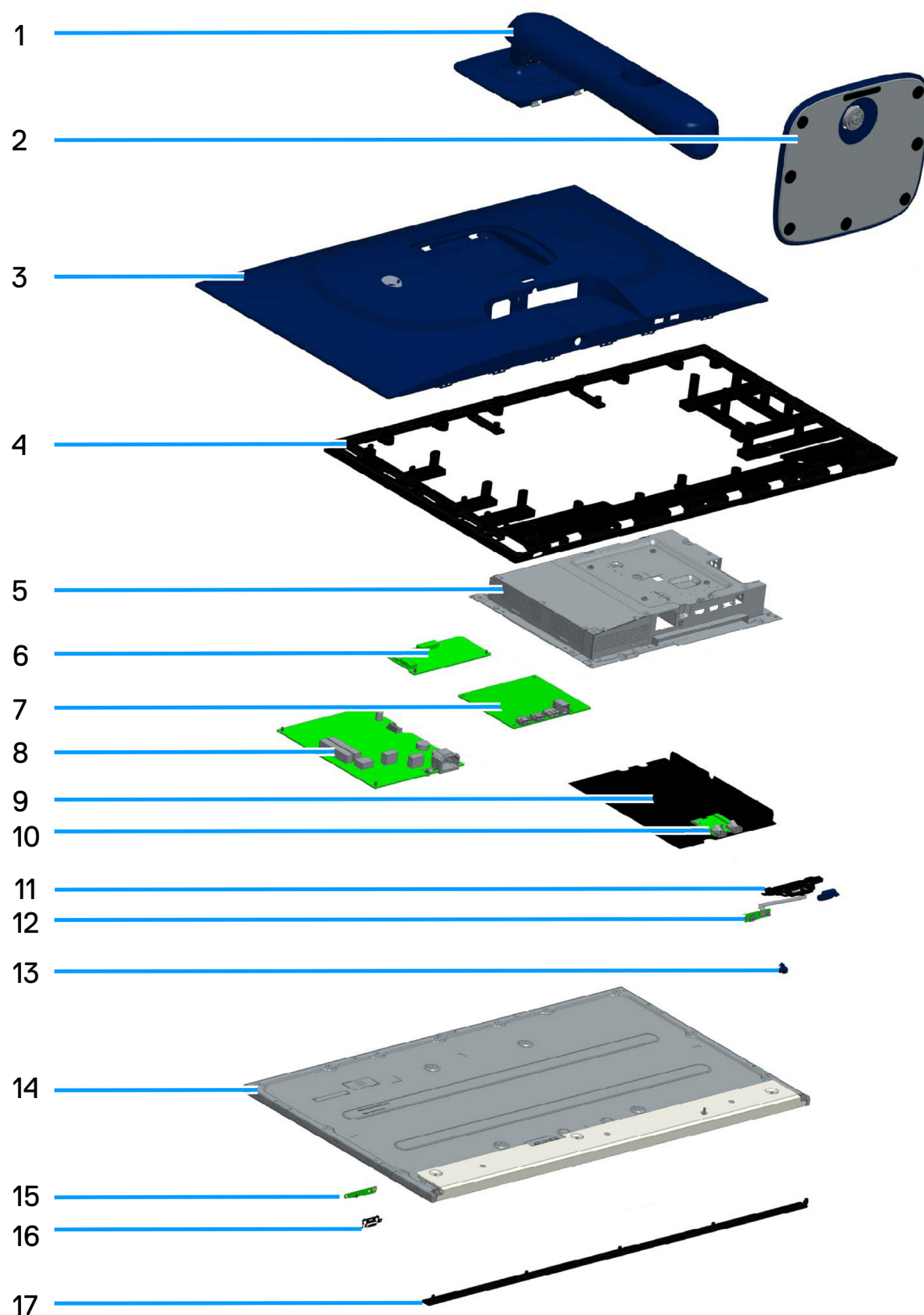
Figura 5. Componenti principali di AW2725DM
