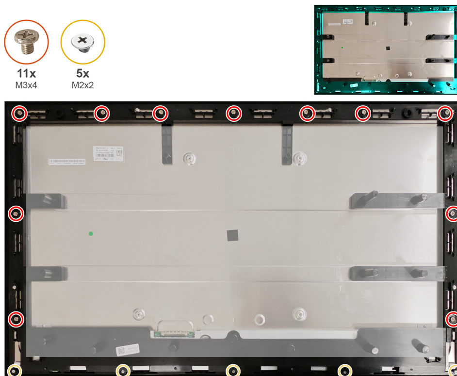
Figura 37. Installazione della struttura centrale
