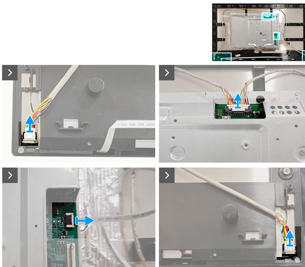
Figura 21. Rimozione della schermatura metallica
