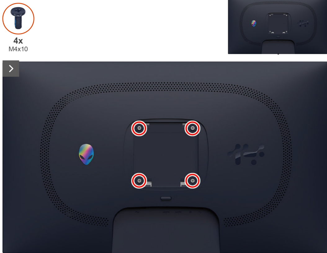
Figura 3. Quitar la cubierta posterior
