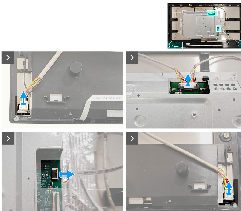
Figura 11. Quitar la protección metálica
