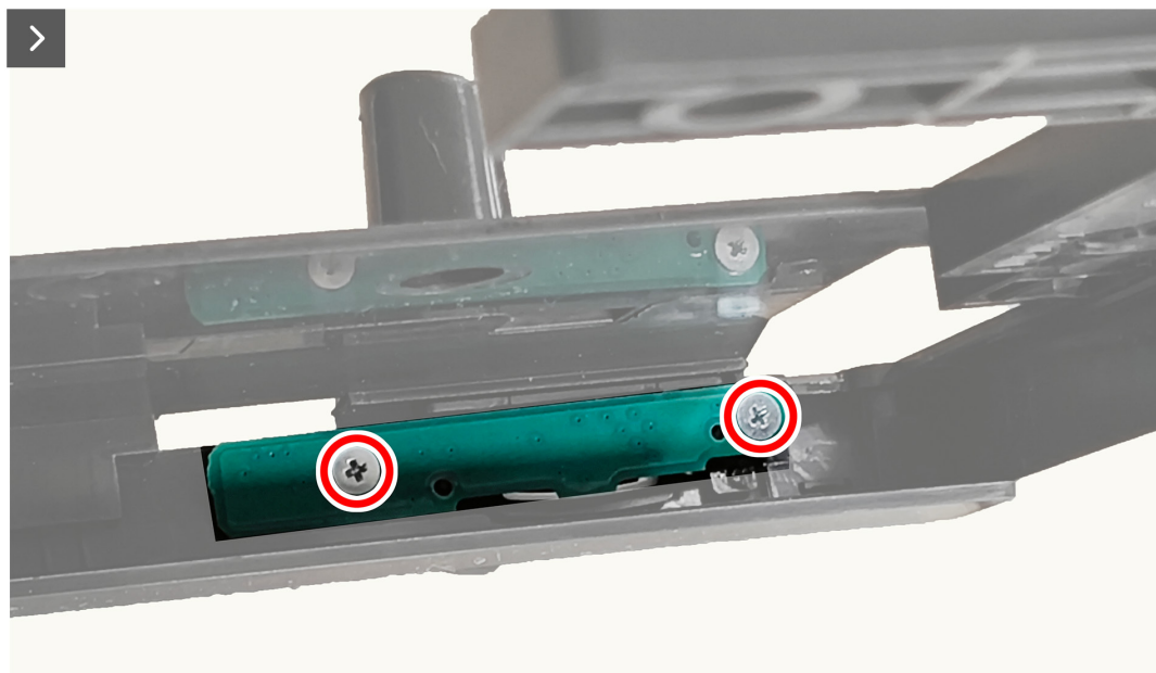
Figura 28. Quitar la placa del botón de alimentación
