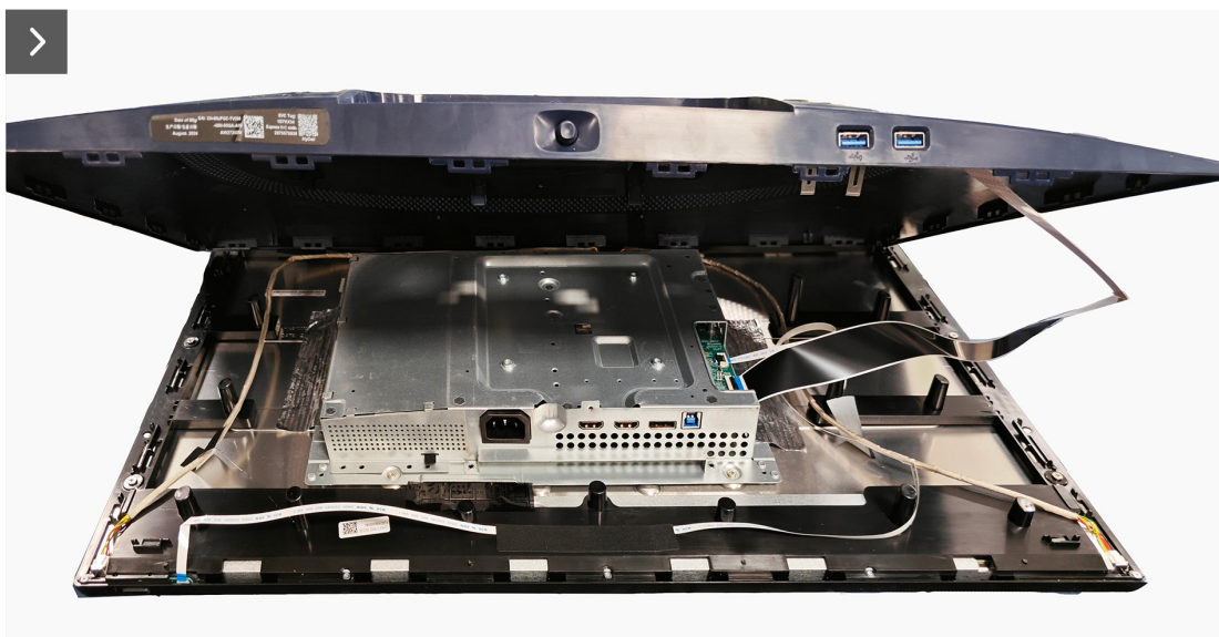
Figura 5. Quitar la cubierta posterior
