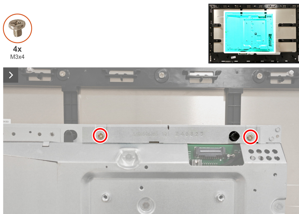
Figura 12. Quitar la protección metálica
