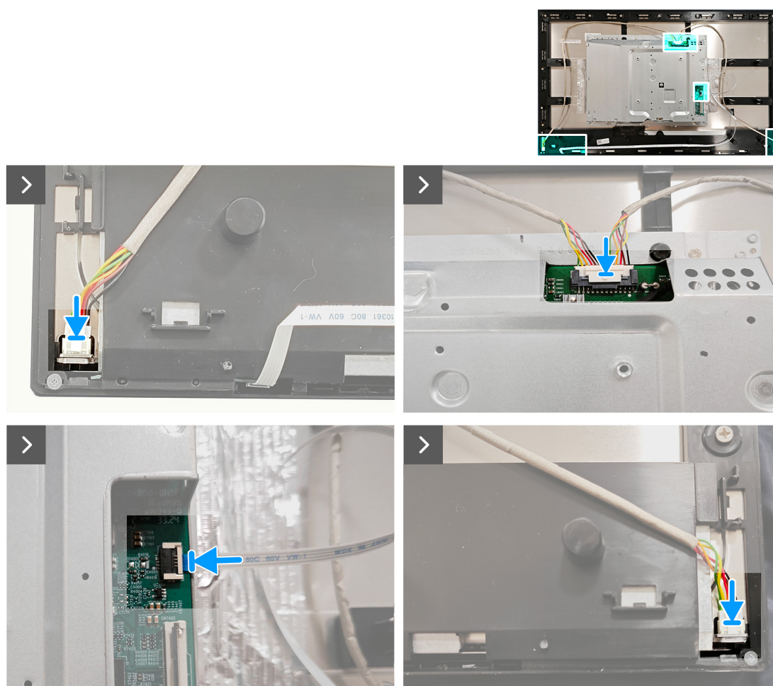
Figura 18. Instalar la protección metálica
