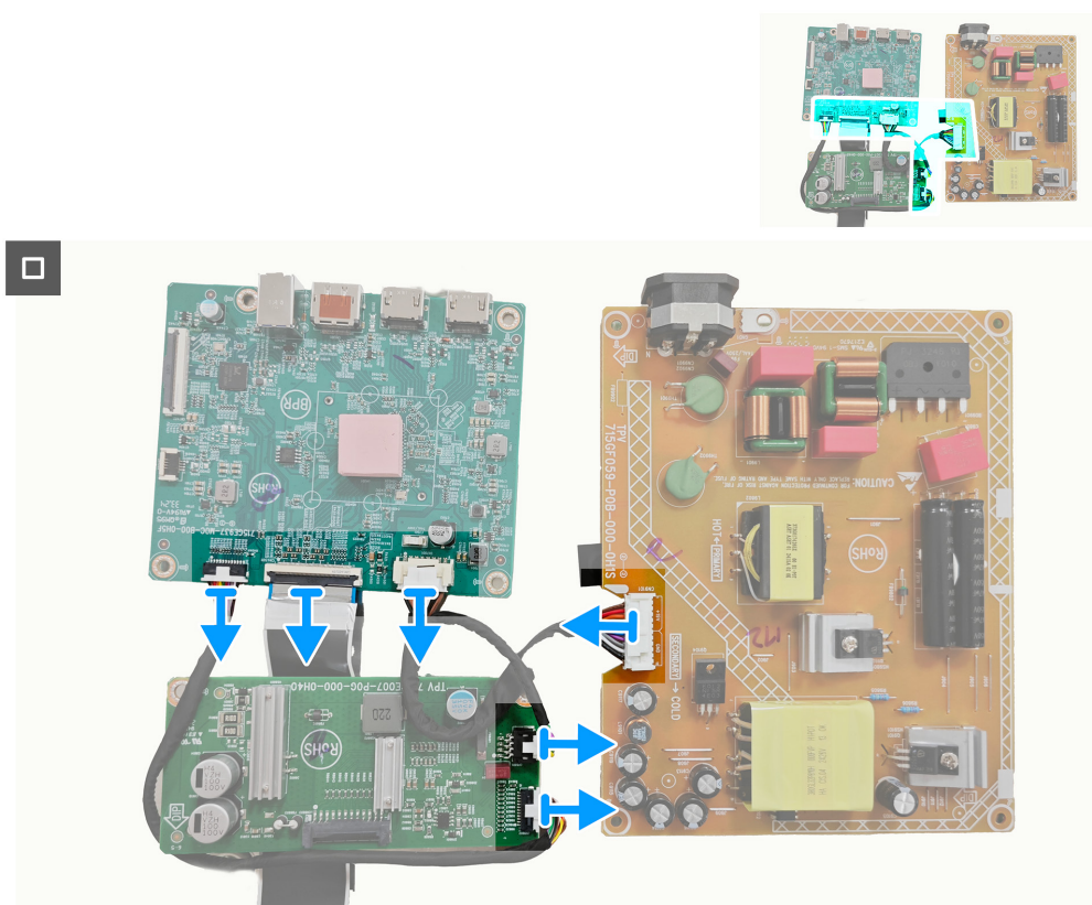
Figura 22. Quitar la placa del sistema y la placa de alimentación
