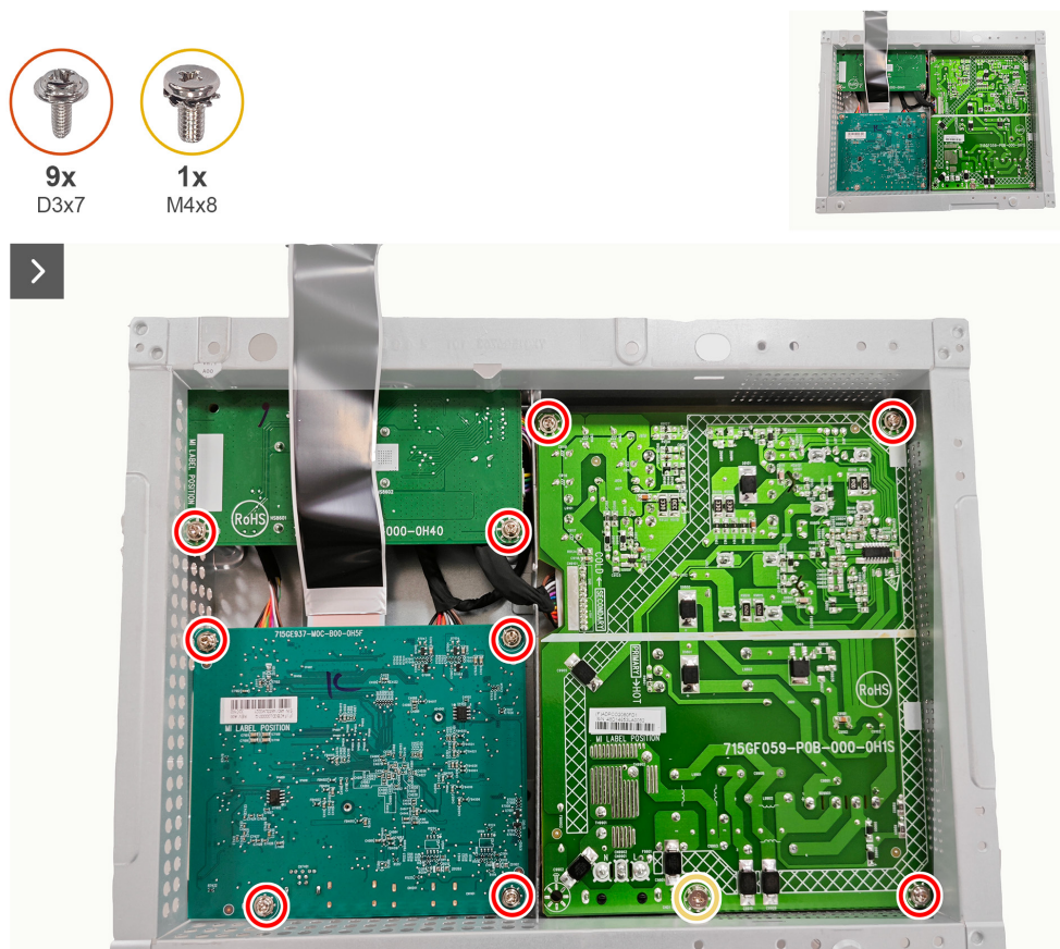
Figura 21. Quitar la placa del sistema y la placa de alimentación
