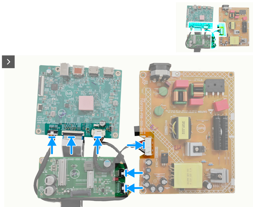
Figura 23. Instalar la placa del sistema y la placa de alimentación
