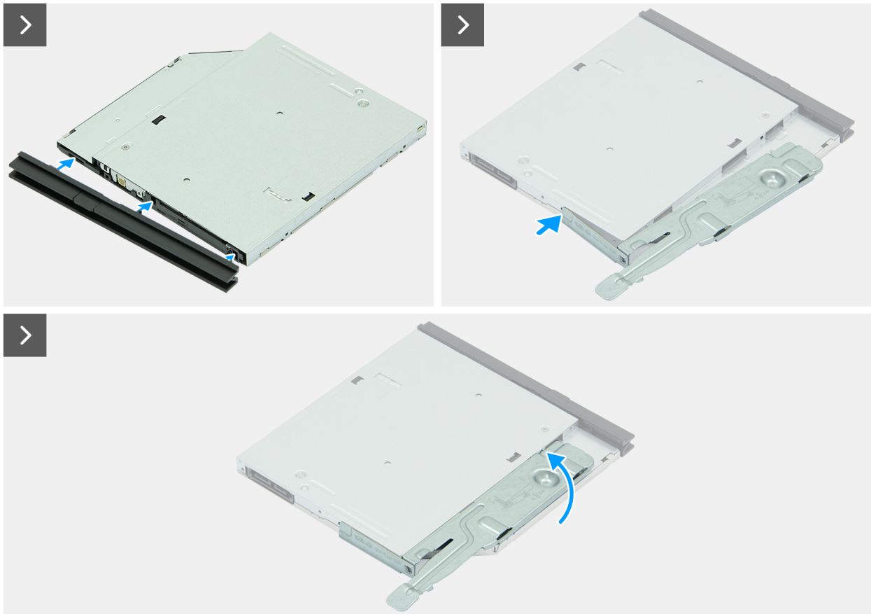
Abbildung 19. Installieren des optischen Laufwerks
