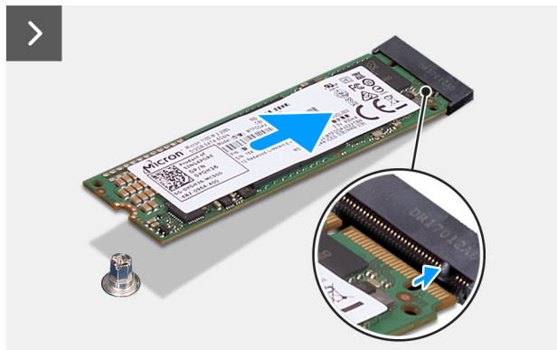
Abbildung 36. Einbauen des M.2-2280-Solid-State-Laufwerks
