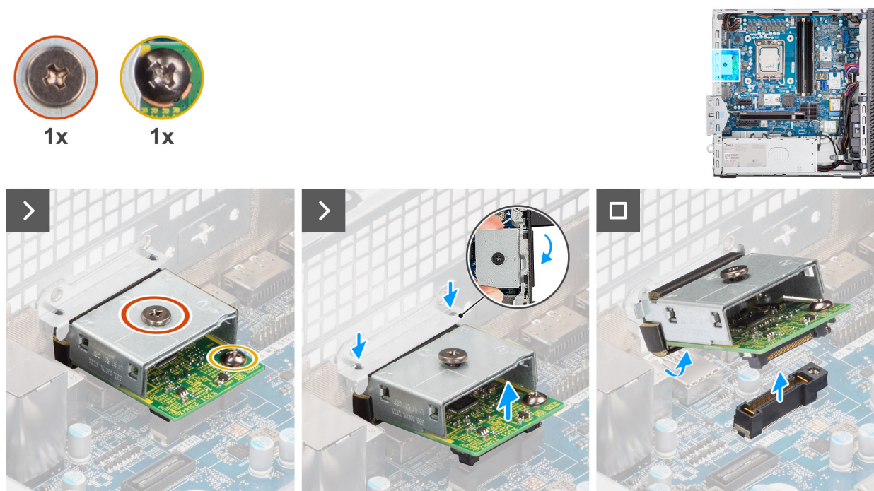
Abbildung 76. Entfernen des optionalen DisplayPort-Moduls
