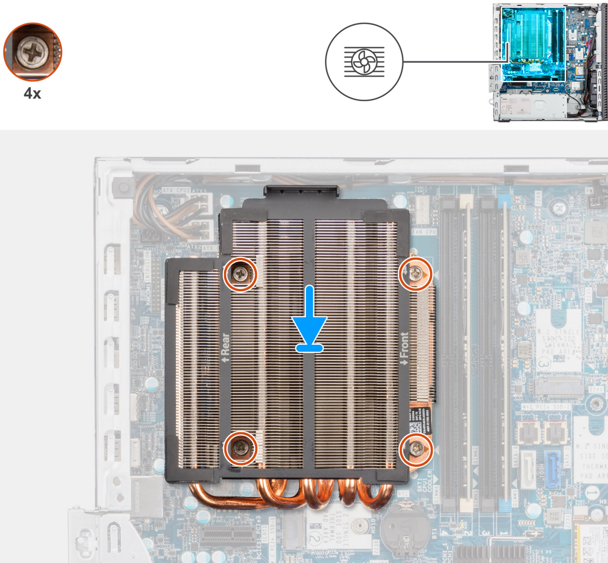
Abbildung 54. Installieren der Kühlkörperbaugruppe des Prozessors
