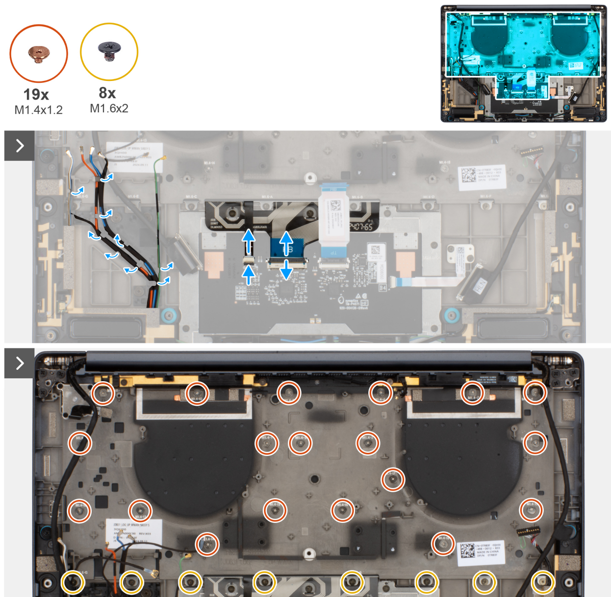
Afbeelding 71. De toetsenbordeenheid verwijderen
