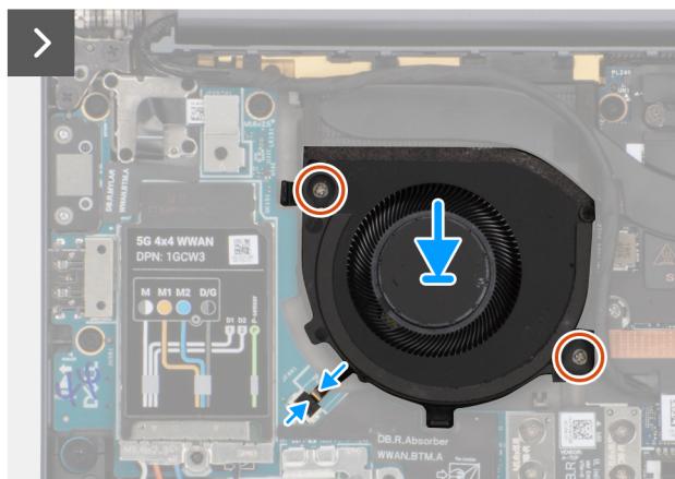
Afbeelding 31. De rechterventilator plaatsen
