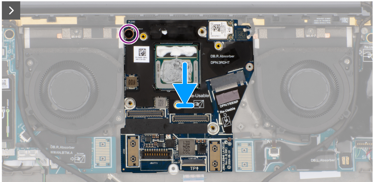
Afbeelding 67. De systeemkaart plaatsen
