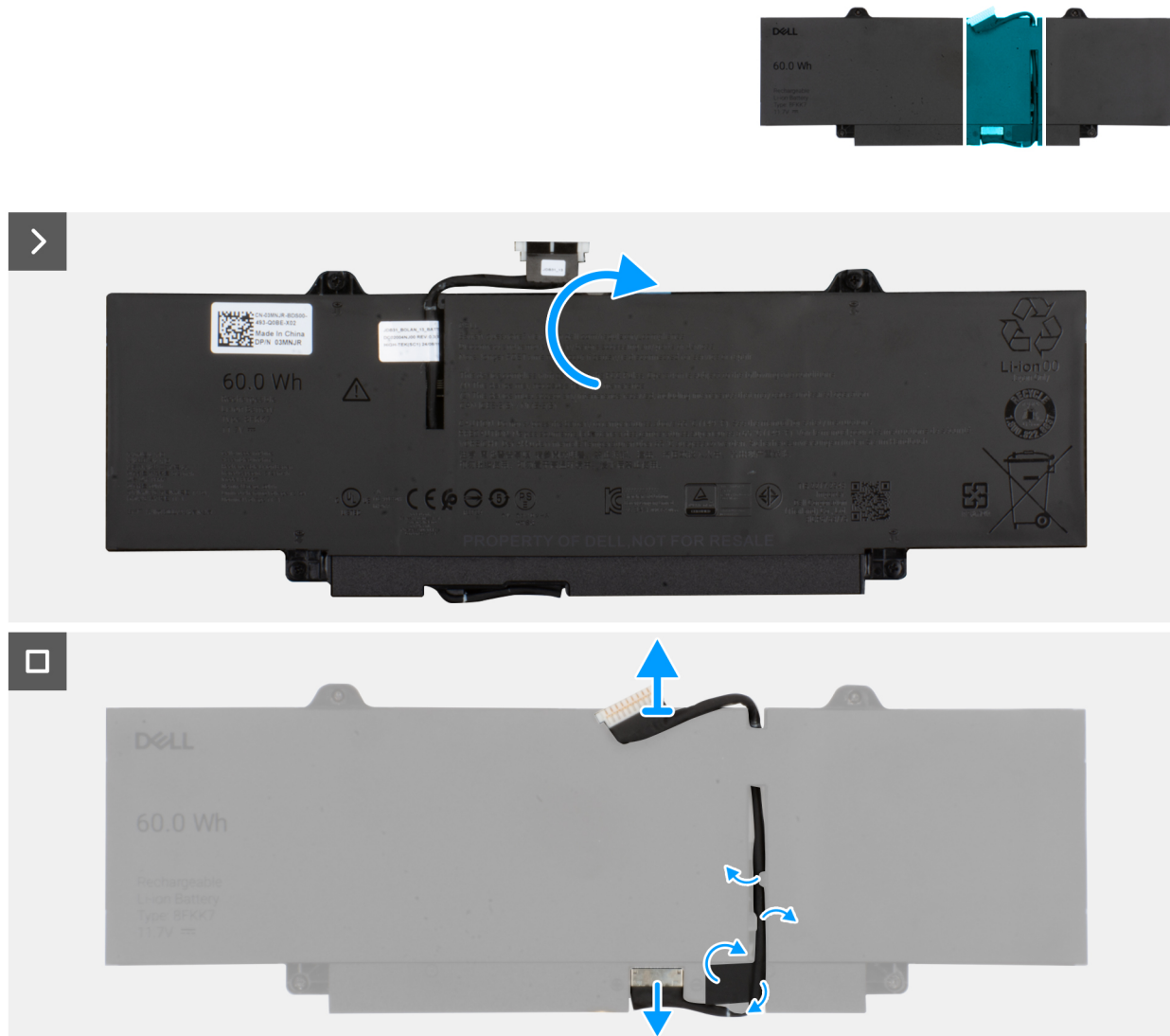
Afbeelding 22. De batterijkabel verwijderen en loskoppelen
