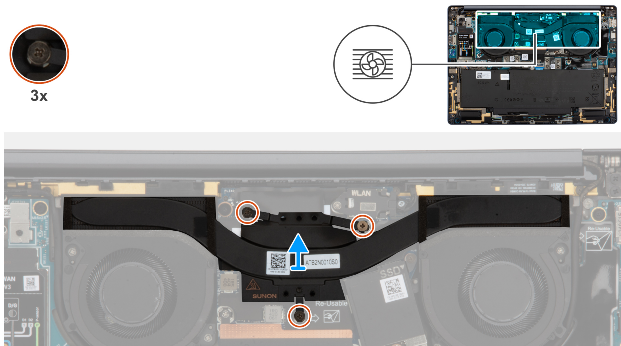
Afbeelding 36. De koelplaat verwijderen
