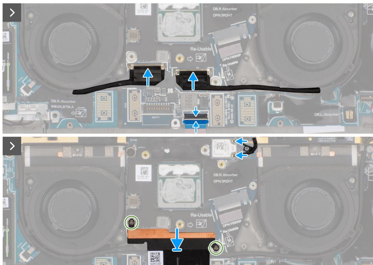
Afbeelding 68. De systeemkaart plaatsen
