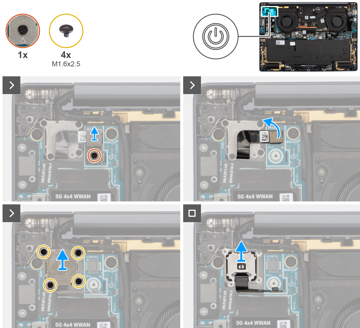
Afbeelding 54. De aan-uitknop verwijderen
