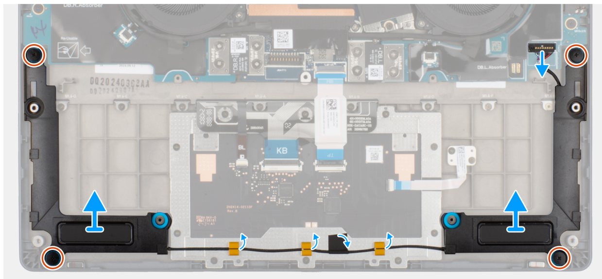
Afbeelding 32. De luidsprekers zonder antenne verwijderen (WLAN-configuratie)
