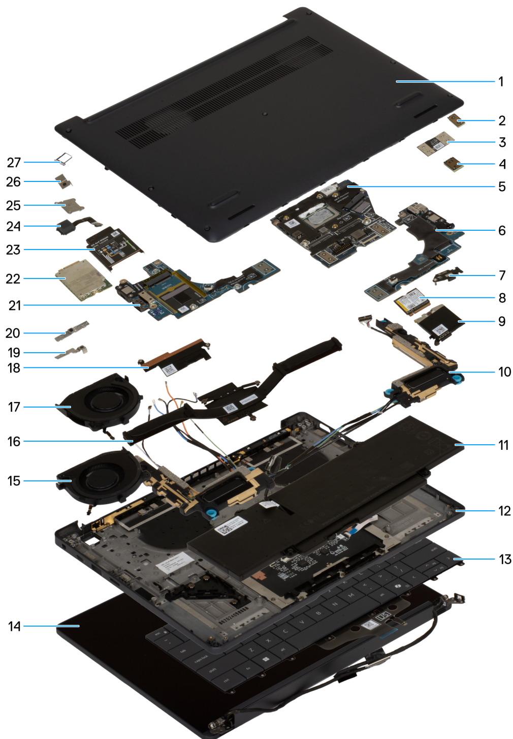
Afbeelding 9. Belangrijkste onderdelen van uw systeem/opengewerkte tekening
