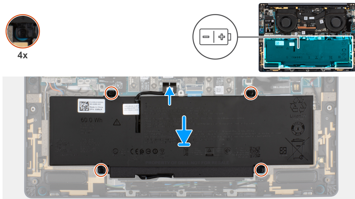
Afbeelding 21. De batterij plaatsen
