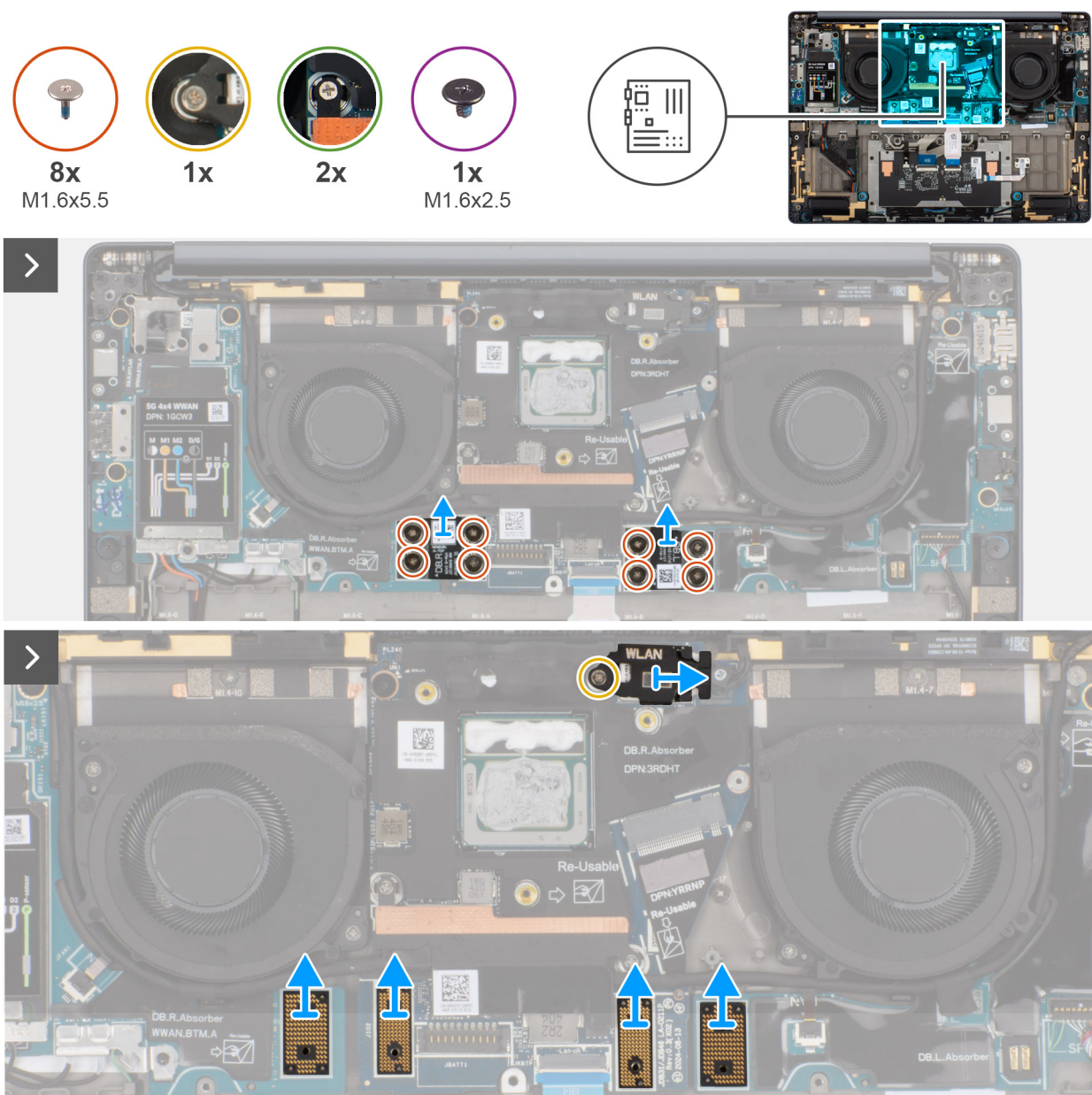
Afbeelding 62. De systeemkaart verwijderen
