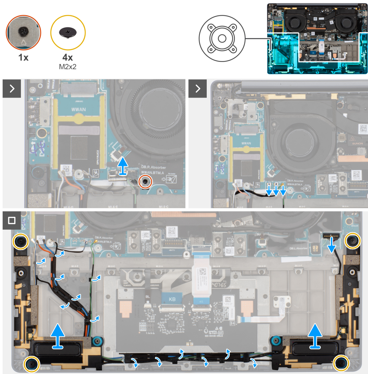
Afbeelding 34. De luidsprekers met antennes verwijderen (WWAN-configuratie)
