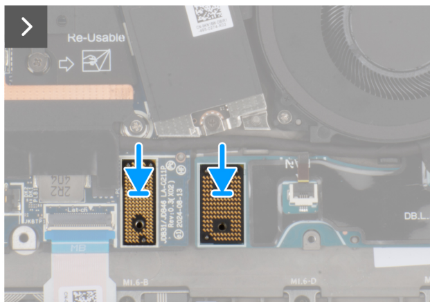
Afbeelding 40. De linker-I/O-kaart installeren
