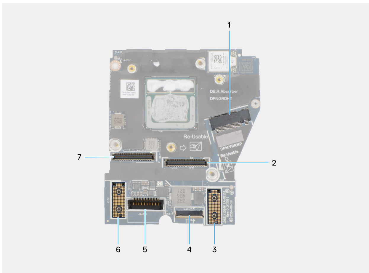
Afbeelding 66. Bijschriften voor de systeemkaart
