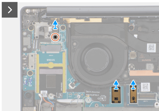
Afbeelding 46. De rechter I/O-kaart verwijderen (met WWAN)
