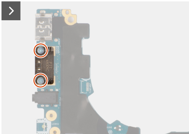
Afbeelding 52. De rechter USB Type-C-module verwijderen
