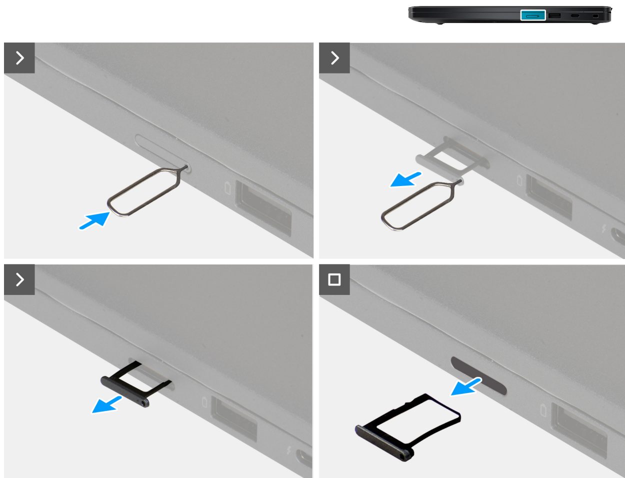
Afbeelding 10. De nanosimkaartlade verwijderen
