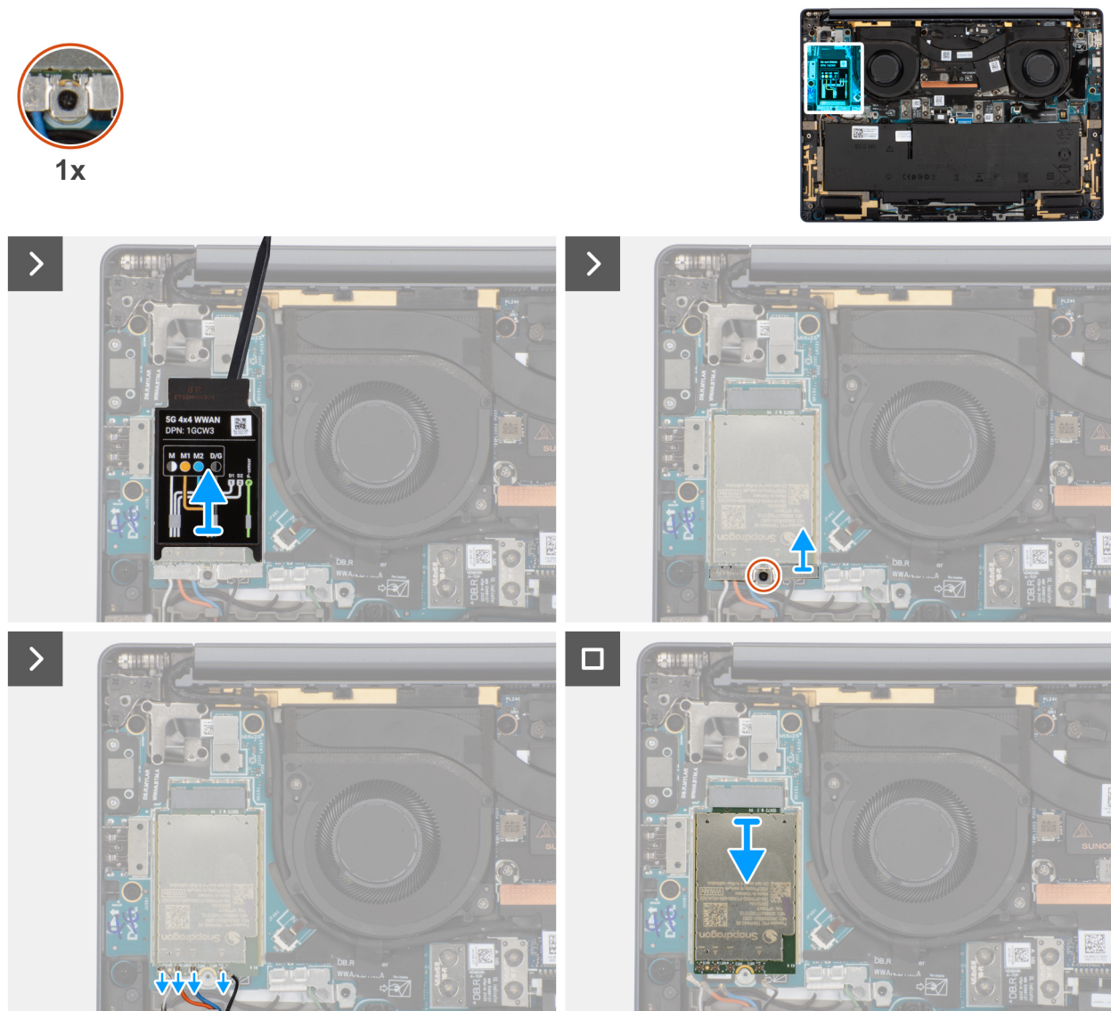
Afbeelding 26. De WWAN-kaart verwijderen
