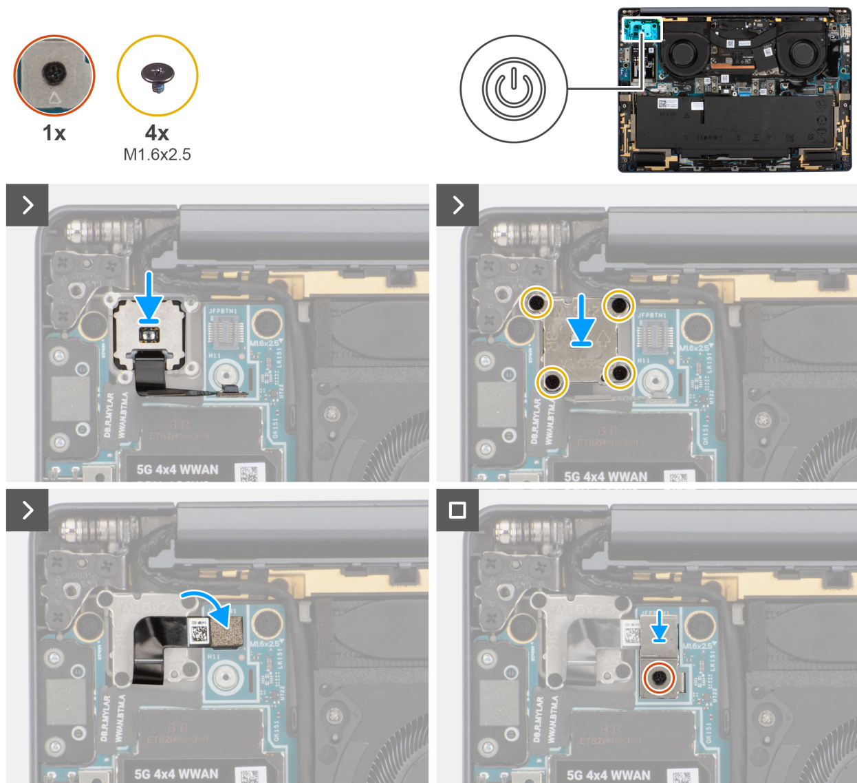
Afbeelding 55. De aan-uitknop plaatsen
