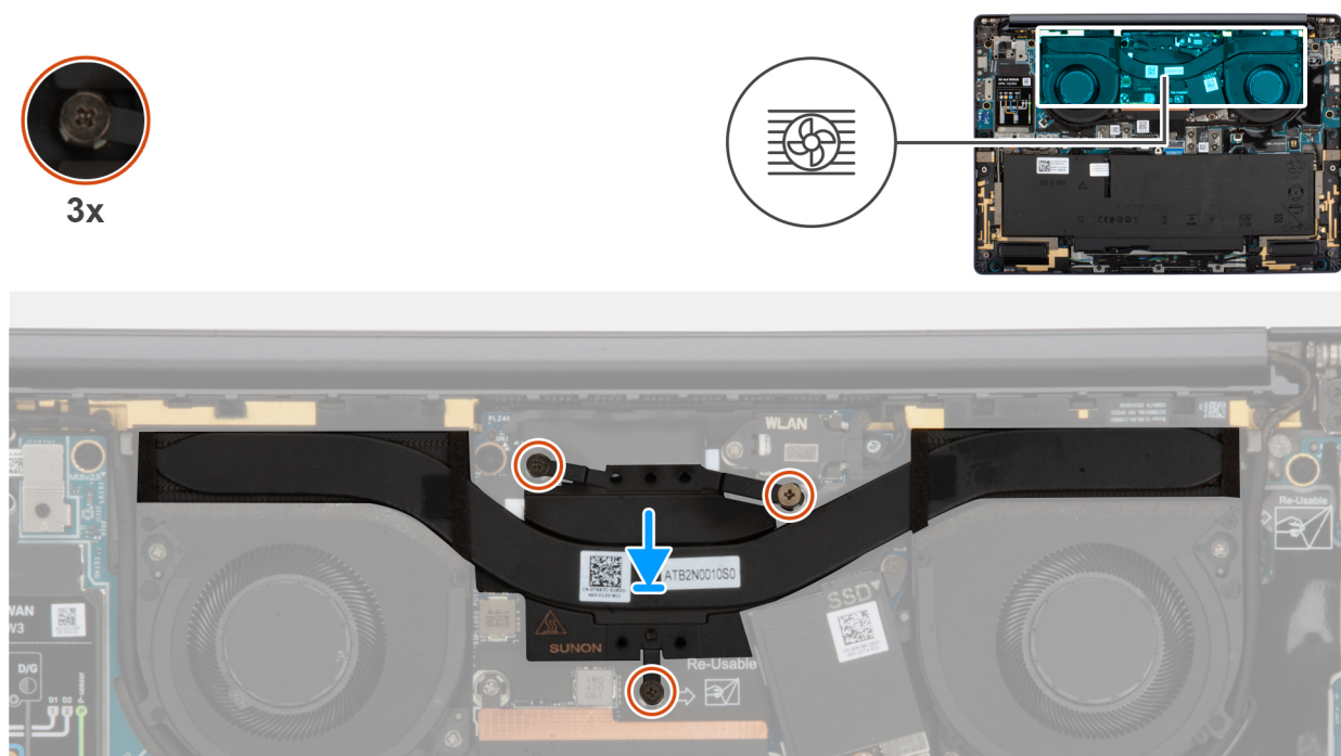
Afbeelding 37. De koelplaat plaatsen
