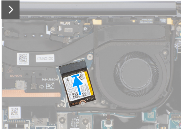
Afbeelding 25. SSD installeren
