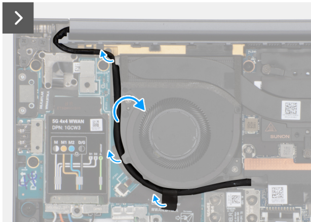
Afbeelding 30. De rechterventilator verwijderen
