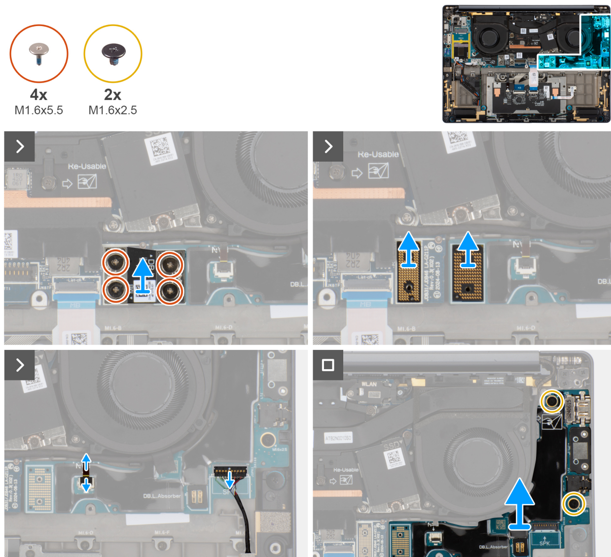
Afbeelding 38. De linker-I/O-kaart verwijderen
