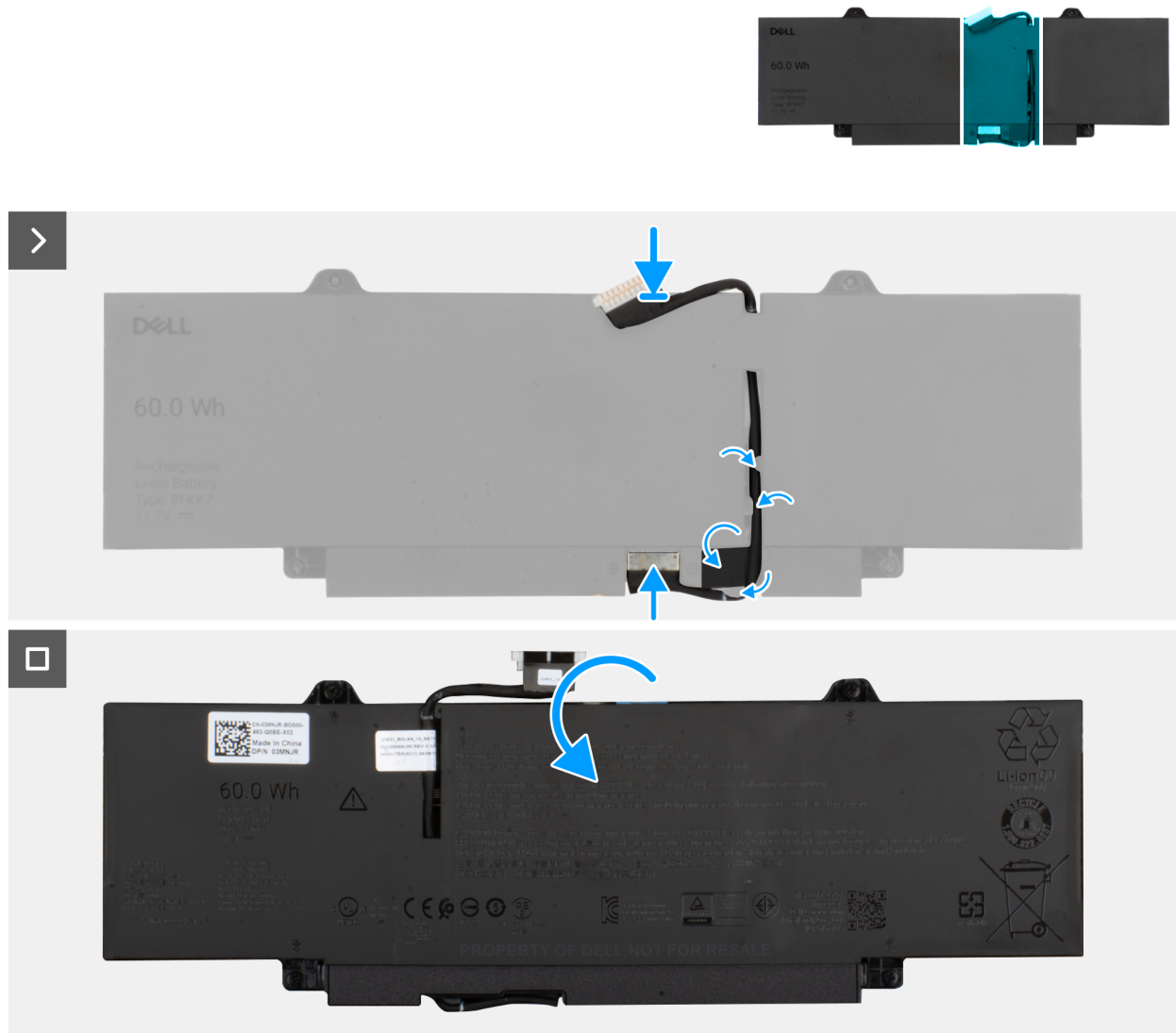
Afbeelding 23. De batterijkabel aansluiten en installeren
