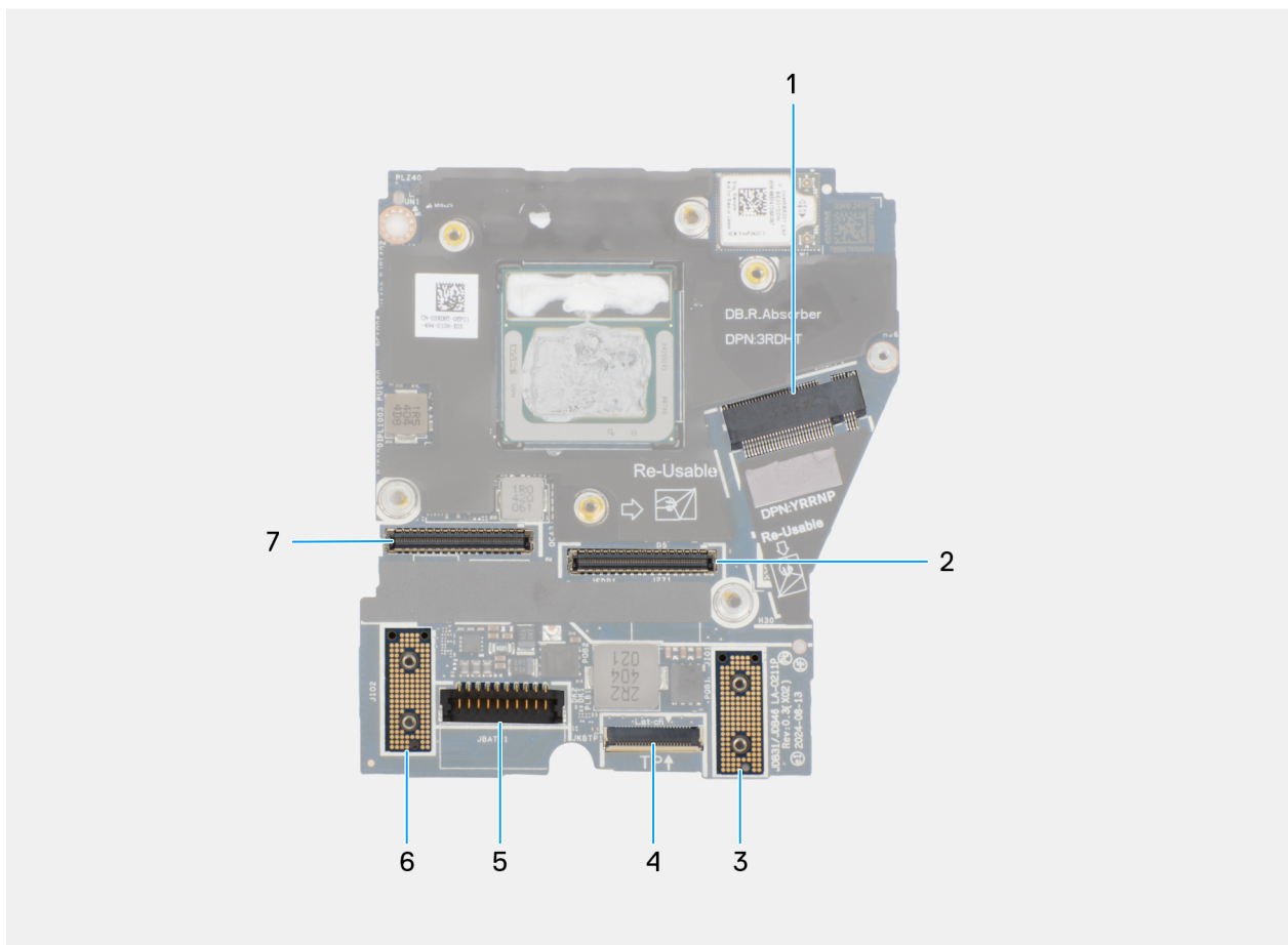
Afbeelding 61. Bijschriften voor de systeemkaart
