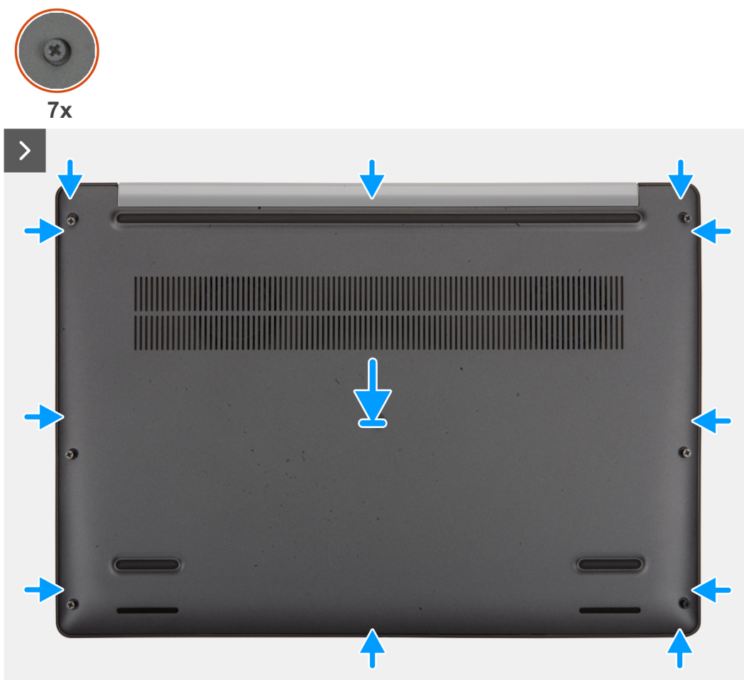
Afbeelding 18. De onderplaat plaatsen
