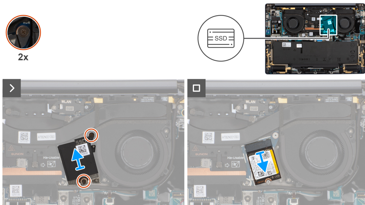
Afbeelding 24. De SSD verwijderen
