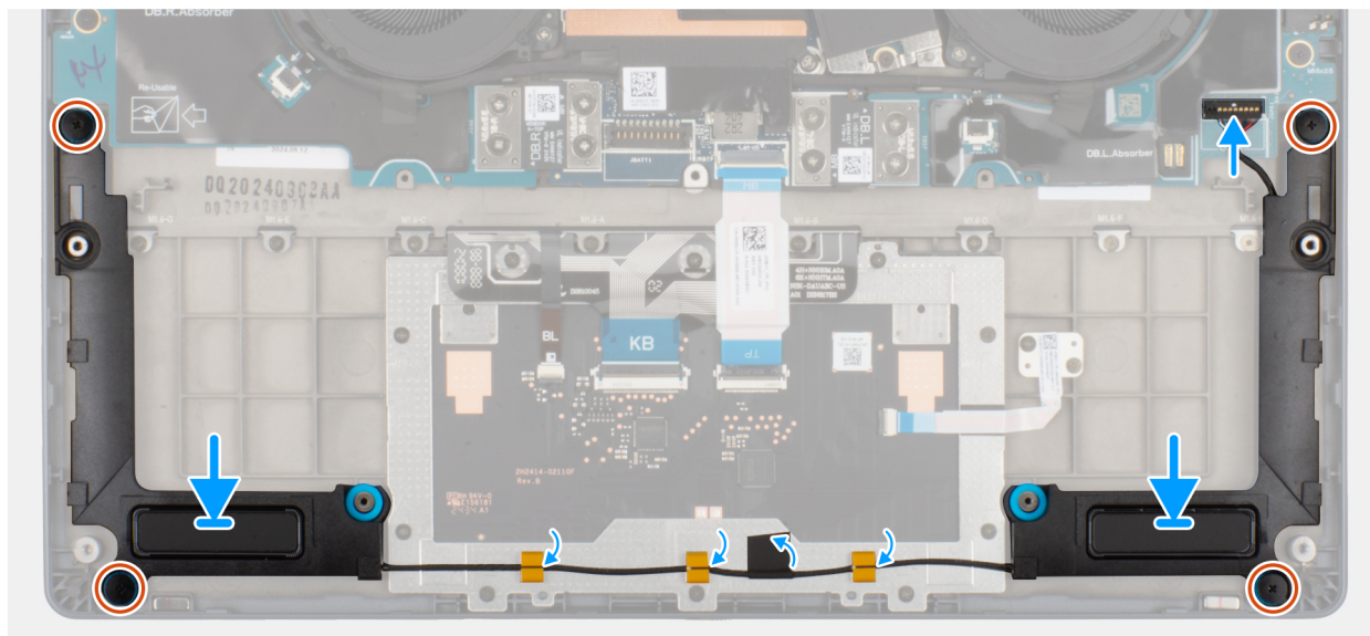
Afbeelding 33. De luidsprekers installeren (zonder WWAN)
