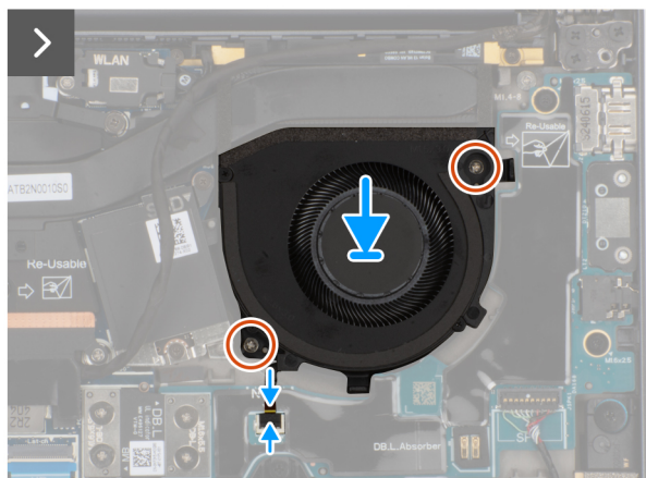
Afbeelding 29. De linkerventilator plaatsen
