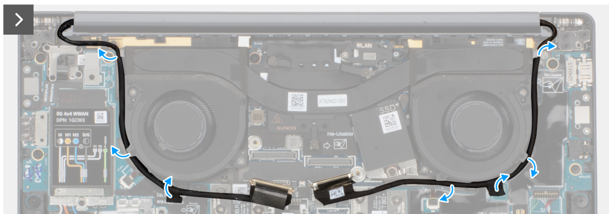
Afbeelding 56. Koppel de beeldschermkabels en de camerakabels los
