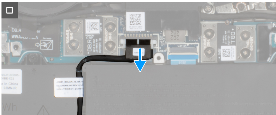
Afbeelding 16. De batterijkabel van de systeemkaart loskoppelen
