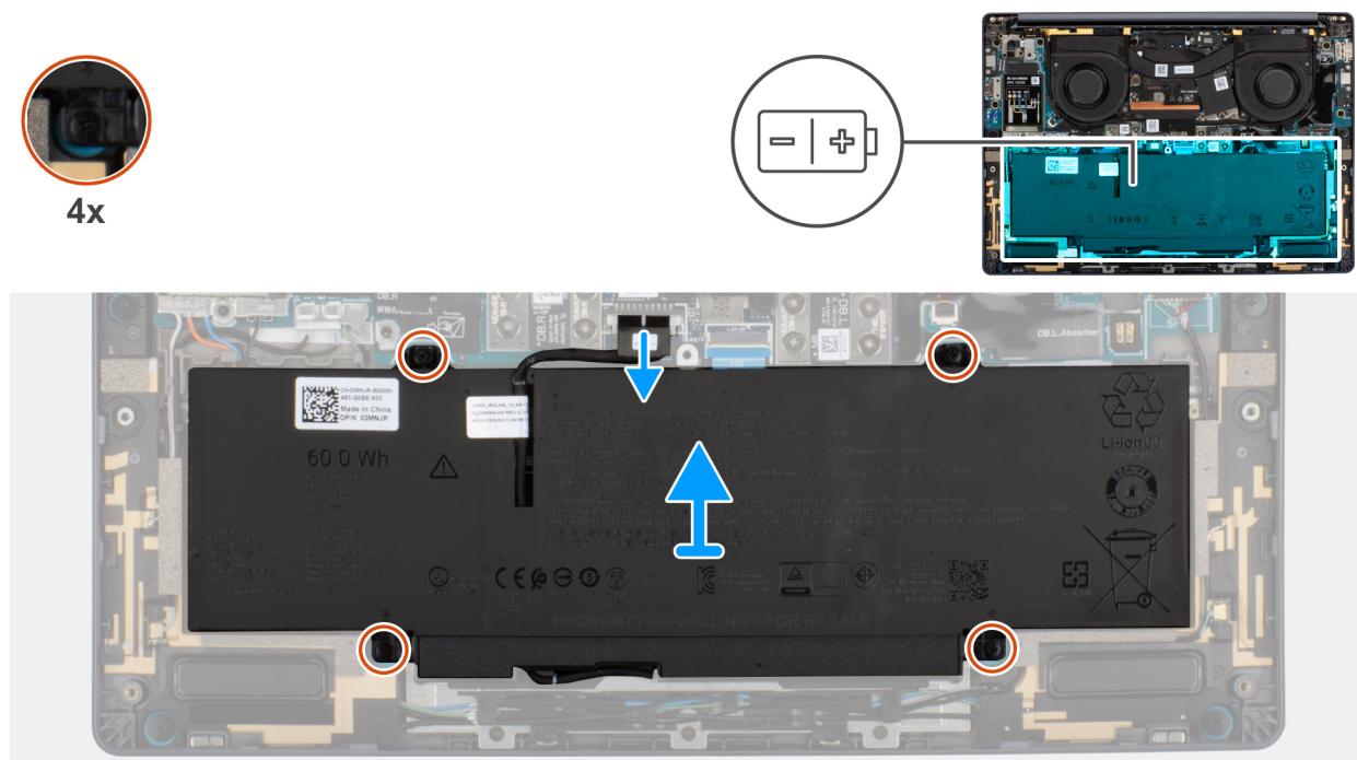
Afbeelding 20. De geborgde schroeven losdraaien
