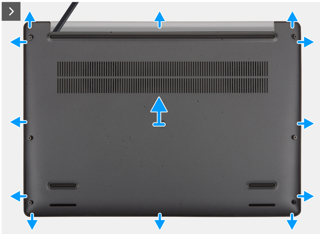
Afbeelding 15. De onderplaat verwijderen
