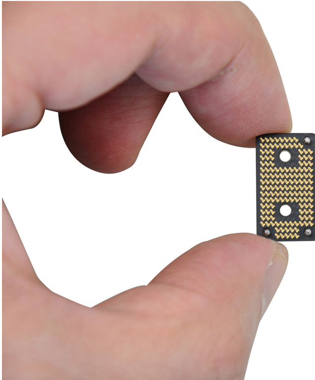
Afbeelding 39. Verwerking interposerkaart
