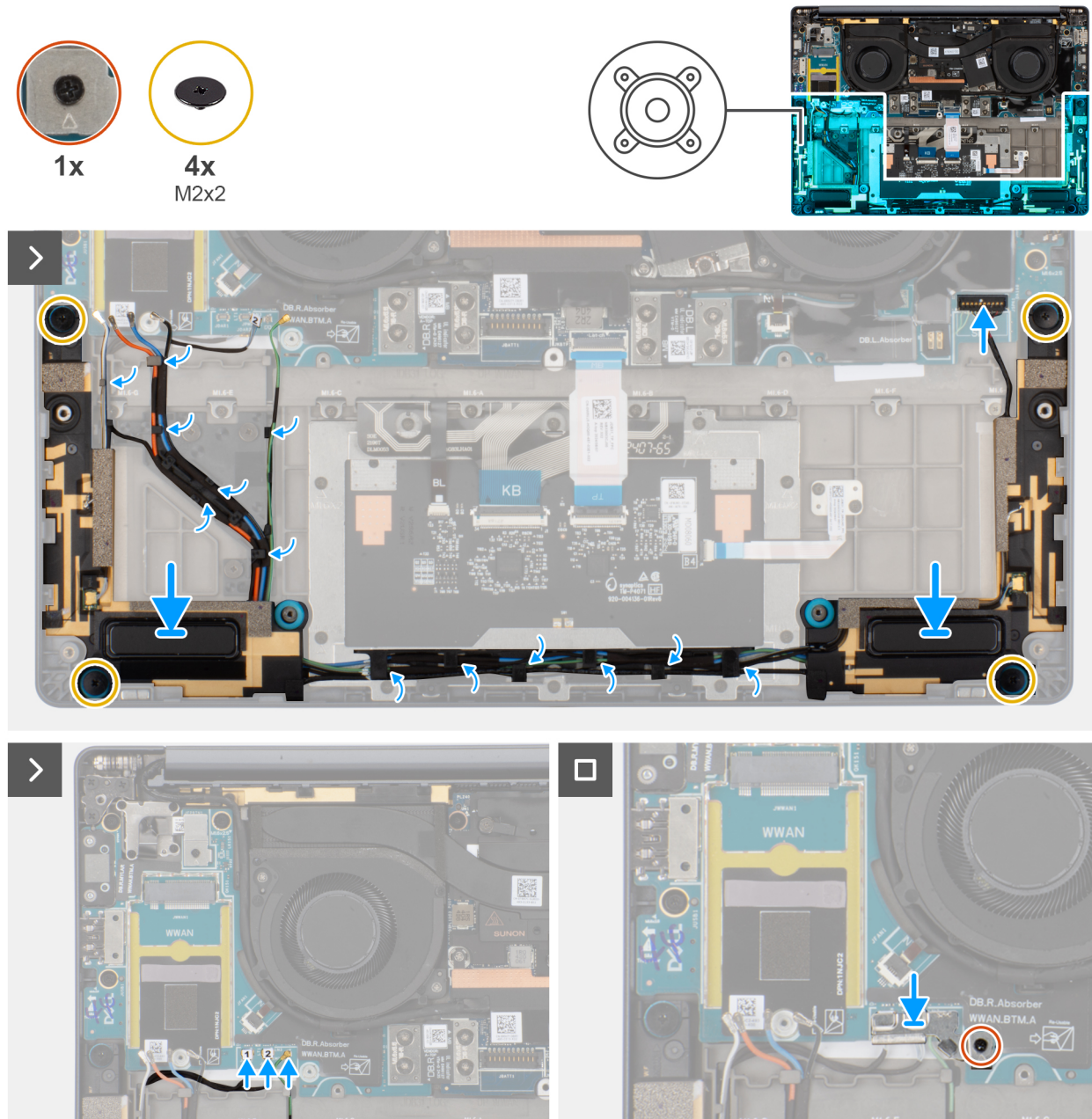
Afbeelding 35. De luidsprekers met antennes installeren (WWAN-configuratie)
