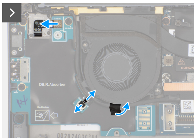
Afbeelding 42. De rechter I/O-kaart verwijderen (zonder WWAN-antennes)
