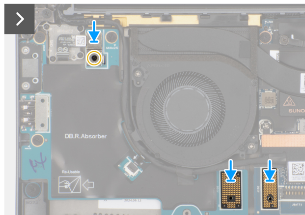
Afbeelding 44. De rechter I/O-kaart installeren (zonder WWAN-antennes)
