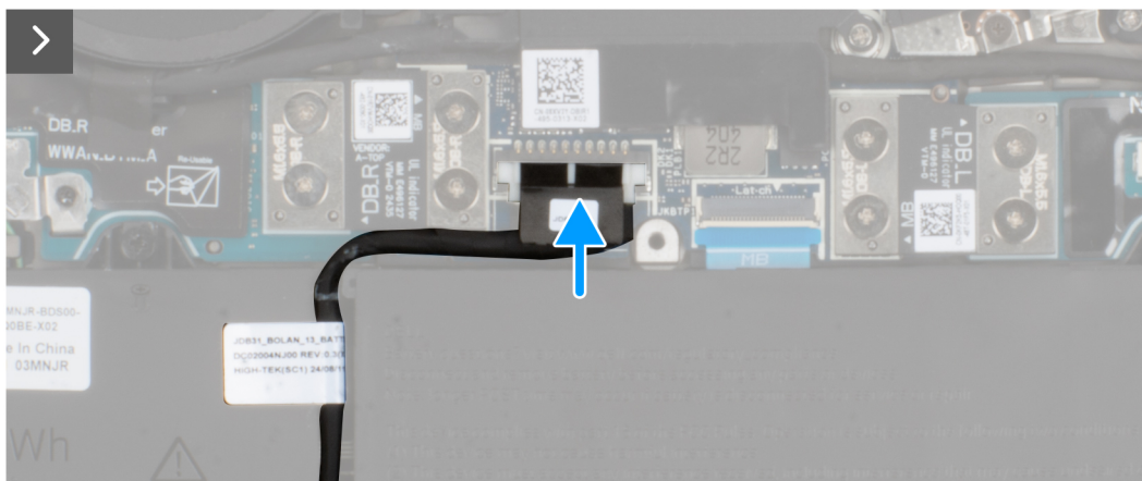
Afbeelding 17. Sluit de batterijkabel aan op de systeemkaart
