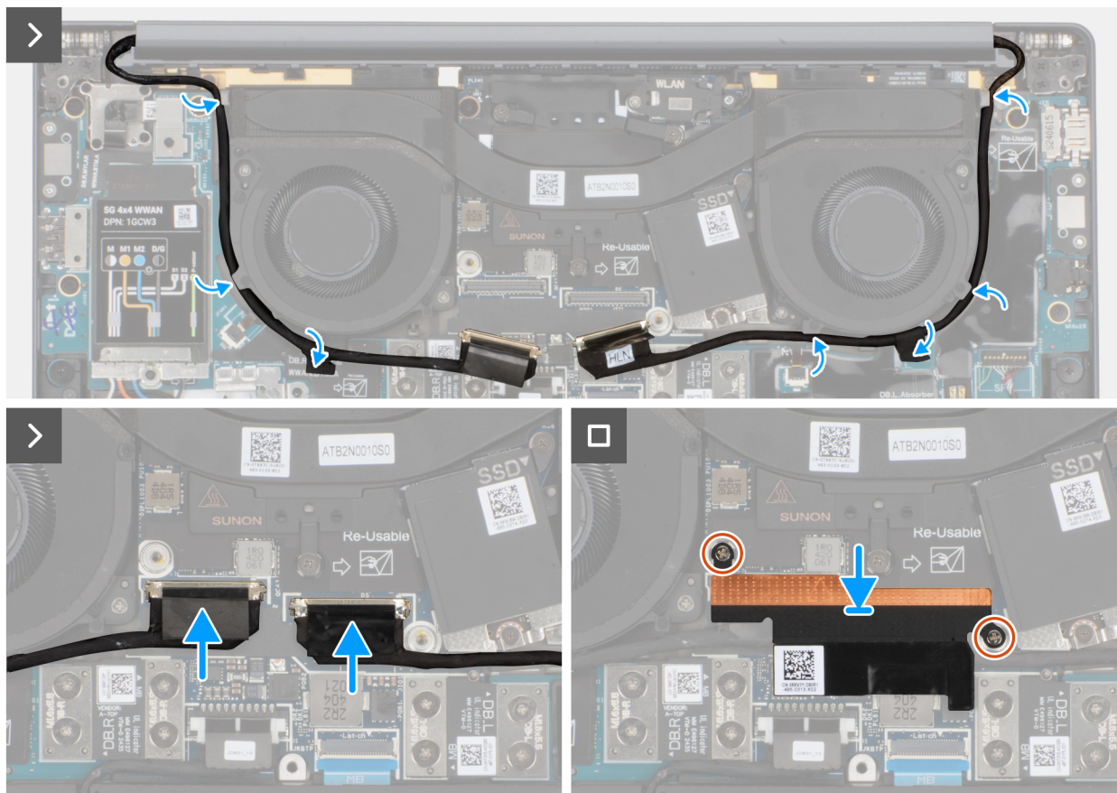
Afbeelding 60. De kabels van het beeldscherm en de camera aansluiten
