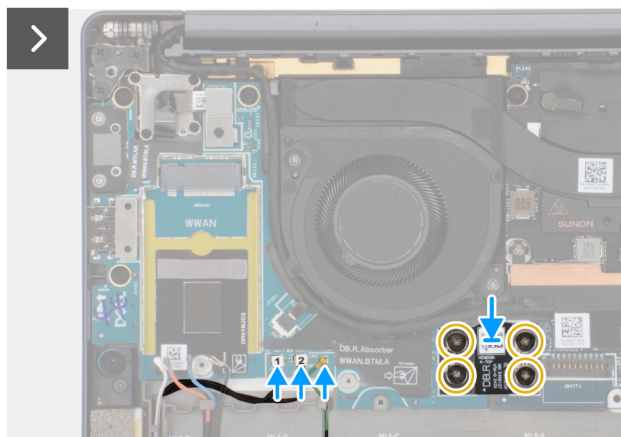
Afbeelding 48. De rechter I/O-kaart installeren (met WWAN)
