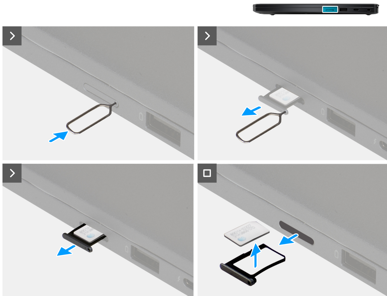
Afbeelding 12. De nano-simkaart verwijderen
