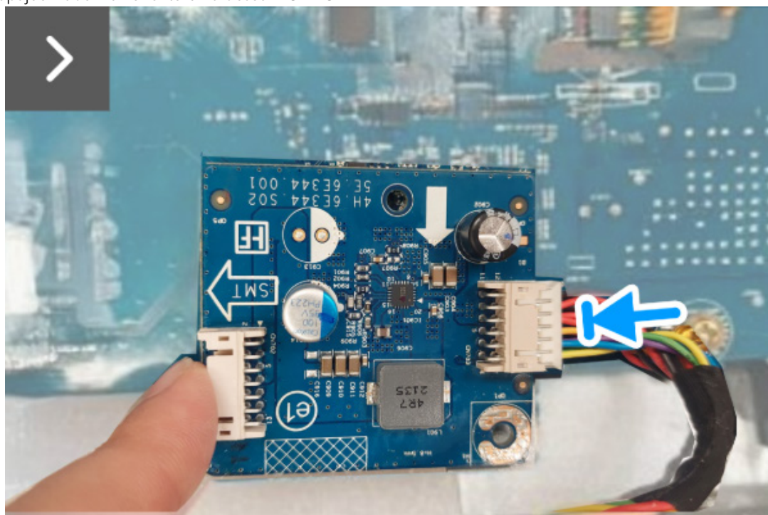
Obrázek 26. Instalace desky DC-DC
