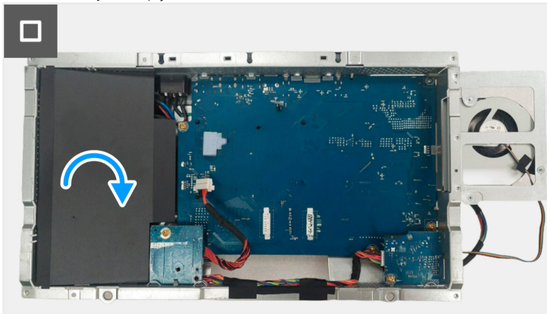
Obrázek 22. Instalace spínací desky
