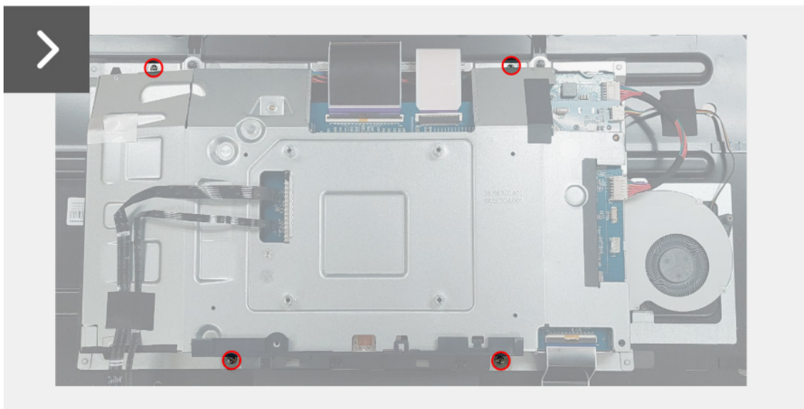
Obrázek 15. Instalace kovového štítu
