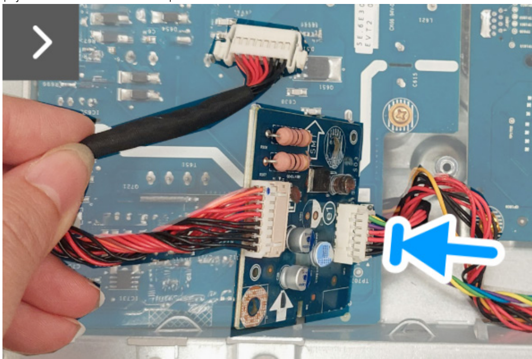
Obrázek 20. Instalace spínací desky
