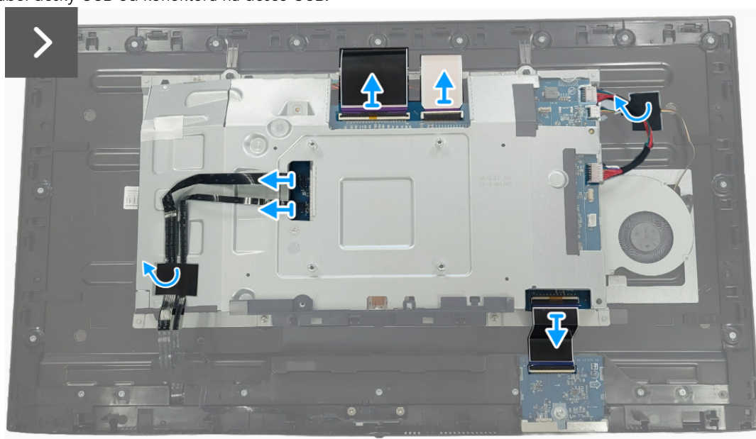
Obrázek 10. Demontáž kovového štítu
