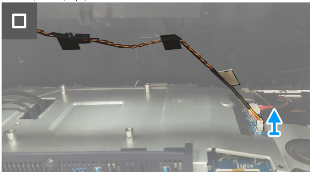
Obrázek 6. Sejmutí zadního krytu
