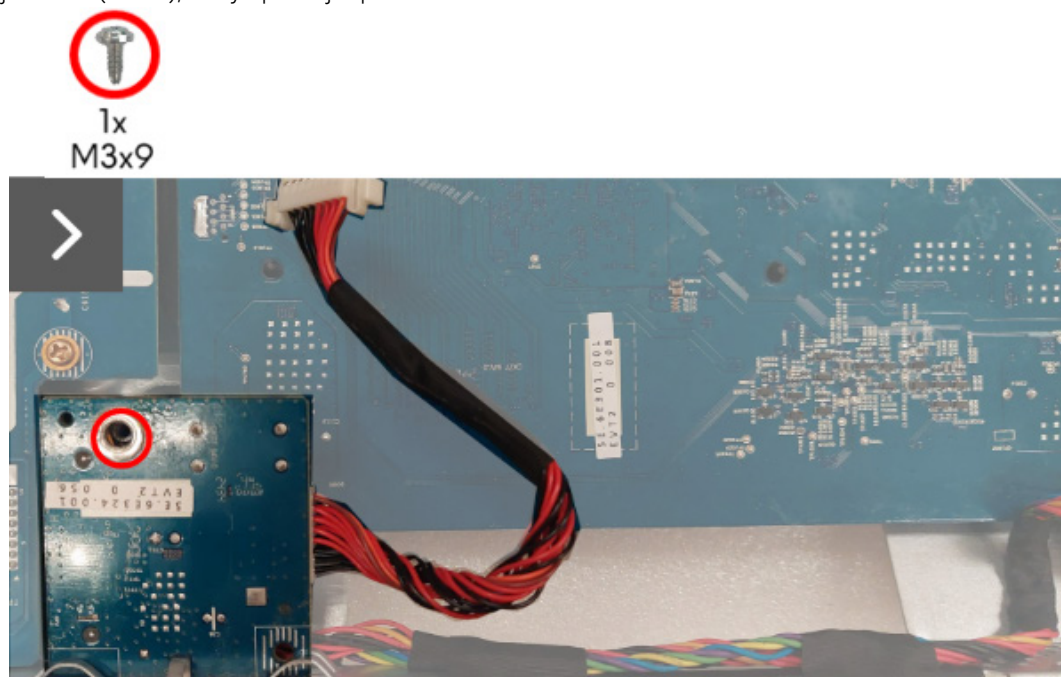
Obrázek 18. Demontáž spínací desky
