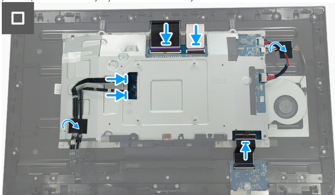
Obrázek 16. Instalace kovového štítu
