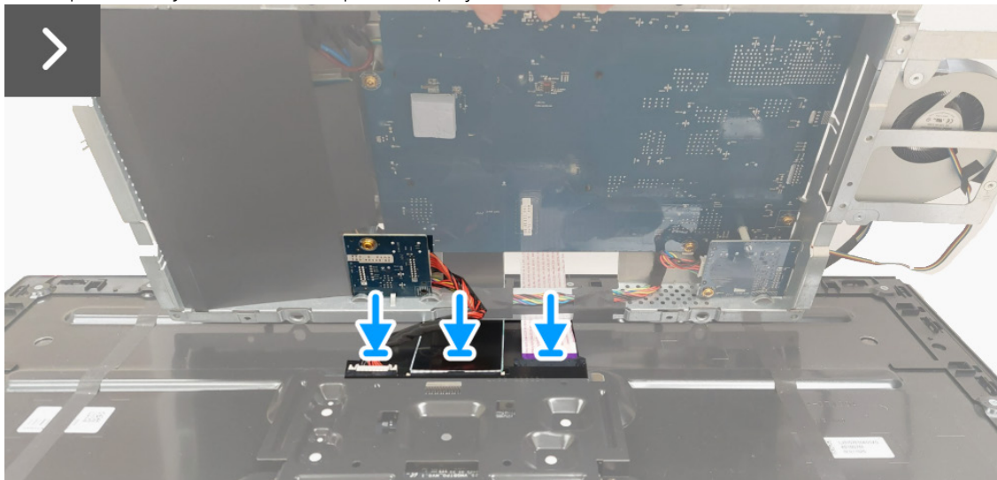
Obrázek 14. Instalace kovového štítu
