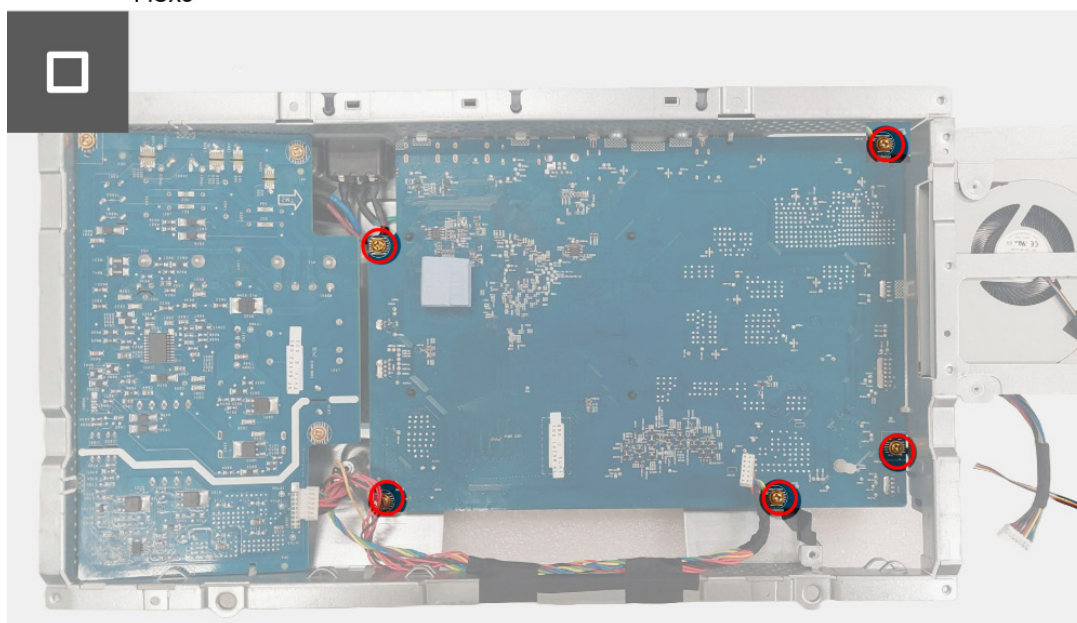
Obrázek 32. Instalace desky rozhraní
