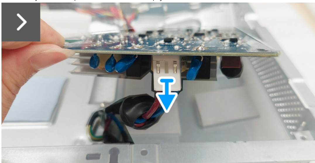
Obrázek 34. Demontáž napájecí desky
