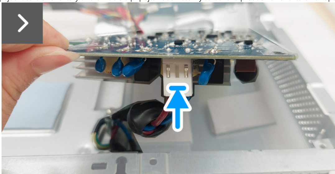
Obrázek 37. Instalace napájecí desky
