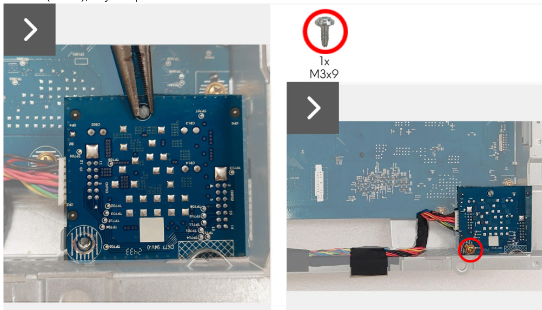
Obrázek 27. Instalace desky DC-DC
