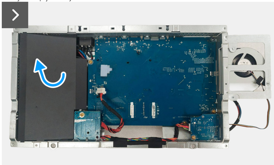
Obrázek 17. Demontáž spínací desky
