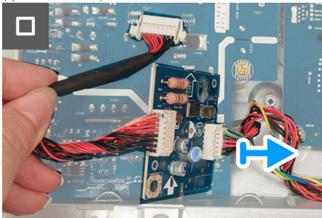
Obrázek 19. Demontáž spínací desky
