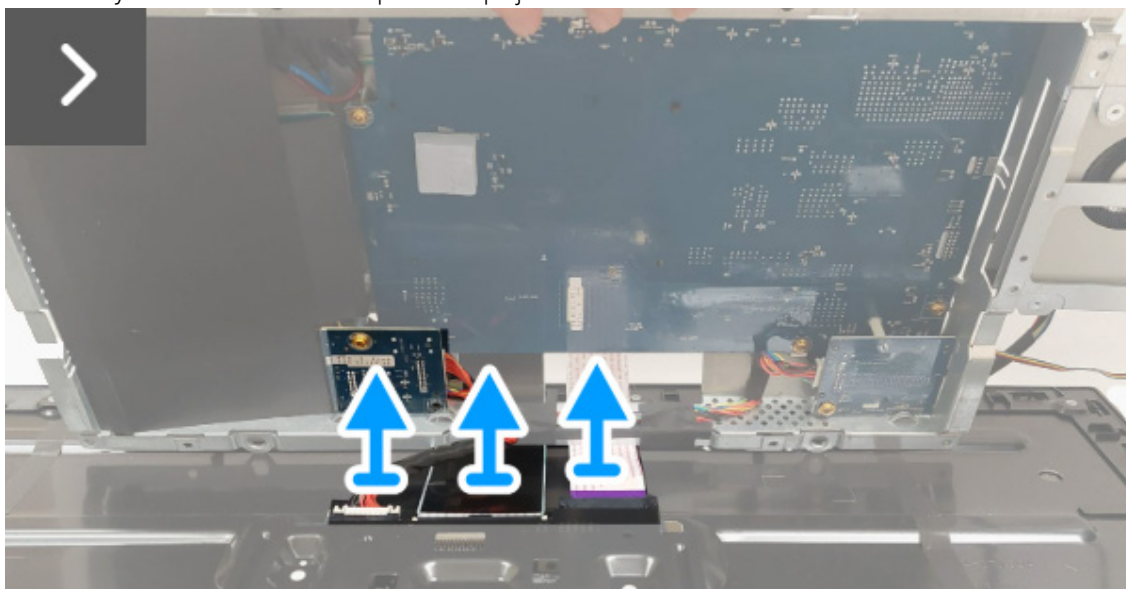
Obrázek 12. Demontáž kovového štítu
