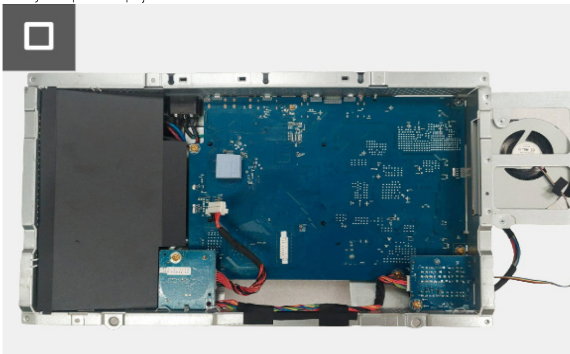
Obrázek 13. Demontáž kovového štítu
