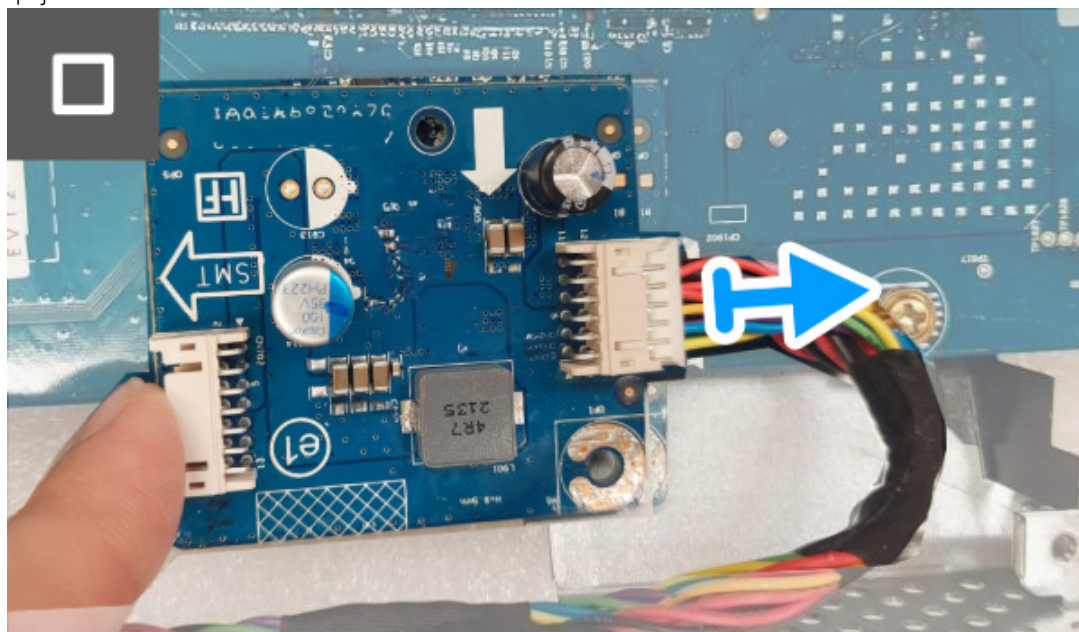
Obrázek 25. Demontáž desky DC-DC
