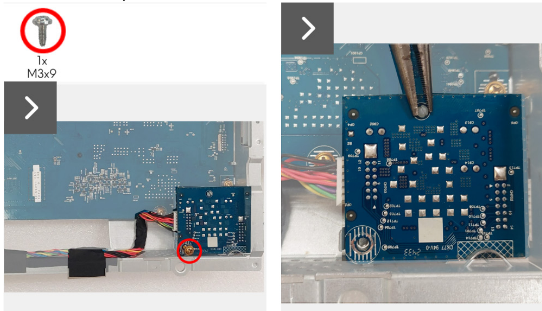
Obrázek 24. Demontáž desky DC-DC
