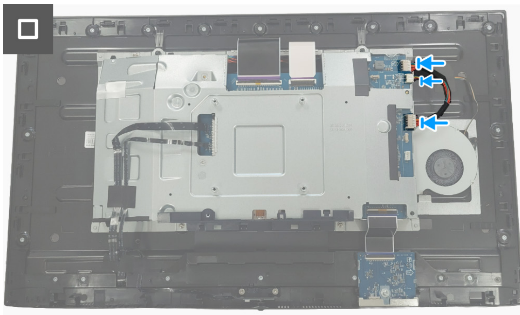
Obrázek 28. Instalace desky DC-DC
