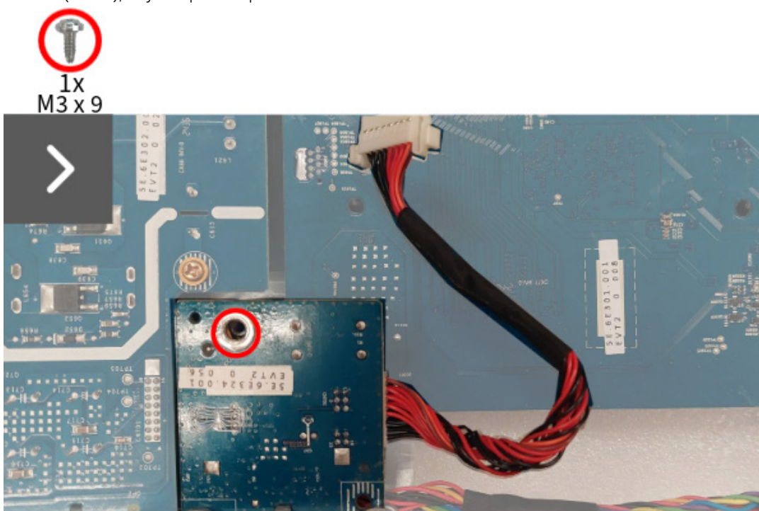
Obrázek 21. Instalace spínací desky
