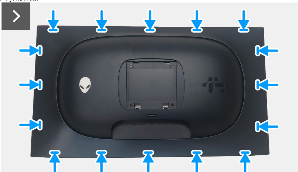
Obrázek 8. Instalace zadního krytu
