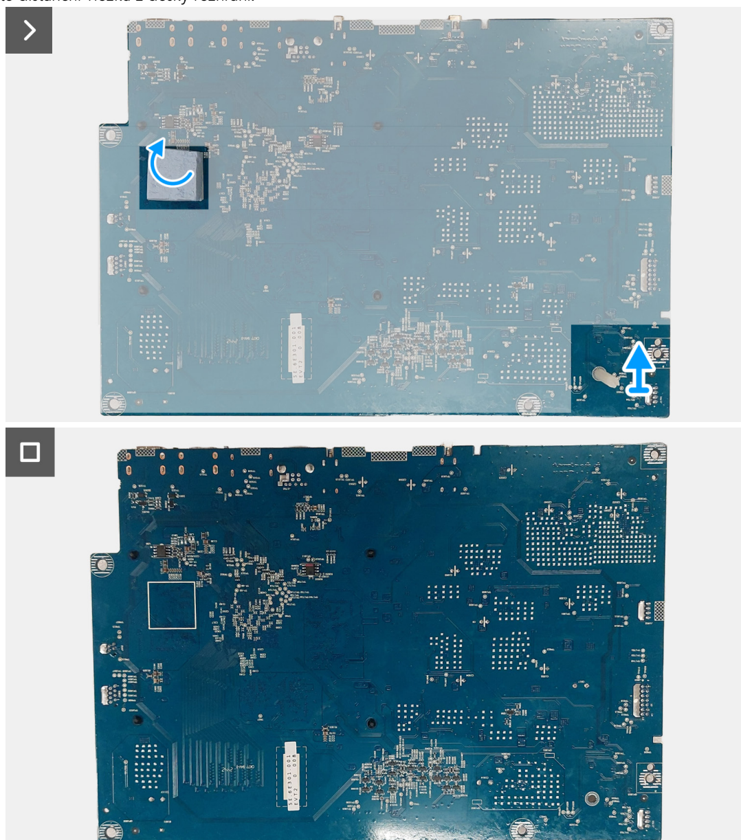
Obrázek 30. Demontáž desky rozhraní
