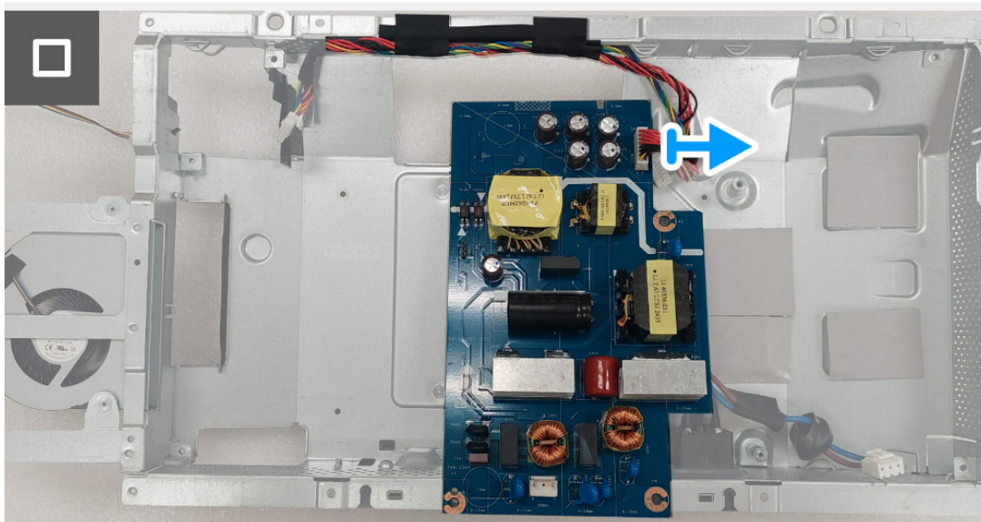
Obrázek 35. Demontáž napájecí desky
