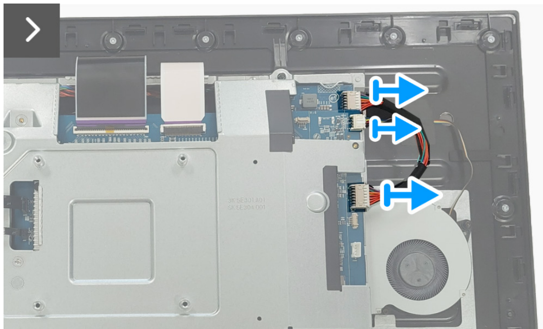
Obrázek 23. Demontáž desky DC-DC
