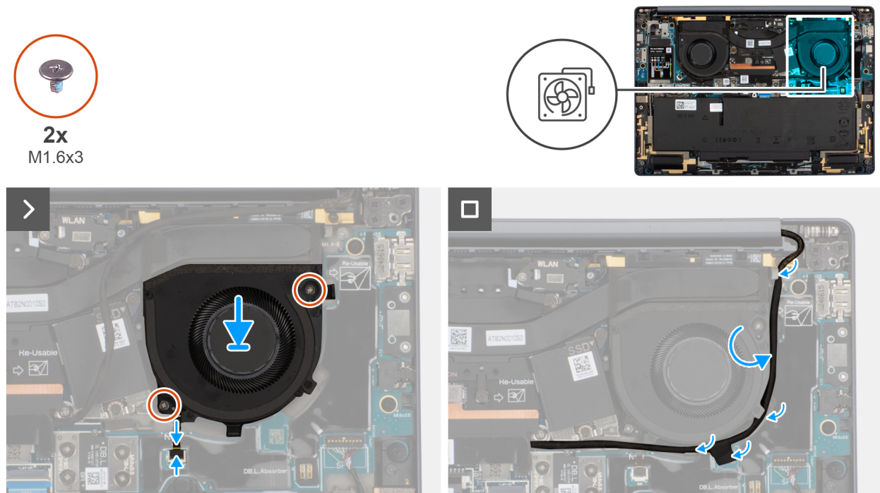
Figure 29. Installing the left fan
