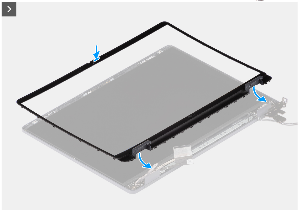
Abbildung 82. Einbauen der Bildschirmblende
