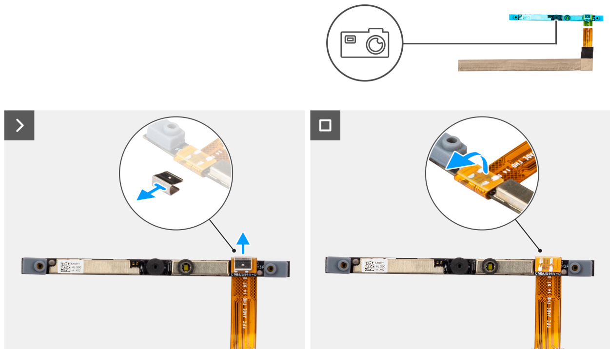
Abbildung 92. Entfernen der Kamera
