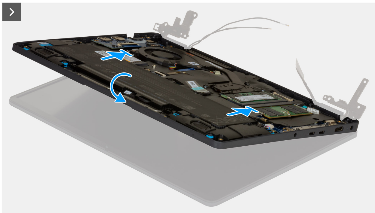
Abbildung 75. Einbauen der Displaybaugruppe
