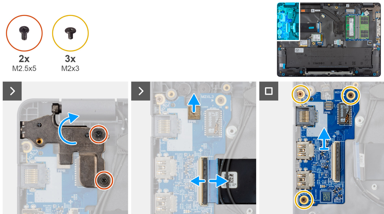
Abbildung 38. Entfernen der E/A-Platine
