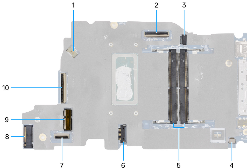
Abbildung 46. Hauptplattenanschlüsse
