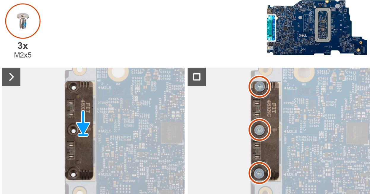
Abbildung 59. Installieren des USB-Type-C-Moduls
