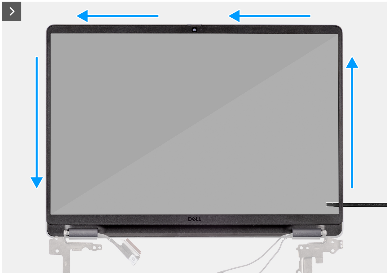
Abbildung 80. Entfernen der Bildschirmblende
