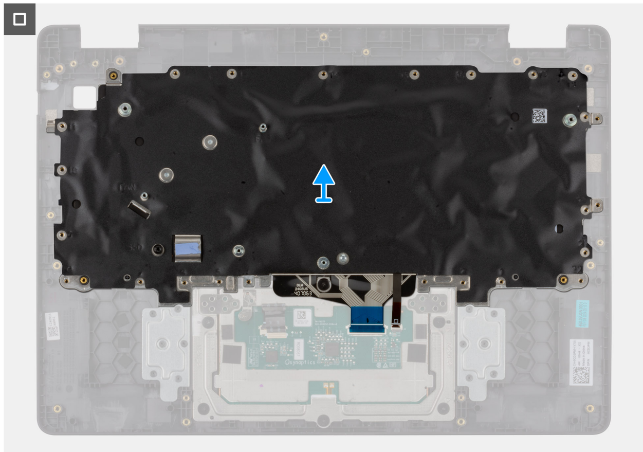
Abbildung 61. Entfernen der Tastatur
