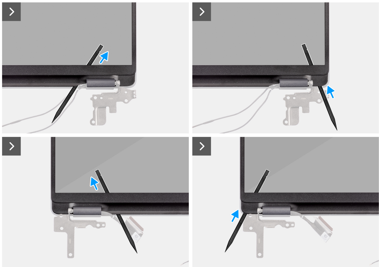
Abbildung 79. Entfernen der Bildschirmblende
