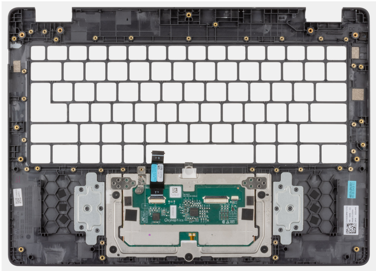
Abbildung 71. Installieren der Handauflagenbaugruppe
