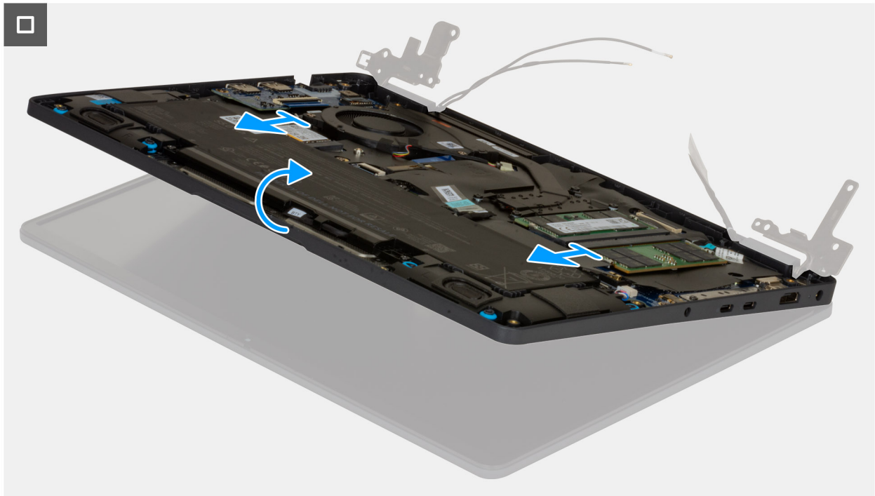
Abbildung 73. Entfernen der Bildschirmbaugruppe
