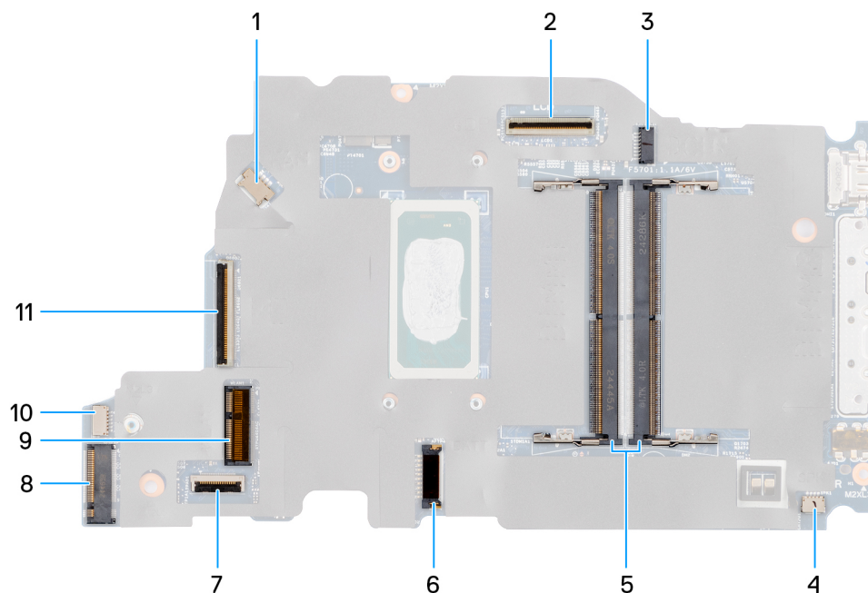
Abbildung 52. Hauptplattenanschlüsse
