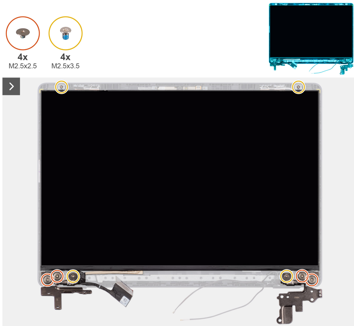
Abbildung 84. Entfernen der Bildschirmbaugruppe
