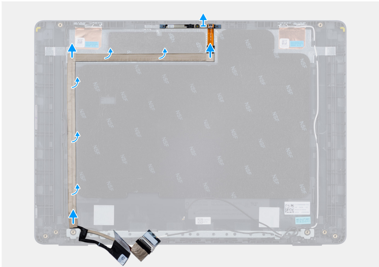
Abbildung 94. Entfernen des eDP-Kabels
