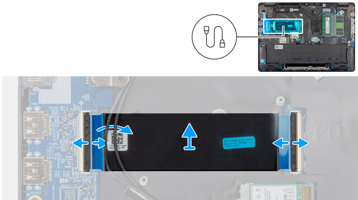
Abbildung 42. Entfernen des FPC-Kabels der I/O-Platine
