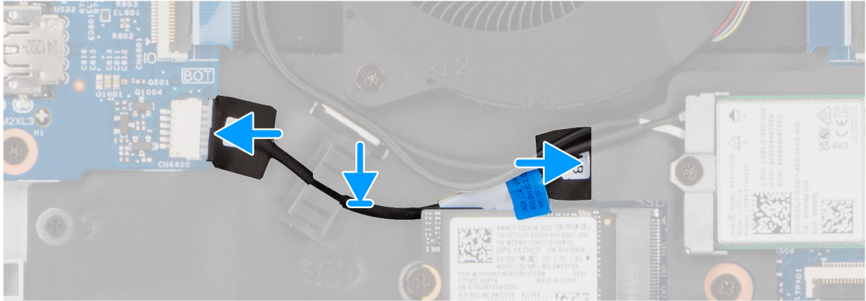
Abbildung 37. Installieren des vPro-Kabels
