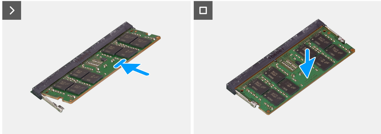
Abbildung 22. Installieren der Speichermodule
