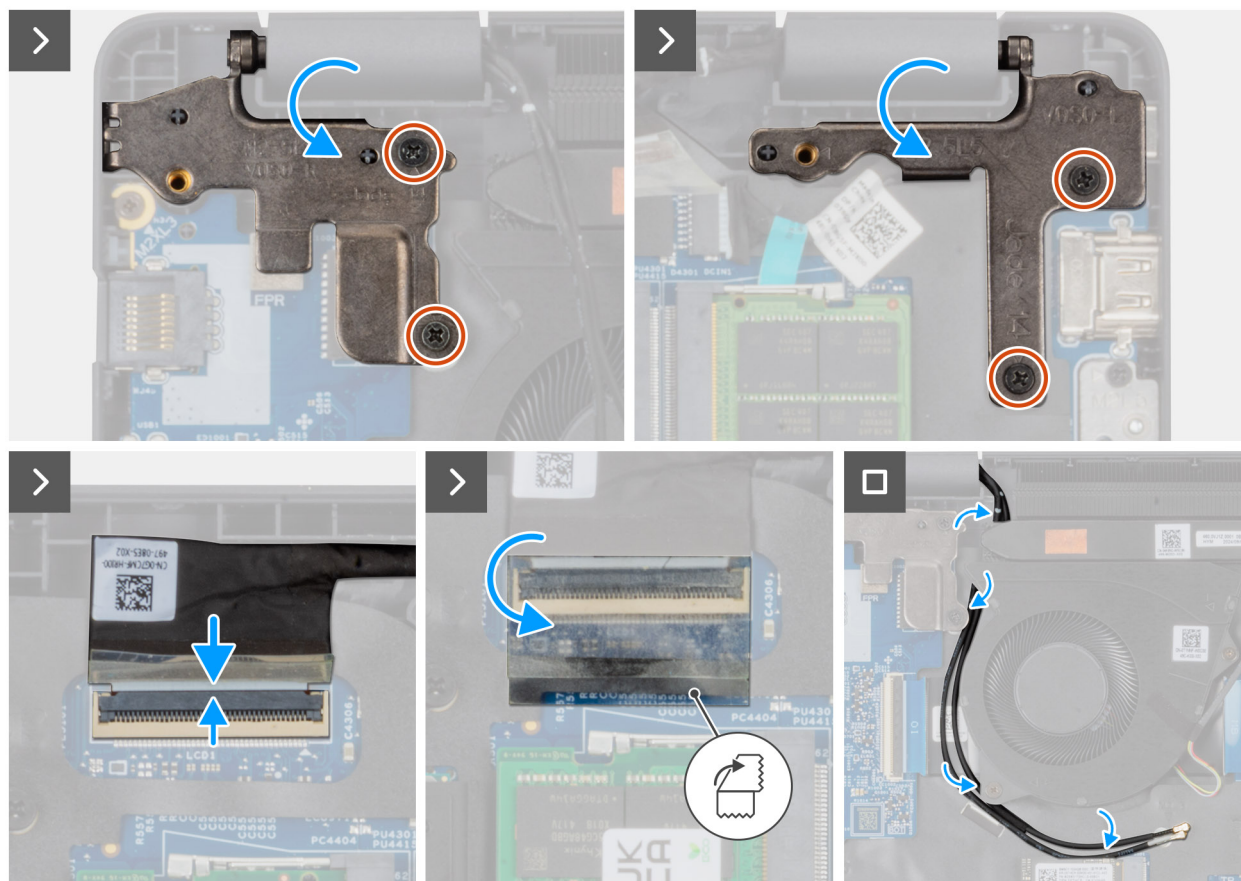
Abbildung 76. Einbauen der Displaybaugruppe
