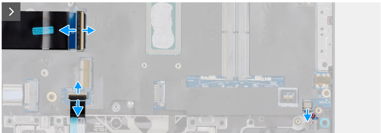
Abbildung 47. Entfernen der Systemplatine
