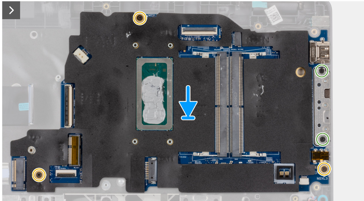
Abbildung 50. Einbauen der Systemplatine
