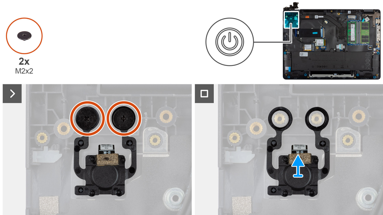
Abbildung 44. Entfernen des Netzschalters mit Fingerabdruck-Lesegerät
