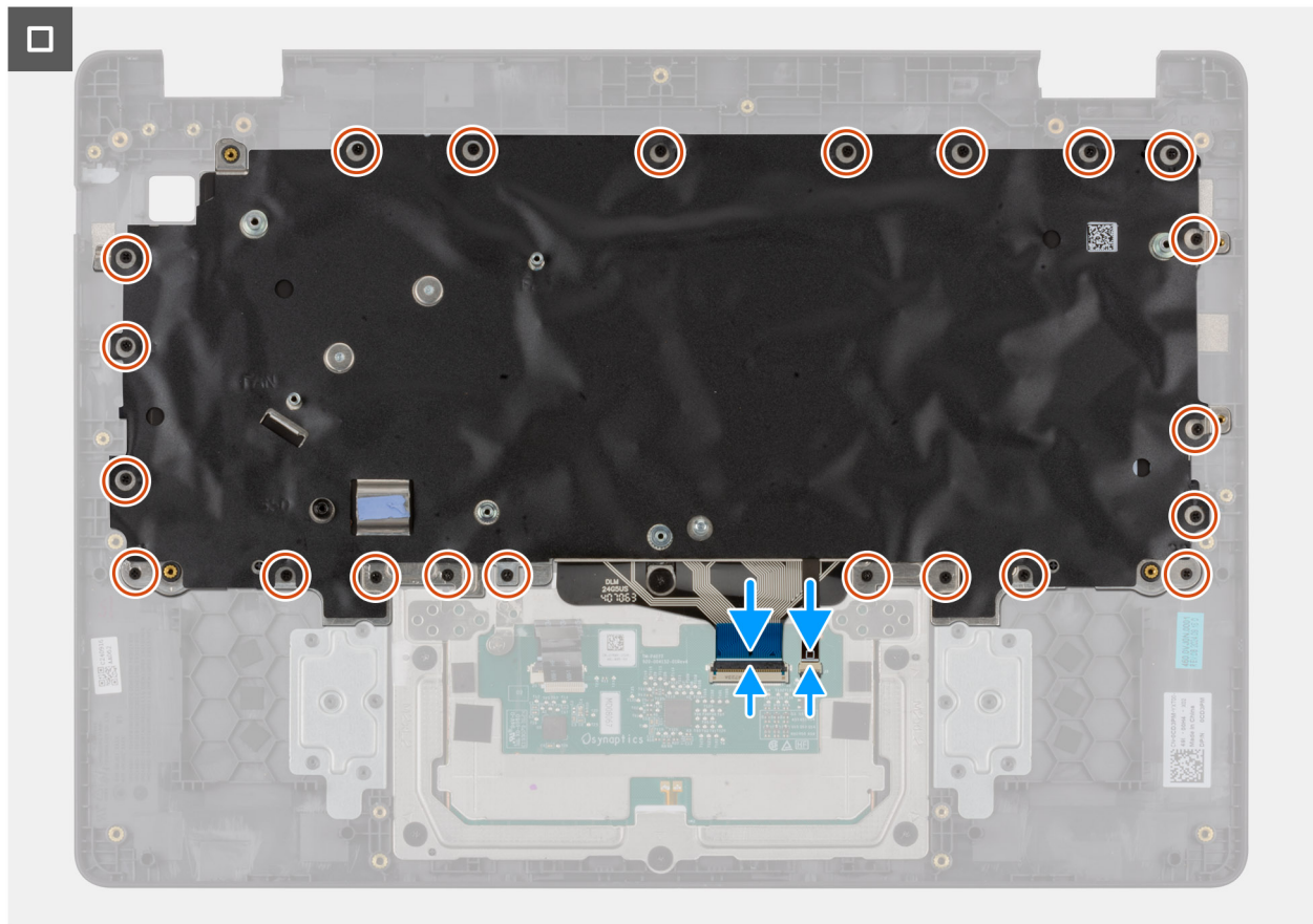
Abbildung 65. Einbauen der Tastatur
