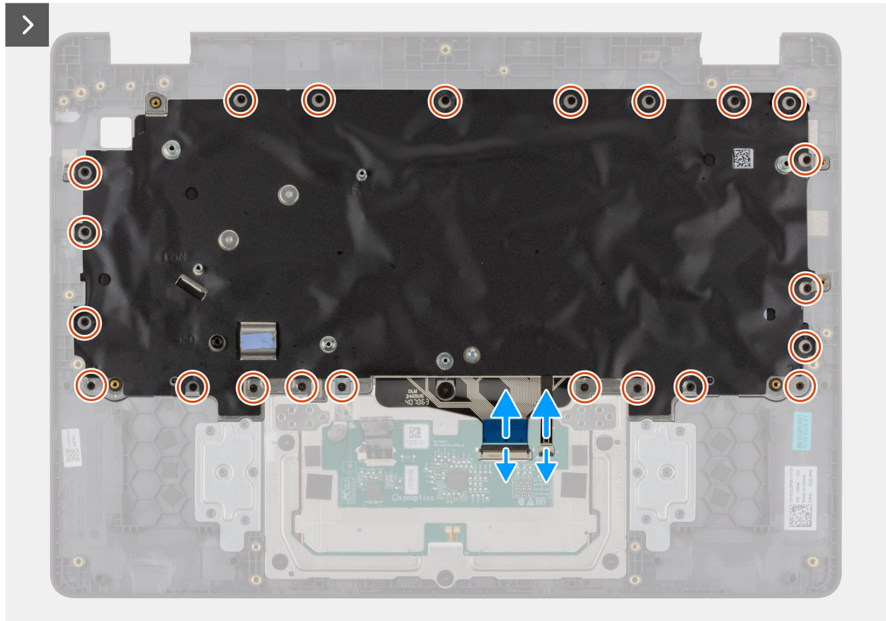
Abbildung 60. Entfernen der Tastatur
