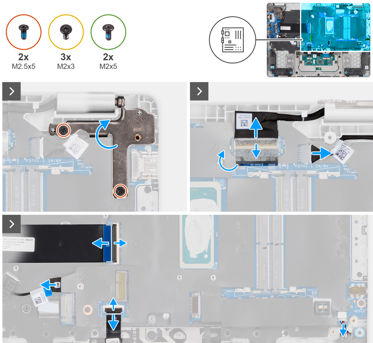
Abbildung 53. Entfernen der Systemplatine
