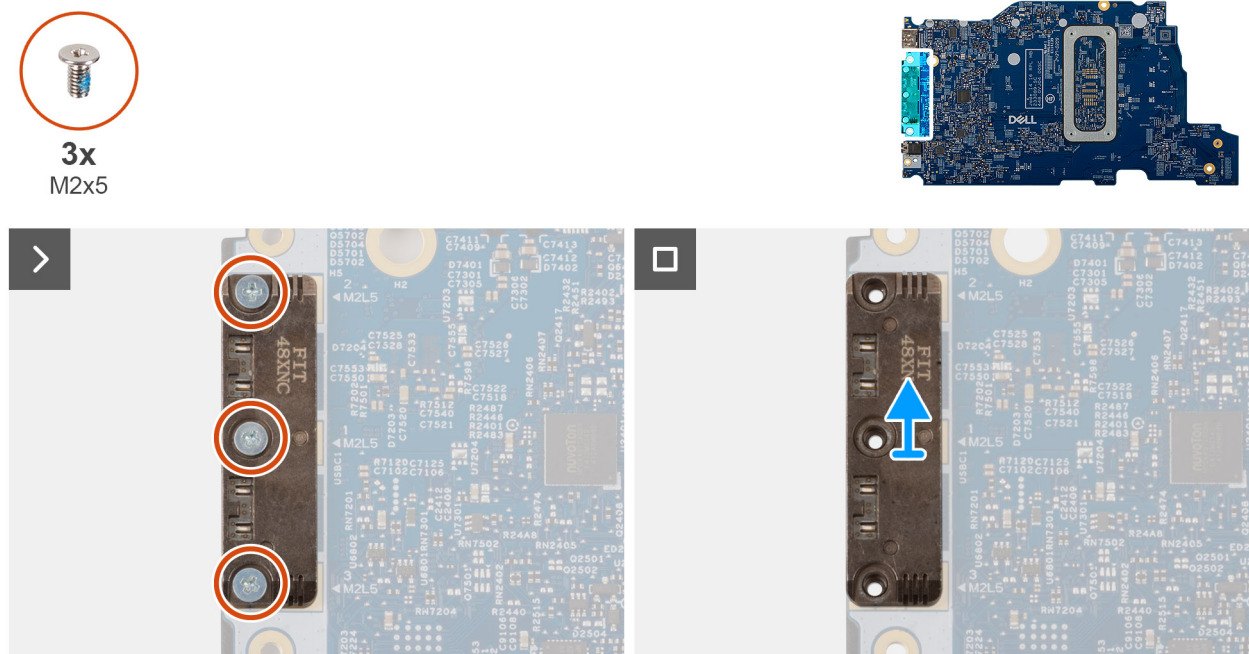
Abbildung 58. Entfernen des USB-Type-C-Moduls
