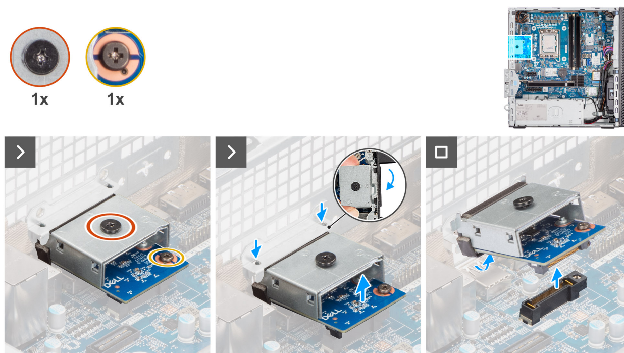
Figura 61. Rimozione del modulo VGA opzionale
