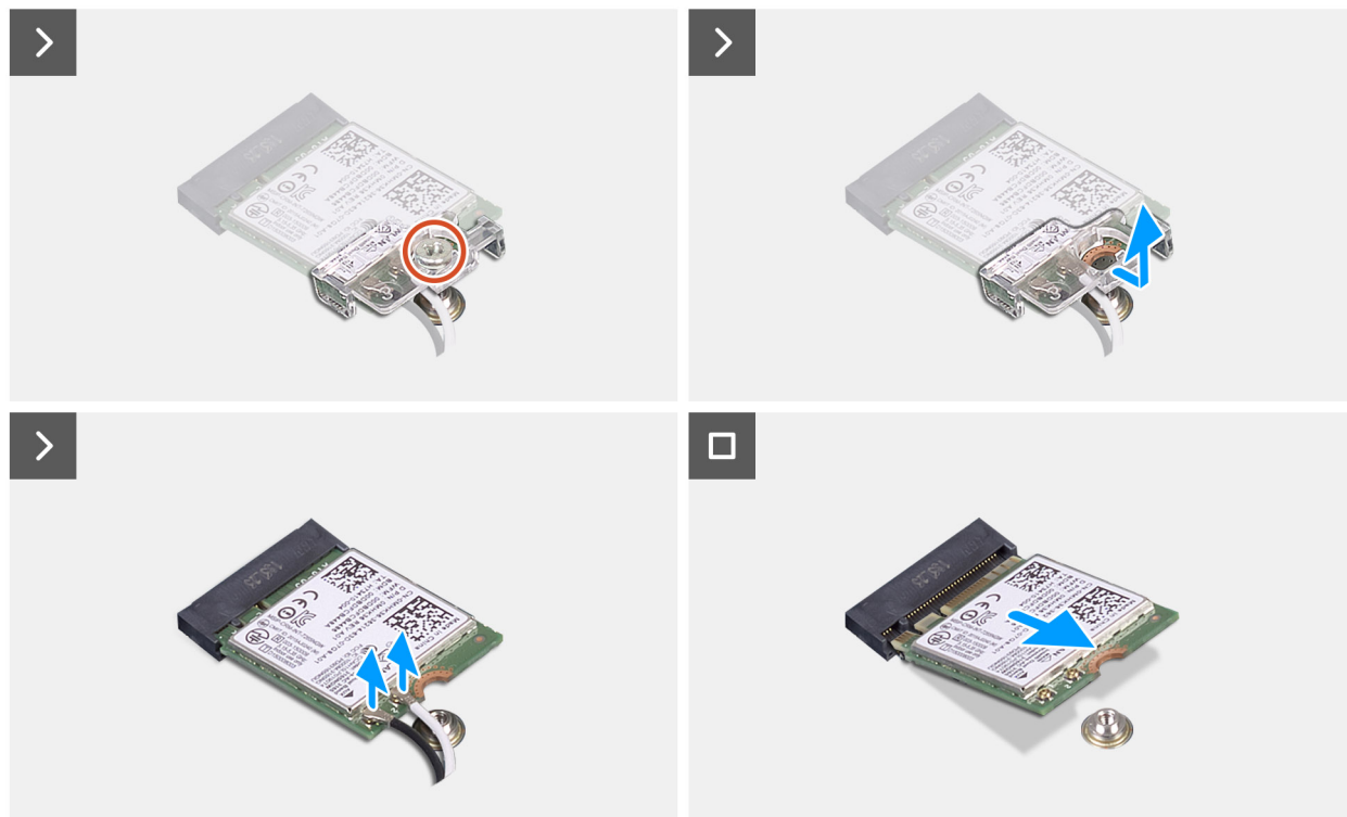
Figura 41. Rimozione della scheda wireless
